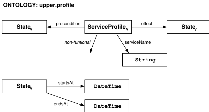
Abbildung 37: Verkürzte Darstellung der Ontologie upper.profile . Die vollständige Ontologie findet sich in Anhang A.2.
