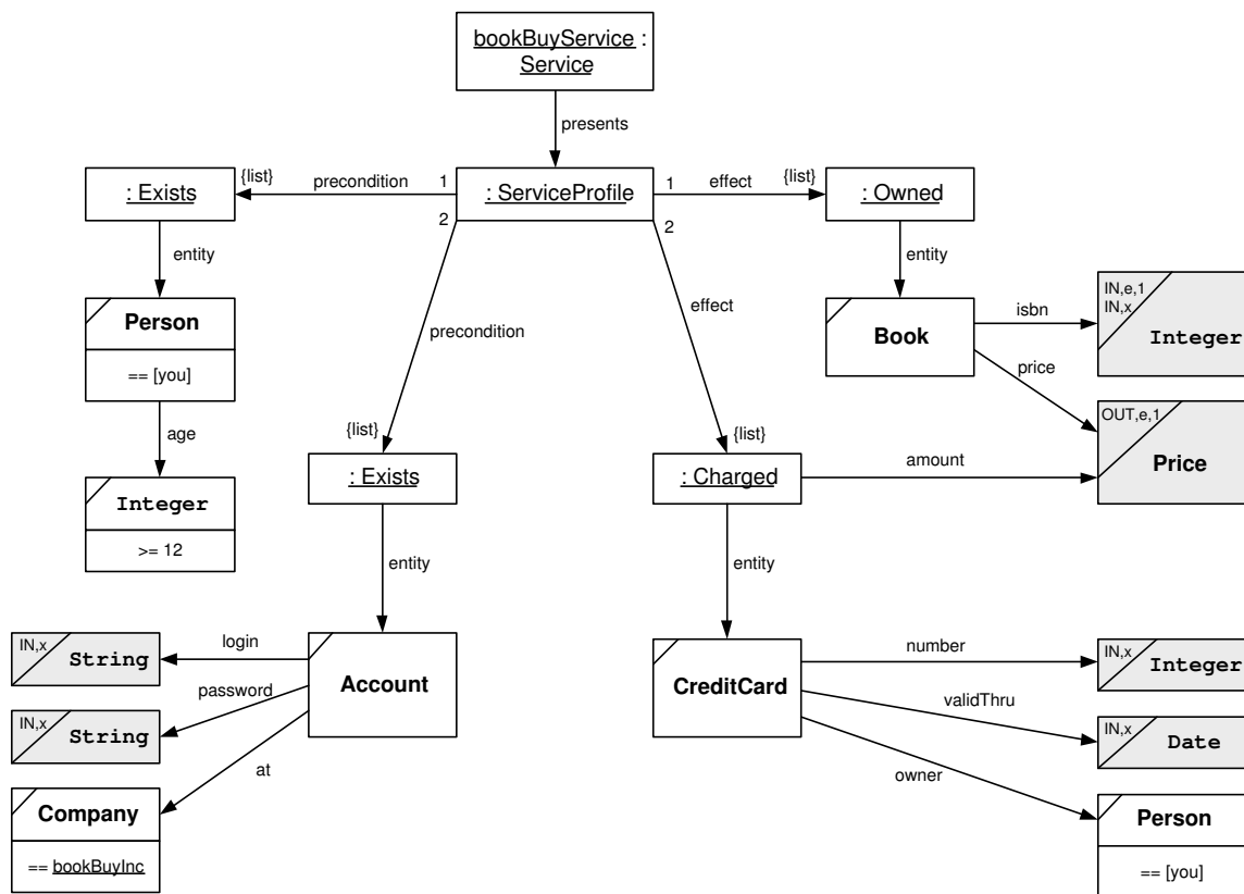
Abbildung 48: Beispielhafte Angebotsbeschreibung, die die Verwendung von Vorbedingungen in DSD illustriert.
