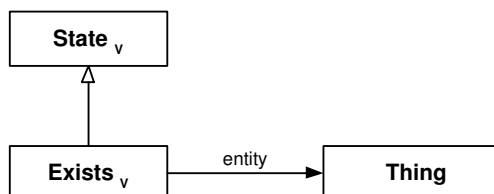
Abbildung 47: Zustand Exists aus der Ontologie upper.profile
