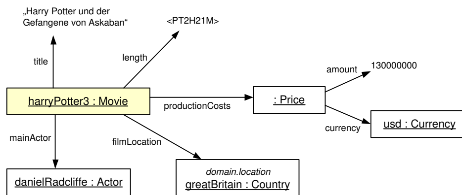
Abbildung 15: Ausfüllen von Attributen in g-dsd.
