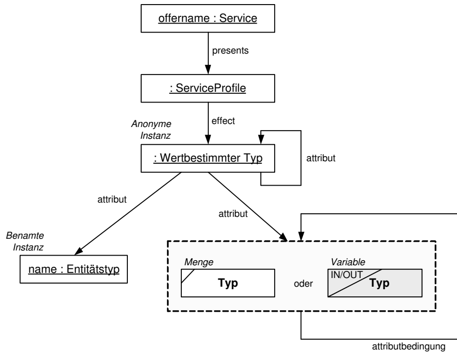
Abbildung 34: Genereller Aufbau von Angebotsbeschreibungen.
