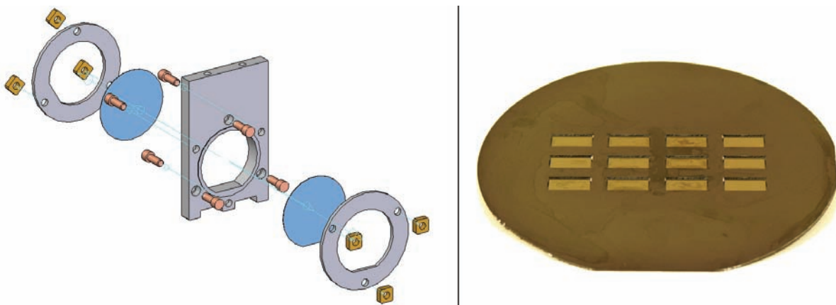
Abb. A-2 Ätzen von Silizium. Links: Explosionszeichnung der Ätzhalterung zum Freiätzen der Si 3 N 4 -Membran, der Grundkörper und die Ringe bestehen aus PTFE, die Schrauben und Muttern aus PVDF. Rechts: Ansicht der Maske mit 12 freigeätzten Fenstern von je 6 x 12 mm 2 .
