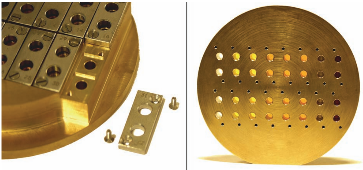
Abb. A-1 Filterhalter für Experimente zur Abtragsbestimmung. Links: Detailansicht der Vorderseite mit einem der 16 Stahlrähmchen in demontiertem Zustand. Rechts: Rückansicht des bestückten Filterhalters.
