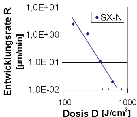
Abb. 2-8 Entwicklungsrates R als Funktion der abgelagerten Dosis für das in negativem Ton arbei- tende Resistsystem AllResist AR SX-N 4400, Entwicklung bei Raumtemperatur. Die Proben wurden an ANKA Litho3 bestrahlt und mit einem Profilometer vermessen.
