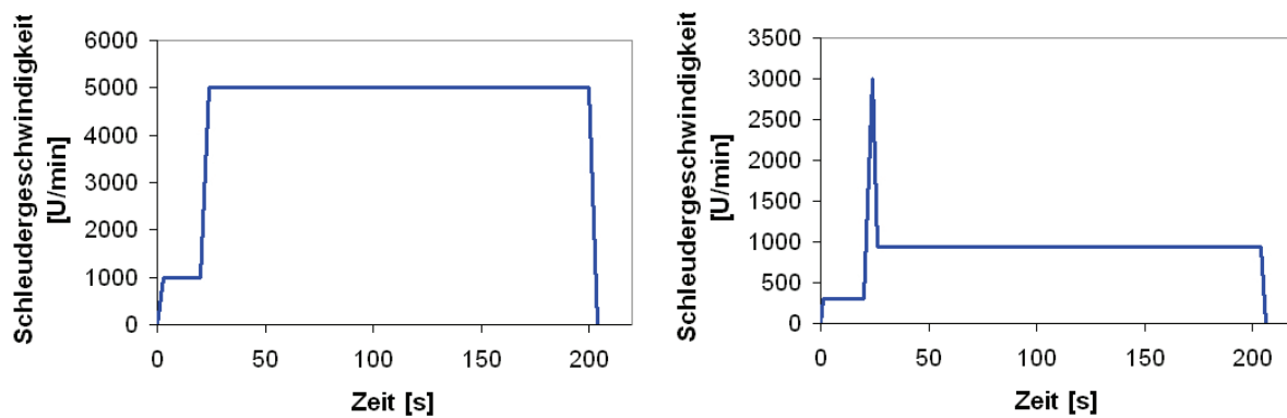
Abb. 3-10 Belackungskurven für Experimentalresist zur Belackung von 100 mm Wafern. Links: Kurve zur Belackung mit AllResist AR SX-P 6510.14. Rechts: Kurve zur Belackung mit AllResist SX-N 4400/33.1.
