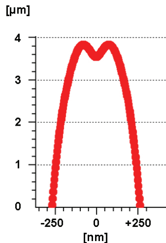
Abb. 3-28 Ergebnis der Simulation des Einflusses von Beugungseffekten bei der Bestrahlung von langen Wänden in PMMA-Resist (Schnittansicht). Probe von 4 \mu\text{m} Höhe, Bestrahlungsdosis 0,87 \text{kJ}/\text{cm}^3 mit Proximityabstand 90 \mu\text{m} und Absorberbreite von 550 nm. Die Grafik zeigt den Schnitt durch eine Wand nach 1510 min GG-Entwicklung. Die zentrale Vertiefung ist die Folge von Beugungseffekten [Nazm00].
