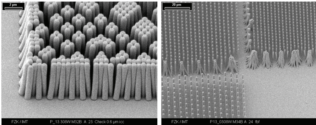
Abb. 3-11 Röntgenbelichtete Strukturen mit einer Bestrahlungsdosis von 4 \text{ kJ/cm}^3 und einem Abstand zwischen Maske und Substrat von 15 \mu\text{m} , Entwicklung in GG für 120 - 132 min. Links: Säulenfeld mit 550 \text{ nm} breiten Strukturen in 5 \mu\text{m} hohem Micro-Chem 950k PMMA A11. Rechts: Freistehende Säulen von 1,3 \mu\text{m} Durchmesser mit unterschiedlichen Mittenabständen in 11 \mu\text{m} hohem PMMA SX AR-P 6510.14.
