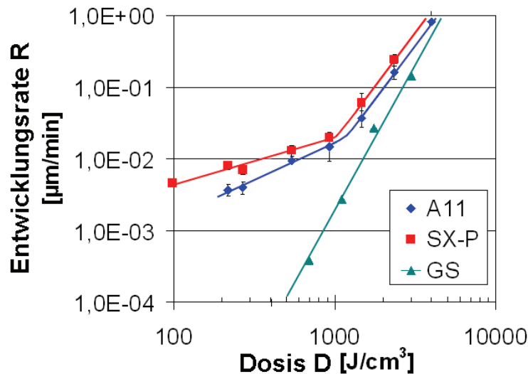
Abb. 2-7 Entwicklungsrates R als Funktion der abgelagerten Dosis für verschiedene Resistsysteme (A11: MicroChem 950k PMMA A11; SX-P: AllResist AR SX-P 6540.14; GS: Referenzmessung mit Röhm GS-233 wie in [Pant98a] verwendet), Entwicklung bei Raumtemperatur. Die Proben wurden an ANKA Litho3 bestrahlt und mit einem Profilometer vermessen.
