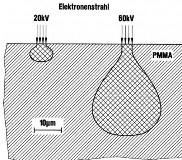
Abb. 3-3 Schematische Darstellung der von Elektronen mit unterschiedlicher Anfangsenergie abgelagerten Dosis in einem dicken Resist [Menz97].
