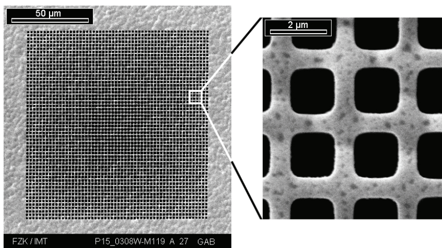
Abb. 4-5 IR-Filterstrukturen aus Gold. Links: Ansicht des kompletten galvanisch abgeformten Filters in 4,0 \pm 0,2 μm Gold. Rechts: Detailansicht der quadratischen Goldporen, die Wandstärke misst 720 \pm 30 nm.
