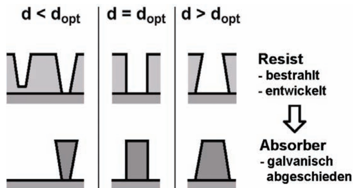
Abb. 3-6 Schnittzeichnung durch Resist/Absorber auf einem Substrat (Maskenmembran): Gezeigt wird der Einfluss der elektronenstrahlolithografisch abgelagerten Dosis d auf den Flankenwinkel des entwickelten Resists (oben) und die daraus resultierenden galvanisch abgeschiedenen Absorber (unten).
