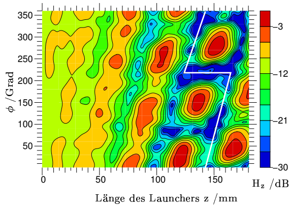
(a) Wandströme, TE 17,6 -Mode
