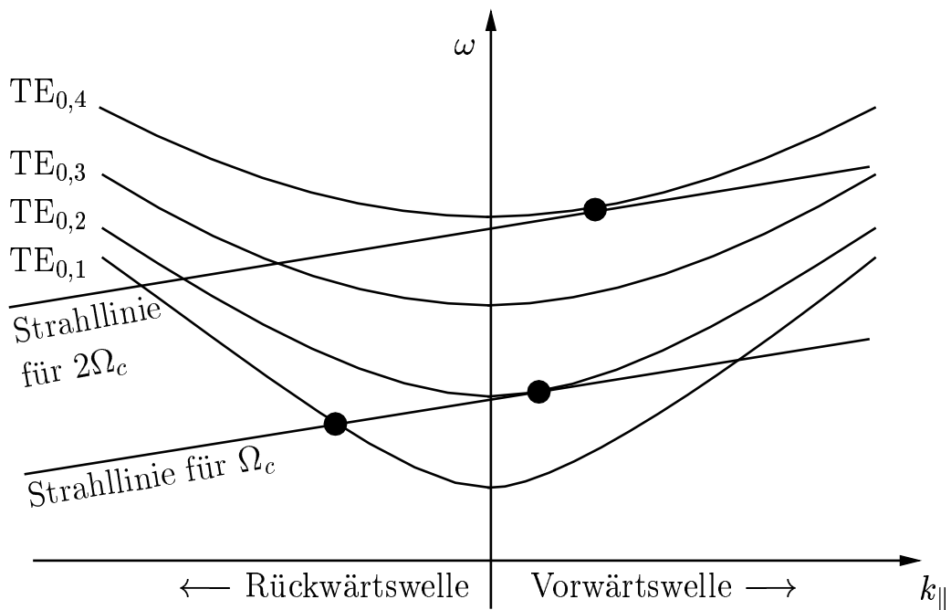
Bild 1.6: Brillouin-Diagramm.
