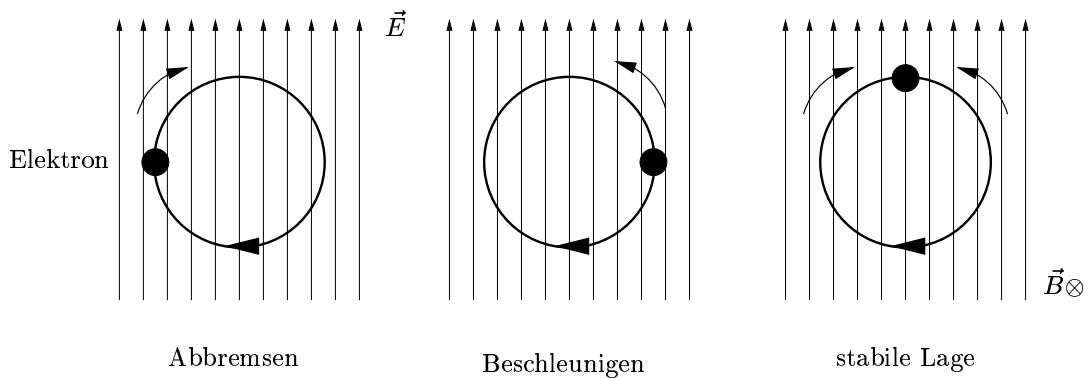
Bild 1.5: Phasensynchronisation.
