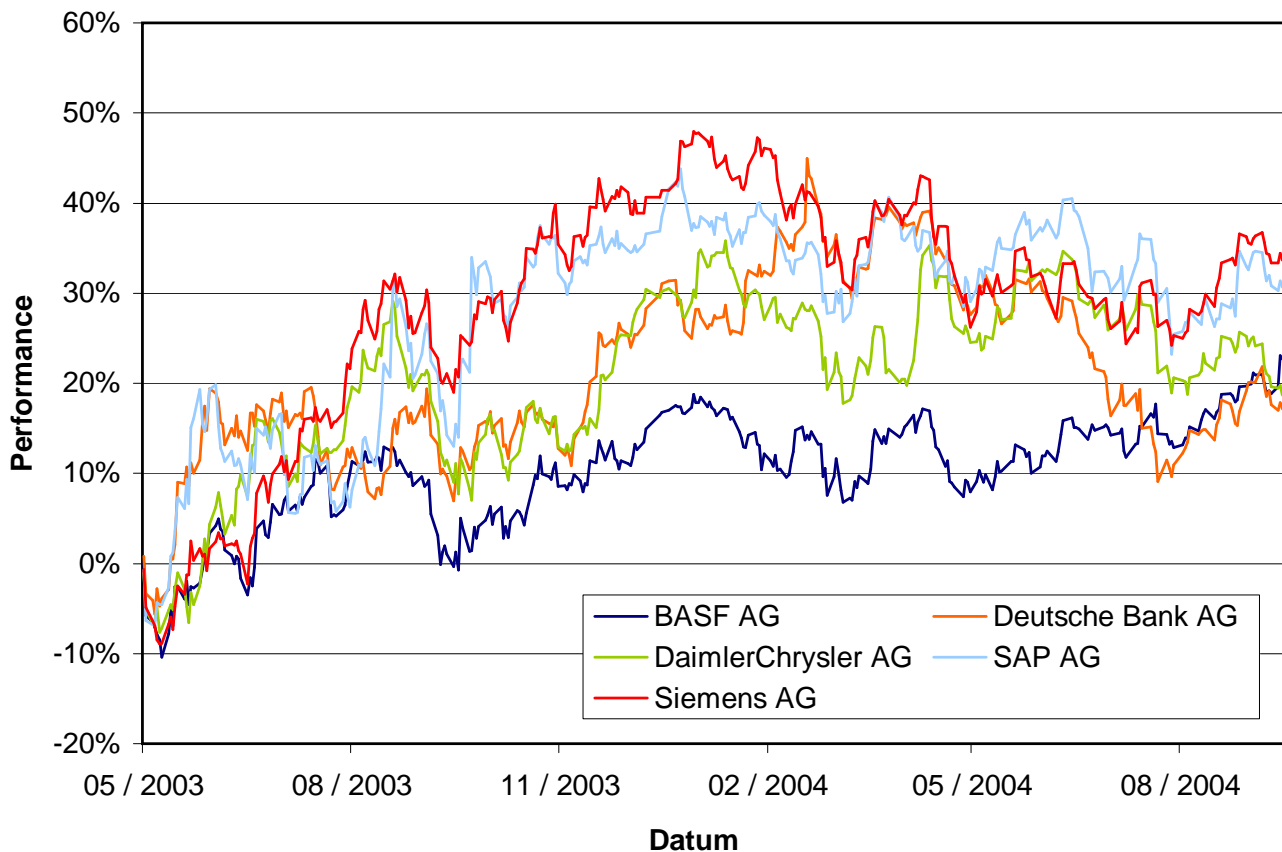
Abbildung 10.1: Performance der DAX ® -Aktien im Zeitraum vom 15.05.2003 bis 30.09.2004
