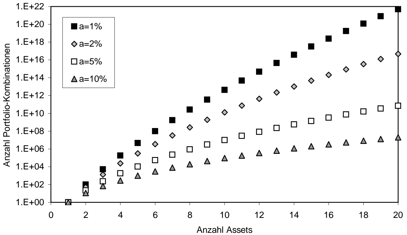
Abbildung 4.2: Wachstum möglicher Portfolios abhängig von der Anzahl der Assets und der Schrittweite a (logarithmische Skala)
