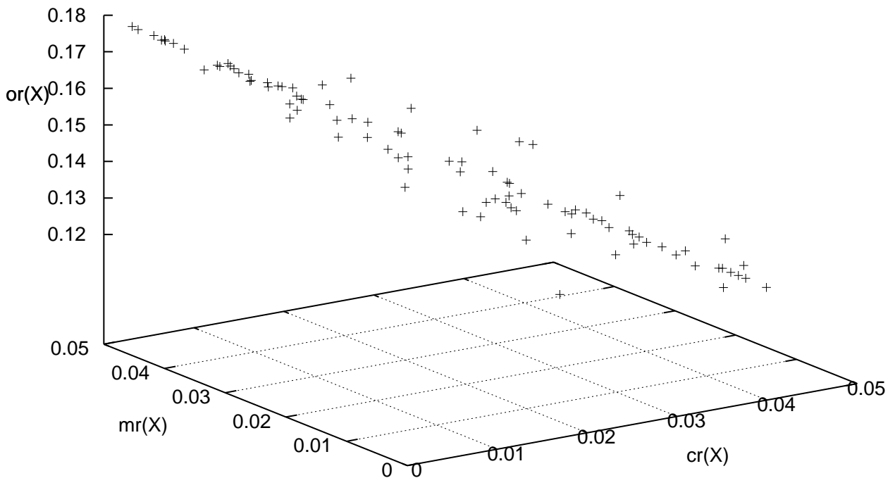
Abbildung 10.6: 3D-Streudiagramm für mr(x) , cr(x) und or(x)
