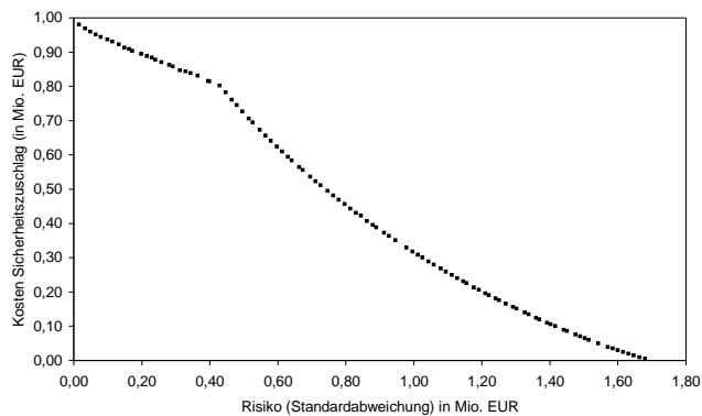
Abbildung 6.9: Pareto-optimale Front für Problem 2 (QS, XL und SL)
