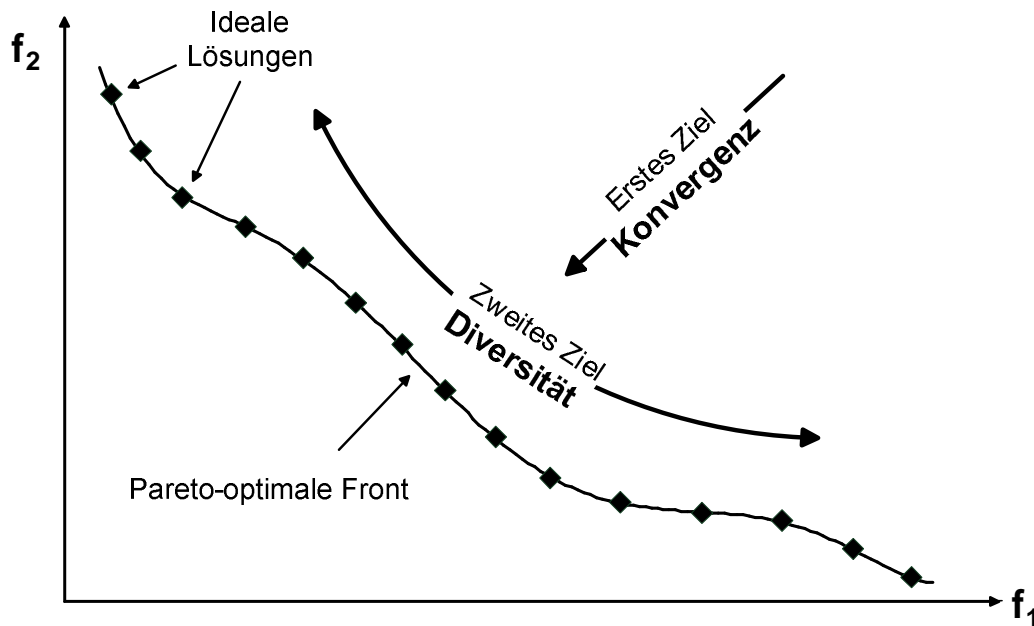
Abbildung 5.5: Zentrale Zielsetzungen und ideale Lösungen eines multikriteriellen evolutionären Algorithmus
