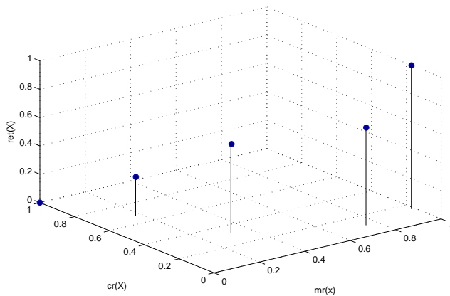
Abbildung 7.1: 3D-Streudiagramm für mr(x) , cr(x) und ret(x) (Beispieldaten aus Tab. 7.2)
