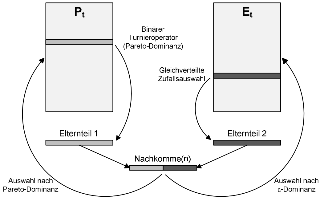
Abbildung 5.9: Schematischer Ablauf des \epsilon -MOEA
