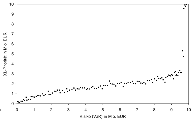
Abbildung 6.15: Anteil XL (Problem 3)
