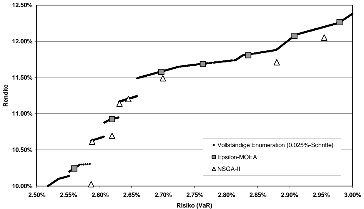
Abbildung 8.4: Vergrößerte Darstellung eines Abschnitts der Pareto-effizienten Portfolios bei drei Assets (ermittelt über vollständige Enumeration mit 0,025%-Schritten sowie mit NSGA-II und \epsilon -MOEA)
