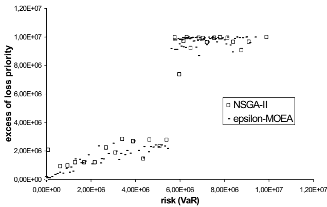
Abbildung 6.16: Pareto-optimale Front für Problem 4 (QS, XL, SL)
