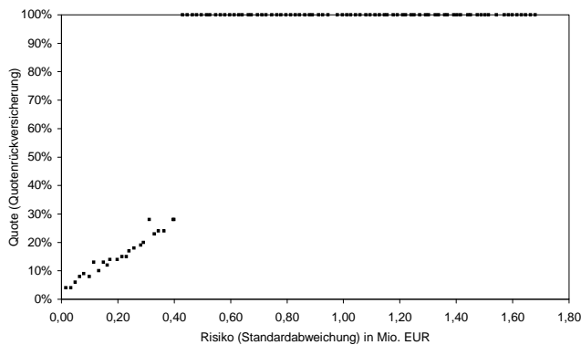
Abbildung 6.10: Quote a (Problem 2)
