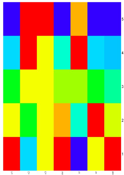
Abbildung 7.6: Heatmap (mit Beispieldaten aus Tabelle 7.2)
