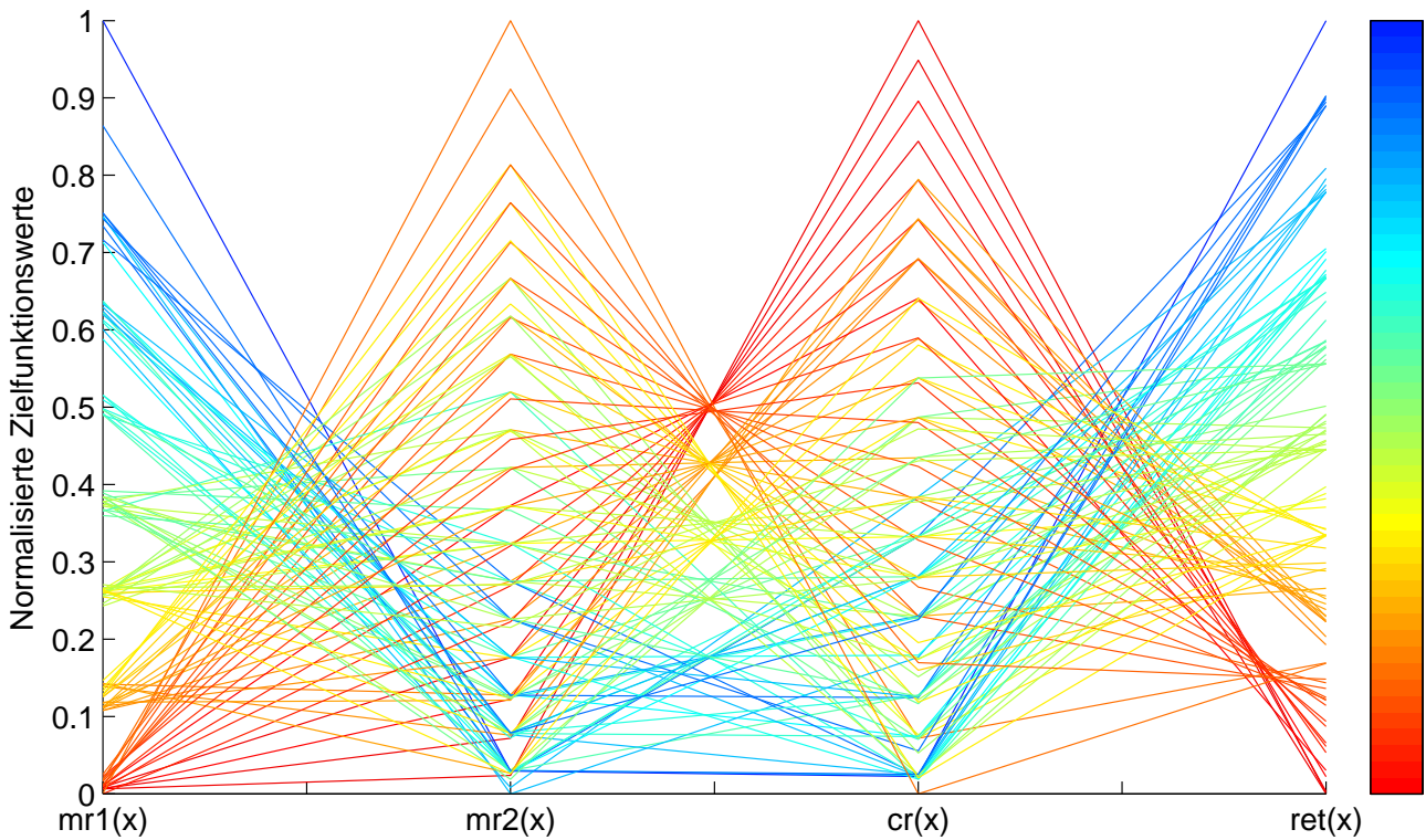
Abbildung 9.8: Parallelkoordinatenplot des beschränkten Problems ( \epsilon -MOEA)
