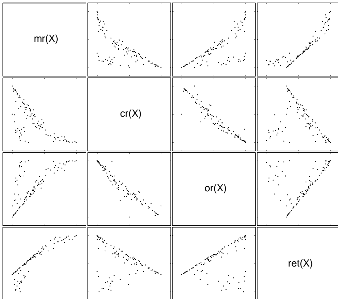
Abbildung 10.7: Streudiagramm-Matrix für mr(x) , cr(x) , or(x) und ret(x)
