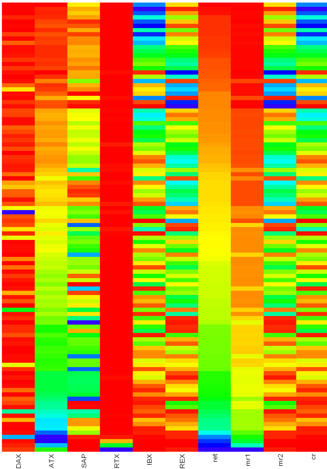
Abbildung 9.6: Veranschaulichung der Parameter- und Zielfunktionswerte des unbeschränkten Portfolioproblems mit einer Heatmap (Ergebnisse \epsilon -MOEA)
