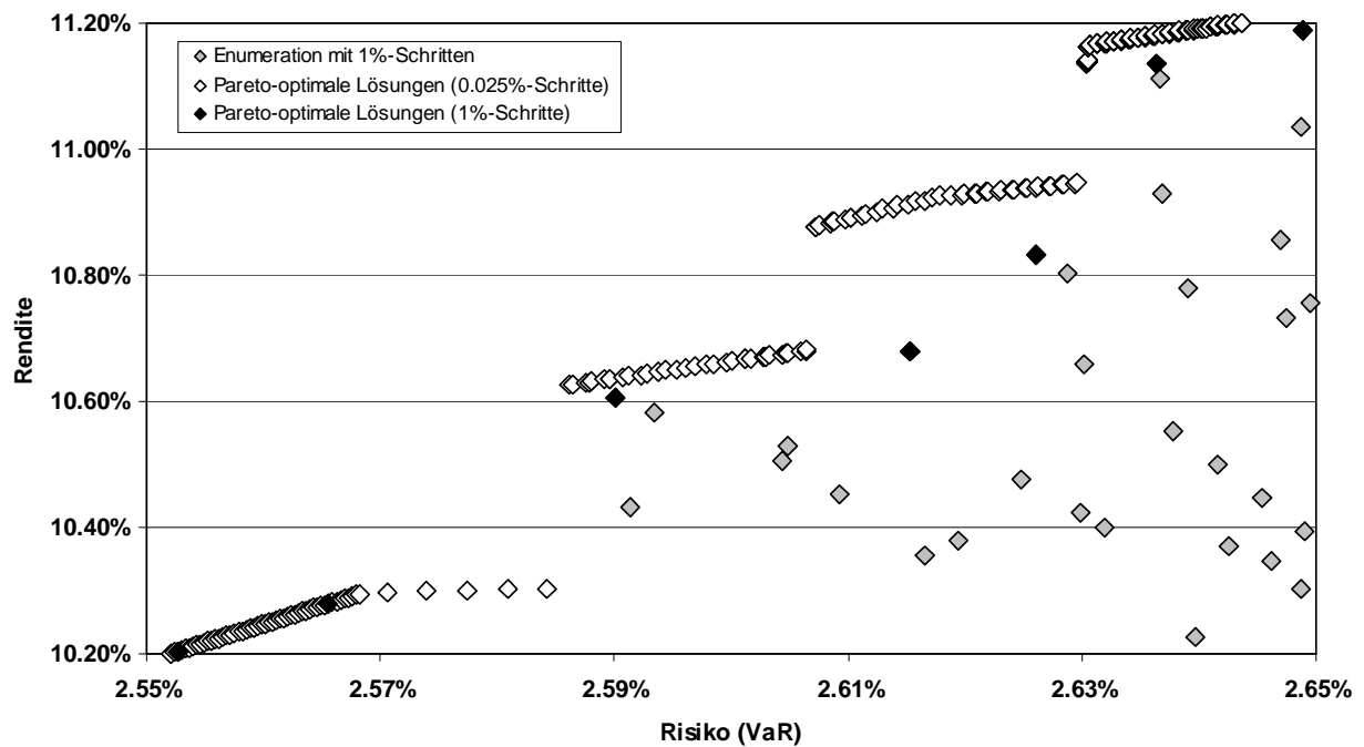
Abbildung 8.2: Vergrößerte Darstellung eines Ausschnitts des Zielfunktionsraums bei Portfolios mit drei Assets (ermittelt über vollständige Enumeration mit 1%-Schritten) sowie entsprechender effizienter Portfolios (ermittelt mit 0,025%- und 1%-Schritten)
