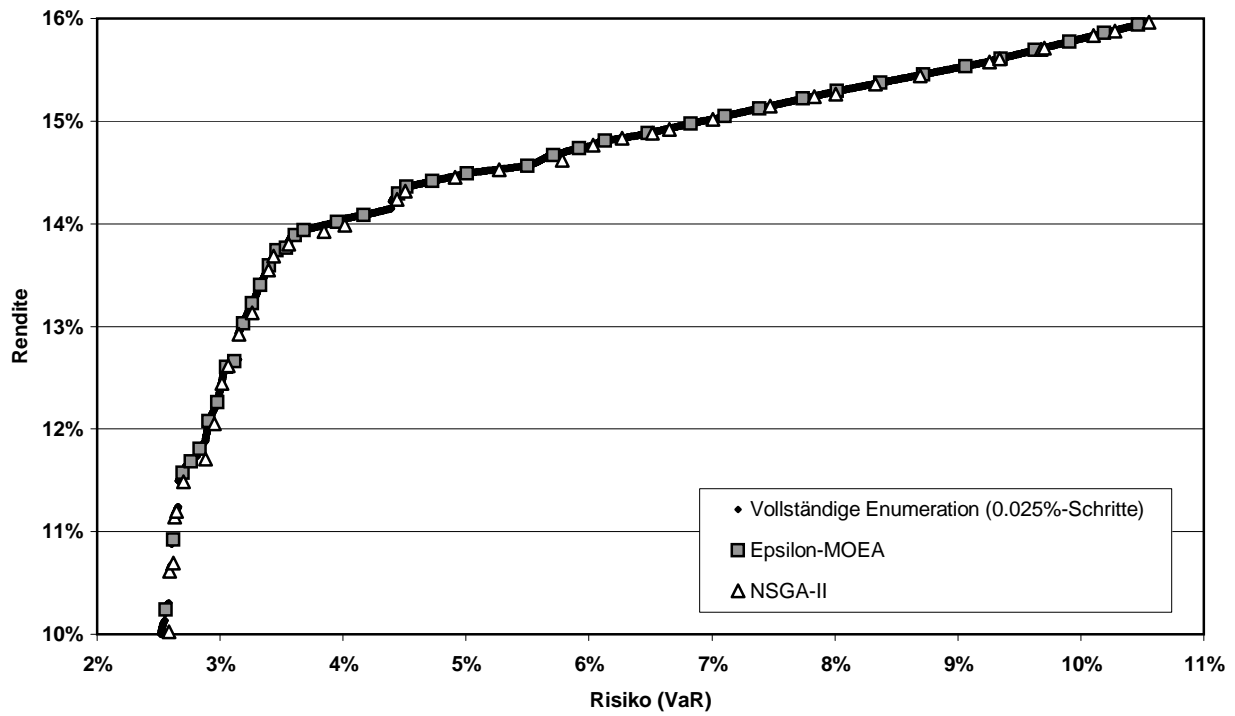
Abbildung 8.3: Effiziente Portfolioallokationen mit drei Assets bei Optimierung mit den beiden Zielfunktionen Rendite und Risiko ermittelt über vollständiger Enumeration mit 0,025%-Schritten sowie mit NSGA-II und \epsilon -MOEA
