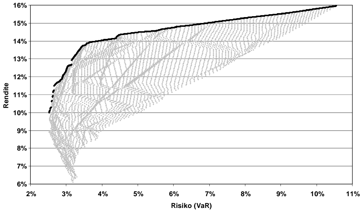
Abbildung 8.1: Mögliche Portfolioallokationen mit drei Assets bei Optimierung mit den beiden Zielfunktionen Risiko und Rendite bei 1%-Schritten sowie effiziente Portfolios bei 0,025%-Schritten (ermittelt über vollständige Enumeration)
