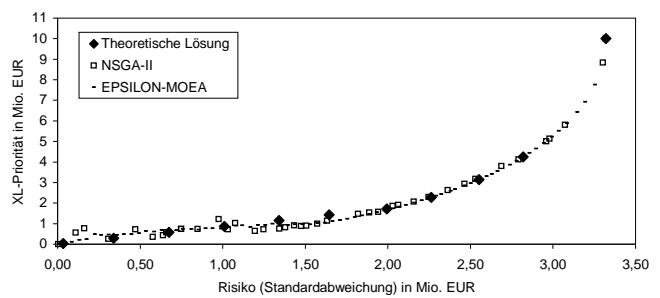
Abbildung 6.8: Anteil XL (Problem 1)
