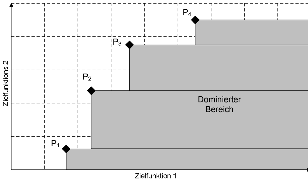
Abbildung 5.4: Dominierter Bereich bzgl. des gewöhnlichen Dominanzprinzips
