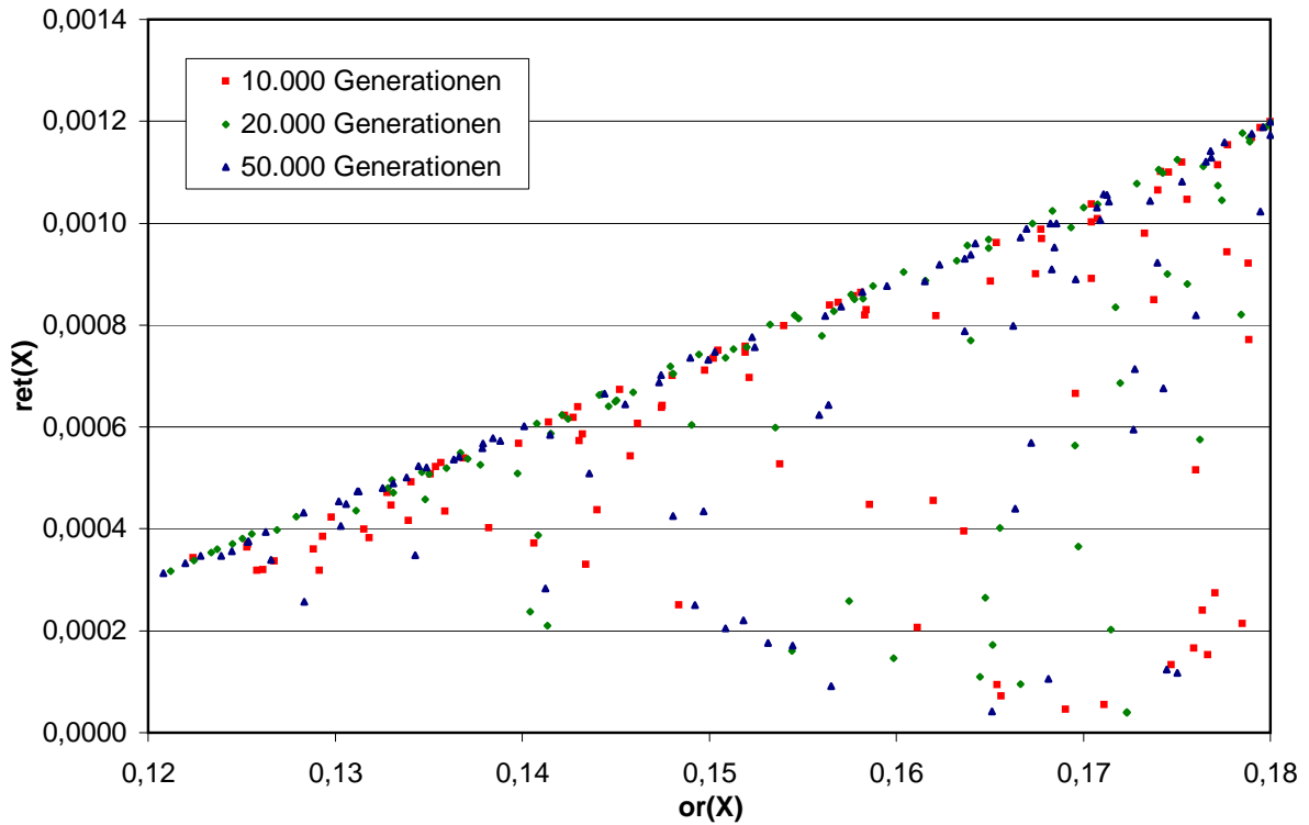
Abbildung 10.4: Konvergenzverhalten bei Optimierung mit 10.000, 20.000 und 50.000 Generationsdurchläufen: or(x) und ret(x)
