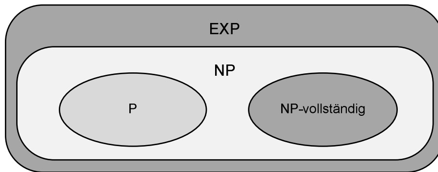
Abbildung 4.1: Komplexitätsklassen EXP , NP und P unter der Annahme \mathbf{P} \neq \mathbf{NP} [Wage03]
