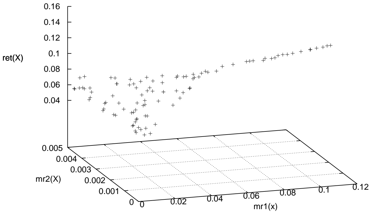
Abbildung 9.2: 3D-Streudiagramm für mr_1(x) , mr_2(x) und ret(x) mit dem NSGA-II
