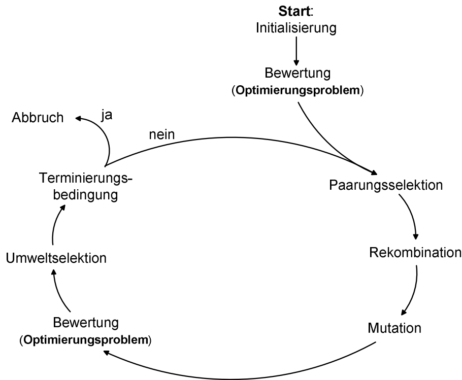
Abbildung 5.1: Klassischer Ablauf eines evolutionären Algorithmus (Darstellung in Anlehnung an [Weic02])
