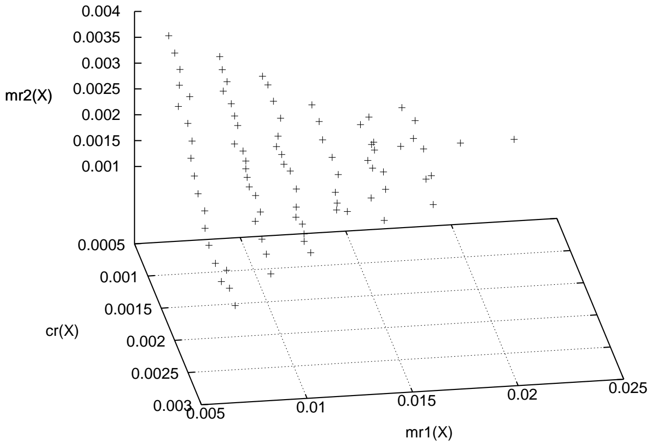
Abbildung 9.7: 3D-Streudiagramm für mr_1(x) , mr_2(x) , cr(x) mit Beschränkungen ( \epsilon -MOEA)
