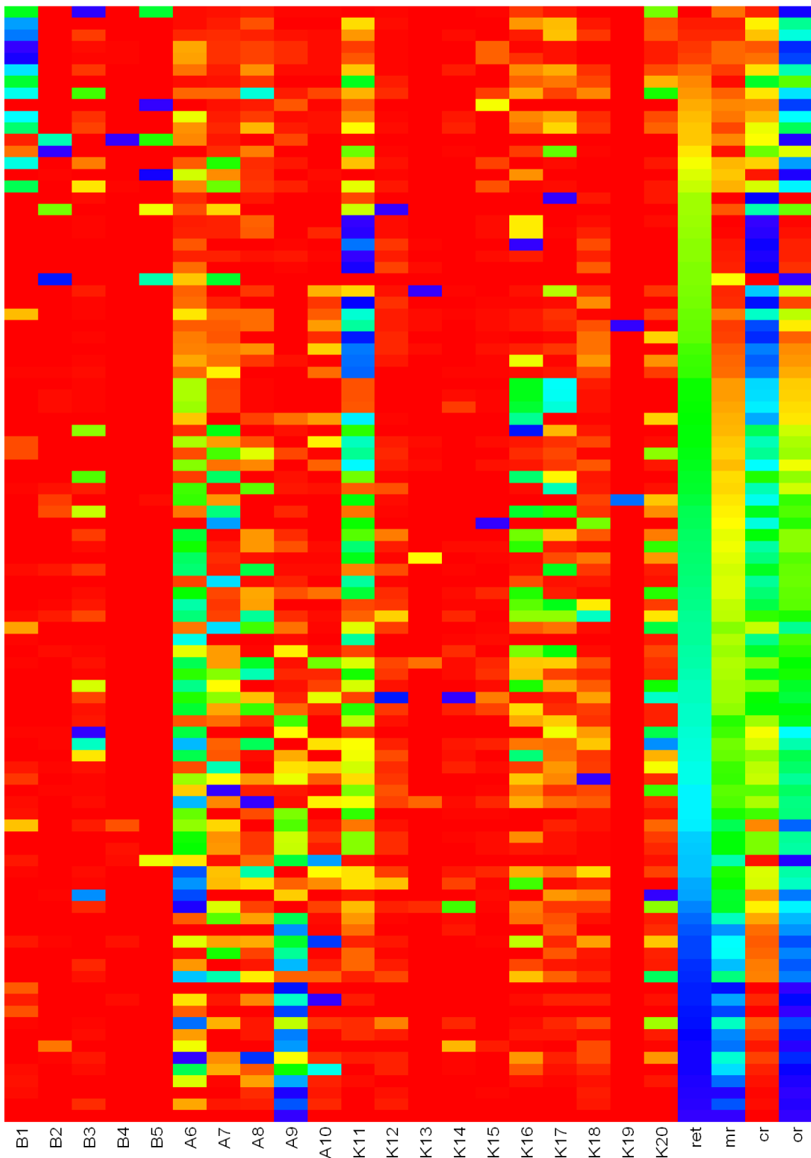
Abbildung 10.9: Heatmap für die Assets 1-20 (Bonds B1-B5, Aktien A6-A10, Kredite K11-K20) sowie die Zielfunktionen ret(x) , mr(x) , cr(x) und or(x) (Sortierung entsprechend ret(x) )
