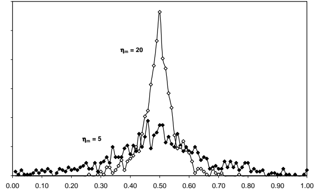
Abbildung 5.3: Empirische Verteilung des mutierten Individuums x' = 0,5 bei 1000 Simulationen des polynomialen Mutationsoperators mit variierendem \eta_m
