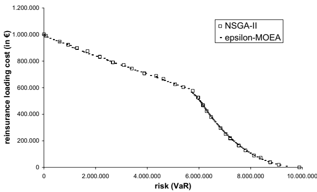
Abbildung 6.16: Pareto-optimale Front für Problem 4 (QS, XL, SL)
