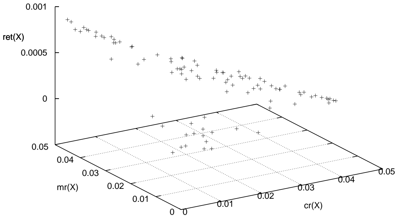
Abbildung 10.5: 3D-Streudiagramm für mr(x) , cr(x) und ret(x)
