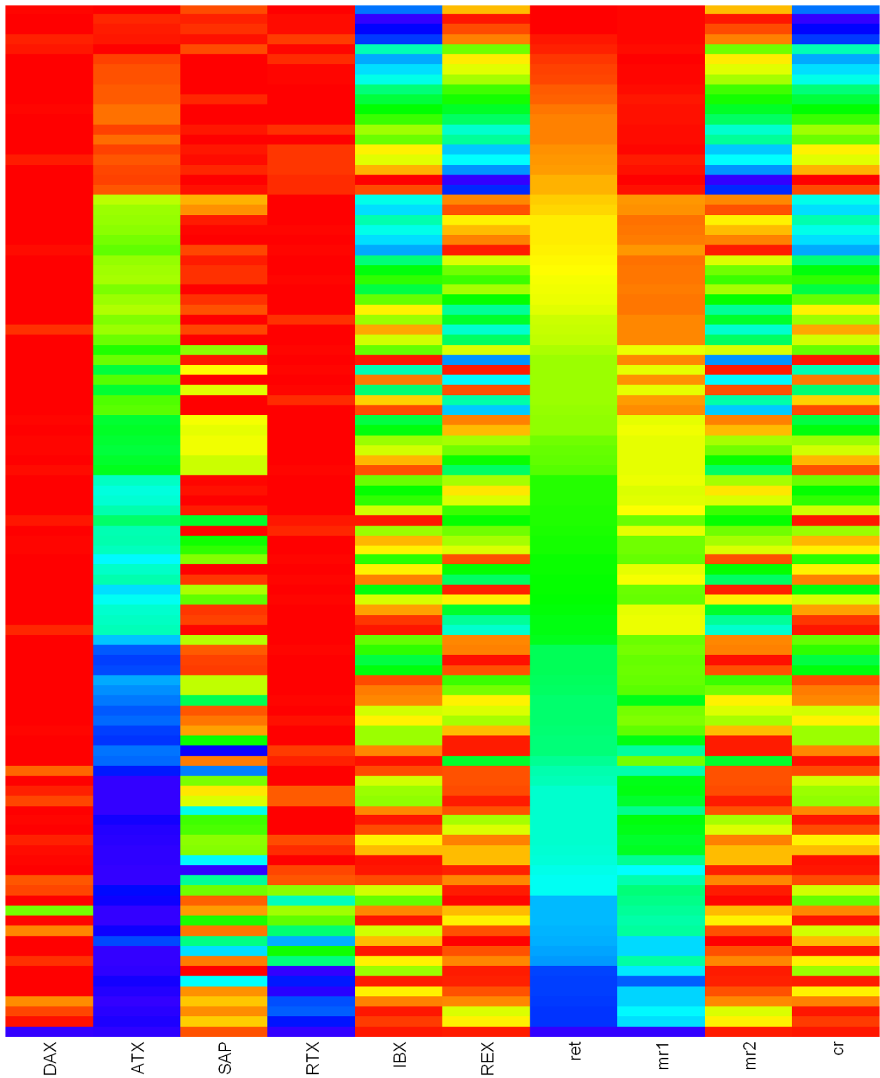
Abbildung 9.9: Veranschaulichung der Parameter- und Zielfunktionswerte des beschränkten Portfolioproblems mit einer Heatmap (Ergebnisse \epsilon -MOEA)
