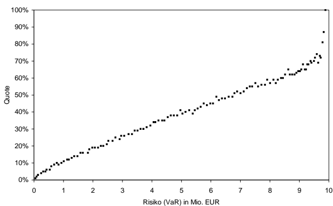
Abbildung 6.14: Anteil QS (Problem 3)
