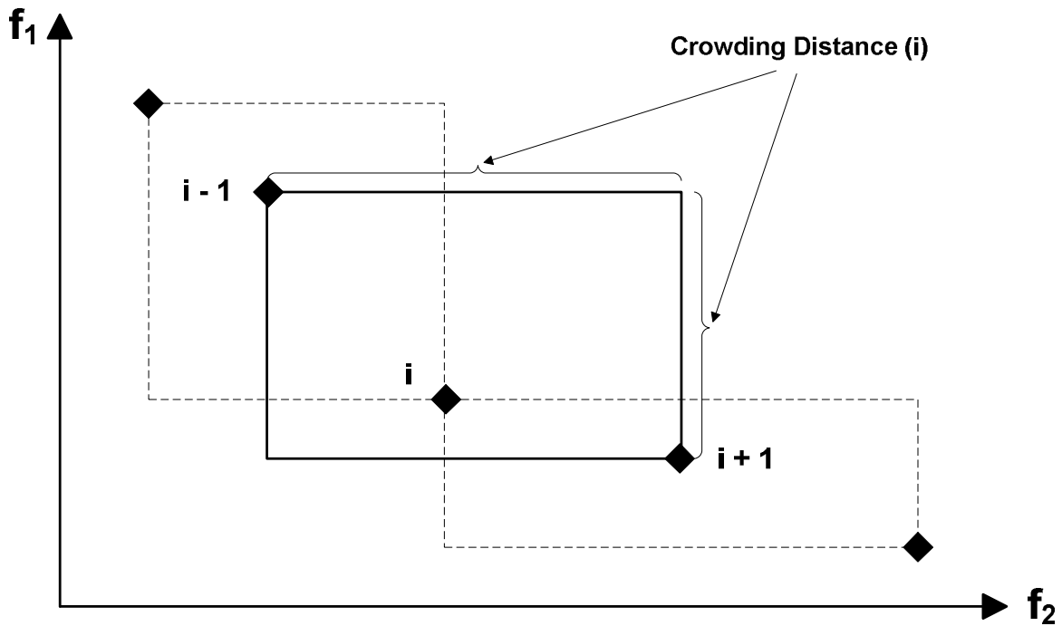
Abbildung 5.7: Rechteck um die Lösung i zur Ermittlung der Crowding Distance
