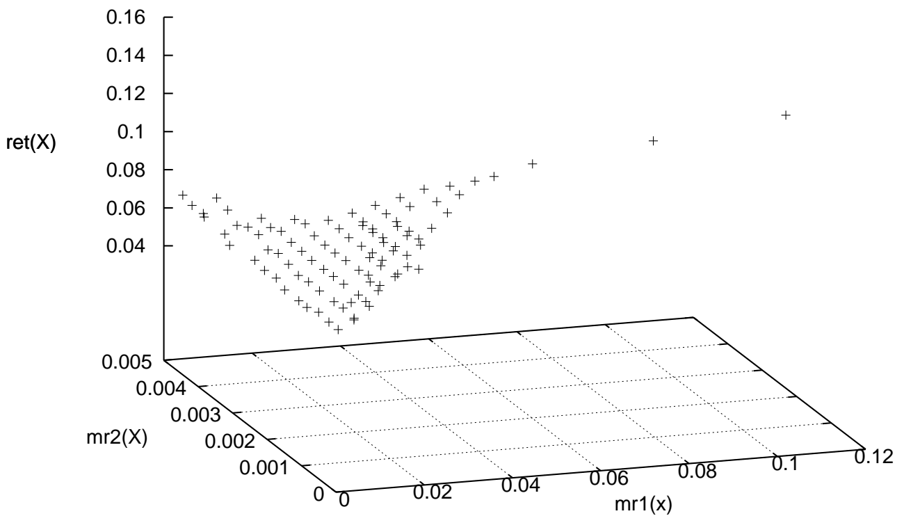
Abbildung 9.3: 3D-Streudiagramm für mr_1(x) , mr_2(x) und ret(x) mit dem \epsilon -MOEA
