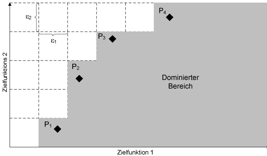
Abbildung 5.8: Dominiertes Bereich bzgl. des \varepsilon -Dominanzprinzips
