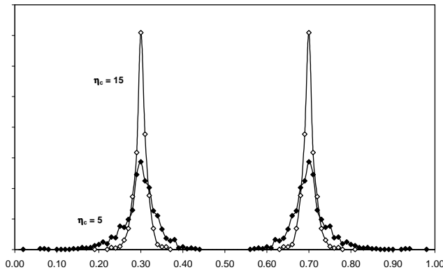
Abbildung 5.2: Empirische Verteilung der Nachkommen von x = 0,3 und y = 0,7 bei 1000 Simulationen des SBX-Operators mit variierendem \eta_c
