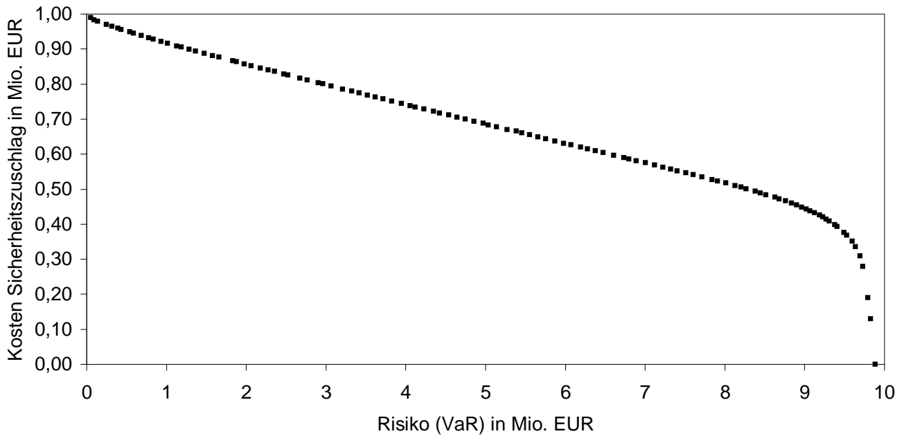
Abbildung 6.13: Pareto-optimale Front mit QS- und XL-Vertrag (Problem 3)
