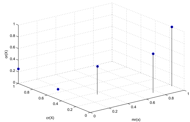
Abbildung 7.2: 3D-Streudiagramm für mr(x) , cr(x) und or(x) (Beispieldaten aus Tab. 7.2)
