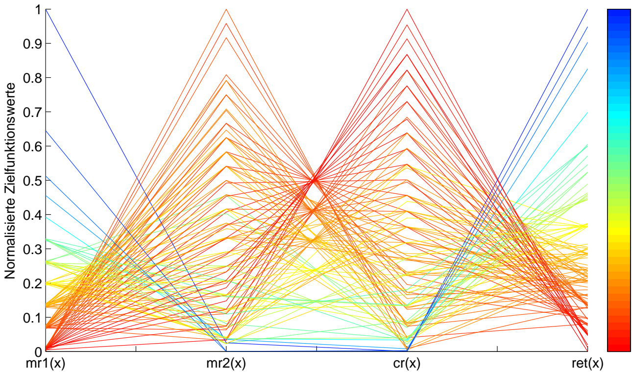
Abbildung 9.5: Parallelkoordinatenplot des unbeschränkten Problems ( \epsilon -MOEA)
