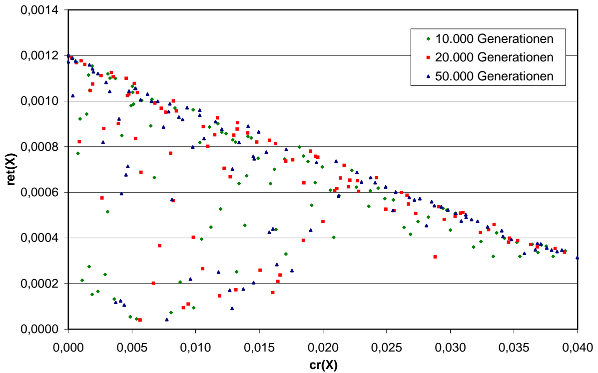
Abbildung 10.3: Konvergenzverhalten bei Optimierung mit 10.000, 20.000 und 50.000 Generationsdurchläufen: cr(x) und ret(x)
