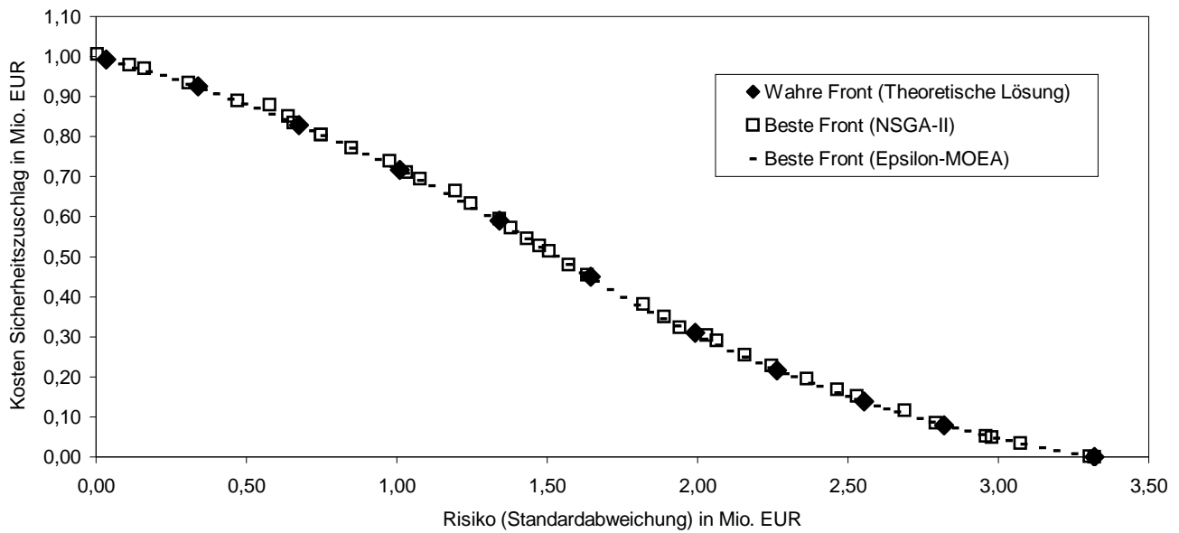
Abbildung 6.6: Pareto-optimale Front mit QS- und XL-Vertrag (Problem 1)
