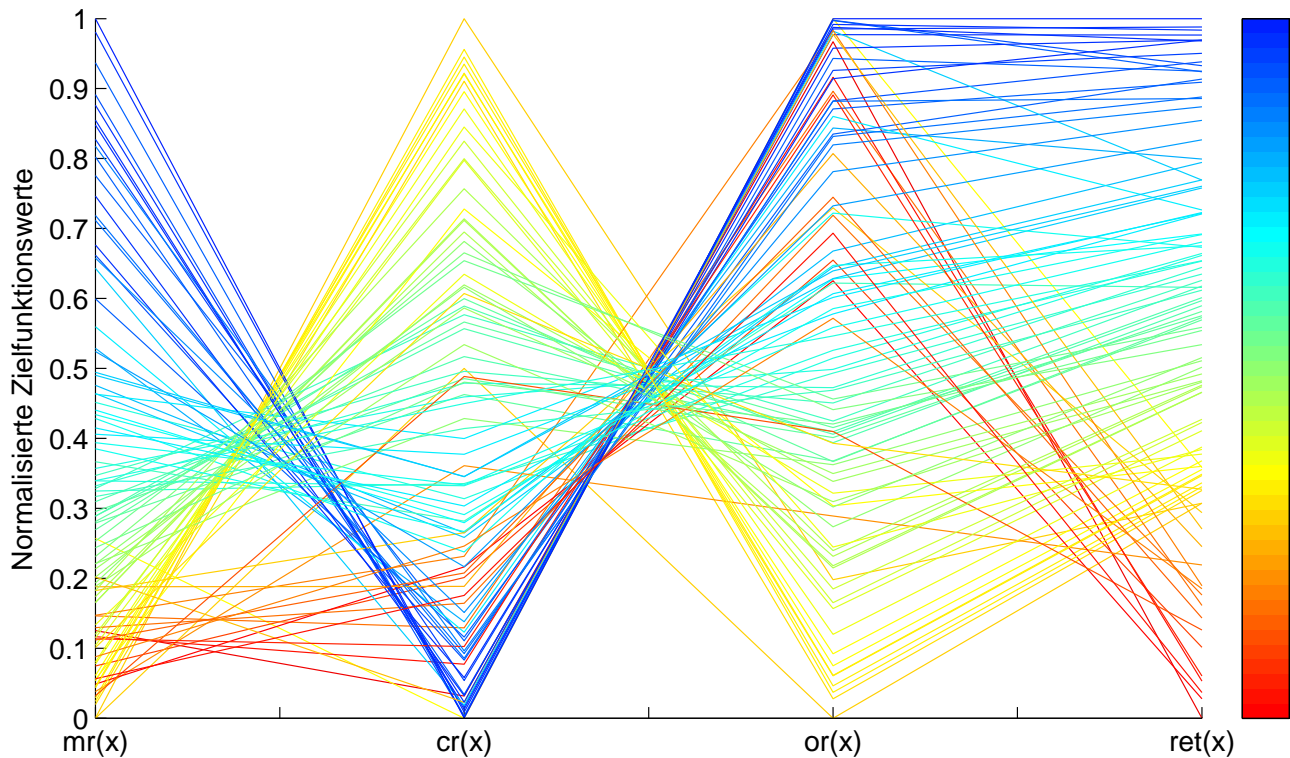
Abbildung 10.8: Parallelkoordinatenplot für mr(x) , cr(x) , or(x) und ret(x) (Das Farbspektrum wurde entsprechend ret(x) gewählt)
