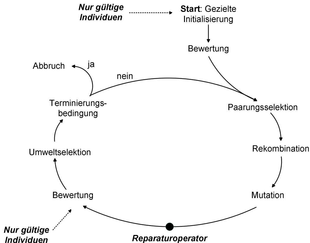
Abbildung 8.5: Anpassungen des generellen GA-Ablaufs in Abbildung 5.1 für Problemstellungen aus dem Integrierten Portfoliomanagement
