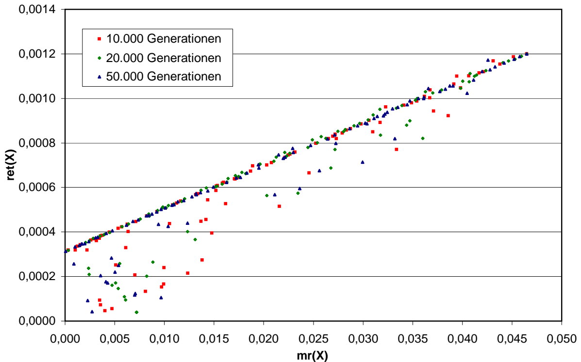
Abbildung 10.2: Konvergenzverhalten bei Optimierung mit 10.000, 20.000 und 50.000 Generationsdurchläufen: mr(x) und ret(x)
