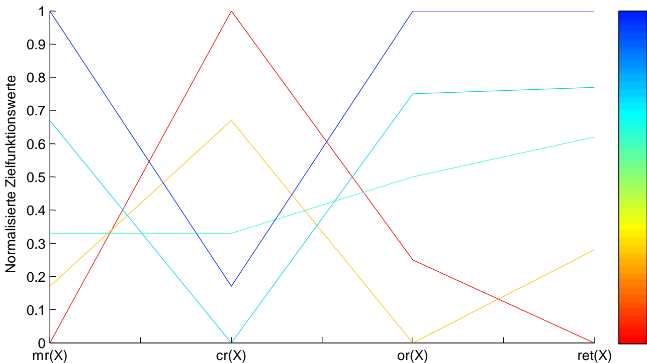
Abbildung 7.4: Parallelkoordinatenplot (mit Beispieldaten aus Tabelle 7.2)
