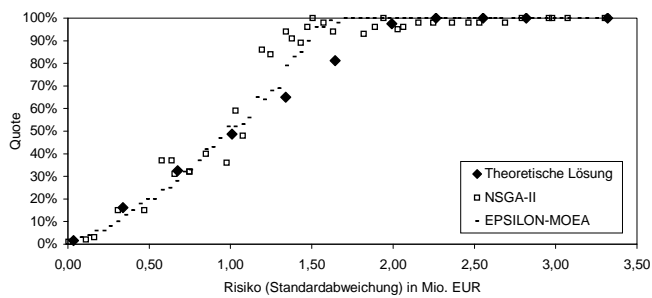
Abbildung 6.7: Anteil QS (Problem 1)
