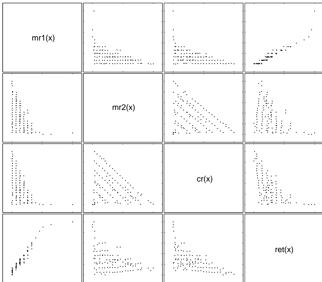
Abbildung 9.4: Streudiagramm-Matrix für mr_1(x) , mr_2(x) , cr(x) und ret(x)
