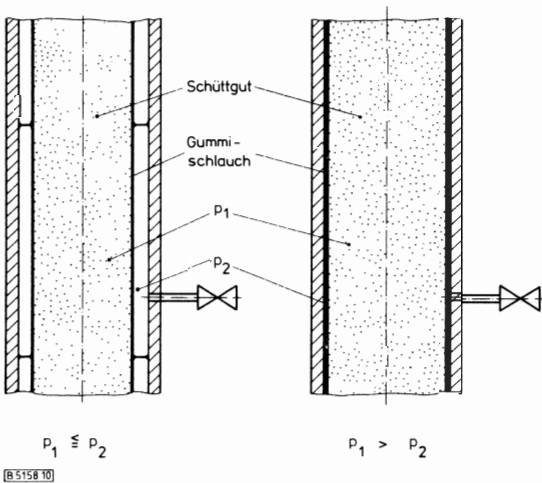
Abb. 10. Rohr mit veränderlichem Durchmesser zur Verdichtung der Feststoffsäule und Steuerung des radialen Haltdrucks (Inst. für MVM, Univ. K'he 1982); Einordnung: A IV 1/1 - 2/1/1 - 2/2/1/2 - 3/2/2/2 - 2/1/2.
