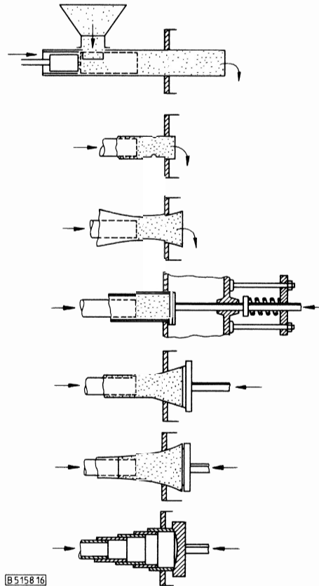
Abb. 16. Kolbenförderer mit Drehschieber und verschiedenen Formstücken sowie Verschlussklappen [30]; Einordnung: B V 1/1/3/3/1/1/1/3/1/1/1.
