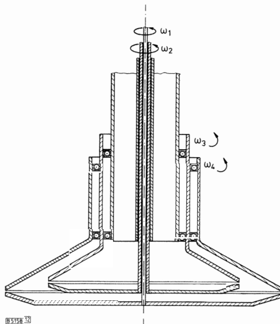
Abb. 12. Erhöhung der Dichtwirkung durch größere Verweilzeit und Steuermöglichkeit (Inst. für MVM, Univ. K'he 1982); Einordnung: A V 3/1/1/1/1/1/2 - 3/1/1 - 2/1/1/2.
