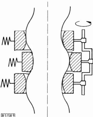
Abb. 9. Feststoffsäule in einem Schlauch mit Beeinflussung des Selbsthemm-Effektes. Der Schlauch hat die Funktionen „niedriger Randreibwert“ und „Abdichtung gegen den Innendruck“. Die Radialspannungen werden nicht vom Schlauch aufgenommen, sondern der Schlauch stützt sich in den einzelnen beweglichen Metallringen ab (Inst. für MVM, Univ. K'he 1982); Einordnung: A IV 1/1 - 2/1/2/1/2 - 3/1/1 - 2/1 - 2/1/2.
