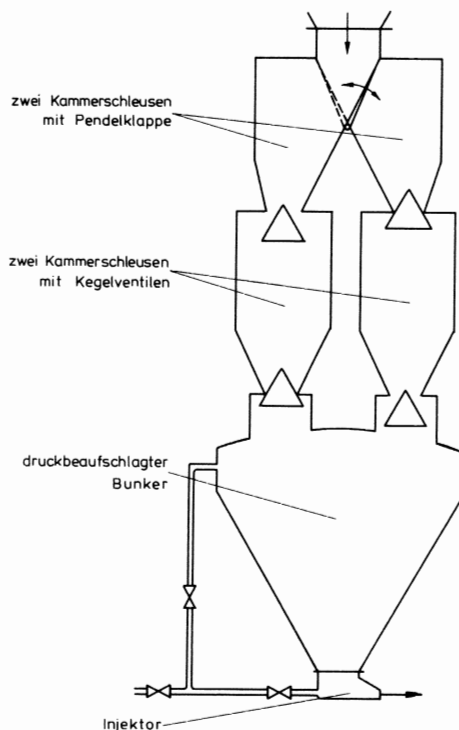
Abb. 6. Mehrkammer-Schleusensystem zur pneumatischen Förderung [16]; Einordnung: A Ia 3/1/2/1/1/1/3/2/2/1/2/1.
