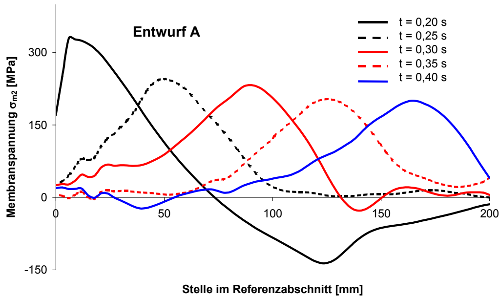
Abbildung 71: Zeitliche Änderung des Verlaufs der Membranspannung
