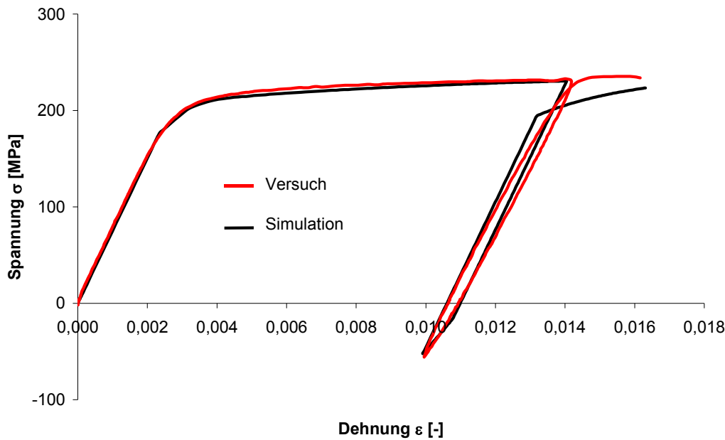
Abbildung 34: Vergleich berechneter und experimentell bestimmter Spannungs-Dehnungshysterese an Aluminiumprobe ab12
