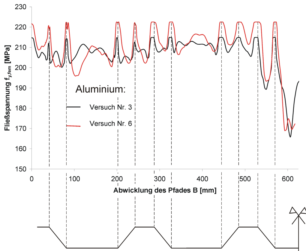
Abbildung 85: Verlauf der Fließspannung entlang Pfad B
