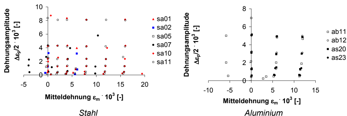
Abbildung 16: Parameterspektrum der durchgeführten Lastwechselversuche
