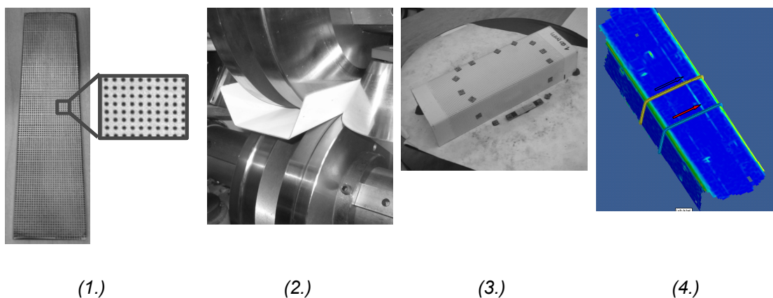
Abbildung 57: Blechplatte mit Punktraster (1.), Umformprozess (2.), Abschnitt des umgeformten Blechs mit Messmarken (3.) und ermittelte Formänderungen (4.)
