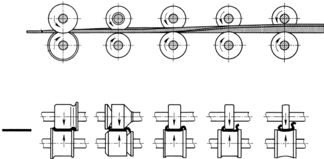
Abbildung 3: Schematische Darstellung einer Profilieranlage, aus DIN 8586
