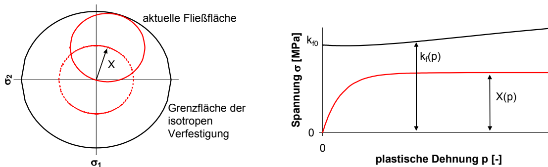
Abbildung 7: Schematische Darstellung des kinematischen Verfestigungsmodells nach Chaboche in der Spannungsebene (links) und im einachsigen Fall (rechts)
