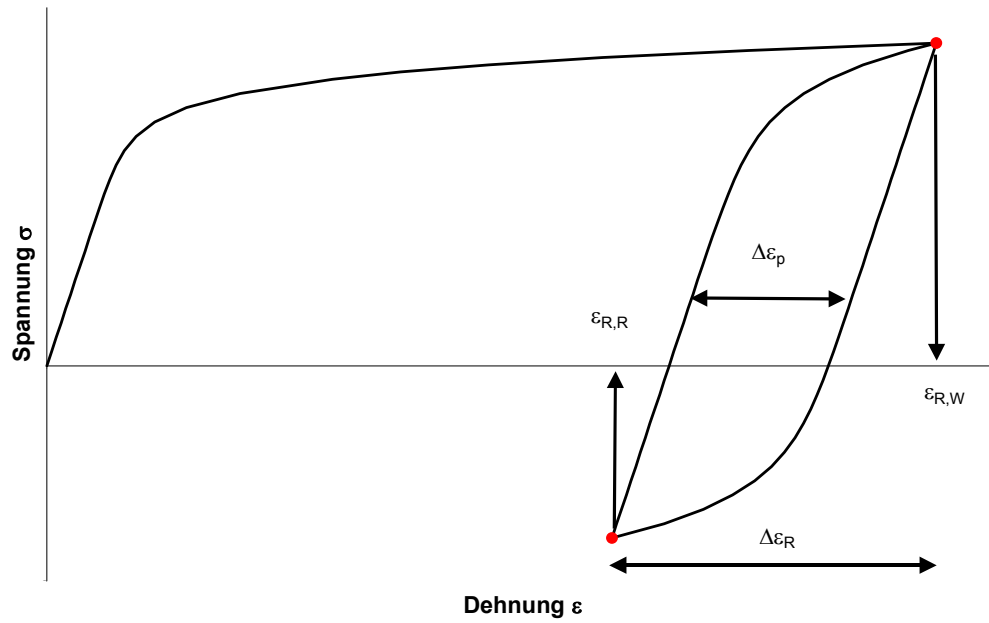
Abbildung 14: Abschätzung der Dehnungsamplitude
