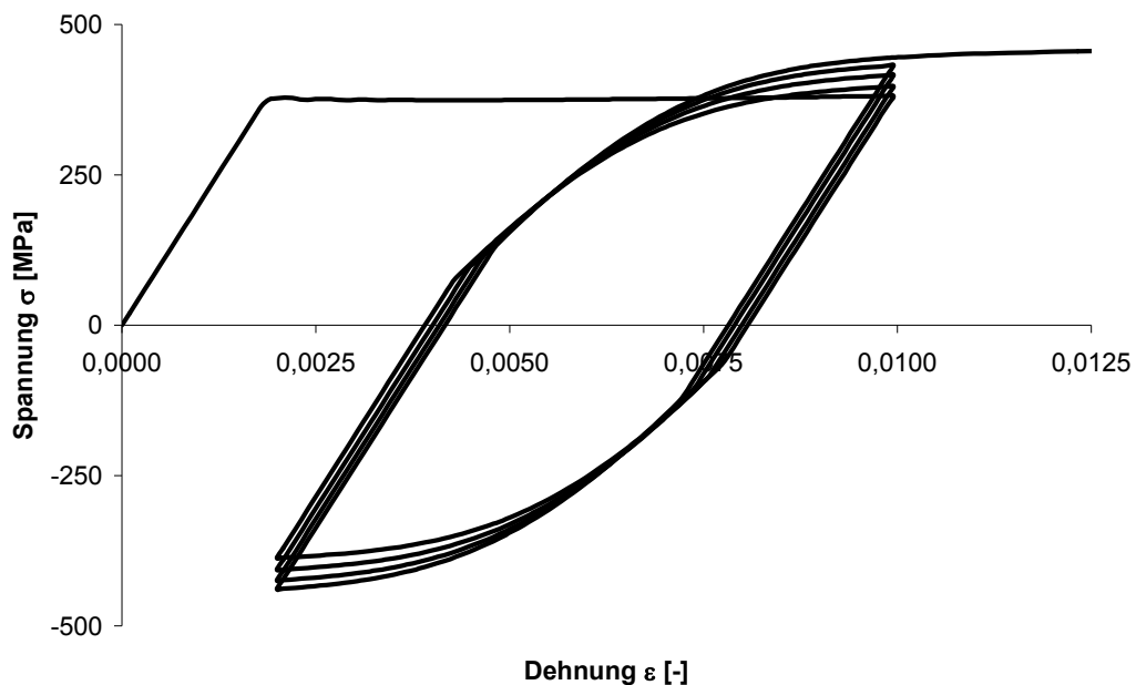
Abbildung 35: Anpassung der isotropen Verfestigungskomponente an Zugversuch
