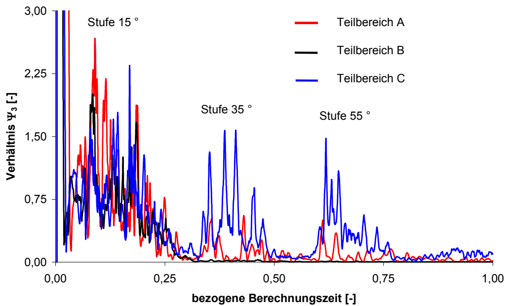
Abbildung 46: Verlauf des Verhältnisses \Psi_3 – nur Symmetriebedingungen
