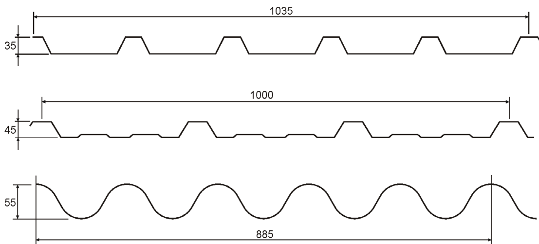
Abbildung 2: Querschnittsformen – Trapezprofil (oben und Mitte) und Wellprofil (unten)
