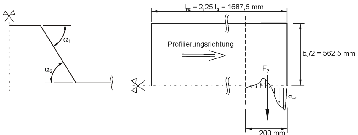
Abbildung 64: Definition der Biegewinkel \alpha_1 und \alpha_2 (links) und der Reaktionskraft F_2 im Bereich des Bändeinlaufs (rechts)
