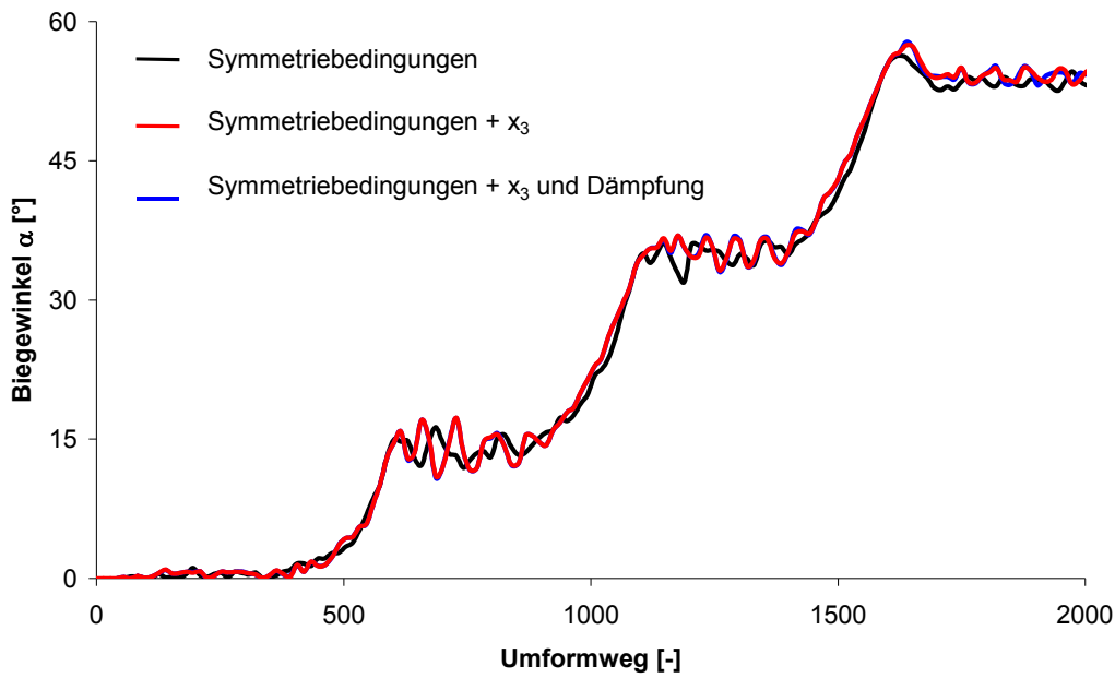
Abbildung 49: Einfluss der Randbedingungen und der Dämpfung auf den Verlauf des Biegewinkel
