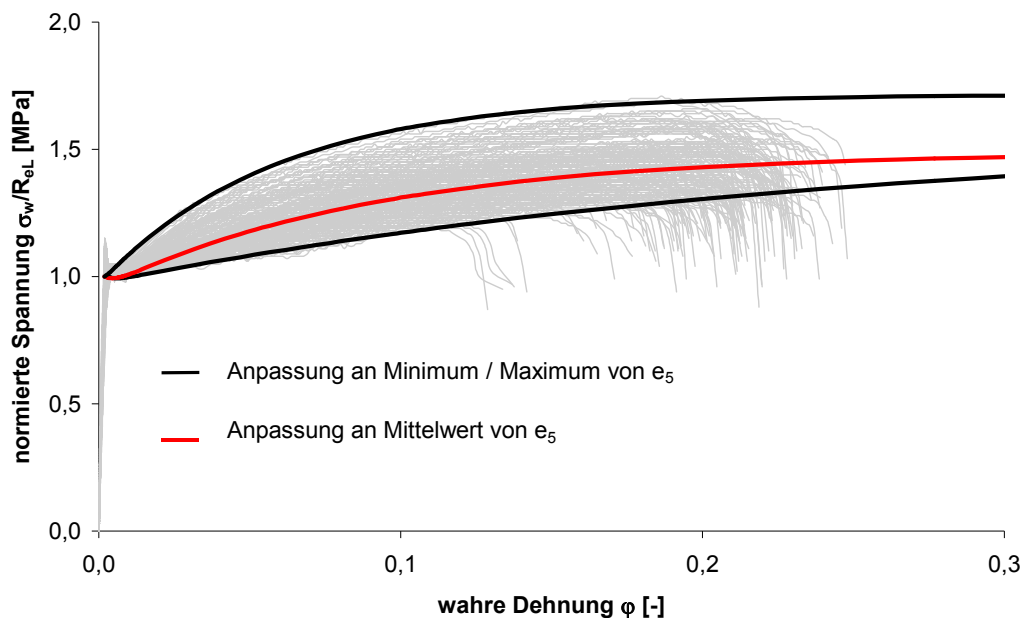
Abbildung 12: Fließkurven und rechnerisch angepasste Kurven bei Stahl
