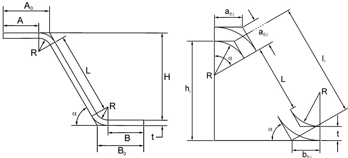
Abbildung 102: Maßbezeichnungen an einem allgemeinen Profiltyp
