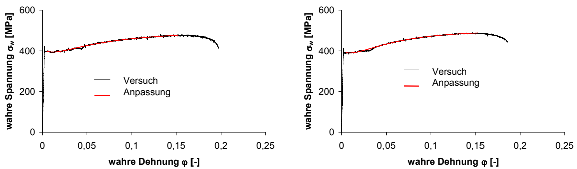
Abbildung 91: Wahre Spannungs-Dehnungs-Kurve quer zur - Probe sa10 (links) und Probe sa11 (rechts)
