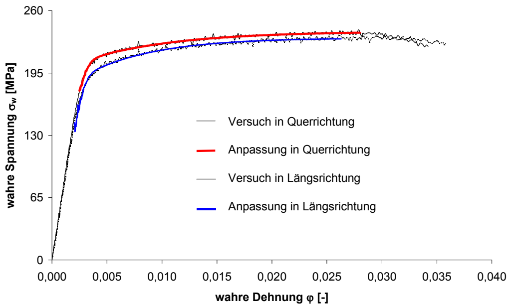
Abbildung 24: Fließkurven der Probe ab12
