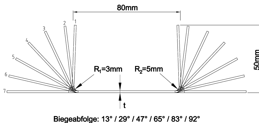
Abbildung 55: Profilblume, nach [17]
