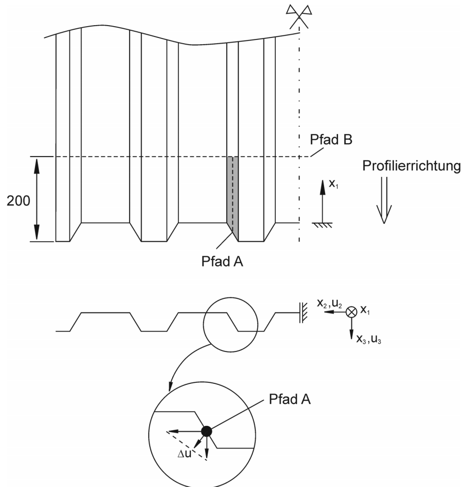
Abbildung 76: Definition der Referenzfläche zur Beurteilung des Auftretens plastischer Beulen und des Pfades zur Berechnung des Grades der Kaltverfestigung
