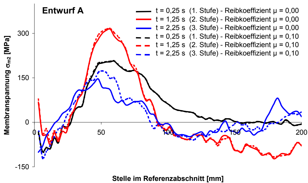
Abbildung 72: Verteilung der Membranspannung beim Einlauf in verschiedene Stufen
