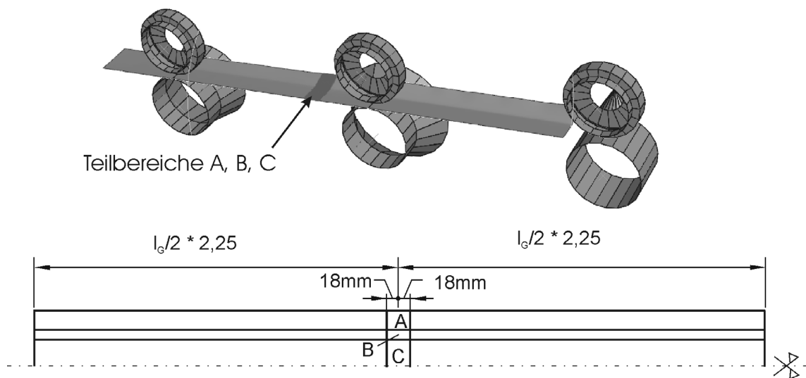
Abbildung 43: Lage der Teilbereiche im Blech – Modell (oben) und Draufsicht (unten)
