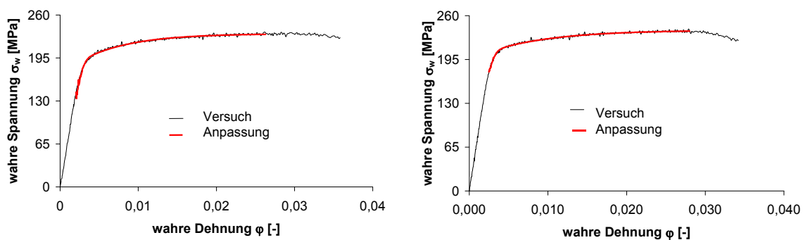
Abbildung 96: Wahre Spannungs-Dehnungs-Kurve der Probe ab12 in Walzrichtung (links) und quer zur Walzrichtung (rechts)
