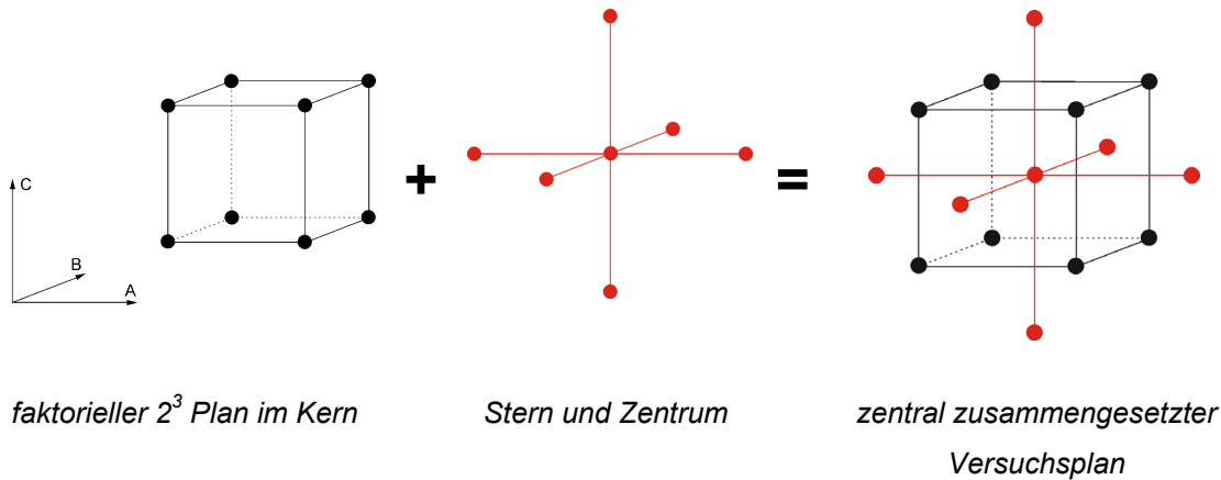
Abbildung 75: Konstruktion eines zentral zusammengesetzten Versuchsplanes mit drei Faktoren
