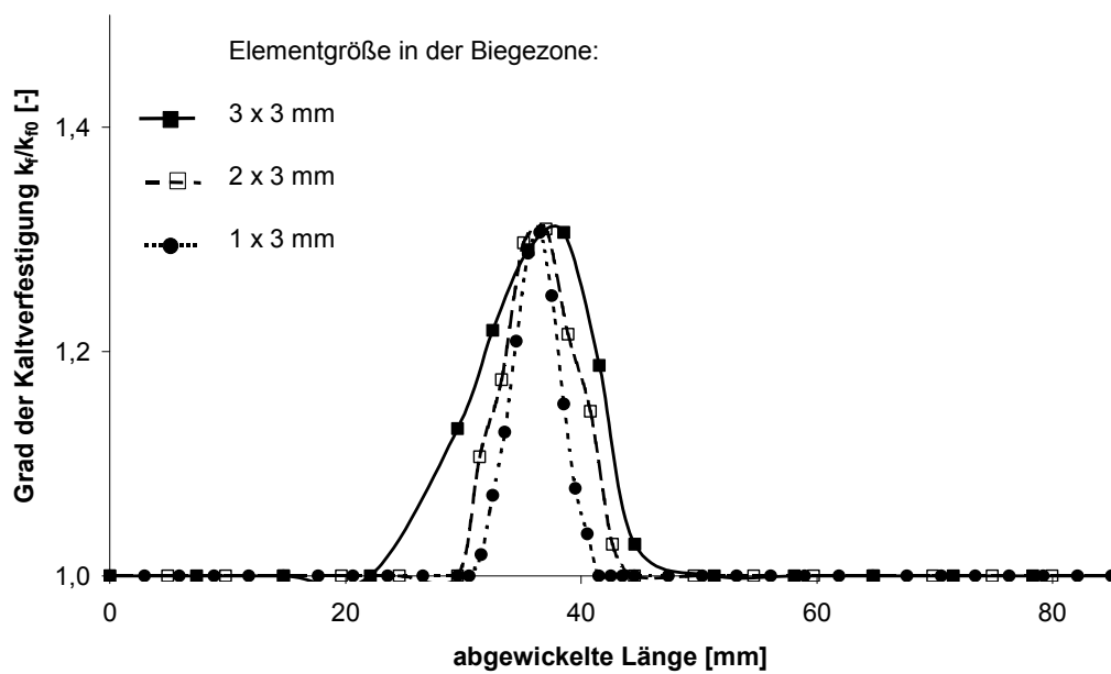
Abbildung 51: Grad der Kaltverfestigung in Abhängigkeit der Elementgröße
