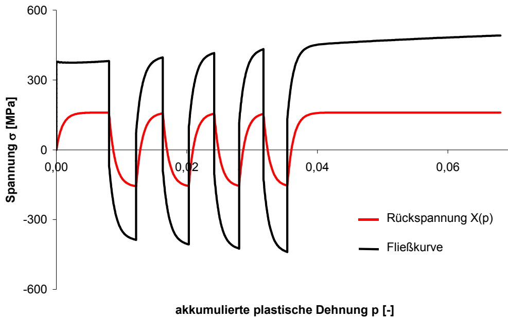
Abbildung 36: Verlauf der Fließkurve und der Rückspannung X in Abhängigkeit der akkumulierten plastischen Dehnung
