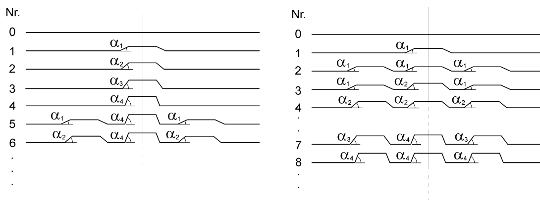
Abbildung 62: Werkzeugentwurf A (links) und Werkzeugentwurf B (rechts)
