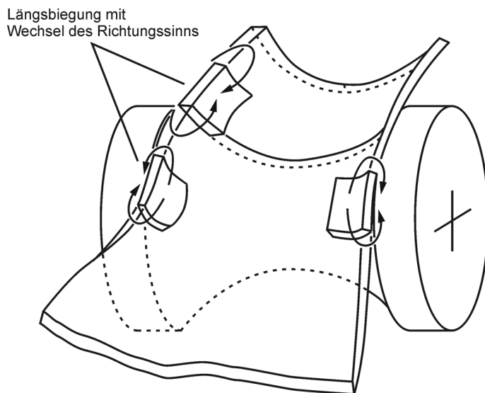
Abbildung 5: Beanspruchung des Werkstoffs während der Umformung
