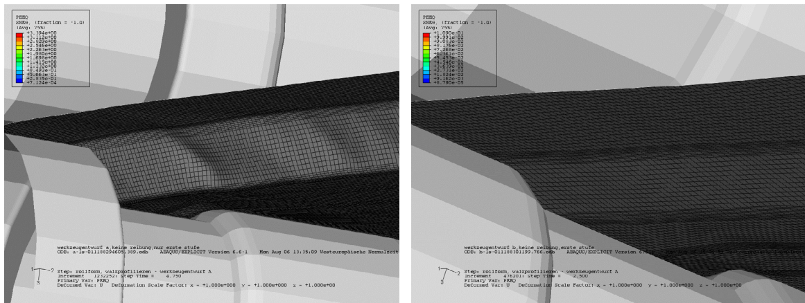
Abbildung 74: Einfallen plastischer Beulen im Steg bei Entwurf A (links) und elastischer Beulen bei Entwurf B (rechts)
