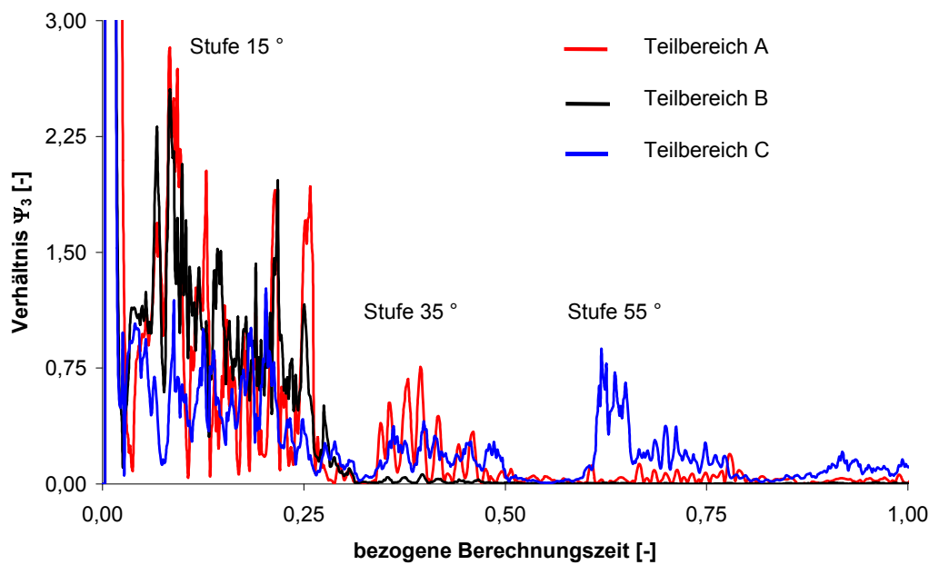
Abbildung 47: Verlauf des Verhältnisses \Psi_3 – Symmetriebedingungen und Freiheitsgrad in 3 – Richtung gehalten
