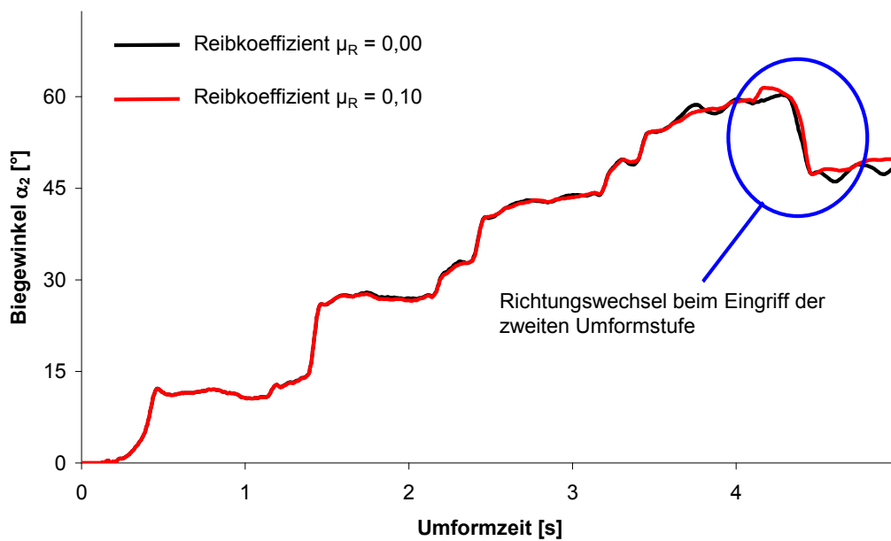
Abbildung 66: Verlauf des Biegewinkels \alpha_2 bei Entwurf A
