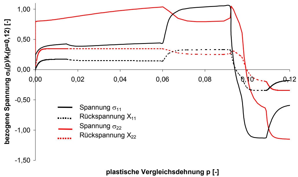
Abbildung 41: Verlauf der Spannungskomponenten \sigma_{ii} und der Rückspannungskomponenten X_{ii}
