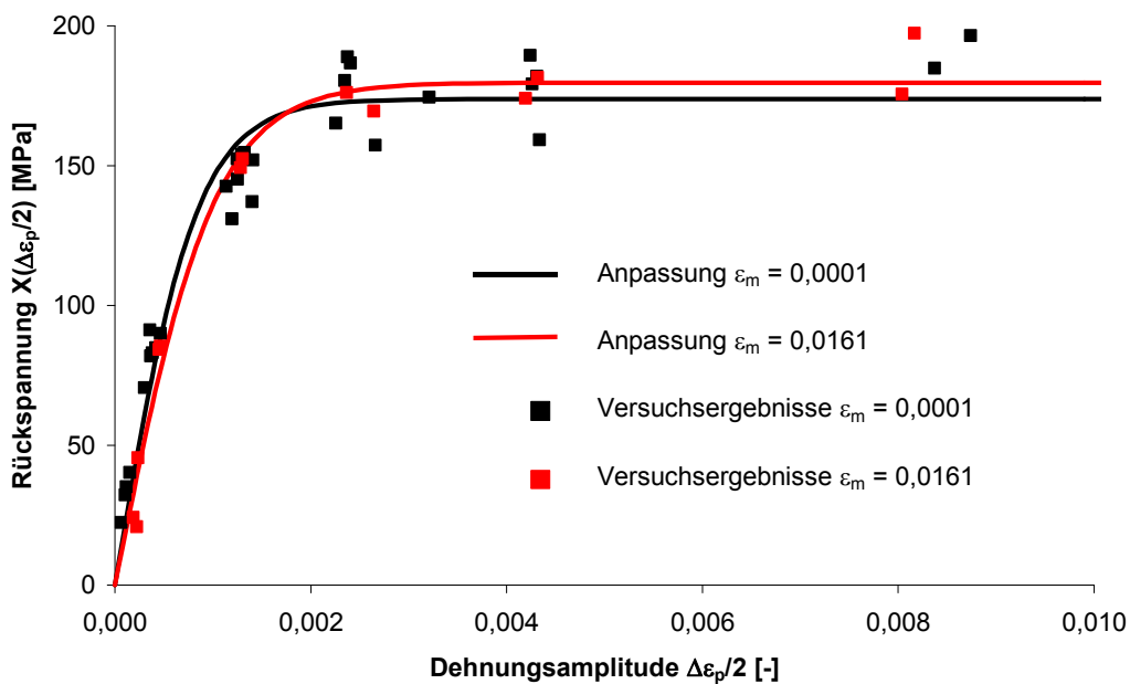
Abbildung 22: Rückspannung X in Abhängigkeit der Dehnungsamplitude \Delta\epsilon_p/2 bei unterschiedlicher Mitteldehnung \epsilon_m
