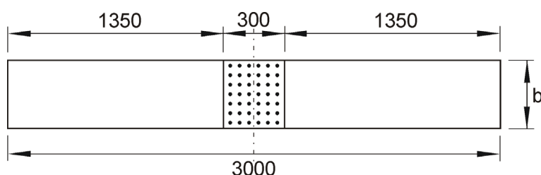
Abbildung 56: Lage der Formänderungsmessung
