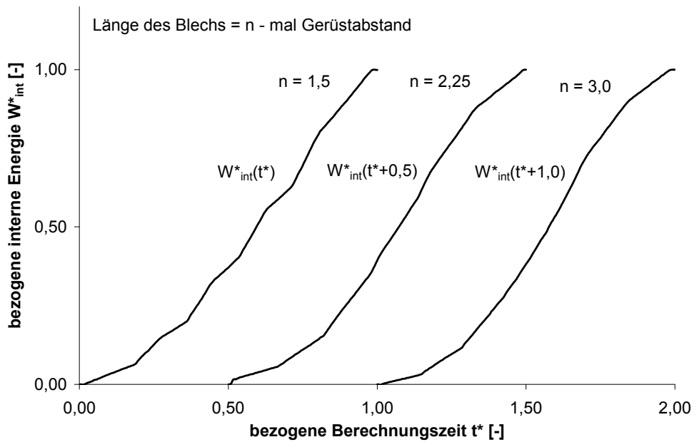
Abbildung 50: Einfluss der Länge des Blechabschnitts im Modell auf den Verlauf der bezogenen internen Energie
