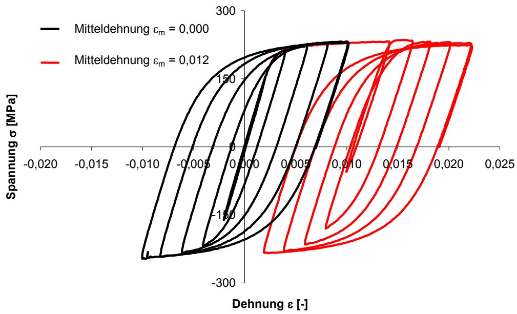
Abbildung 26: Einfluss der Mitteldehnung auf das Verfestigungsverhalten
