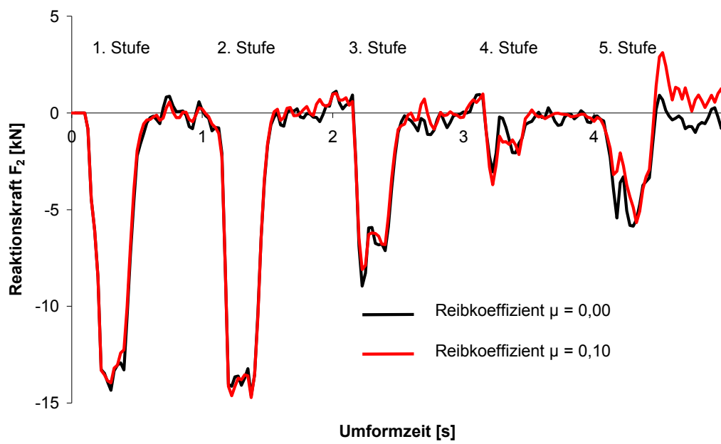
Abbildung 69: Verlauf der Reaktionskraft F_2 bei Entwurf A
