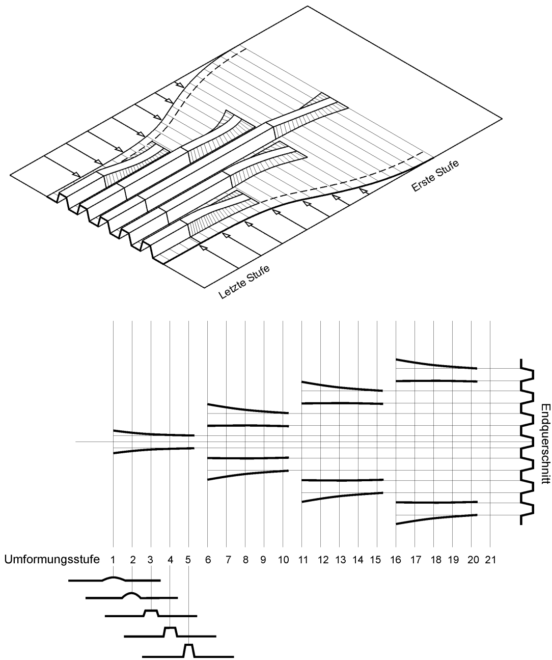
Abbildung 4: Darstellung der Stufenfolge beim Profilieren von Trapezprofilen – Ansicht (oben) und Draufsicht (unten)
