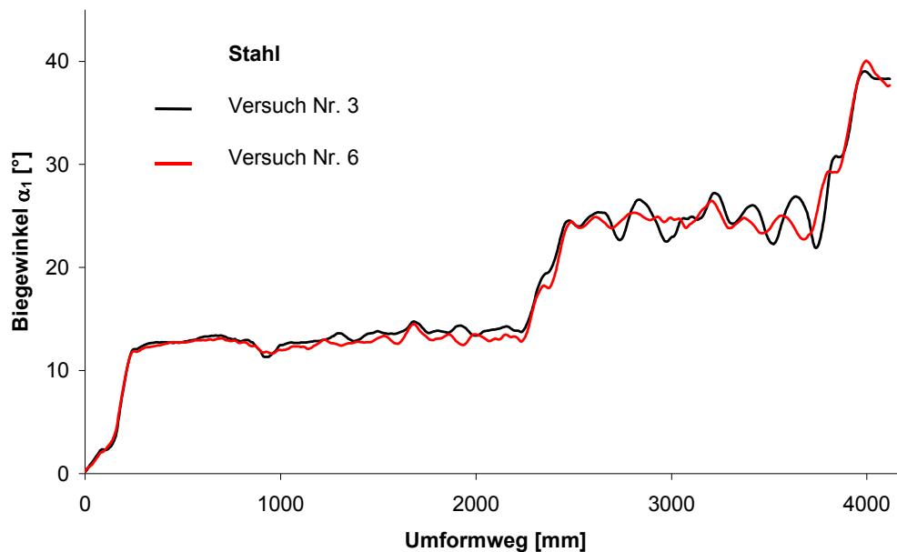
Abbildung 83: Verlauf des Biegewinkels \alpha_1
