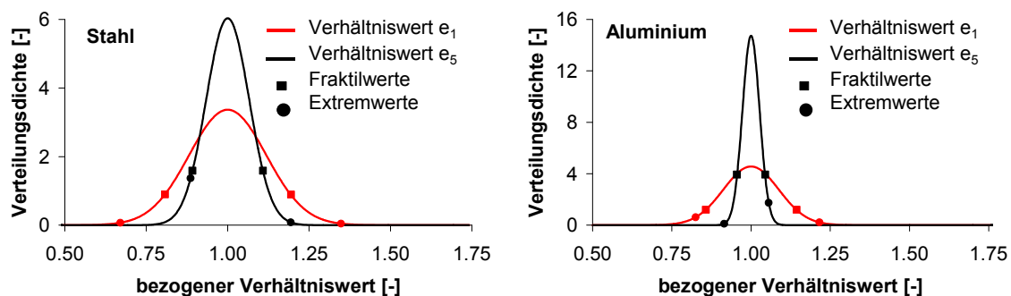
Abbildung 77: Verteilungsdichte der bezogenen Verhältniswerte
