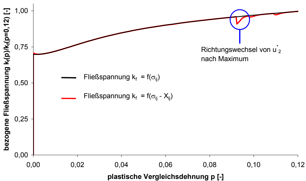
Abbildung 40: Verlauf der Fließspannung k_f in Abhängigkeit des Stoffgesetzes
