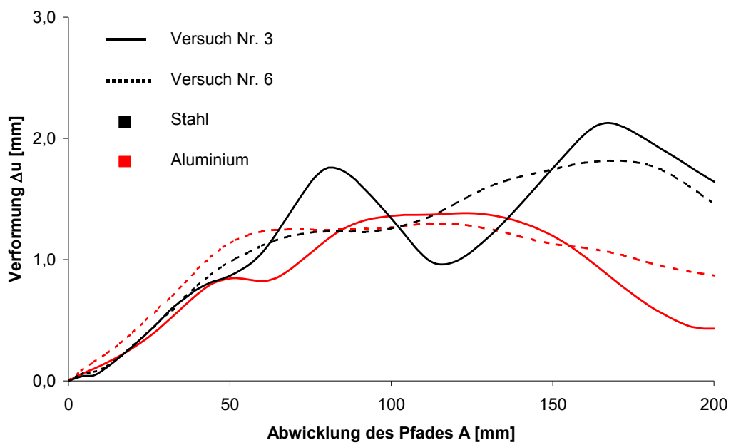
Abbildung 82: Verformungen \Delta u entlang des Pfades A
