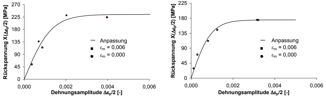
Abbildung 92: Kinematische Verfestigung - Probe sa01 (links) und Probe sa02 (rechts)
