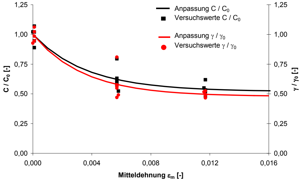
Abbildung 29: Änderung der Parameter C und \gamma in Abhängigkeit der Mitteldehnung \epsilon_m
