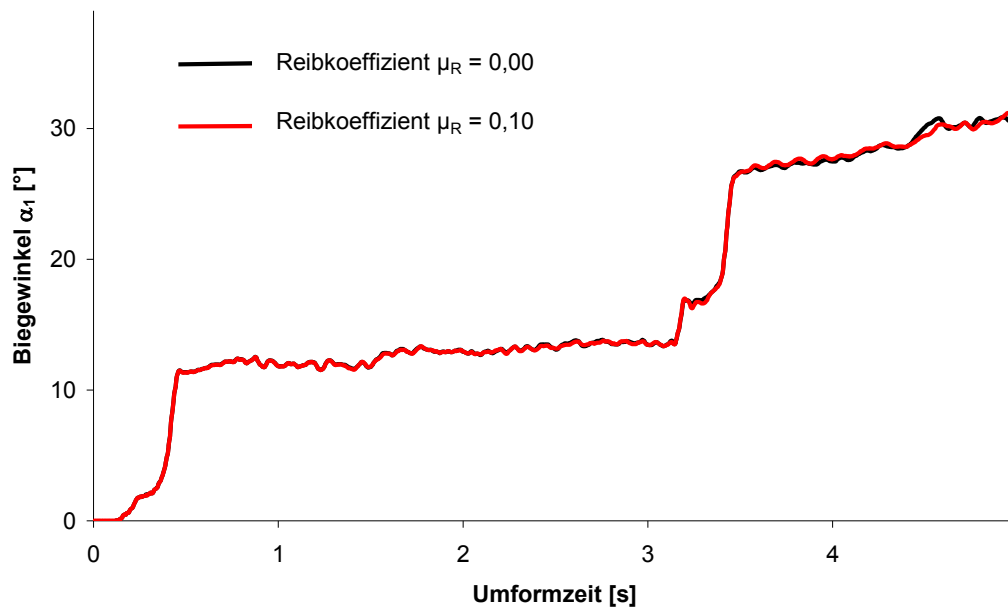
Abbildung 67: Verlauf des Biegewinkels \alpha_1 bei Entwurf B
