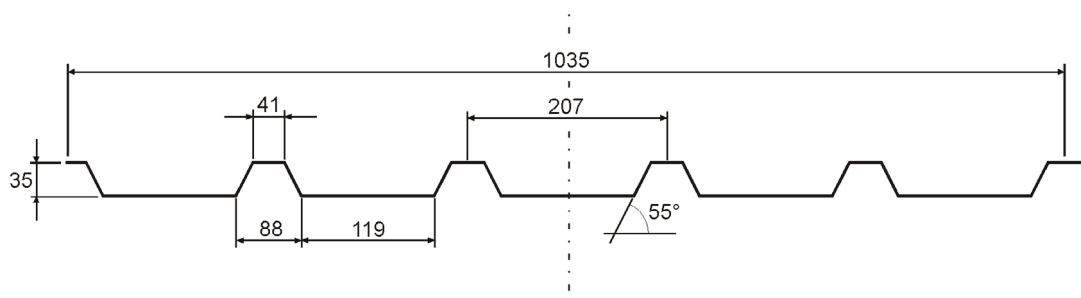
Abbildung 61: Nominelle Abmessungen des Trapezprofils Typ 35/207
