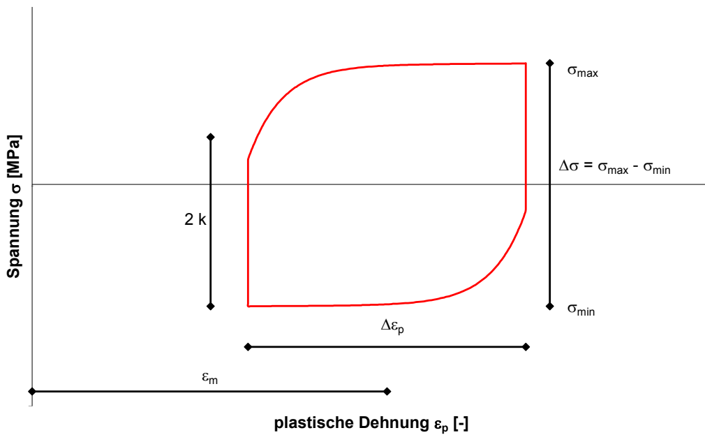
Abbildung 11: Definition der Lastwechselversuche
