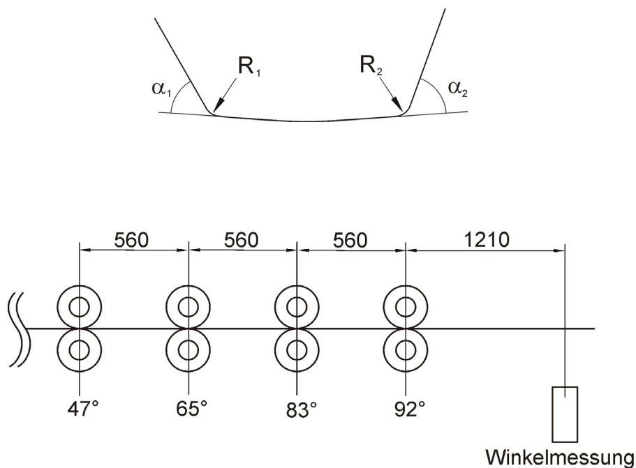
Abbildung 58: Definition der Biegewinkel (oben) und Messstelle für die kontinuierliche Messung der Biegewinkel (unten)
