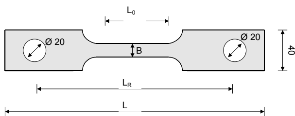
Abbildung 10: Probenform und Vorgaben hinsichtlich der Abmessungen der Probekörper
