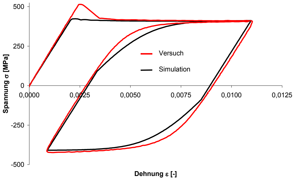
Abbildung 31: Vergleich berechneter und experimentell bestimmter Spannungs-Dehnungshysterese an Stahlprobe sa02
