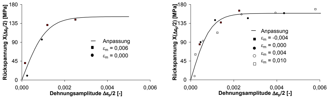
Abbildung 93: Kinematische Verfestigung - Probe sa05 (links) und Probe sa07 (rechts)
