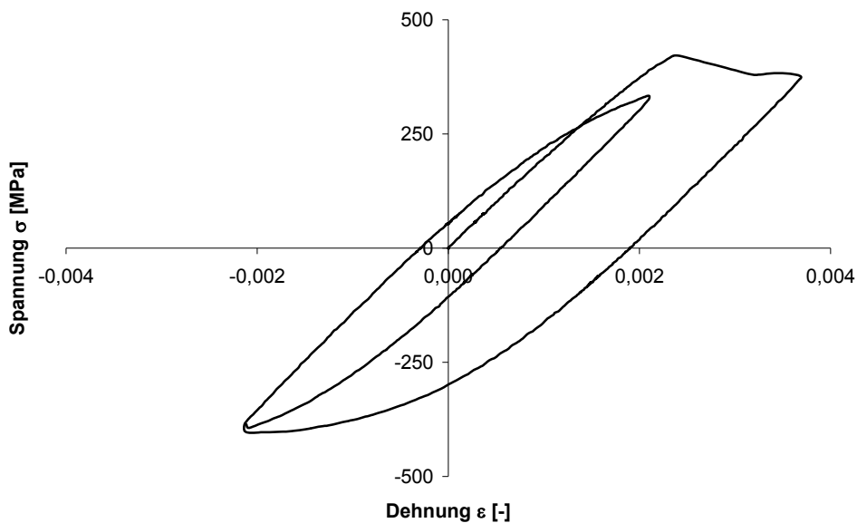
Abbildung 18: Kleine Dehnungsamplitude bei Mitteldehnung \varepsilon_m \approx 0 bei einem Stahl mit ausgeprägter Streckgrenze
