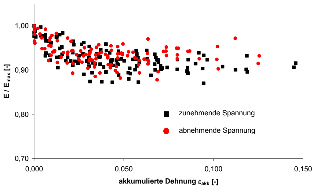
Abbildung 25: Steigung des elastischen Anteils in Abhängigkeit der akkumulierten Dehnung
