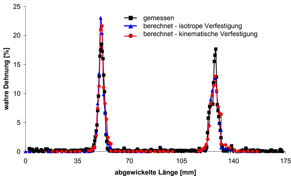
Abbildung 59: Formänderungen an Profilaußenseite in Blechdicke 1,00 mm
