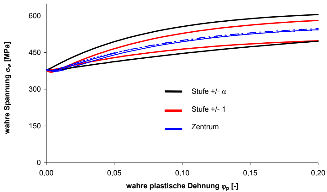
Abbildung 78: Fließkurven von Stahl für die Parameterstudie
