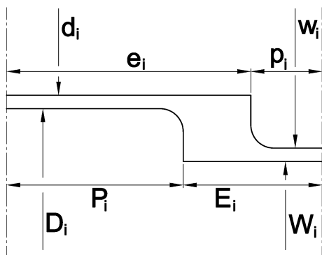
Abbildung 103: Maßbezeichnungen der Werkzeuge eines allgemeinen Profiltyps
