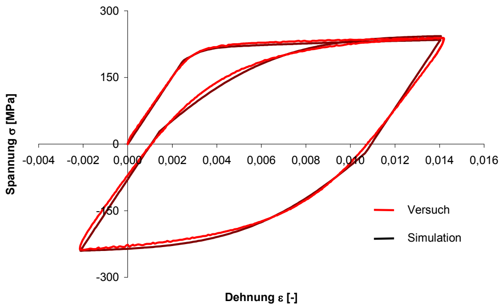
Abbildung 33: Vergleich berechneter und experimentell bestimmter Spannungs-Dehnungshysterese an Aluminiumprobe ab11
