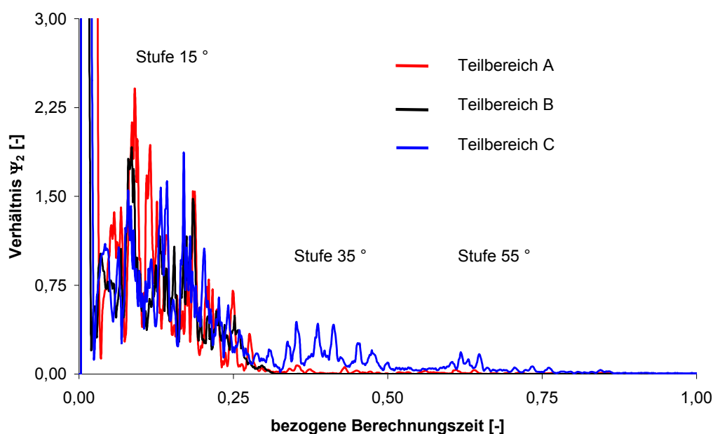
Abbildung 44: Verlauf des Verhältnisses \Psi_2 –nur Symmetriebedingungen
