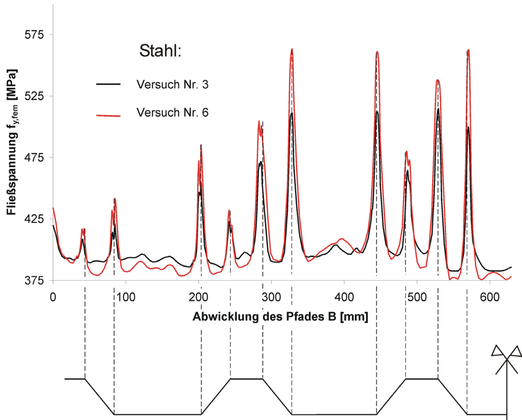
Abbildung 84: Verlauf der Fließspannung entlang Pfad B
