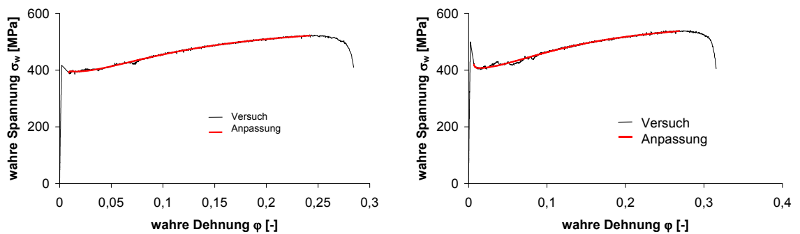
Abbildung 88: Wahre Spannungs-Dehnungs-Kurve der Probe sa02 in Walzrichtung (links) und quer zur Walzrichtung (rechts)
