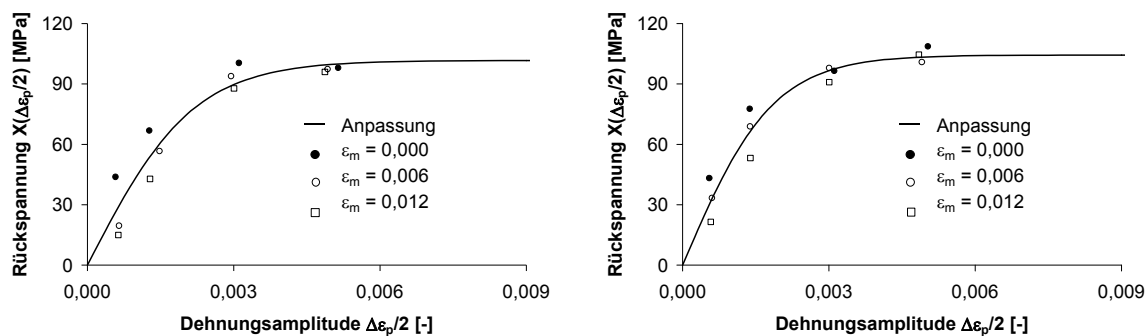
Abbildung 100: Kinematische Verfestigung - Probe as20 (links) und Probe as23 (rechts)
