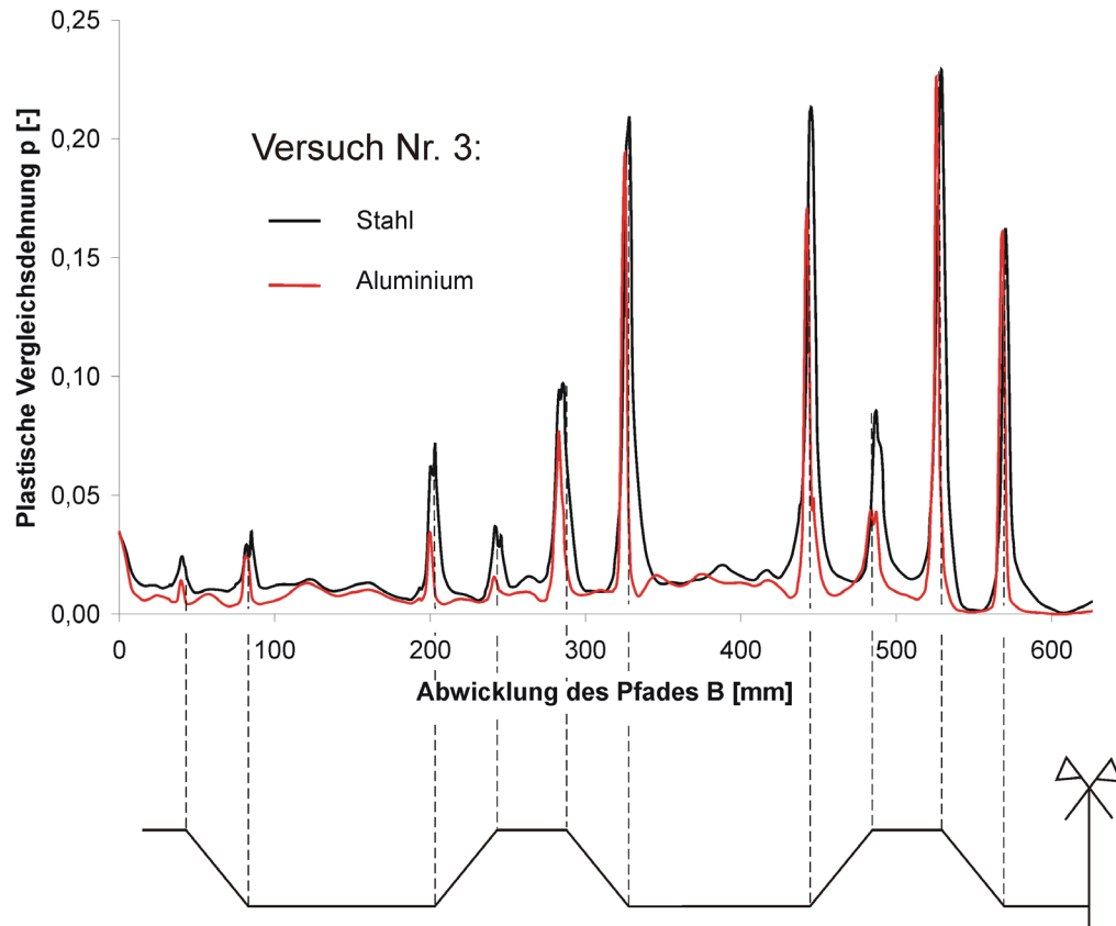
Abbildung 86: Verlauf der plastischen Vergleichsdehnung p
