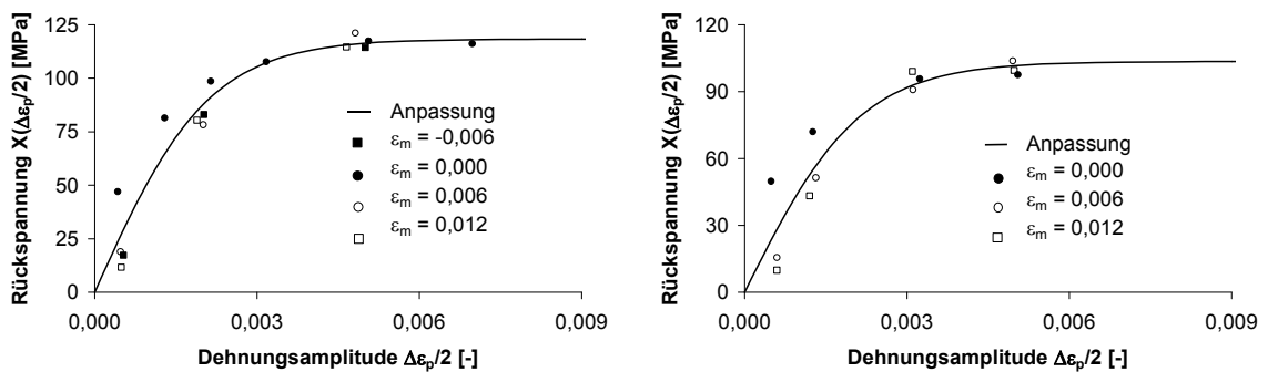
Abbildung 99: Kinematische Verfestigung - Probe ab11 (links) und Probe ab12 (rechts)
