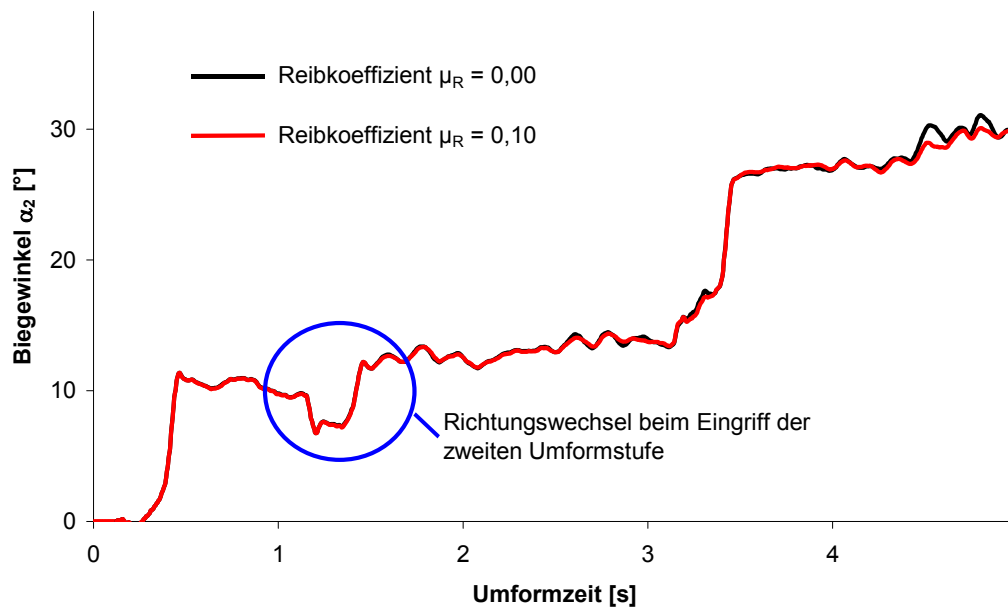
Abbildung 68: Verlauf des Biegewinkels \alpha_2 bei Entwurf B
