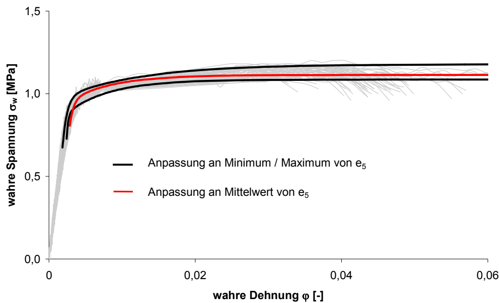
Abbildung 13: Fließkurven und rechnerisch angepasste Kurven bei Aluminium
