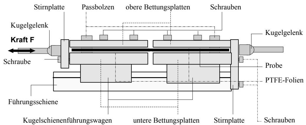
Abbildung 9: Konstruktion der Prüfvorrichtung
