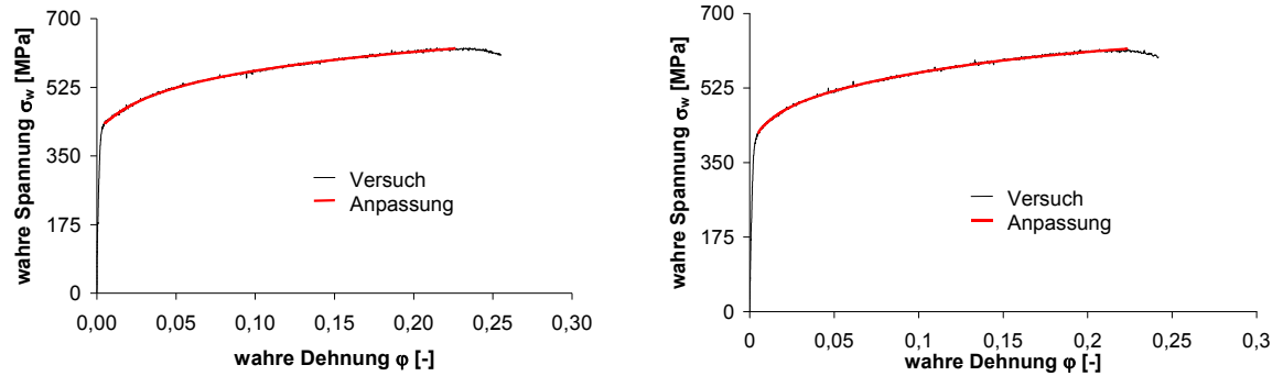
Abbildung 87: Wahre Spannungs-Dehnungs-Kurve der Probe sa01 in Walzrichtung (links) und quer zur Walzrichtung (rechts)
