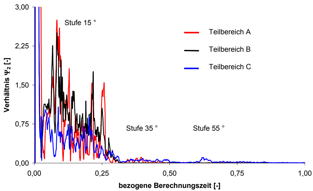
Abbildung 45: Verlauf des Verhältnisses \Psi_2 – Symmetriebedingungen und Freiheitsgrad in 3 – Richtung gehalten
