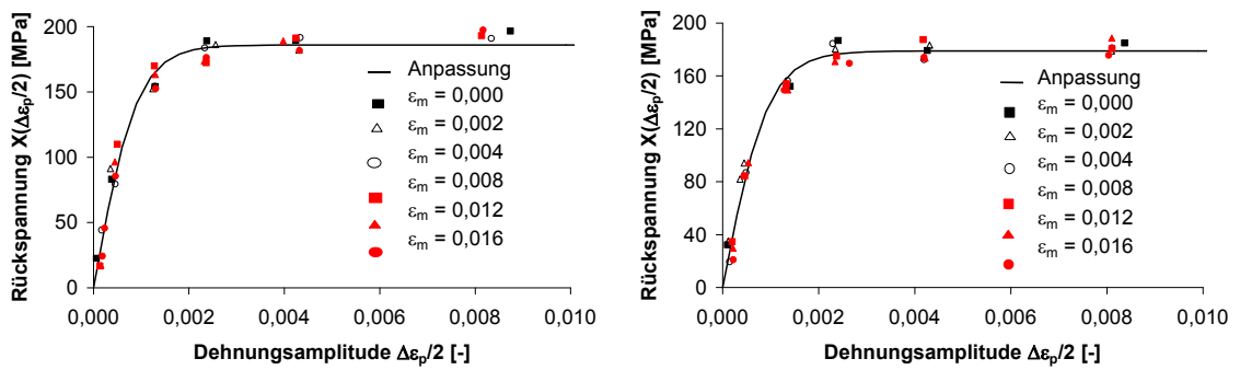
Abbildung 94: Kinematische Verfestigung - Probe sa10 (links) und Probe sa11 (rechts)
