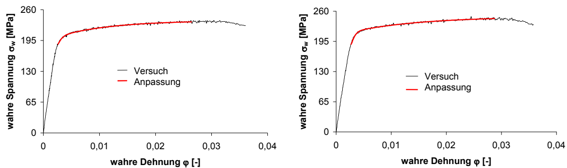
Abbildung 95: Wahre Spannungs-Dehnungs-Kurve der Probe ab11 in Walzrichtung (links) und quer zur Walzrichtung (rechts)
