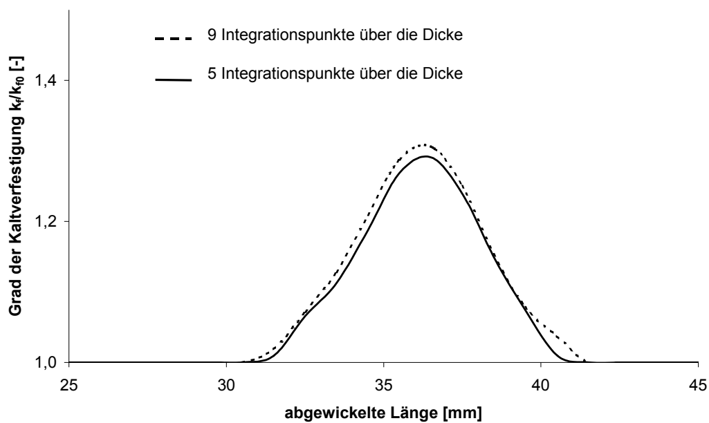
Abbildung 52: Grad der Kaltverfestigung in Abhängigkeit der Anzahl der Integrationspunkte
