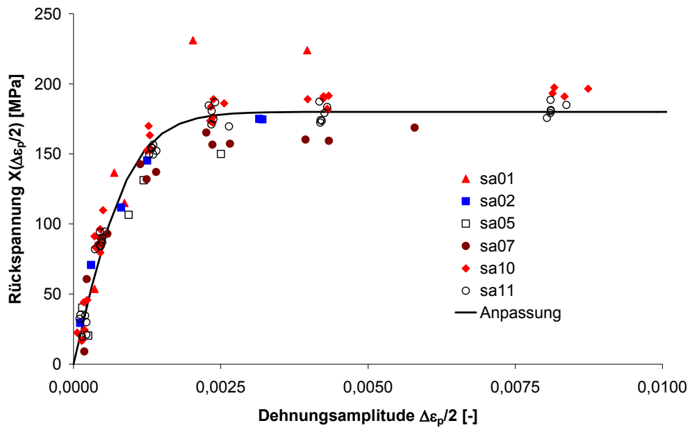
Abbildung 21: Rückspannung X in Abhängigkeit der Dehnungsamplitude \Delta\epsilon_p/2
