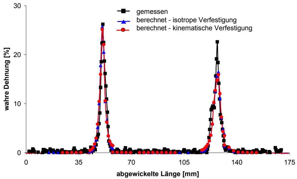
Abbildung 60: Formänderungen an Profilaußenseite in Blechdicke 1,25 mm
