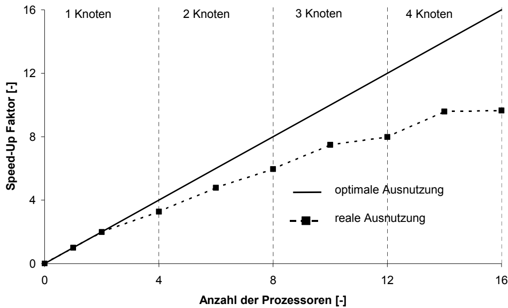
Abbildung 53: Effizienz des Parallelrechners
