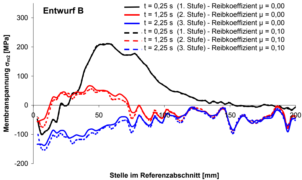
Abbildung 73: Verteilung der Membranspannung beim Einlauf in verschiedene Stufen
