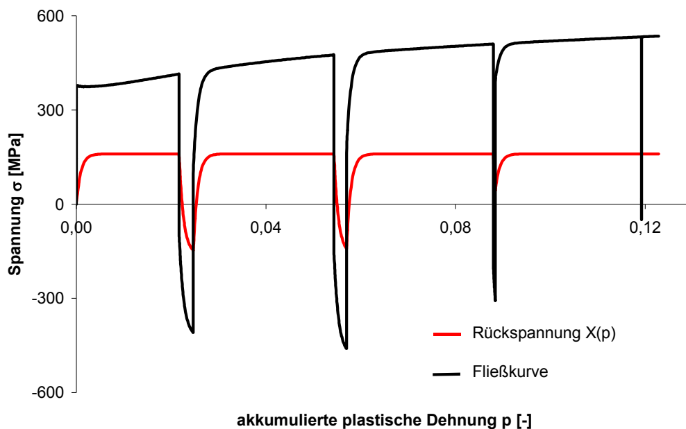
Abbildung 38: Verlauf der Fließkurve und der Rückspannung X in Abhängigkeit der akkumulierten plastischen Dehnung
