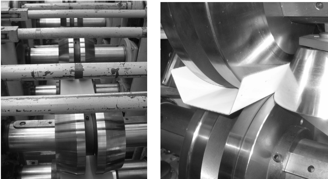
Abbildung 54: Ansicht der Profileranlage des PtU (links) und Blech bei Austritt aus der 4. Biegestufe (rechts)
