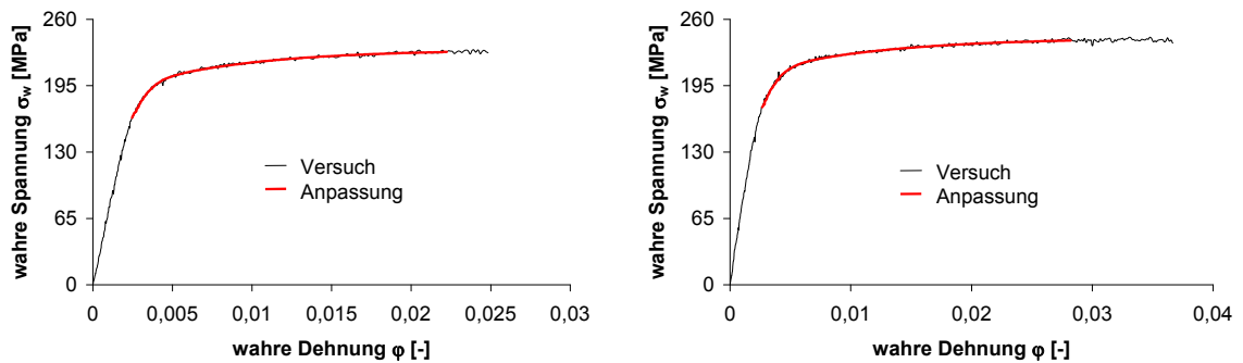
Abbildung 98: Wahre Spannungs-Dehnungs-Kurve der Probe as23 in Walzrichtung (links) und quer zur Walzrichtung (rechts)
