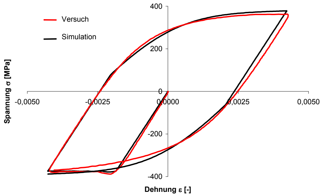
Abbildung 30: Vergleich berechneter und experimentell bestimmter Spannungs-Dehnungshysterese an Stahlprobe sa05
