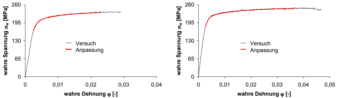
Abbildung 97: Wahre Spannungs-Dehnungs-Kurve der Probe as20 in Walzrichtung (links) und quer zur Walzrichtung (rechts)
