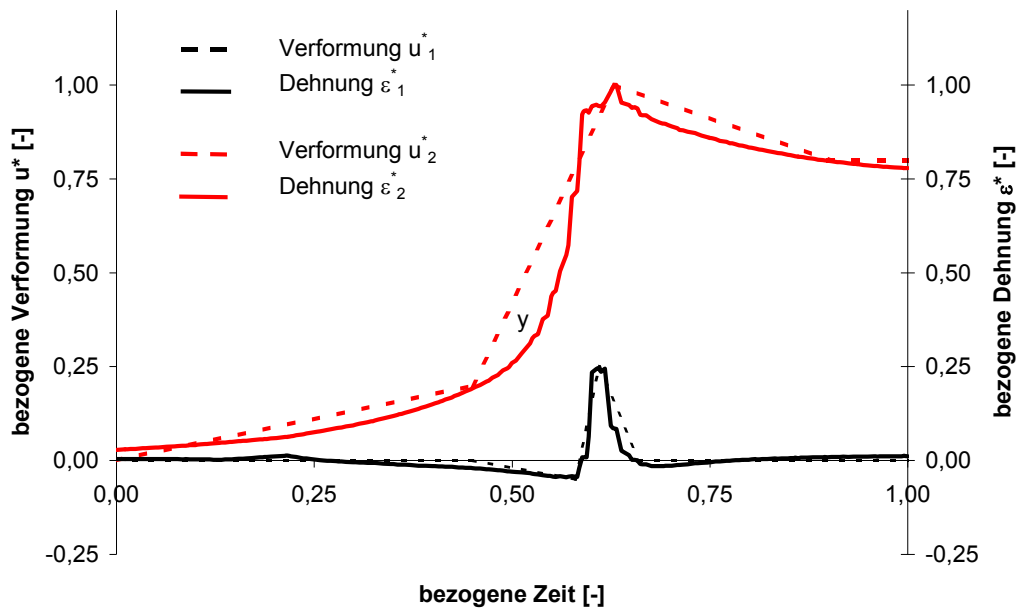
Abbildung 39: Übergang von einem ein- auf einen mehrachsigen Spannungszustand
