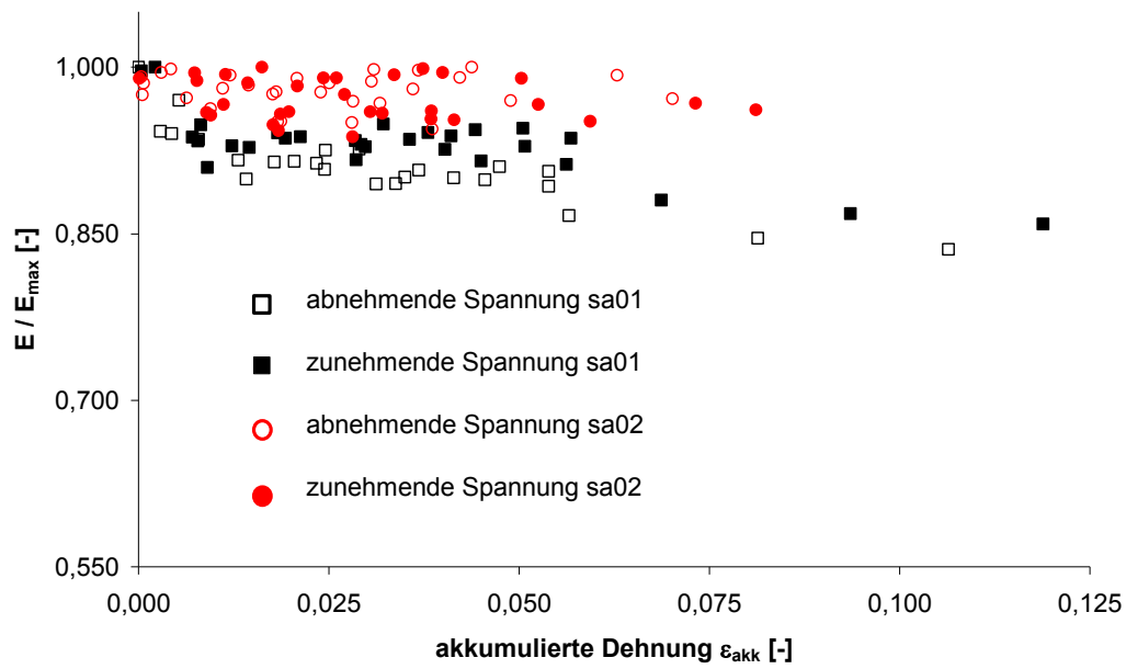
Abbildung 19: Steigung des elastischen Anteils in Abhängigkeit der akkumulierten Dehnung
