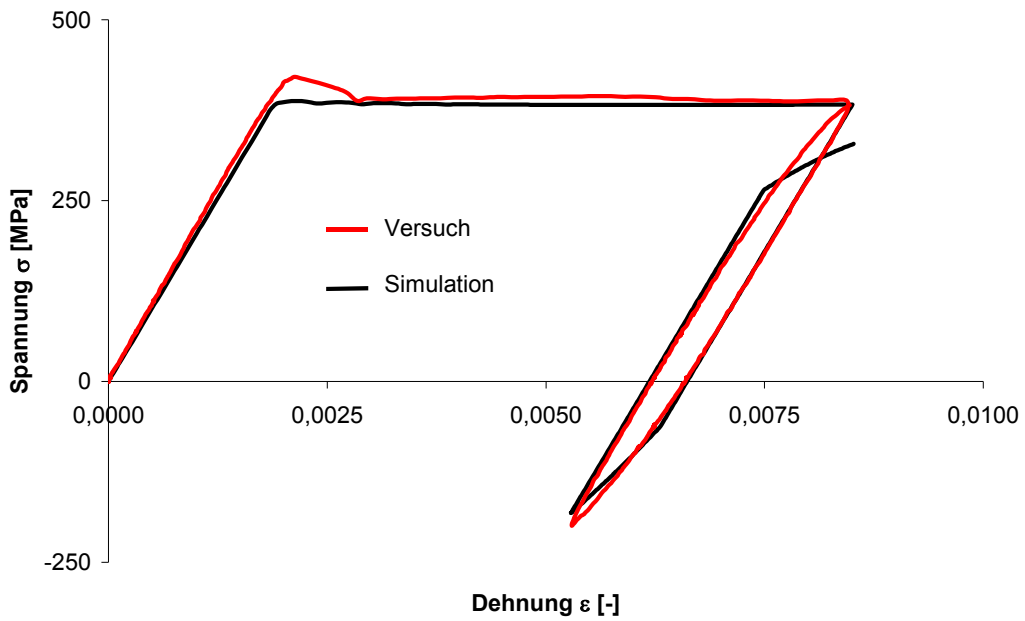
Abbildung 32: Vergleich berechneter und experimentell bestimmter Spannungs-Dehnungshysterese an Stahlprobe sa07
