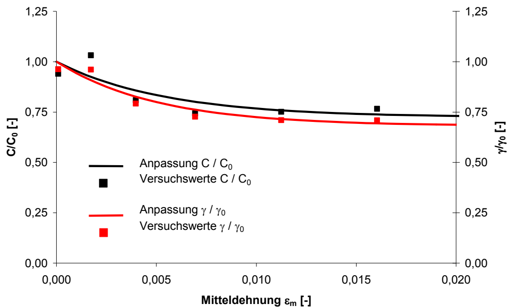
Abbildung 23: Änderung der Parameter C und \gamma in Abhängigkeit der Mitteldehnung \epsilon_m
