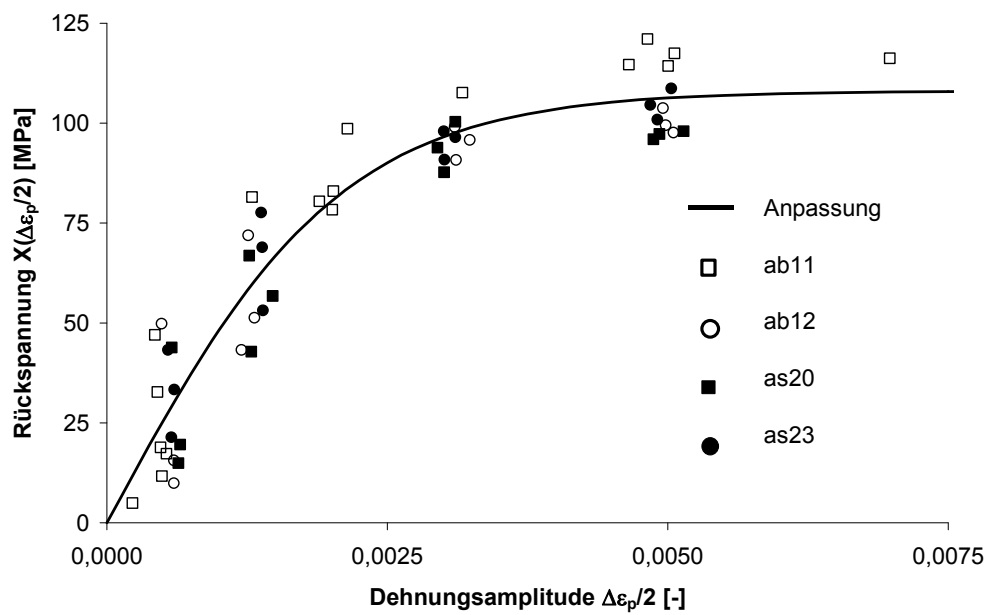
Abbildung 27: Rückspannung X in Abhängigkeit der Dehnungsamplitude \Delta\varepsilon/2
