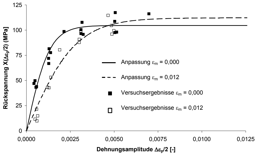
Abbildung 28: Rückspannung X in Abhängigkeit der Dehnungsamplitude \Delta\epsilon/2 bei unterschiedlicher Mitteldehnung \epsilon_m
