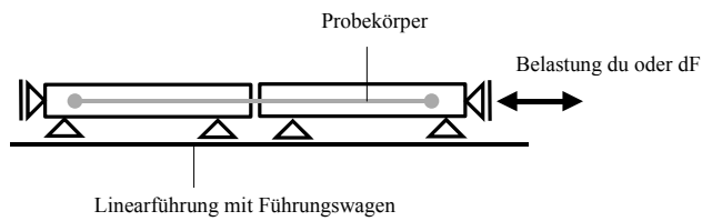
Abbildung 8: Schematische Darstellung des Konstruktionsprinzips
