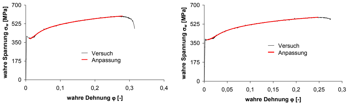
Abbildung 89: Wahre Spannungs-Dehnungs-Kurve der Probe sa05 in Walzrichtung (links) und quer zur Walzrichtung (rechts)
