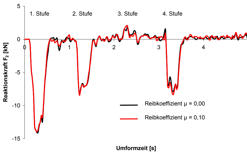
Abbildung 70: Verlauf der Reaktionskraft F_2 bei Entwurf B
