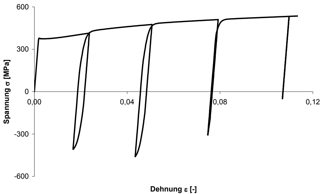
Abbildung 37: Anpassung der isotropen Verfestigungskomponente an den Umformprozess
