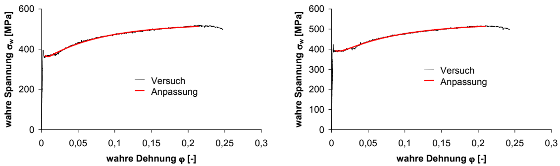
Abbildung 90: Wahre Spannungs-Dehnungs-Kurve der Probe sa07 in Walzrichtung (links) und quer zur Walzrichtung (rechts)
