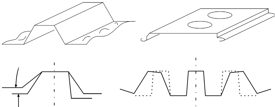
Abbildung 6: Häufig auftretende geometrische Defekte – Randwelligkeit (oben links), Beulen (oben rechts) und unterschiedliche Rückfederungseffekte (unten)
