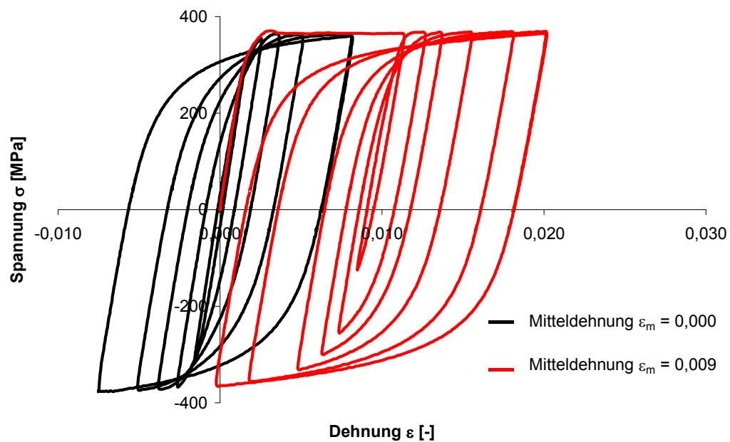
Abbildung 20: Einfluss der Mitteldehnung auf das Verfestigungsverhalten
