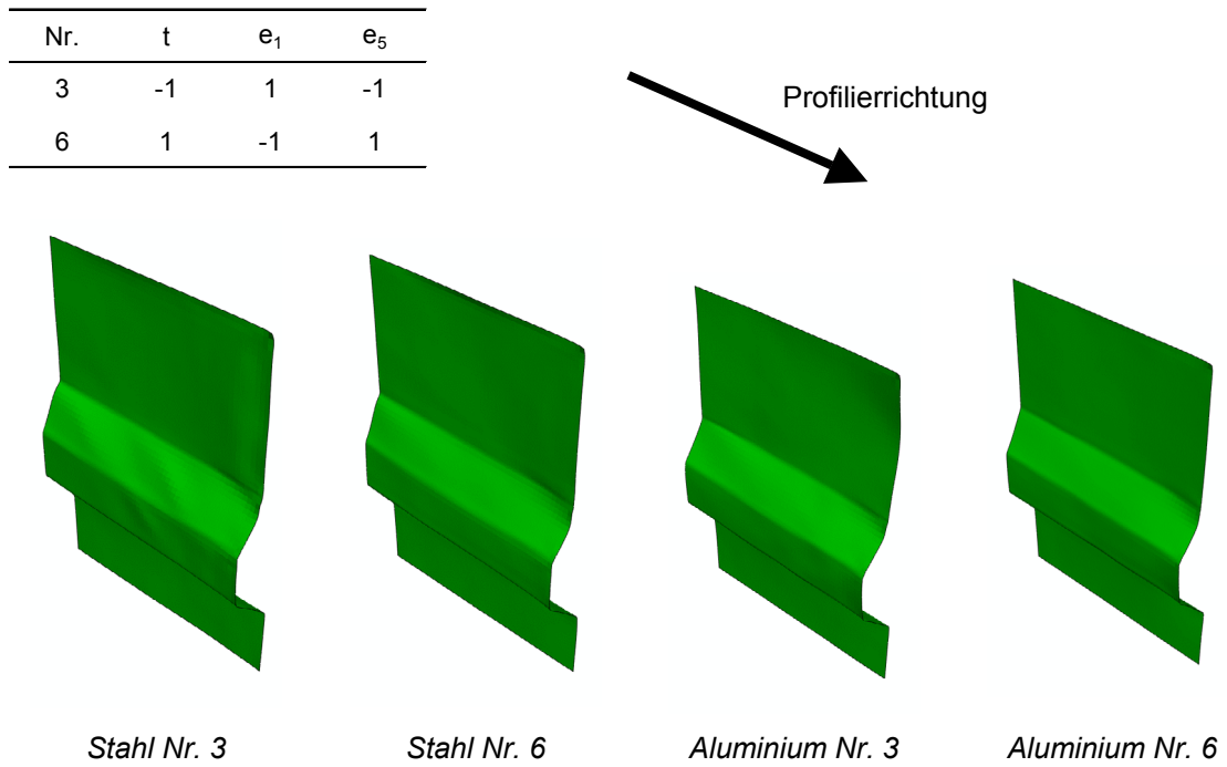
Abbildung 81: Ansicht der Referenzfläche ausgewählter Versuche
