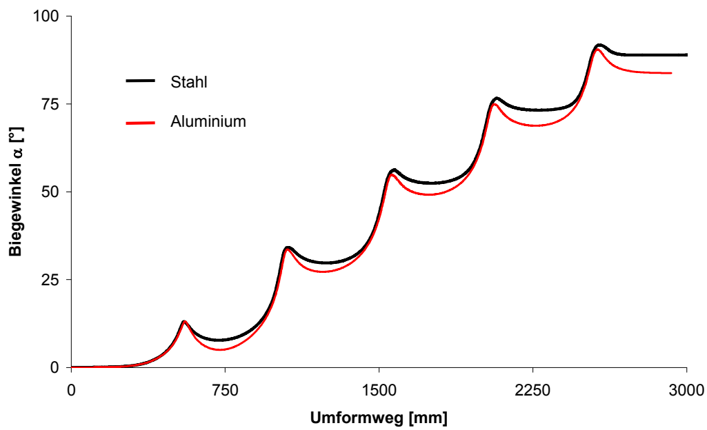
Abbildung 15: Verlauf des Biegewinkels während des Herstellprozess eines U-Profiles aus Stahl und Aluminium
