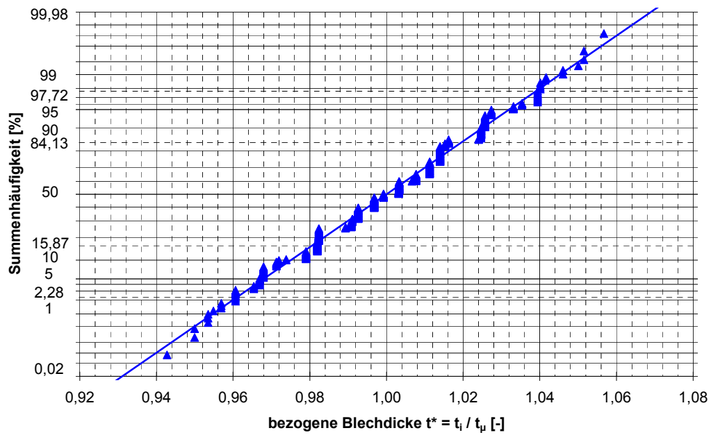
Abbildung 101: Summenhäufigkeitsverteilung der bezogenen Blechdicke t^*
