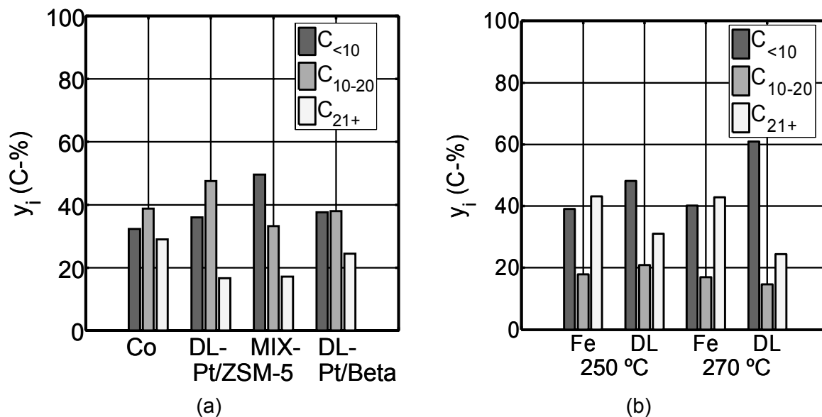
Abb. 9.4: Bifunktionaler Katalysator-, Anordnungs- und Temperatureinfluss auf die Kohlenwasserstoffausbeute (C-Basierte). (a) Co-basierte Anordnungen, (b) Fe-basierte Anordnungen. DL: Zweischichten, MIX: Physicalische Mischung. Reaktionsbedingungen: (p_{H_2}/p_{CO})_{\text{ein}} = 2 , p = 1 \text{ MPa} , \tau_{\text{mod}} = 4000 \text{ kg}\cdot\text{s}/\text{m}^3 (Bezug auf m_{\text{FT-Kat.}} ), m_{\text{HP-Kat.}} / m_{\text{FT-Kat.}} = 0,75 .
