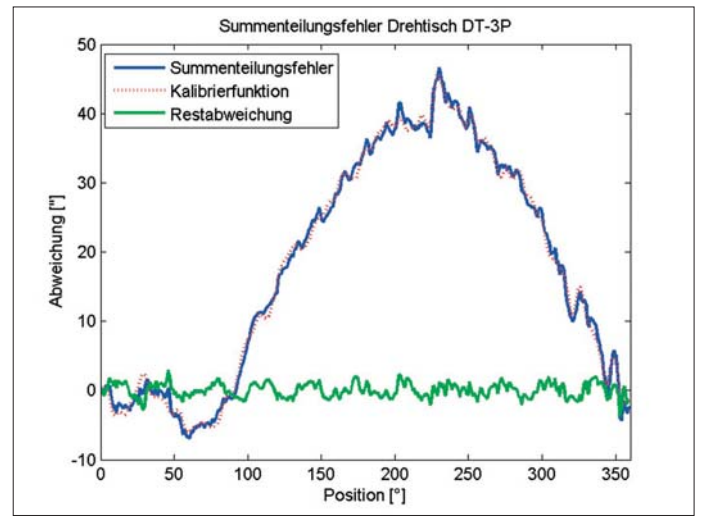
5: Summenteilungsfehler mit F_{\text{Kali}}(x) und Restabweichung für DT-3P.
