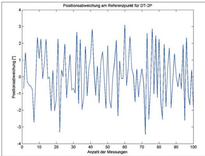
4: Positionenabweichung DT-2P.
