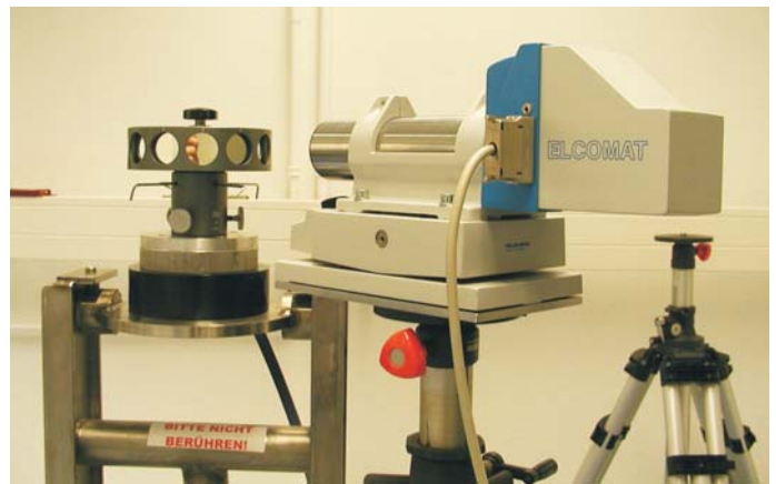
2: Drehtisch mit Spiegelpolygon und Autokollimator.
