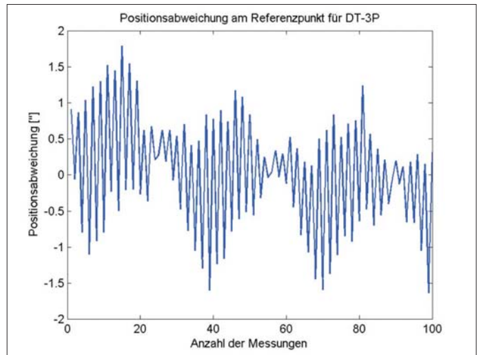
3: Positionsabweichung DT-3P.
