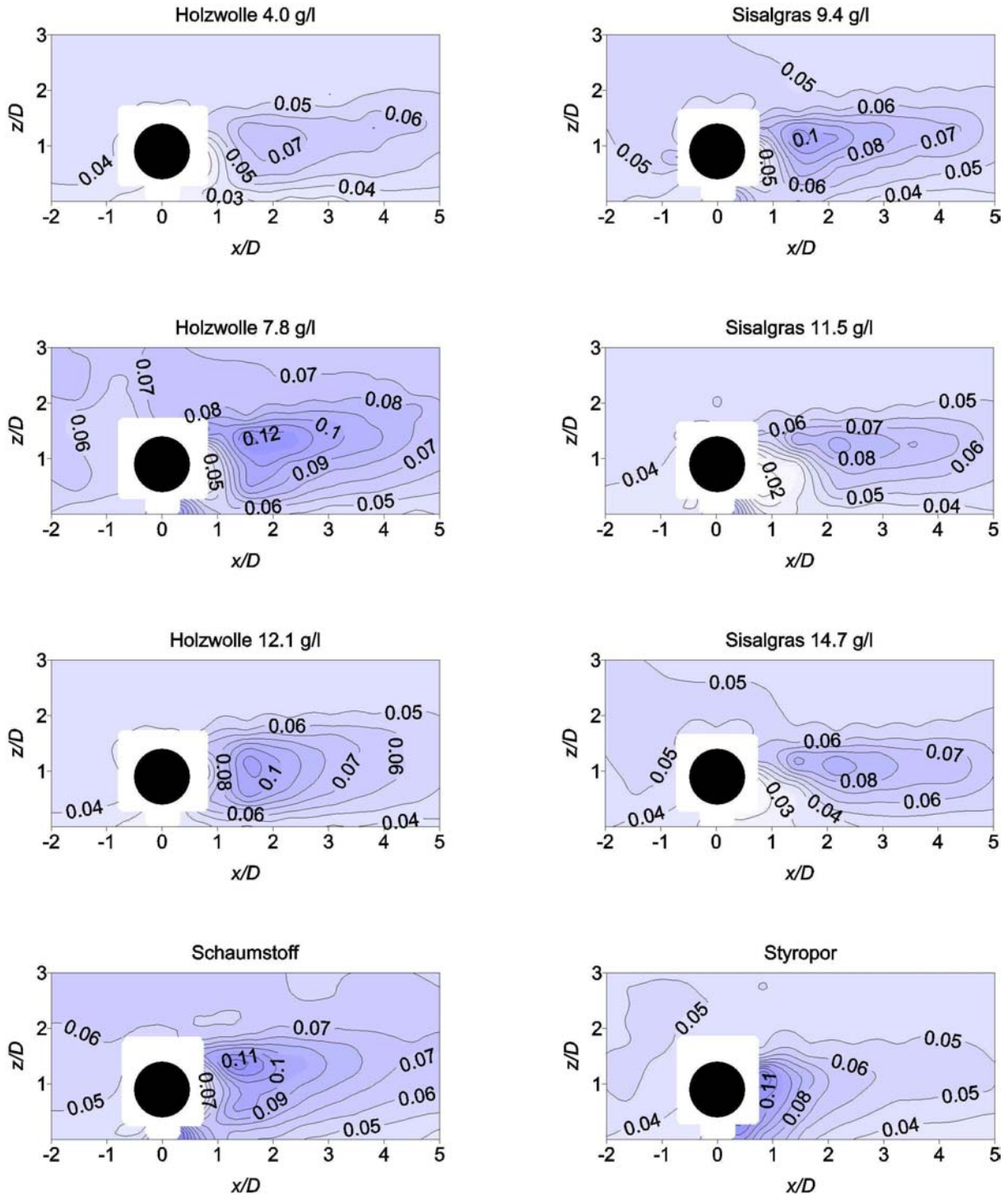
Abb. 6: Normierte Maße für die turbulente kinetische Energie tke^+ = (u^2 + w^2)/u^2(z_{BO}) .
