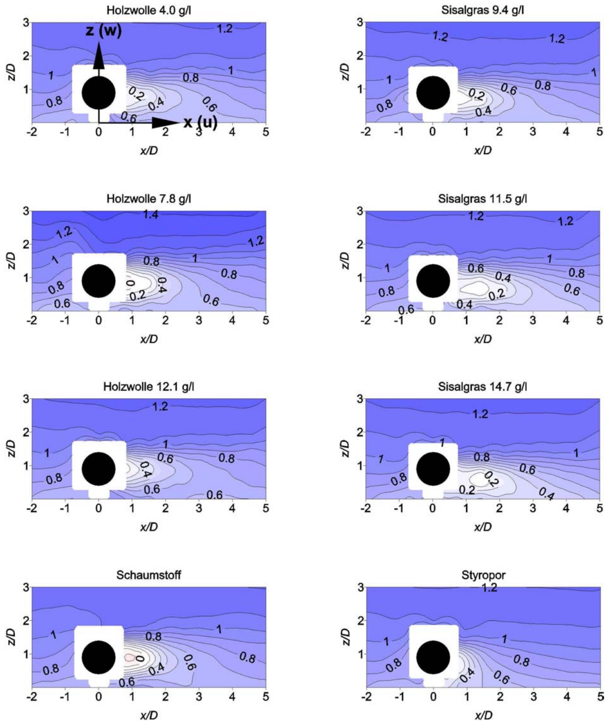
Abb. 4: Normierte Horizontalgeschwindigkeiten u^+ = u/u(z_{B0}) .
