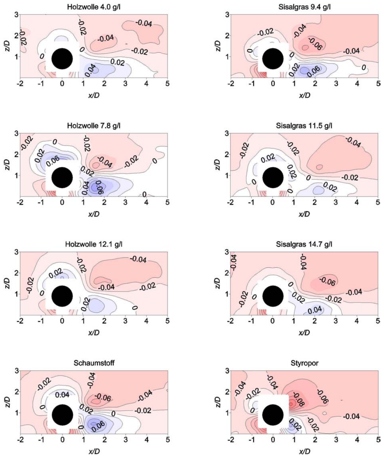
Abb. 5: Normierte Vertikalgeschwindigkeiten w^+ = w/u(z_{B0}) .
