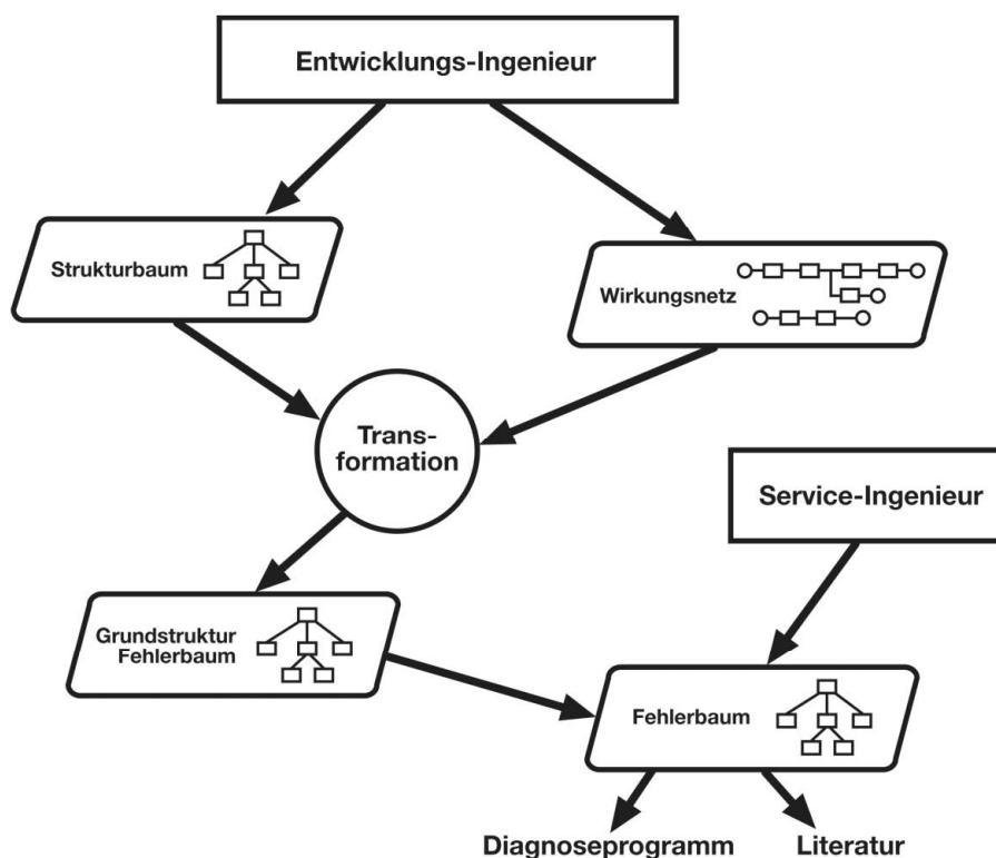
Abbildung 3-21 WDS- Erstellungssystem
