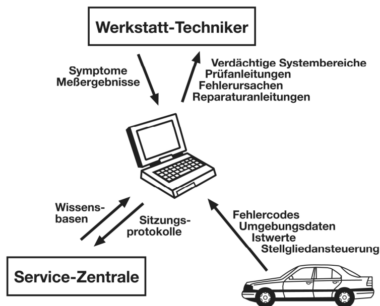
Abbildung 3-20 WDS - Laufzeitsystem
