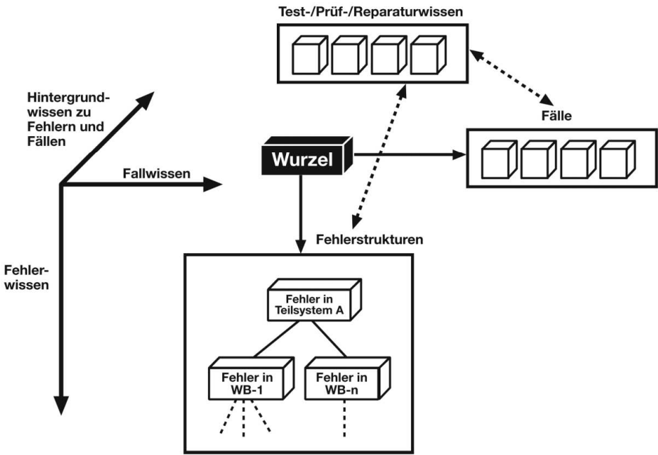
Abbildung 3-25 WDS- Diagnosemodell
