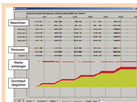
Animation der Interaktion von Personal und Betriebsmitteln in einer Fertigung (Simulationsverfahren FEMOS)
