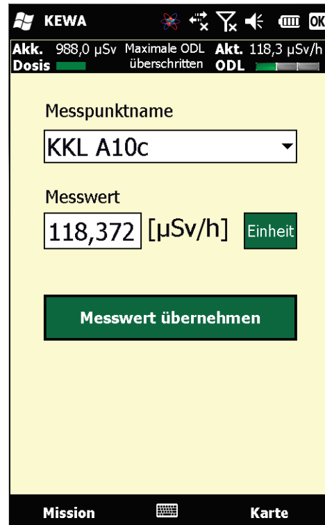
Abbildung 8: Messwerterfassung - Wert übernehmen
