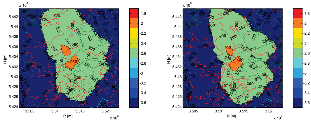
Abbildung 5: GKN II: Modellgebietsgröße mittel, Konzentrationsmaximum für die Jahre 2006 (links) 0,0157 \text{ Bq/m}^3 und 2007 (rechts) 0,0164 \text{ Bq/m}^3
