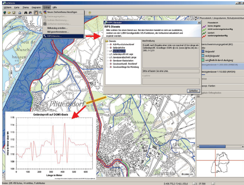
Abbildung 3: Geländeprofil im GISTerm Desktop
