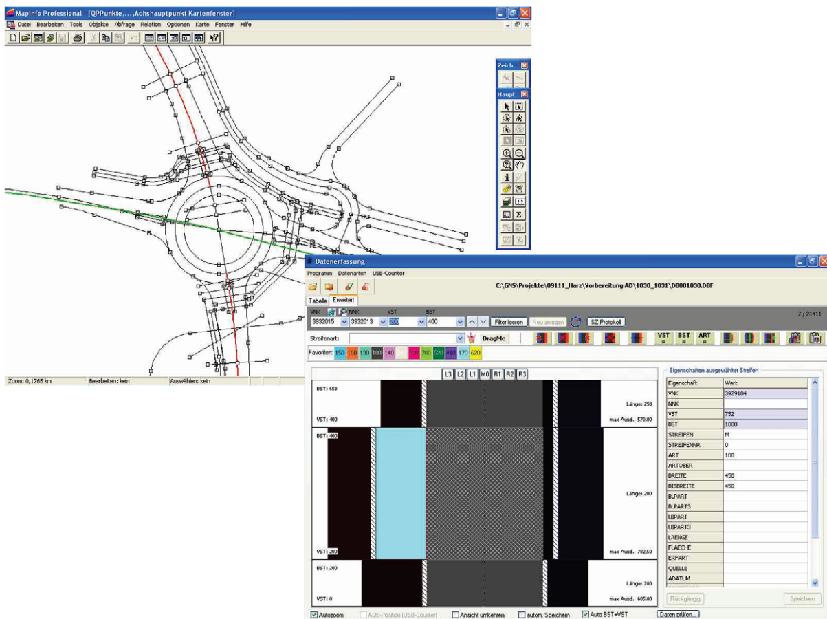
Abbildung 4: Importierter Achssatz mit Querprofilspunkten (links) und Visualisierung beispielhafter Querschnittstreifen in der Kontroll- und Bearbeitungsebene SOV (rechts)
