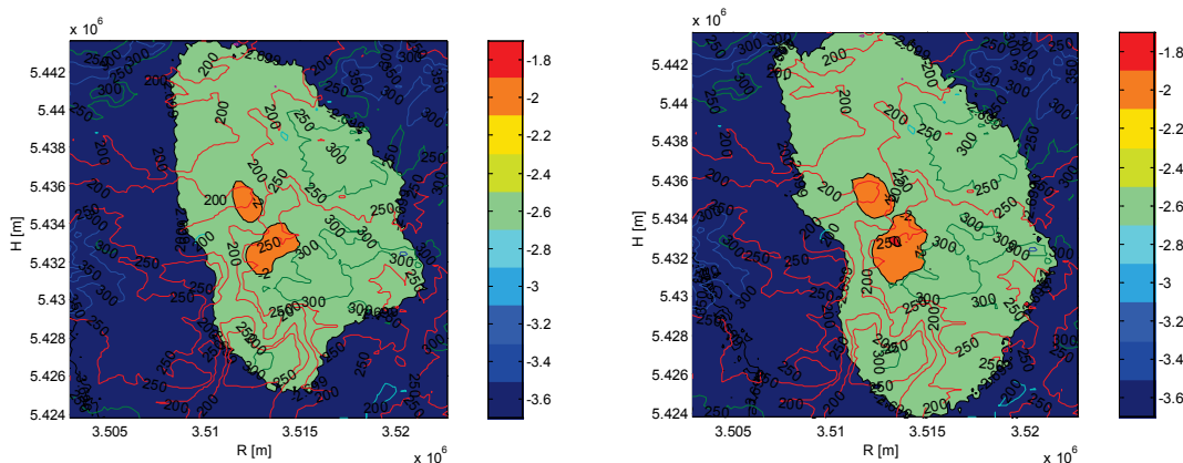
Abbildung 6: GKN II: Modellgebietsgröße mittel, Konzentrationsmaximum für die Jahre 2008 (links) 0,0166 \text{ Bq/m}^3 und 2009 (rechts) 0,0228 \text{ Bq/m}^3
