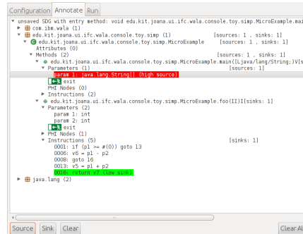
(b) annotation tab
