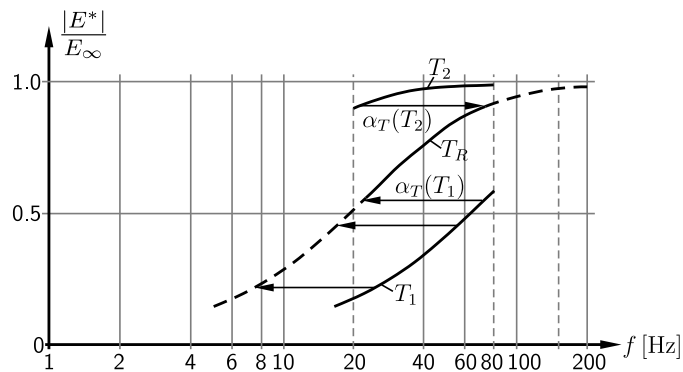
Abbildung 2.14: Temperatur-Frequenz-Äquivalenz aus [108]
