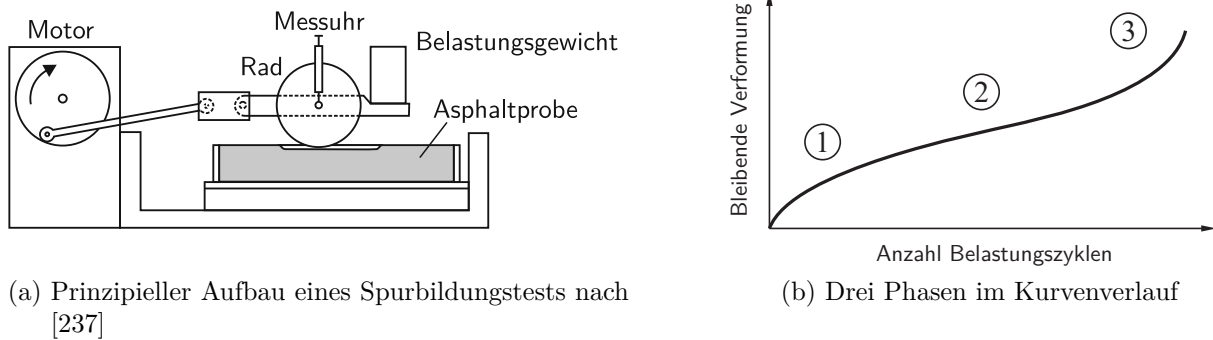
Abbildung 2.9: Spurbildungstest: (a) prinzipieller Aufbau, (b) Ergebnis des Tests
