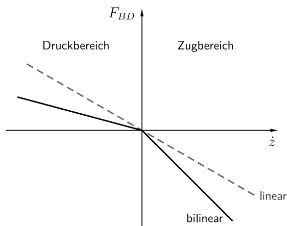
Abbildung 3.10: Bilineare Dämpfung
