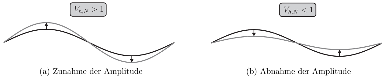
Abbildung 4.3: Änderung der Amplitude in Abhängigkeit von der Vergrößerungsfunktion für \Delta\varphi_N = 0 (schwarz: vor Belastung, grau: nach Belastung)
