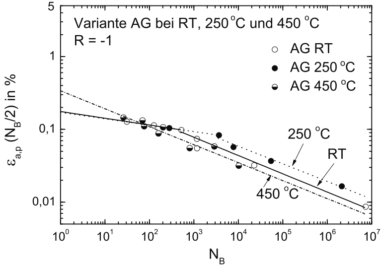
Abb. 7.46. Vergleich der Variante AG in der Manson-Coffin-Darstellung \epsilon_{a,p} über N_B bei RT, 250 °C und 450 °C
