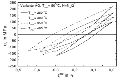
Abb. 8.40. Variante AG: \sigma_n - \epsilon_t^{me} -Hysteresen für TMF-Beanspruchung, T_{max} = 250 \text{ }^\circ\text{C} bis 400 \text{ }^\circ\text{C} , N = N_B/2
