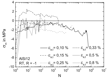
Abb. 7.4. Mittelspannungsverläufe von AISi12 bei RT für \epsilon_{a,t} 0,1 % bis 0,8 %
