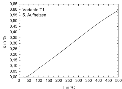
Abb. 5.4. Temperaturabhängiges Ausdehnungsverhalten der MMC-Variante T1 bis 500 ^{\circ}\text{C}
