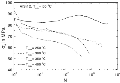
Abb. 8.4. AlSi12: \sigma_a über N für TMF-Beanspruchung mit T_{max} = 250\text{ °C} bis 400\text{ °C}
