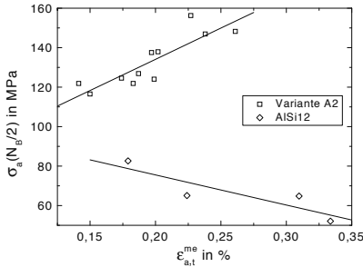
Abb. 8.31. Variante A2 und AlSi12: \sigma_a über \epsilon_{a,t}^{me} für TMF-Bbeanspruchung, T_{min} = 50^\circ C
