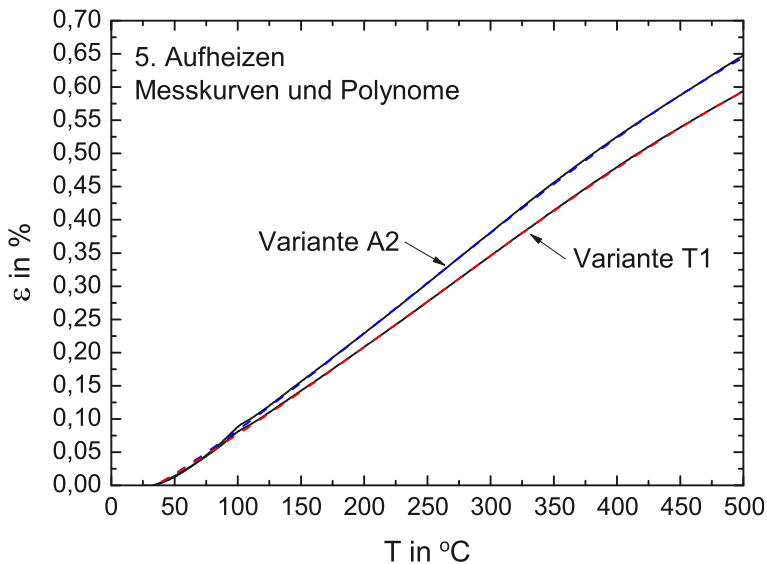
Abb. 5.13. Vergleichende Darstellung zwischen Messkurve und Polynom für die MMC-Varianten A 2 und T I
