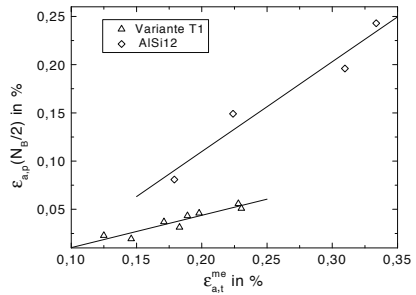
Abb. 8.92. Variante T1 und AISi12: \epsilon_{a,p} über \epsilon_{a,t}^{me} für TMF-Belastung, T_{min} = 50^\circ\text{C}
