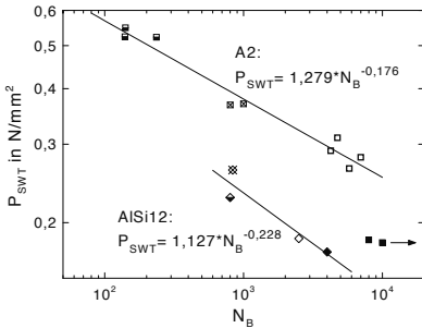
Abb. 8.36. P_{SWT} über N_B für TMF-Bearbeitung, T_{max} = 250^\circ C bis 400^\circ C
