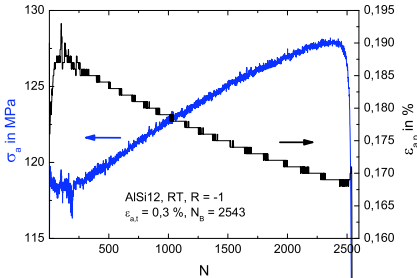
Abb. 10.1. AlSi12: Verlauf von \sigma_a und \epsilon_{a,p} unter Wechselbeanspruchung
