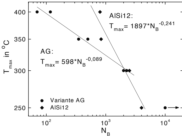
Abb. 8.64. Temperaturwöhlerkurven für TMF-Bbeanspruchung mit T_{min} = 50^\circ C und T_{max} = 250^\circ C bis 400^\circ C
