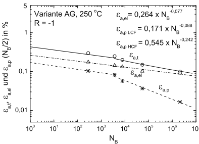
Abb. 7.31. Lebensdauerverhalten der MMC-Variante AG bei 250 °C nach Manson-Coffin und Basquin
