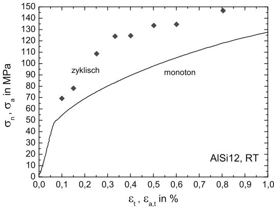
Abb. 7.7. AISi12: Monotones und zyklisches Spannungs-Dehnungs-Diagramm bei Raumtemperatur
