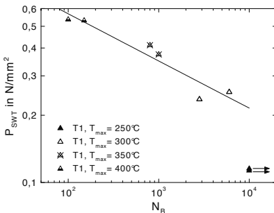
Abb. 8.82. Variante T1: P_{SWT} über N_B für TMF-Beanspruchung, T_{max} = 250\text{ °C} bis 400\text{ °C}
