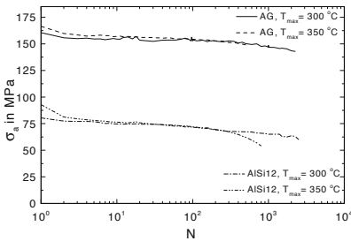
Abb. 8.57. Variante AG im Vergleich zu AlSi12: \sigma_a über N
