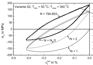
Abb. 10.21. Schädigungsentwicklung der MMC-Variante A2 unter TMF-Beanspruchung
