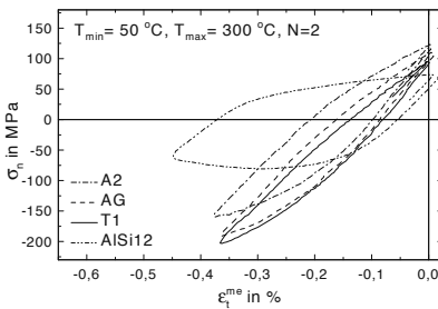
Abb. 8.101. \sigma_n - \epsilon_t^{\text{me}} -Hysteresen für TMF-Beanspruchung mit T_{\min} = 50\text{ °C} und T_{\max} = 300\text{ °C} , N = 2
