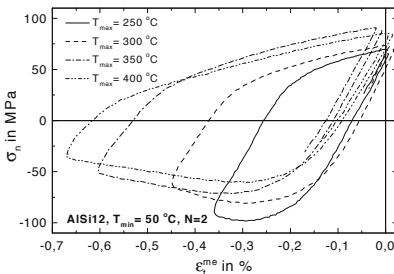
Abb. 8.2. AlSi12: \sigma_n - \epsilon_t^{\text{mc}} -Hysterese für TMF-Beanspruchung mit T_{\max} = 250^\circ\text{C} bis 400^\circ\text{C} , N = 2
