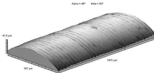
Abb. 3.10. Oberflächenkontur T 1 -Rundprobe
