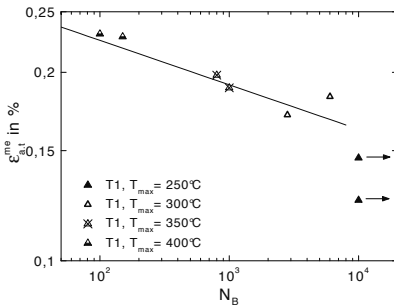
Abb. 8.80. Variante T1: \epsilon_{a,t}^{me} über N_B für TMF-Beanspruchung mit T_{max} = 250\text{ °C} bis 400\text{ °C}
