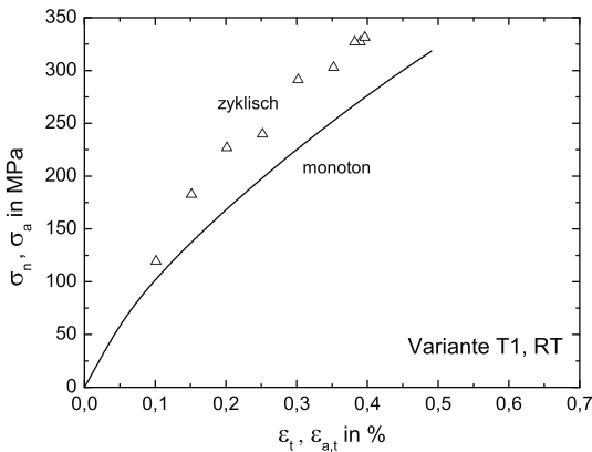
Abb. 7.38. Variante T1: Monotones und zyklisches Spannungs-Dehnungs-Diagramm bei RT
