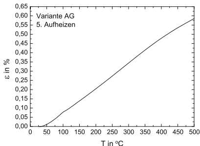
Abb. 5.3. Temperaturabhängiges Ausdehnungsverhalten der MMC-Variante AG bis 500 ^{\circ}\text{C}
