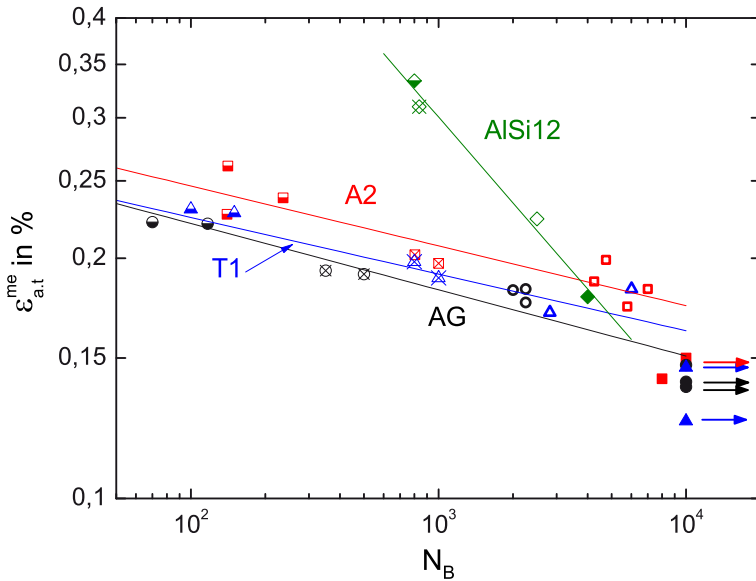
Abb. 8.120. MMCs und AISi12: \epsilon_{a,t}^{me} über N_B für TMF-Beanspruchung mit T_{min} = 50^\circ\text{C} bei totaler Dehnungsbehinderung
