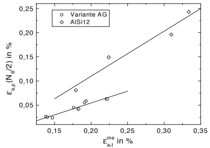
Abb. 8.61. Variante AG und AISi12: \epsilon_{a,p} über \epsilon_{a,t}^{me} für TMF-Bbeanspruchung mit T_{min} = 50^\circ C
