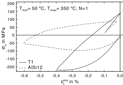
Abb. 8.86. Variante T1 und AlSi12: Hystereseschleifen für TMF-Bearbeitung mit T_{max} = 350^\circ\text{C} bei N = 1
