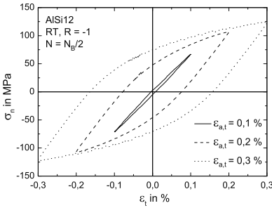
Abb. 7.3. \sigma_n - \epsilon_i -Hysteresen des Matrixwerkstoffs AISi12 bei RT für N = N_B/2
