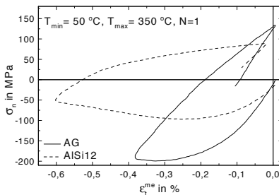
Abb. 8.55. Variante AG und AlSi12: Hystereseschleifen für TMF-Beanspruchung mit T_{max} = 350 °C bei N = 1
