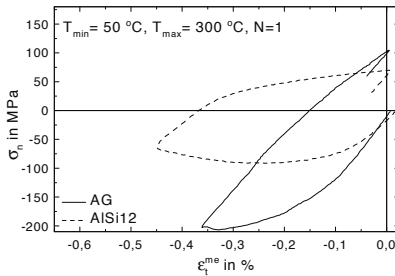
Abb. 8.53. Variante AG und AlSi12: Hystereseschleifen für TMF-Beanspruchung mit T_{max} = 300 °C, N = 1
