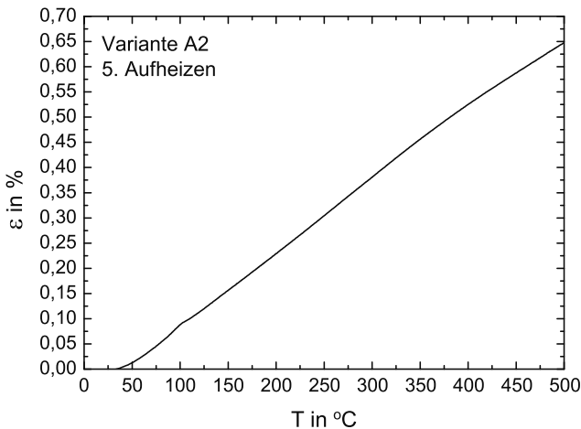
Abb. 5.2. Temperaturabhängiges Ausdehnungsverhalten der MMC-Variante A2 bis 500 °C
