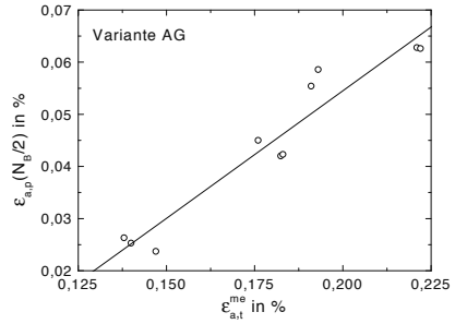
Abb. 8.45. Variante AG: \epsilon_{a,p} über \epsilon_{a,t}^{me} , TMF-Beanspruchung mit T_{\min} = 50^\circ\text{C}
