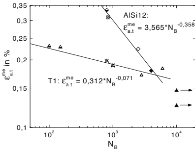
Abb. 8.96. \epsilon_{a,t}^{me} über N_B für TMF-Beanspruchung, T_{max} = 250\text{ °C} bis 400\text{ °C}
