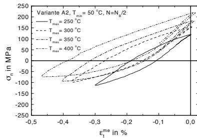
Abb. 8.9. Variante A2: \sigma_n - \epsilon_t^{\text{me}} -Hysteresen für TMF-Beanspruchung, T_{\max} = 250 \text{ °C} bis 400 \text{ °C} , N = N_B/2
