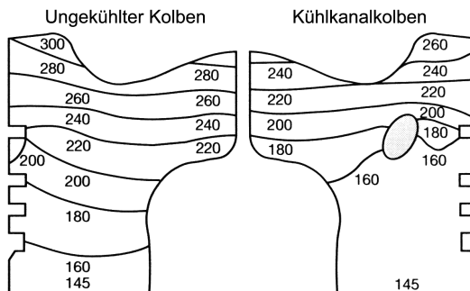
Abb. 2.1. Temperaturverteilung in einem Kolben (Angaben in °C) (Alc83)
