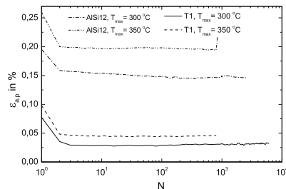
Abb. 8.89. Variante T1 im Vergleich zu AlSi12: \epsilon_{a,p} über N
