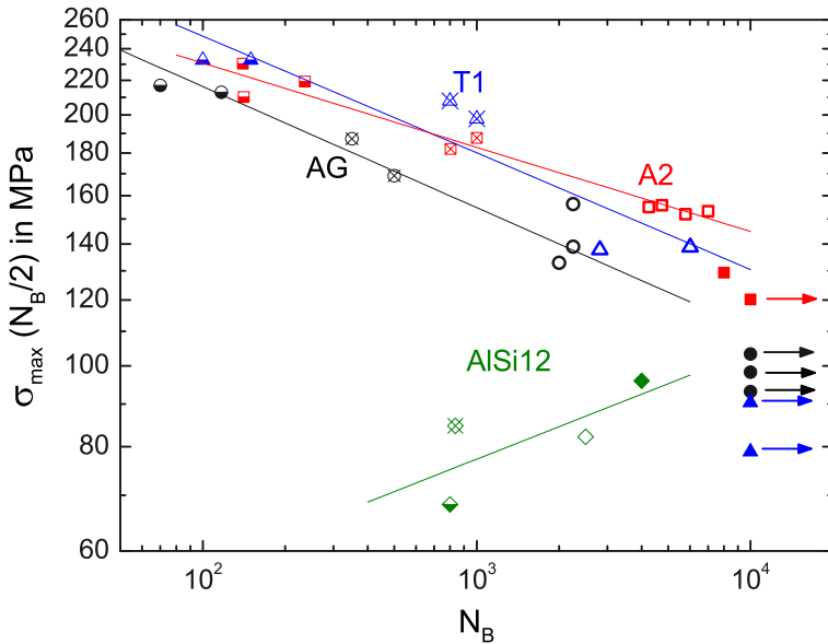
Abb. 8.119. MMCs und AlSi12: \sigma_{\max} über N_B für TMF-Belastung mit T_{\min} = 50^\circ\text{C} bei totaler Dehnungsbehinderung
