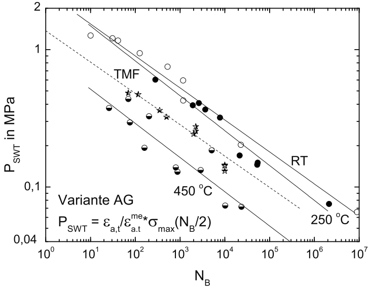
Abb. 9.6. Variante AG, Vergleich zwischen isothermer und TMF-Beanspruchung: P_{SWT} über N_B
