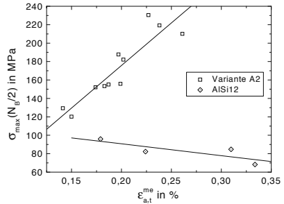
Abb. 8.32. Variante A2 und AlSi12: \sigma_{max} über \epsilon_{a,t}^{me} für TMF-Bbeanspruchung, T_{min} = 50^\circ C
