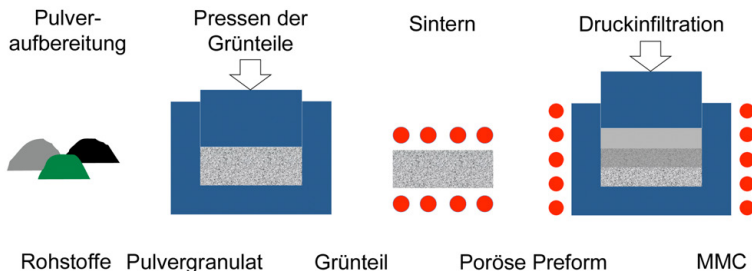
Abb. 3.1. Herstellung der untersuchten Preform-MMCs
