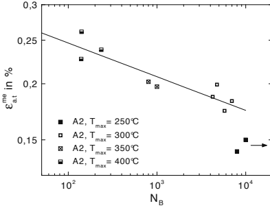
Abb. 8.18. Variante A2: \epsilon_{a,t}^{mc} über N_B für TMF-Beanspruchung mit T_{max} = 250\text{ °C} bis 400\text{ °C}
