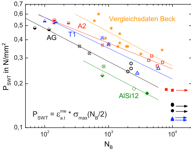
Abb. 8.122. MMCs, AlSi12 und faserverstärkte AlSi12CuMgNi nach Beck (Becoob): P_{SWT} über N_B für TMF-Belastung mit T_{min} = 50 °C bei totaler Dehnungsbehinderung
