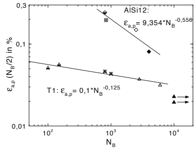
Abb. 8.97. Manson-Coffin-Darstellung für TMF-Beanspruchung, T_{max} = 250\text{ °C} bis 400\text{ °C}
