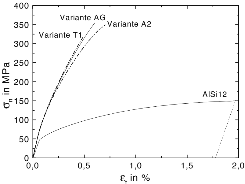
Abb. 6.3. MMCs und Matrixlegierung AlSi12: \sigma_n - \epsilon_t -Kurven für quasistatische Beanspruchung bei RT
