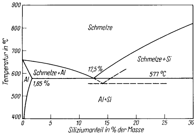
Abb. 2.2. System Aluminium-Silizium bis 30 % Si; gestrichelte Linien deuten die Unterkühlbarkeit der veredelten Legierung an (Huf88)
