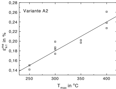
Abb. 8.13. Variante A2: \epsilon_{a,t}^{me} über T_{\max} für TMF-Beanspruchung mit T_{\min} = 50\text{ °C}
