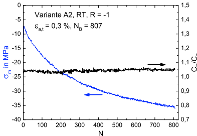
Abb. 10.7. Variante A2: Verlauf von \sigma_m und C_D/C_Z unter Wechselbeanspruchung
