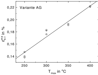
Abb. 8.44. Variante AG: \epsilon_{a,t}^{me} über T_{\max} , TMF-Beanspruchung mit T_{\min} = 50^\circ\text{C}
