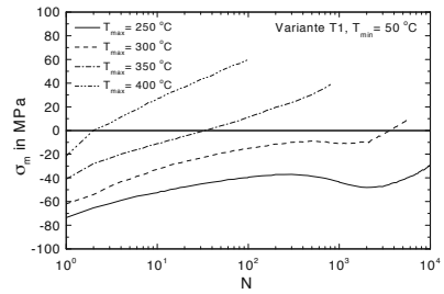
Abb. 8.73. Variante T1: \sigma_m über N für TMF-Beanspruchung mit T_{max} = 250^\circ\text{C} bis 400^\circ\text{C}
