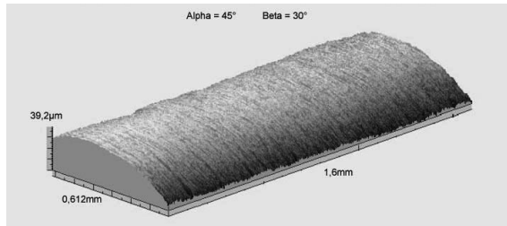
Abb. 3.12. Oberflächenkontur AG-Rundprobe
