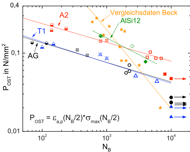
Abb. 8.123. MMCs, AlSi12 und faserverstärkte AlSi12CuMgNi nach Beck (Becoob): P_{OST} über N_B für TMF-Belastung mit T_{min} = 50 °C bei totaler Dehnungsbehinderung
