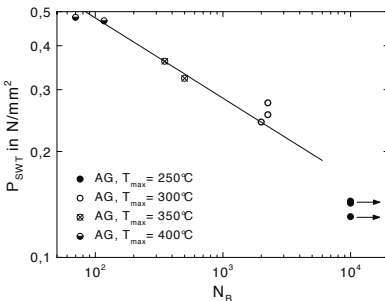
Abb. 8.51. Variante AG: P_{SWT} über N_B für TMF-Beanspruchung, T_{max} = 250\text{ }^\circ\text{C} bis 400\text{ }^\circ\text{C}
