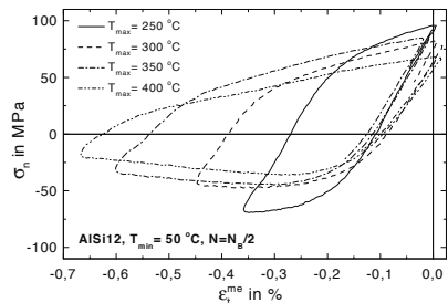
Abb. 8.3. AlSi12: \sigma_n - \epsilon_t^{\text{mc}} -Hysterese für TMF-Beanspruchung mit T_{\max} = 250^\circ\text{C} bis 400^\circ\text{C} , N = N_B/2
