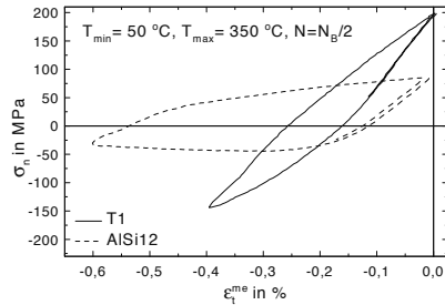
Abb. 8.87. Variante T1 und AlSi12: Hystereseschleifen für TMF-Bearbeitung mit T_{max} = 350^\circ\text{C} bei N = N_B/2
