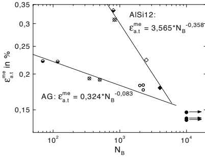
Abb. 8.65. \epsilon_{a,t}^{me} über N_B für TMF-Beanspruchung mit T_{\max} = 250 \text{ }^\circ\text{C} bis 400 \text{ }^\circ\text{C}
