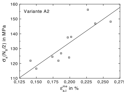
Abb. 8.15. Variante A2: \sigma_a über \epsilon_{a,t}^{me} für TMF-Beanspruchung mit T_{\min} = 50\text{ °C}
