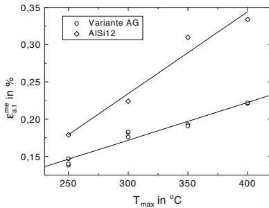
Abb. 8.60. Variante AG und AISi12: \epsilon_{a,t}^{me} über T_{max} für TMF-Bbeanspruchung, T_{min} = 50^\circ C
