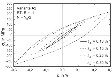
Abb. 7.10. \sigma_n - \epsilon_t -Hysteresen der Probenvariante A2 bei RT für N = N_B/2
