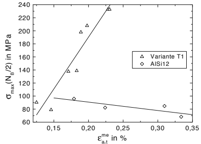
Abb. 8.94. Variante T1 und AlSi12: \sigma_{max} über \epsilon_{a,t}^{me} für TMF-Beanspruchung mit T_{min} = 50^\circ C
