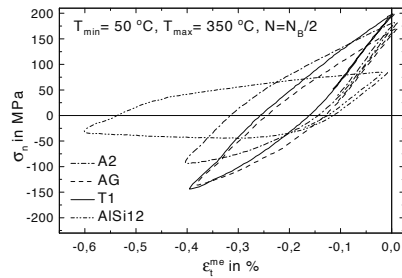
Abb. 8.109. \sigma_n - \epsilon_t^{me} -Hysteresen, TMF-Belastung mit T_{max} = 350 °C, N = N_B/2
