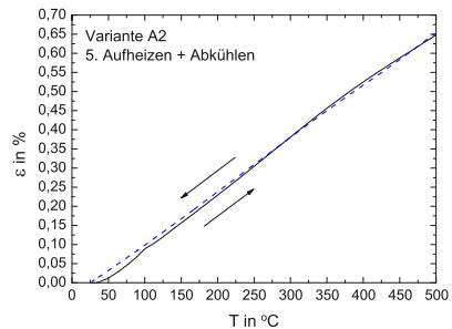
Abb. 5.10. MMC-Variante A2, Hysterese im 5. Temperaturzyklus
