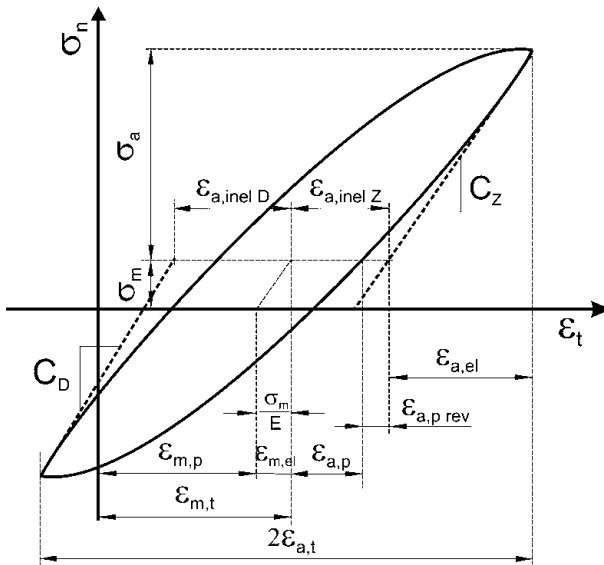
Abb. 2.7. Hystereseschleife bei elastisch-plastischer Wechselbeanspruchung
