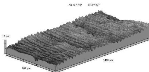
Abb. 3.11. Mikrogeometrie T 1 -Rundprobe mit herausgerechnetem Zylinderprofil
