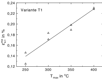
Abb. 8.75. Variante T1: \epsilon_{a,t}^{mc} über T_{max} für TMF-Bearspruchung mit T_{min} = 50\text{ °C}
