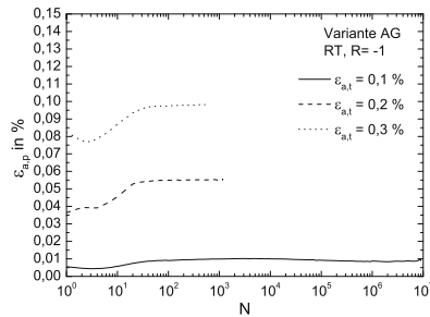
Abb. 7.21. Variante AG: Verlauf von \epsilon_{a,p} über N bei Raumtemperatur
