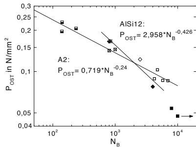
Abb. 8.37. P_{OST} über N_B für TMF-Bearbeitung, T_{max} = 250^\circ C bis 400^\circ C
