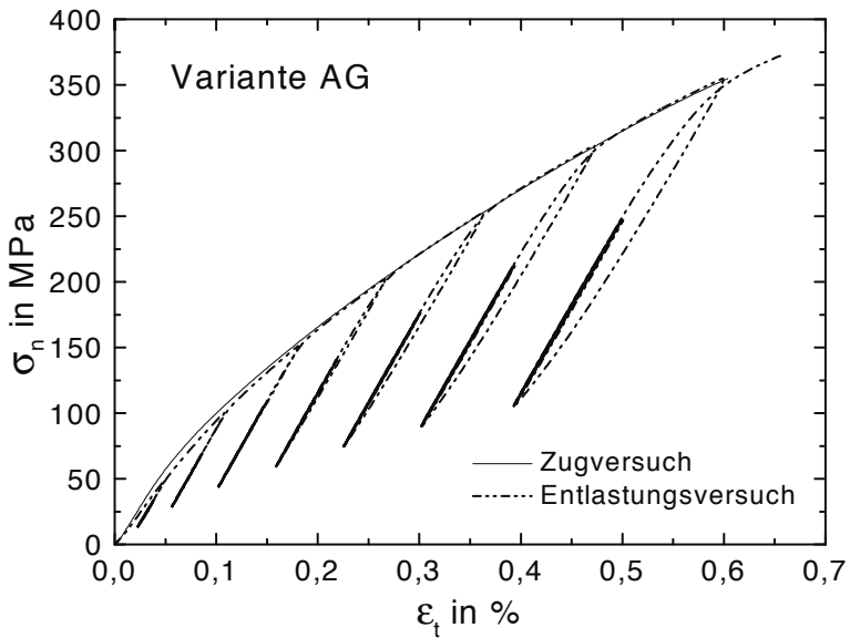
Abb. 6.8. Probenvariante AG: Entlastungsversuch und Zugversuch
