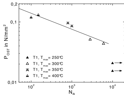
Abb. 8.83. Variante T1: P_{OST} über N_B für TMF-Beanspruchung, T_{max} = 250\text{ °C} bis 400\text{ °C}
