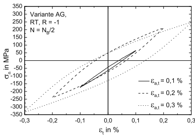
Abb. 7.17. \sigma_n - \epsilon_t -Hysteresen der Probenvariante AG bei RT für N = N_B/2
