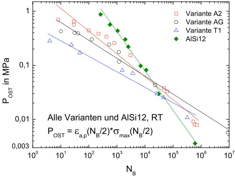
Abb. 7.49. P_{OST} über N_B für alle Varianten und AlSi12 bei Raumtemperatur, dehnungskontrolliert
