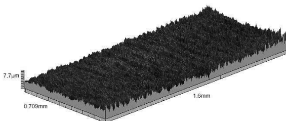
Abb. 3.9. Mikrogeometrie AlSi 12 -Rundprobe mit herausgerechnetem Zylinderprofil
