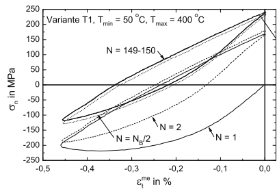
Abb. 10.22. Schädigungsentwicklung der MMC-Variante T1 unter TMF-Beanspruchung
