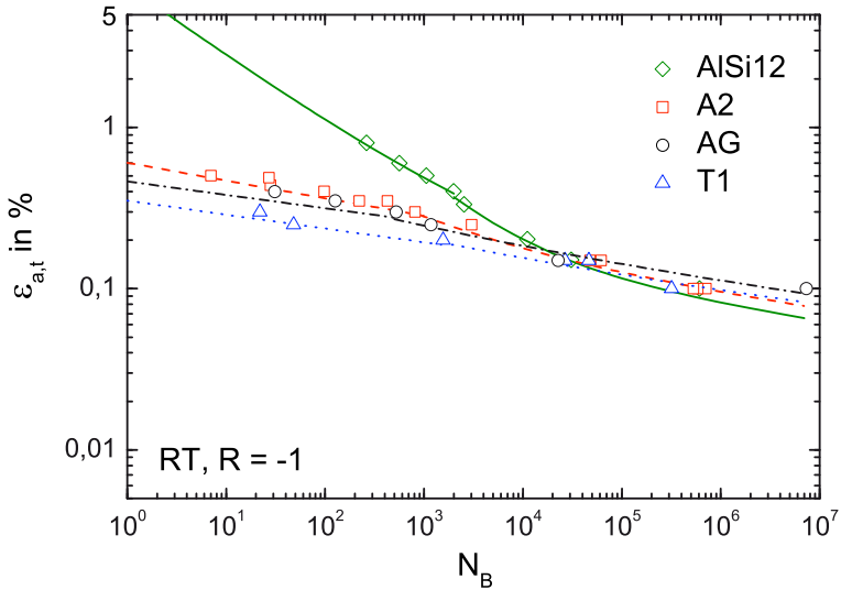
Abb. 7.42. Totaldehnungswöhlerkurven aller Varianten mit AlSi12 bei Raumtemperatur
