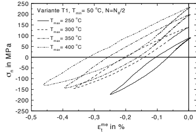
Abb. 8.71. Variante T1: \sigma_n - \epsilon_t^{me} -Hysteresen für TMF-Beanspruchung, T_{max} = 250^\circ\text{C} bis 400^\circ\text{C} , N = N_B/2
