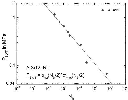
Abb. 7.9. P_{\text{SWT}} über N_B der unverstärkten Matrixlegierung AlSi12 bei Raumtemperatur, dehnungskontrolliert
