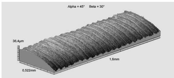
Abb. 3.14. Oberflächenkontur A2-Rundprobe
