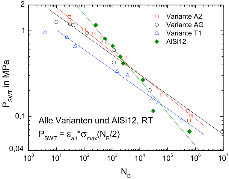
Abb. 7.48. P_{\text{SWT}} über N_B für alle Varianten und AlSi12 bei Raumtemperatur, dehnungskontrolliert
