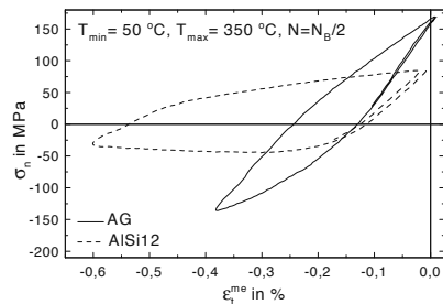
Abb. 8.56. Variante AG und AlSi12: Hystereseschleifen für TMF-Beanspruchung mit T_{max} = 350 °C bei N = N_B/2
