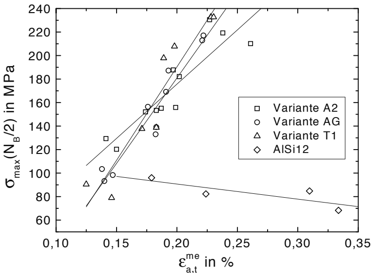
Abb. 8.117. MMCs und AlSi12: \sigma_{max} über \epsilon_{a,t}^{me} für TMF-Belastung mit T_{min} = 50^\circ\text{C}
