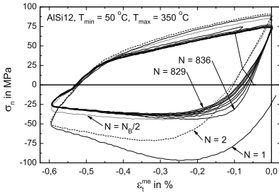
Abb. 10.17. Schädigungsentwicklung der Matrixlegierung AlSi12 unter TMF-Beanspruchung
