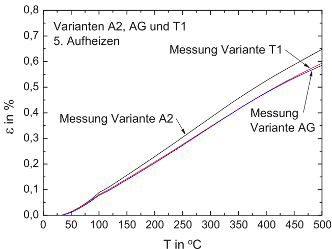
Abb. 5.5. Temperaturabhängiges Ausdehnungsverhalten aller MMC-Varianten bis 500 ^{\circ}\text{C}
