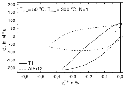
Abb. 8.84. Variante T1 und AlSi12: Hystereseschleifen für TMF-Beanspruchung mit T_{max} = 300 °C, N = 1
