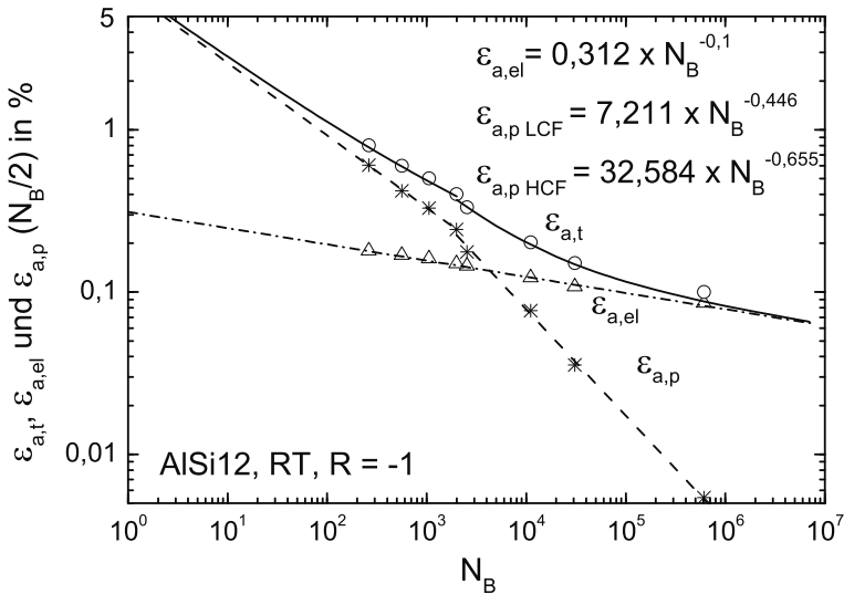
Abb. 7.8. Lebensdauerverhalten der unverstärkten Matrixlegierung AISi12 bei Raumtemperatur nach Manson-Coffin und Basquin
