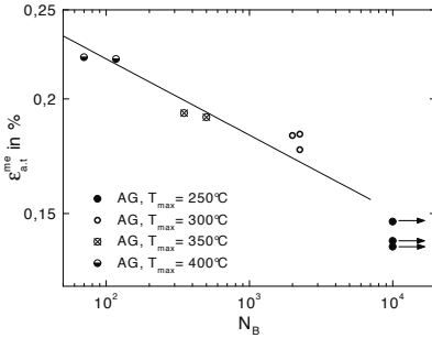
Abb. 8.49. Variante AG: \epsilon_{a,t}^{me} über N_B für TMF-Beanspruchung mit T_{max} = 250\text{ }^\circ\text{C} bis 400\text{ }^\circ\text{C}
