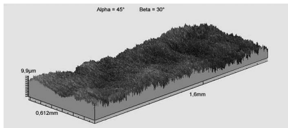
Abb. 3.13. Mikrogeometrie AG-Rundprobe mit herausgerechnetem Zylinderprofil
