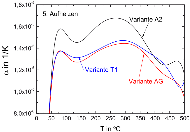
Abb. 5.7. Temperaturabhängige Ausdehnungskoeffizienten der drei MMC-Varianten bis 500 °C, 5. Aufheizen
