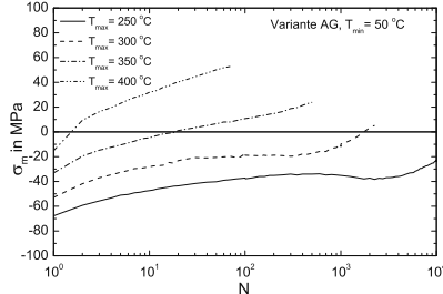
Abb. 8.42. Variante AG: \sigma_m über N für TMF-Beanspruchung mit T_{max} = 250 \text{ }^\circ\text{C} bis 400 \text{ }^\circ\text{C}
