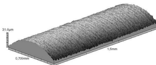
Abb. 3.8. Oberflächenkontur AlSi 12 -Rundprobe
