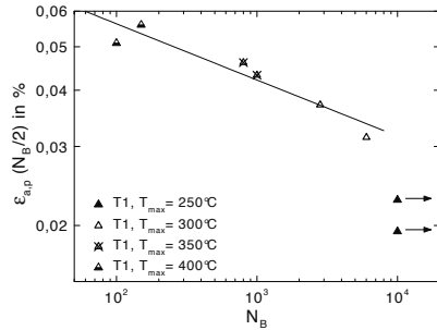
Abb. 8.81. Variante T1: Manson-Coffin-Darstellung für TMF-Beanspruchung mit T_{max} = 250\text{ °C} bis 400\text{ °C}
