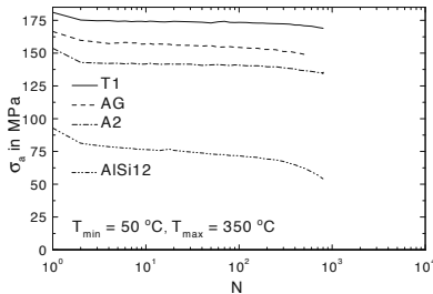
Abb. 8.110. Vergleich aller Varianten: \sigma_a über N für T_{max} = 350 °C
