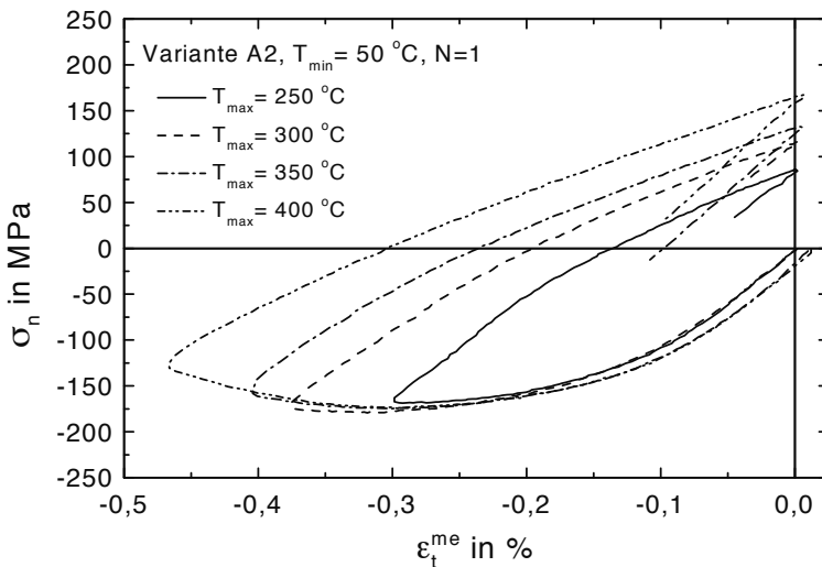
Abb. 8.7. Probenvariante A2: \sigma_n - \epsilon_t^{mc} -Hysteresen für TMF-Beanspruchung mit T_{\max} = 250 \text{ °C} bis 400 \text{ °C} , N = 1
