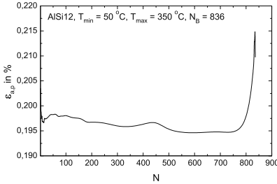
Abb. 10.19. \epsilon_{a,p} über N für die Matrixlegierung AlSi12 unter TMF-Beanspruchung
