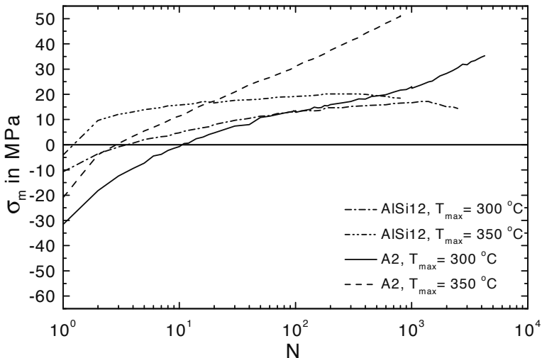
Abb. 8.28. Variante A2 im Vergleich zu AlSi12: \sigma_m über N
