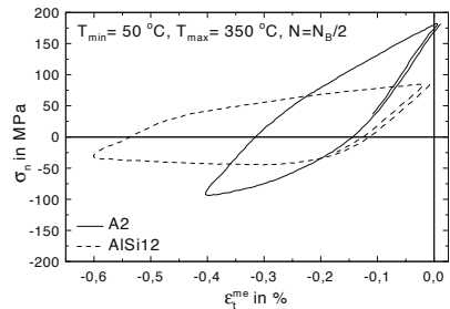
Abb. 8.25. Variante A2 und AlSi12: Hystereseschleifen für TMF-Beanspruchung mit T_{\max} = 350\text{ °C} bei N = N_B/2
