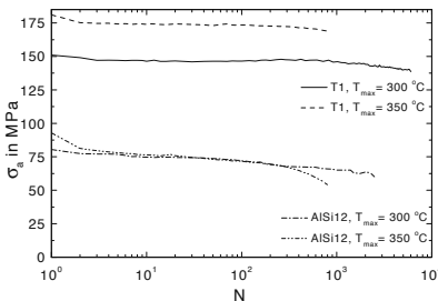
Abb. 8.88. Variante T1 im Vergleich zu AlSi12: \sigma_a über N
