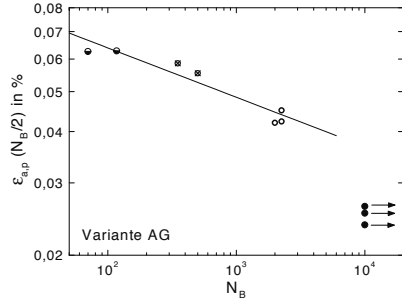
Abb. 8.50. Variante AG: Manson-Coffin-Darstellung für TMF-Beanspruchung mit T_{max} = 250\text{ }^\circ\text{C} bis 400\text{ }^\circ\text{C}
