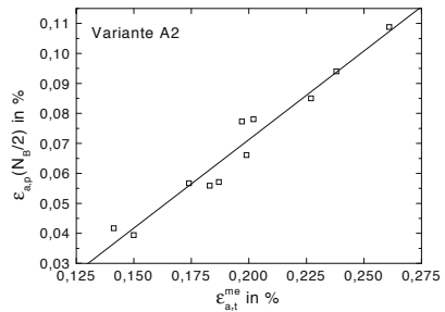
Abb. 8.14. Variante A2: \epsilon_{a,p} über \epsilon_{a,t}^{me} für TMF-Beanspruchung, T_{\min} = 50\text{ °C}
