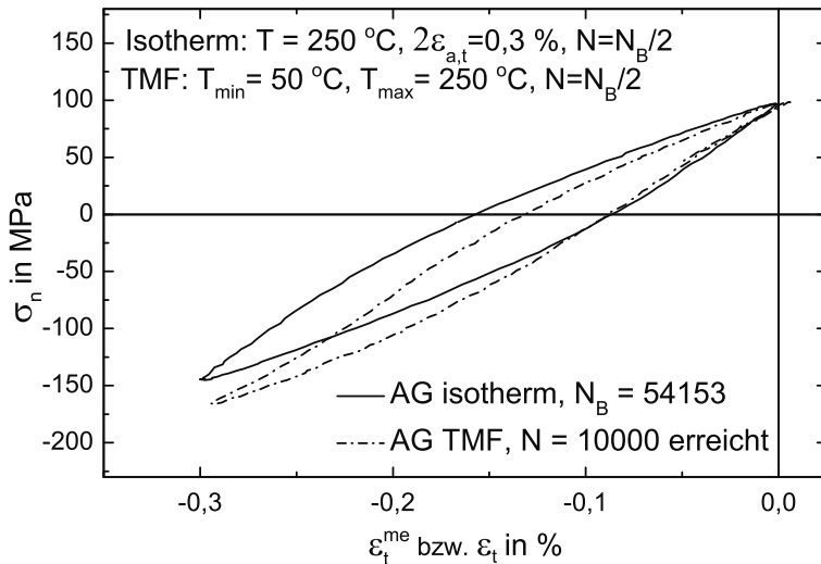
Abb. 9.1. \sigma_n - \epsilon_t -Hysterese und \sigma_n - \epsilon_t^{me} -Hysterese für isotherme und TMF-Bearbeitung mit T_{max} = 250\text{ °C} , N = N_B/2
