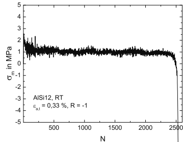
Abb. 10.2. AlSi12: Verlauf von \sigma_m über N unter Wechselbeanspruchung
