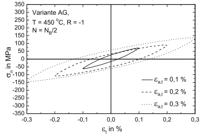
Abb. 7.23. \sigma_n - \epsilon_t -Hysteresen der Probenvariante AG bei 450 °C, N = N_B/2
