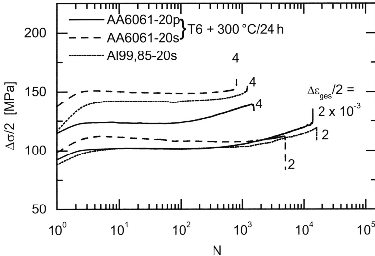
Abb. 7.41. Wechselerformungskurven von partikel- und kurzfaserverstärkten MMCs mit AA6061-Matrix bei unterschiedlichen Dehnungsamplituden (Raumtemperatur, Lastverhältnis R = -1 ) (Haro2b; Haro3)
