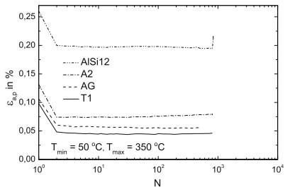
Abb. 8.111. Vergleich aller Varianten: \epsilon_{a,p} über N für T_{max} = 350 °C
