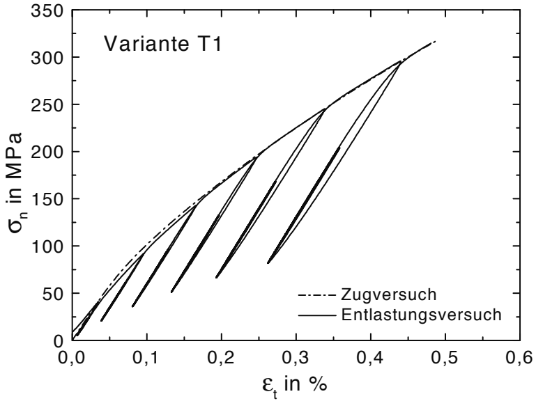
Abb. 6.9. Probenvariante T1: Entlastungsversuch und Zugversuch
