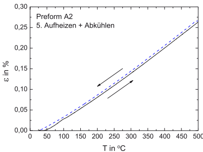
Abb. 5.9. Preform A2, Hysterese im 5. Temperaturzyklus
