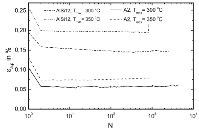
Abb. 8.27. Variante A2 im Vergleich zu AlSi12: \epsilon_{a,p} über N
