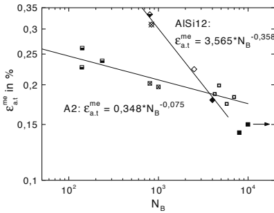
Abb. 8.34. \epsilon_{a,t}^{me} über N_B für TMF-Bearbeitung, T_{max} = 250^\circ C bis 400^\circ C
