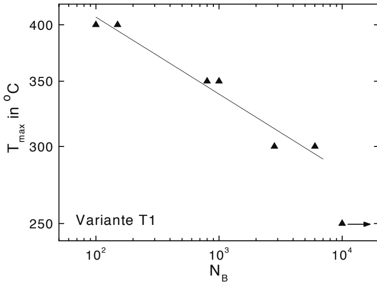
Abb. 8.79. Probenvariante T1: Temperaturwöhlerkurve für TMF-Beanspruchung mit T_{min} = 50^\circ C und T_{max} = 250^\circ C bis 400^\circ C
