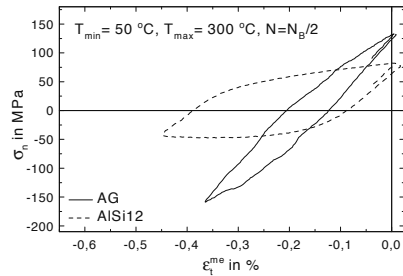
Abb. 8.54. Variante AG und AlSi12: Hystereseschleifen für TMF-Beanspruchung mit T_{max} = 300 °C, N = N_B/2
