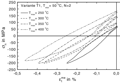
Abb. 8.70. Variante T1: \sigma_n - \epsilon_t^{me} -Hysteresen für TMF-Beanspruchung, T_{max} = 250^\circ\text{C} bis 400^\circ\text{C} , N = 2
