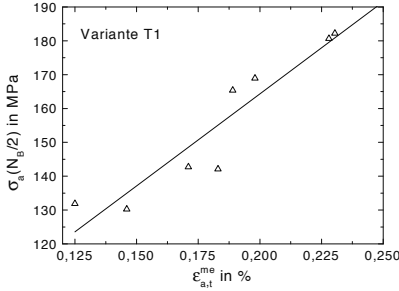
Abb. 8.77. Variante T1: \sigma_a über \epsilon_{a,t}^{me} für TMF-Beanspruchung mit T_{min} = 50^\circ C
