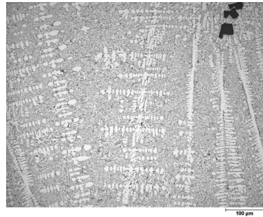
Abb. 2.4. Gefüge einer eutektischen Al-Si-Legierung, Druckguss
