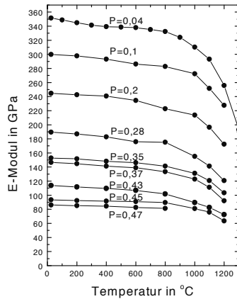
Abb. 5.12. E-Modul in Abhängigkeit von Porosität und Temperatur am Beispiel Al 2 O 3 (Cob56)
