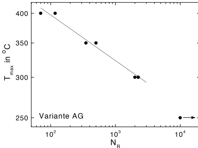
Abb. 8.48. Probenvariante AG: Temperaturwöhlerkurve für TMF-Beanspruchung mit T_{\min} = 50^\circ\text{C} und T_{\max} = 250^\circ\text{C} bis 400^\circ\text{C}
