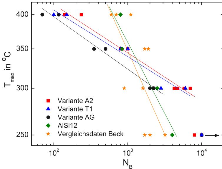
Abb. 8.118. MMCs, AlSi 12 und faserverstärkte AlSi 12 CuMgNi nach Beck (Becoob): Temperaturwöhlerkurven für TMF-Beanspruchung mit T_{\min} = 50^{\circ}\text{C} bei totaler Dehnungsbehinderung
