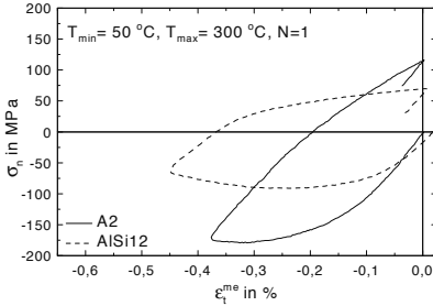
Abb. 8.22. Variante A2 und AlSi12: Hystereseschleifen für TMF-Beanspruchung mit T_{\max} = 300\text{ °C} , N = 1
