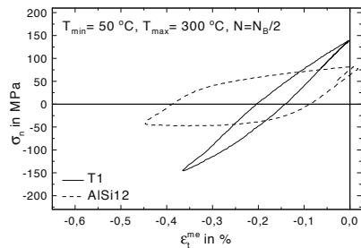
Abb. 8.85. Variante T1 und AlSi12: Hystereseschleifen für TMF-Beanspruchung mit T_{max} = 300 °C, N = N_B/2
