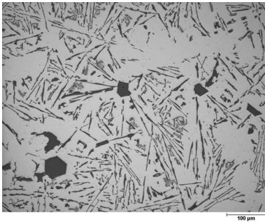
Abb. 2.3. Gefüge einer eutektischen Al-Si-Legierung, Kokillenguss
