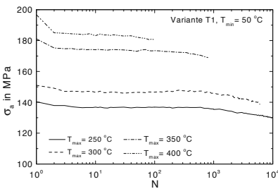
Abb. 8.72. Variante T1: \sigma_a über N für TMF-Beanspruchung mit T_{max} = 250^\circ\text{C} bis 400^\circ\text{C}
