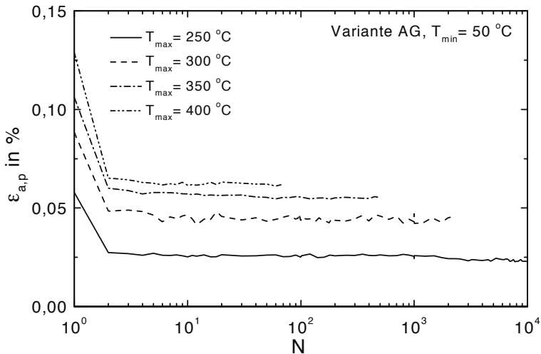
Abb. 8.43. Variante AG: \epsilon_{a,p} über N für TMF-Beanspruchung, T_{\max} = 250\text{ °C} bis 400\text{ °C}
