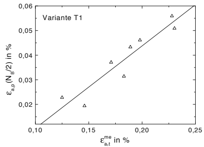
Abb. 8.76. Variante T1: \epsilon_{a,p} über \epsilon_{a,t}^{mc} für TMF-Bearspruchung mit T_{min} = 50\text{ °C}
