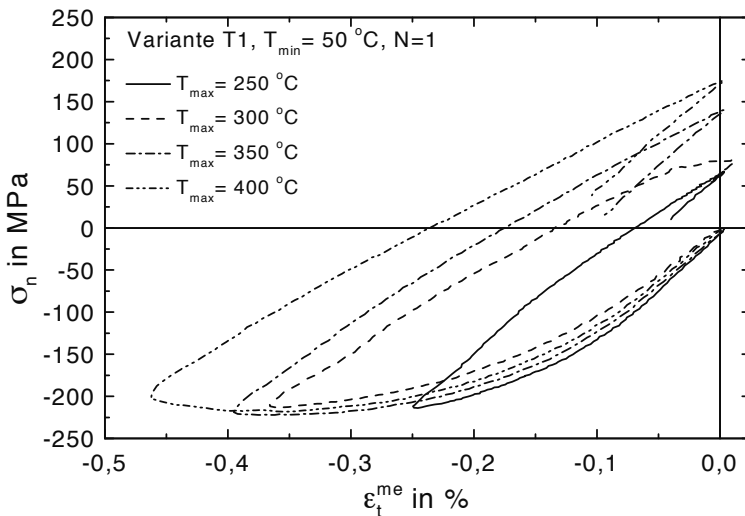
Abb. 8.69. Probenvariante T1: \sigma_n - \epsilon_t^{\text{me}} -Hysteresen für TMF-Beanspruchung mit T_{\text{max}} = 250 \text{ }^\circ\text{C} bis 400 \text{ }^\circ\text{C} , N = 1
