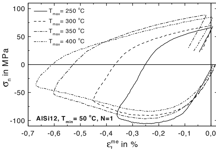
Abb. 8.1. Matrixwerkstoff AlSi12: \sigma_n - \epsilon_t^{me} -Hysteresen für TMF-Beanspruchung mit T_{max} = 250 \text{ °C} bis 400 \text{ °C} , N = 1
