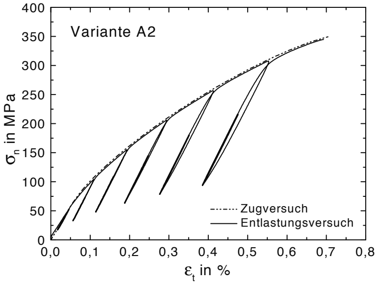
Abb. 6.7. Probenvariante A2: Entlastungsversuch und Zugversuch
