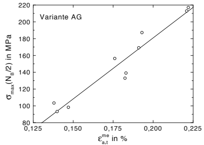
Abb. 8.47. Variante AG: \sigma_{\max} über \epsilon_{a,t}^{me} , TMF-Beanspruchung mit T_{\min} = 50^\circ\text{C}
