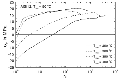
Abb. 8.5. AlSi12: \sigma_m über N für TMF-Beanspruchung mit T_{max} = 250\text{ °C} bis 400\text{ °C}
