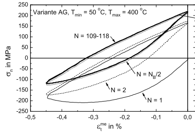
Abb. 10.18. Schädigungsentwicklung der MMC-Variante AG unter TMF-Beanspruchung
