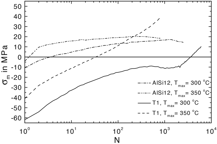
Abb. 8.90. Probenvariante T1 im Vergleich zu AISi12: \sigma_m über N
