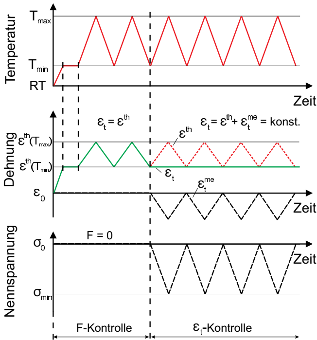
Abb. 4.2. Versuchsführung der TMF Out-of-Phase-Versuche
