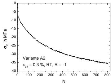
Abb. 10.4. Variante A2: Verlauf von \sigma_m über N unter Wechselbeanspruchung
