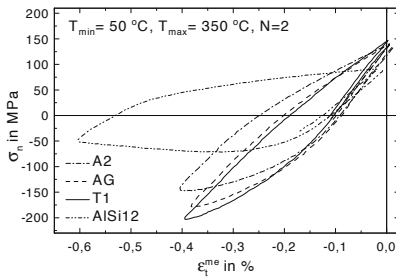
Abb. 8.108. \sigma_n - \epsilon_t^{me} -Hysteresen, TMF-Belastung mit T_{max} = 350 °C, N = 2
