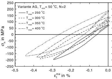
Abb. 8.39. Variante AG: \sigma_n - \epsilon_t^{me} -Hysteresen für TMF-Beanspruchung, T_{max} = 250 \text{ }^\circ\text{C} bis 400 \text{ }^\circ\text{C} , N = 2
