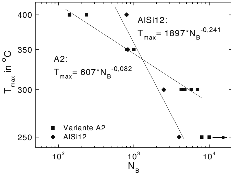
Abb. 8.33. Temperaturwöhlerkurven für TMF-Bbeanspruchung, T_{min} = 50^\circ C und T_{max} = 250^\circ C bis 400^\circ C
