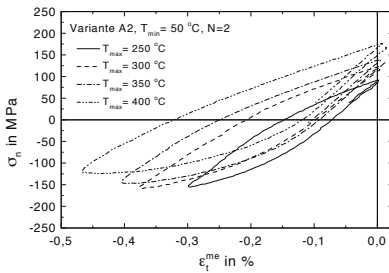
Abb. 8.8. Variante A2: \sigma_n - \epsilon_t^{\text{me}} -Hysteresen für TMF-Beanspruchung, T_{\max} = 250 \text{ °C} bis 400 \text{ °C} , N = 2
