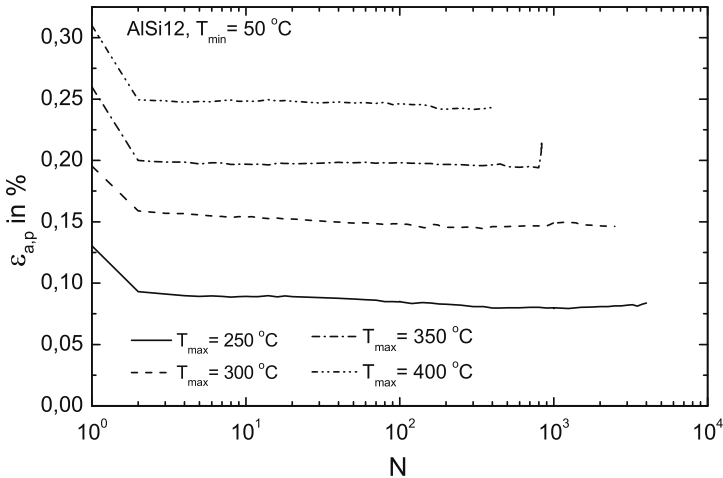
Abb. 8.6. AlSi12: \epsilon_{a,p} über N für TMF-Beanspruchung, T_{max} = 250\text{ °C} bis 400\text{ °C}
