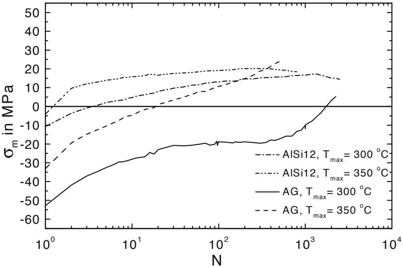
Abb. 8.59. Probenvariante AG im Vergleich zu AISi12: \sigma_m über N
