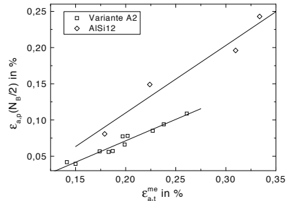
Abb. 8.30. Variante A2 und AlSi12: \epsilon_{a,p} über \epsilon_{a,t}^{me} für TMF-Beanspruchung, T_{\min} = 50\text{ °C}
