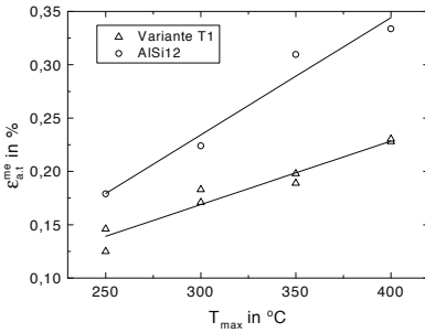
Abb. 8.91. Variante T1 und AISi12: \epsilon_{a,t}^{me} über T_{max} für TMF-Belastung, T_{min} = 50^\circ\text{C}
