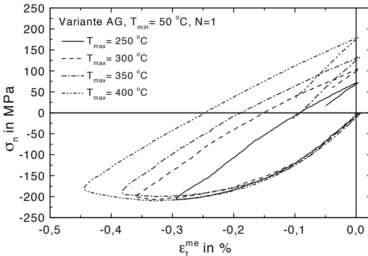
Abb. 8.38. Probenvariante AG: \sigma_n - \epsilon_t^{me} -Hysteresen für TMF-Beanspruchung mit T_{max} = 250 °C bis 400 °C, N = 1
