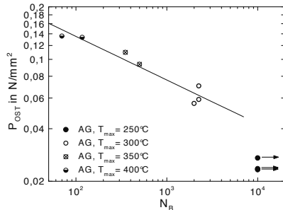
Abb. 8.52. Variante AG: P_{OST} über N_B für TMF-Beanspruchung mit T_{max} = 250\text{ }^\circ\text{C} bis 400\text{ }^\circ\text{C}
