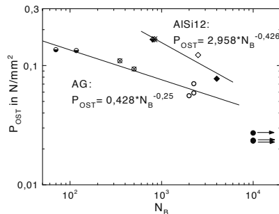
Abb. 8.68. P_{OST} über N_B für TMF-Beanspruchung, T_{\max} = 250 \text{ }^\circ\text{C} bis 400 \text{ }^\circ\text{C}
