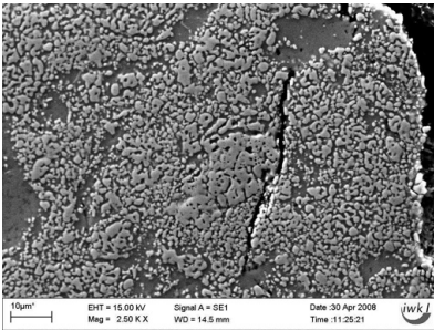
Abb. 10.13. Sekundärrisse an einer MMC-Probe der Variante AG
