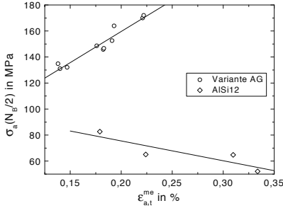
Abb. 8.62. Variante AG und AlSi12: \sigma_a über \epsilon_{a,t}^{me} für TMF-Bbeanspruchung mit T_{min} = 50^\circ C
