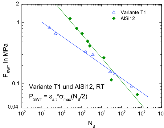
Abb. 7.40. P_{SWT} über N_B von AlSi12 und der Variante T1 bei Raumtemperatur, dehnungskontrolliert
