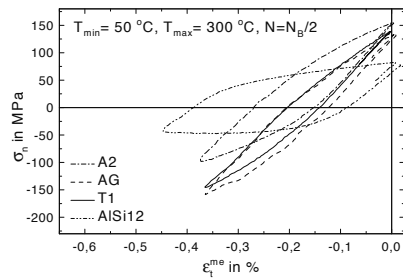
Abb. 8.102. \sigma_n - \epsilon_t^{\text{me}} -Hysteresen für TMF-Beanspruchung mit T_{\min} = 50\text{ °C} und T_{\max} = 300\text{ °C} , N = N_B/2
