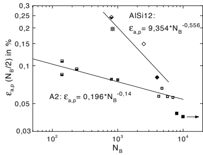
Abb. 8.35. Manson-Coffin-Darstellung für TMF-Bearbeitung, T_{max} = 250^\circ C bis 400^\circ C
