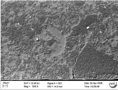
Abb. 10.11. Oberflächennaher Riss einer MMC-Probe der Variante A2
