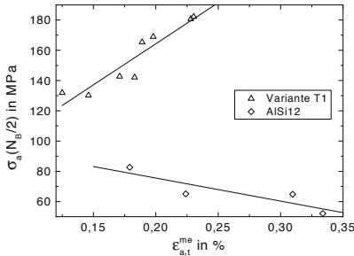
Abb. 8.93. Variante T1 und AlSi12: \sigma_a über \epsilon_{a,t}^{me} für TMF-Beanspruchung mit T_{min} = 50^\circ C
