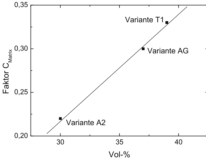
Abb. 5.14. Faktor C_{Matrix} in Abhängigkeit des Keramikanteils
