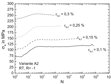
Abb. 7.12. Variante A2: Verlauf von \sigma_a über N bei Raumtemperatur
