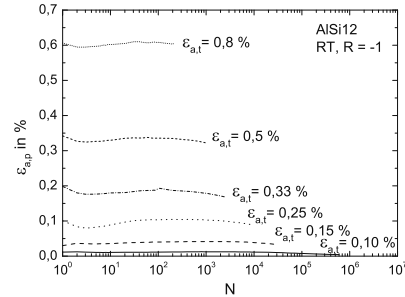
Abb. 7.6. Matrixwerkstoffs AISi12: Verlauf von \epsilon_{a,p} über N bei RT
