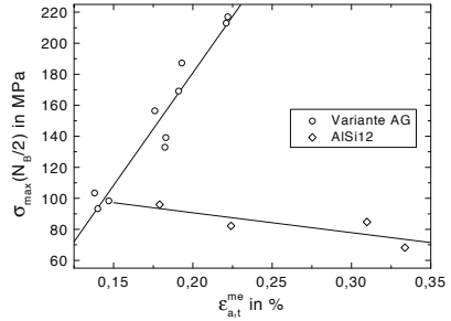
Abb. 8.63. Variante AG und AlSi12: \sigma_{max} über \epsilon_{a,t}^{me} für TMF-Bbeanspruchung mit T_{min} = 50^\circ C
