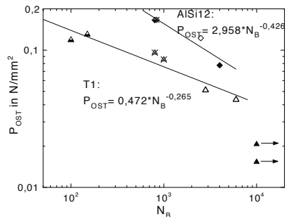
Abb. 8.99. P_{OST} über N_B für TMF-Beanspruchung, T_{max} = 250 °C bis 400 °C
