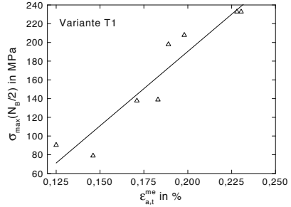
Abb. 8.78. Variante T1: \sigma_{max} über \epsilon_{a,t}^{me} , TMF-Beanspruchung mit T_{min} = 50^\circ C
