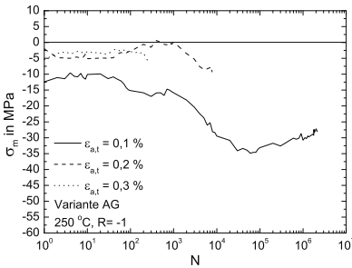
Abb. 7.24. Mittelspannungsverläufe bei 250 °C für \epsilon_{a,t} von 0,1 % bis 0,3 %
