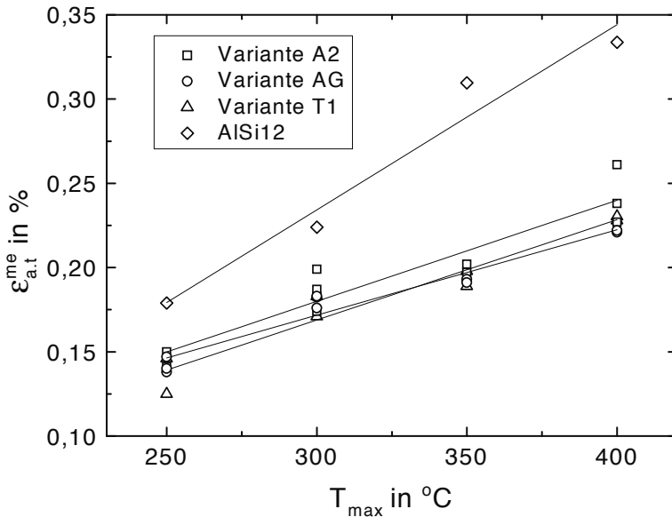
Abb. 8.114. MMCs und AlSi12: \epsilon_{a,t}^{me} über T_{max} für TMF-Belastung mit T_{min} = 50^\circ\text{C}
