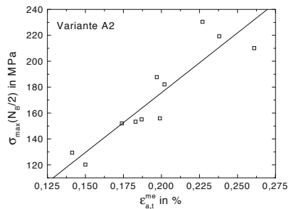
Abb. 8.16. Variante A2: \sigma_{\max} über \epsilon_{a,t}^{me} für TMF-Beanspruchung, T_{\min} = 50\text{ °C}
