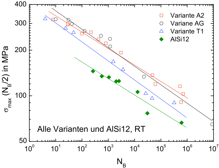
Abb. 7.43. Maximalspannungen aller Varianten und AISi12 bei Raumtemperatur
