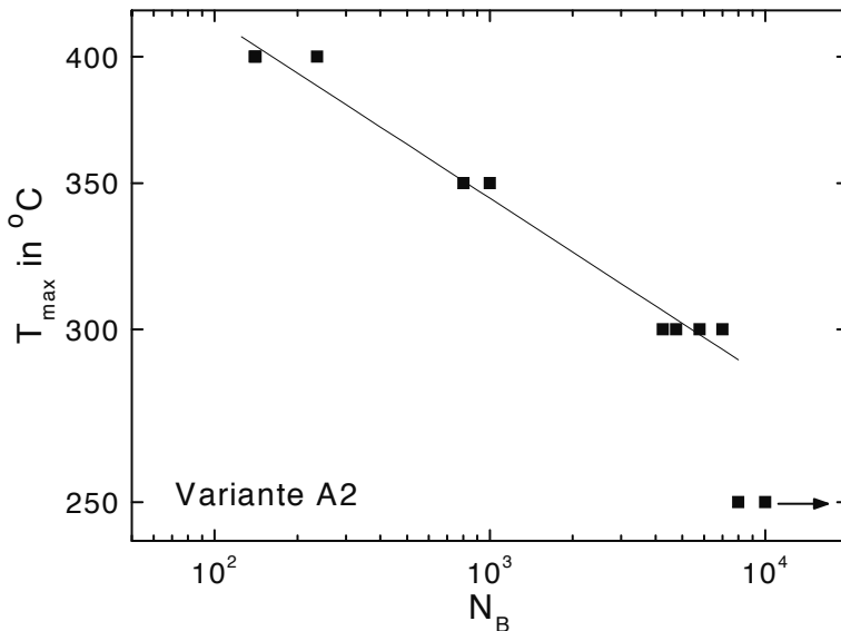
Abb. 8.17. Variante A2: Temperaturwöhlerkurve für TMF-Beanspruchung mit T_{\min} = 50^\circ\text{C} und T_{\max} = 250^\circ\text{C} bis 400^\circ\text{C}
