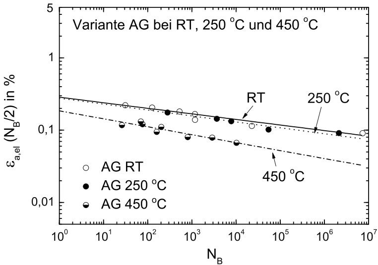
Abb. 7.47. Vergleich der Variante AG in der Basquin-Darstellung \epsilon_{a,el} über N_B bei RT, 250 °C und 450 °C
