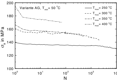
Abb. 8.41. Variante AG: \sigma_a über N für TMF-Beanspruchung mit T_{max} = 250 \text{ }^\circ\text{C} bis 400 \text{ }^\circ\text{C}
