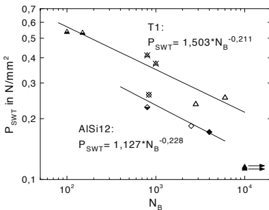
Abb. 8.98. P_{SWT} über N_B für TMF-Beanspruchung mit T_{max} = 250 °C bis 400 °C
