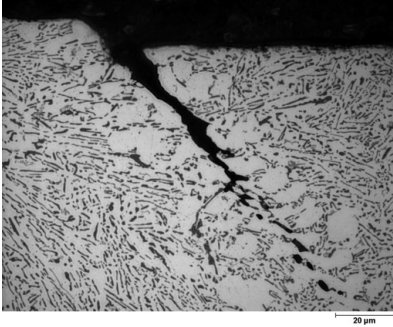
Abb. 10.9. Oberflächennaher Mikroriss einer AlSi 12 -Probe
