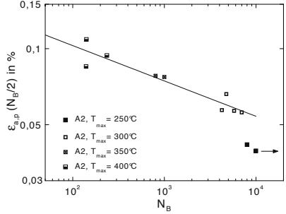
Abb. 8.19. Variante A2: Manson-Coffin-Darstellung für TMF-Beanspruchung mit T_{max} = 250\text{ °C} bis 400\text{ °C}
