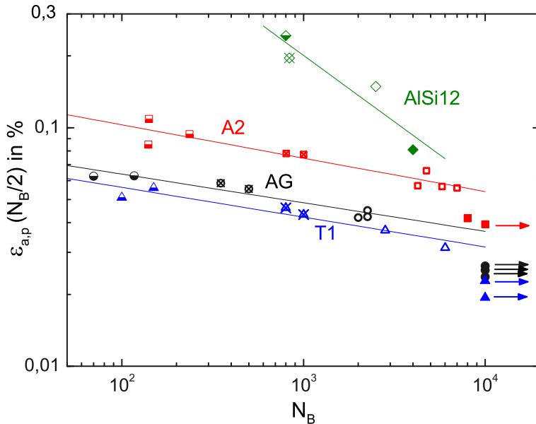
Abb. 8.121. MMCs und AlSi12: \epsilon_{a,p} über N_B für TMF-Belastung mit T_{\min} = 50\text{ °C} bei totaler Dehnungsbehinderung
