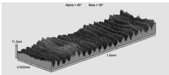
Abb. 3.15. Mikrogeometrie A2-Rundprobe mit herausgerechnetem Zylinderprofil
