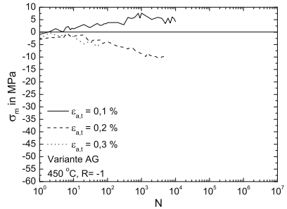
Abb. 7.25. Mittelspannungsverläufe bei 450 °C für \epsilon_{a,t} von 0,1 % bis 0,3 %
