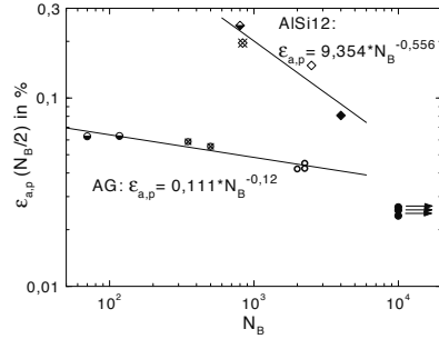
Abb. 8.66. Manson-Coffin-Darstellung für TMF-Beanspruchung, T_{\max} = 250 \text{ }^\circ\text{C} bis 400 \text{ }^\circ\text{C}
