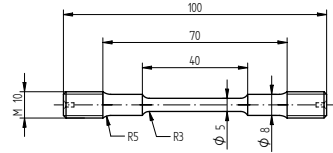
Abb. 3.6. Probegeometrie für Zugversuche an der Matrixlegierung AlSi12
