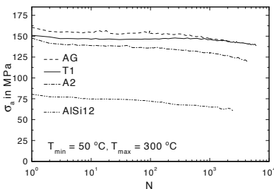
Abb. 8.103. Vergleich aller Varianten: \sigma_a über N für T_{\max} = 300\text{ °C}
