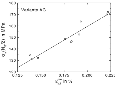
Abb. 8.46. Variante AG: \sigma_a über \epsilon_{a,t}^{me} für TMF-Beanspruchung mit T_{\min} = 50^\circ\text{C}
