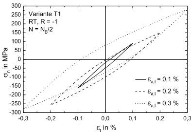
Abb. 7.34. \sigma_n - \epsilon_t -Hysteresen der Probenvariante T1 bei RT für N = N_B/2
