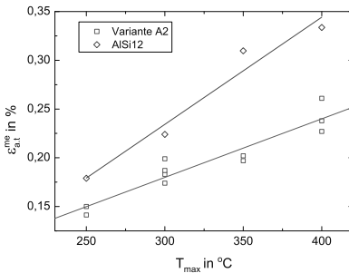
Abb. 8.29. Variante A2 und AlSi12: \epsilon_{a,t}^{me} über T_{\max} für TMF-Beanspruchung, T_{\min} = 50\text{ °C}
