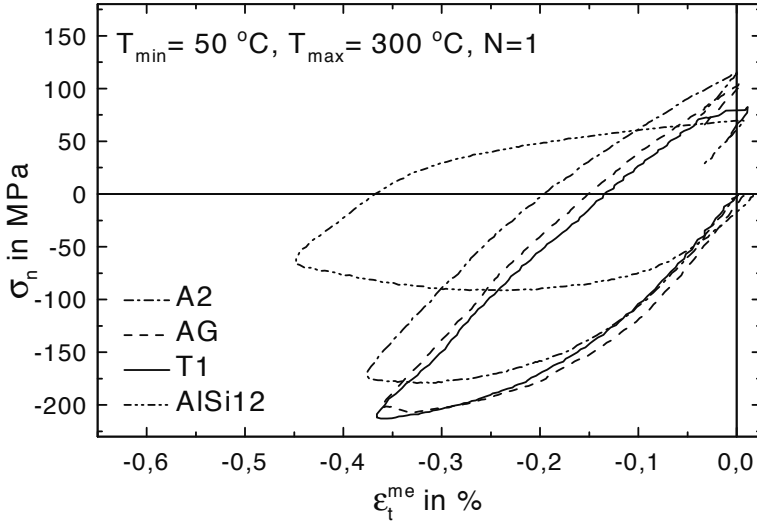
Abb. 8.100. \sigma_n - \epsilon_t^{\text{me}} -Hysteresen für TMF-Beanspruchung mit T_{\min} = 50\text{ °C} und T_{\max} = 300\text{ °C} , N = 1
