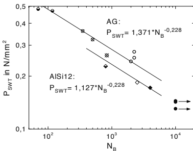
Abb. 8.67. P_{SWT} über N_B für TMF-Beanspruchung mit T_{\max} = 250 \text{ }^\circ\text{C} bis 400 \text{ }^\circ\text{C}
