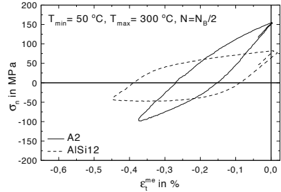
Abb. 8.23. Variante A2 und AlSi12: Hystereseschleifen für TMF-Beanspruchung mit T_{\max} = 300\text{ °C} , N = N_B/2
