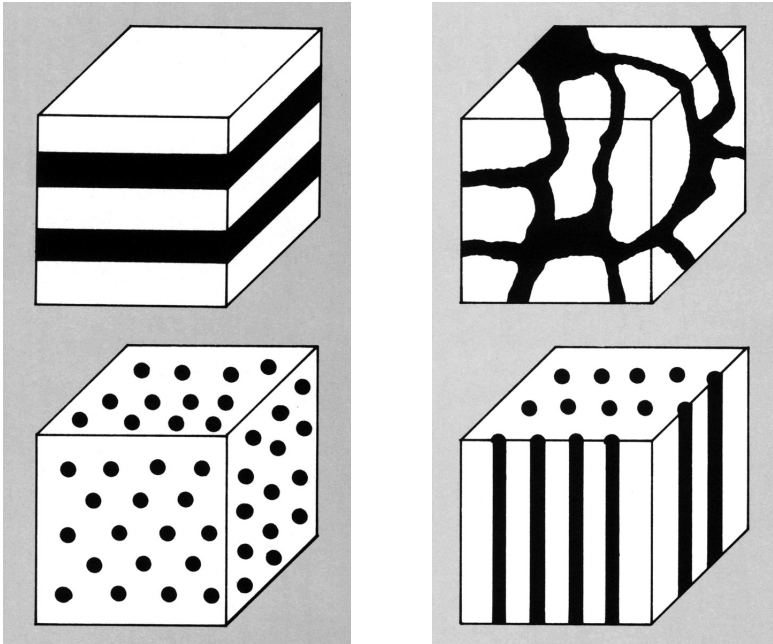
Abb. 2.9. Schicht- und Teilchenverbundwerkstoff (Rau77)
