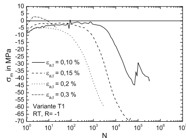
Abb. 7.35. Mittelspannungsverläufe der Probenvariante T1 bei RT, \epsilon_{a,t} von 0,1 % bis 0,3 %
