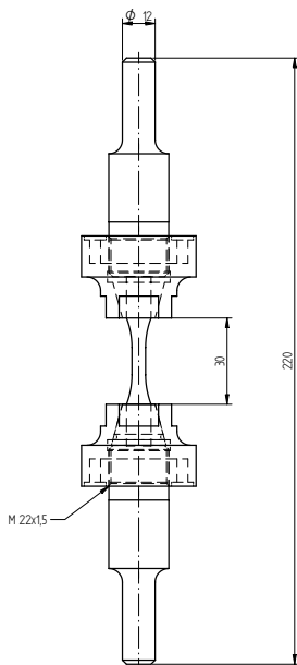
Abb. 3.3. Adapter für die TMF-Versuche
