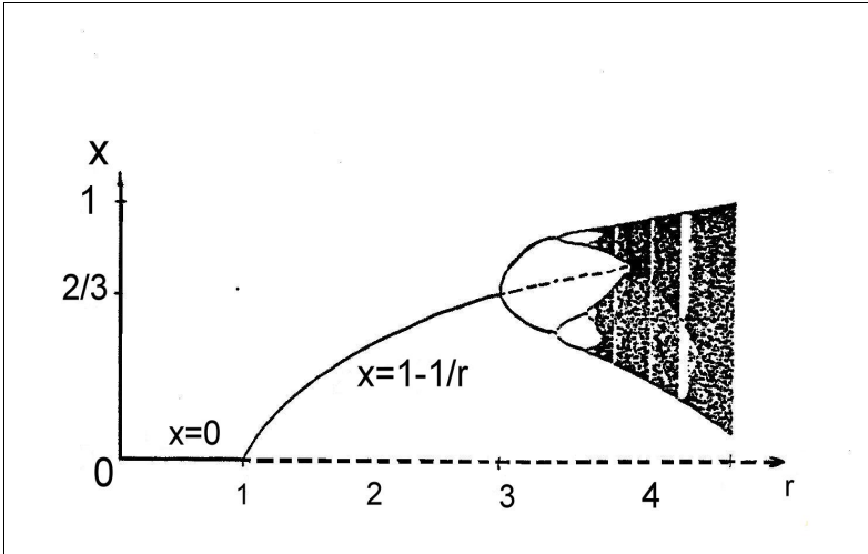
Abb. A1.5 9 : Bifurkationsdiagramm für die logistische Gleichung (3)
