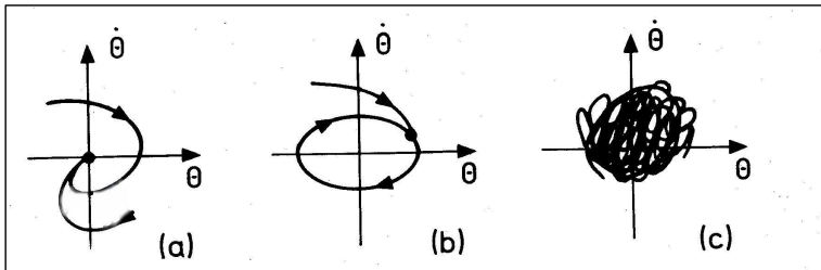
Abb. A1.2: Attraktoren bei erzwungenen Schwingungen eines Pendels. \theta ist der Auslenkwinkel aus der Ruhelage. (a) Fixpunkt bei Dämpfung, (b) Grenzyklus, (c) Seltsamer Attraktor 5
