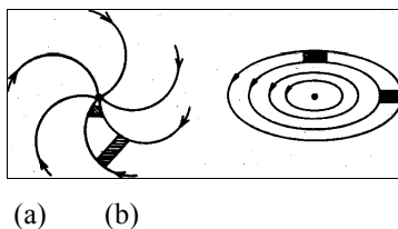
Abb. A1.3 7 : (a) Dissipatives System: Die Trajektorien laufen alle gegen den stabilen Fixpunkt (Attraktor) und das Phasenraumvolumen schrumpft; (b) Konservatives System: Das Zentrum ist stabil, aber kein Attraktor; und das Phasenraumvolumen ist konstant.
