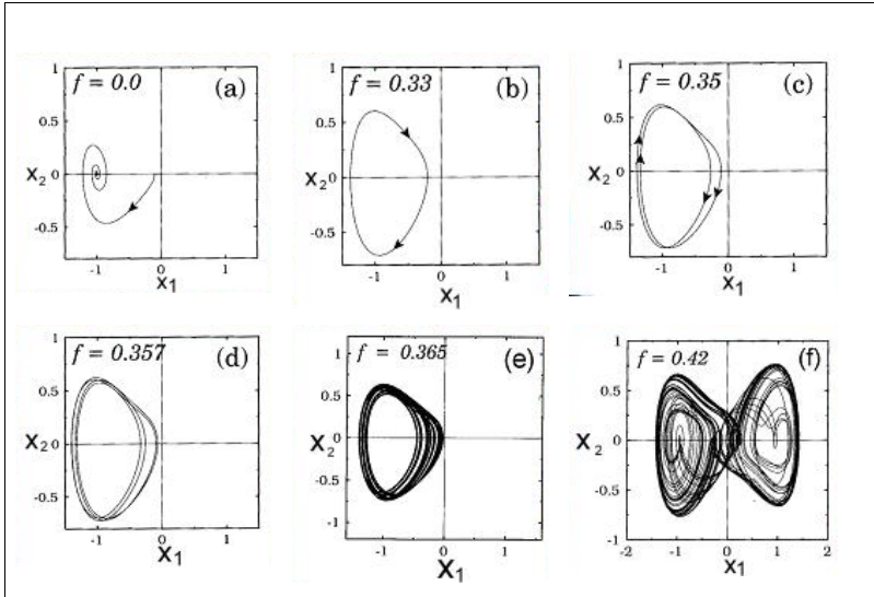
Abb. A1.6 10 : Phasenportraits x_2 = x_2(x_1) für den Duffing-Oszillator Gl. (1) für verschiedene Werte der Kraftamplitude f . Für die andern Parameter wurde gewählt: \gamma = 0,25 ; \alpha = -1 ; \beta = 1 ; \omega = 1 . Man hätte die Anfangsbedingung auch so wählen können, dass der rechts liegende Fixpunkt Ausgangspunkt der Trajektorien gewesen wäre
