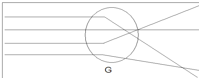
Abb. 5.1: Verschiedene mögliche denkbare Weltverläufe, die dem Determinismus genügen. G = Gegenwart. Die Abbildung gilt jetzt aber für den „schwachen Determinismus“: Kleine Abweichungen in den Anfangswerten können zu riesigen Abweichungen in den Endwerten führen.
