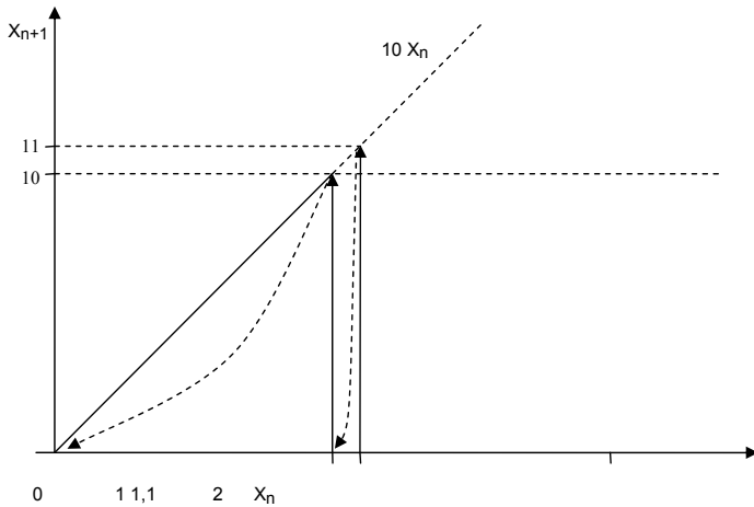
Abb. A1.1: Gleichung (4). Auf der Abszissenachse wählt man z. B. x_0=1,1 , dann ist 10x_0=11 . Der modulo-Operator teilt durch 10 und nimmt den Rest: 11/10=1 +\text{Rest } 1 , also x_1=1 . Dann ist 10x_1=10 . Erneute Anwendung des modulo-Operators liefert 10/10=1 +\text{Rest } 0 , also x_2=0 , und von hier kommt das System nicht mehr weg.
