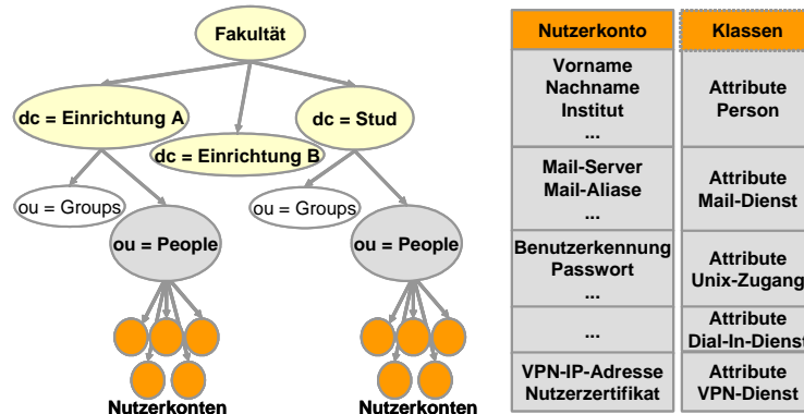
Abbildung 2: Dienstorientierte LDAP-Struktur der Nutzerdaten
