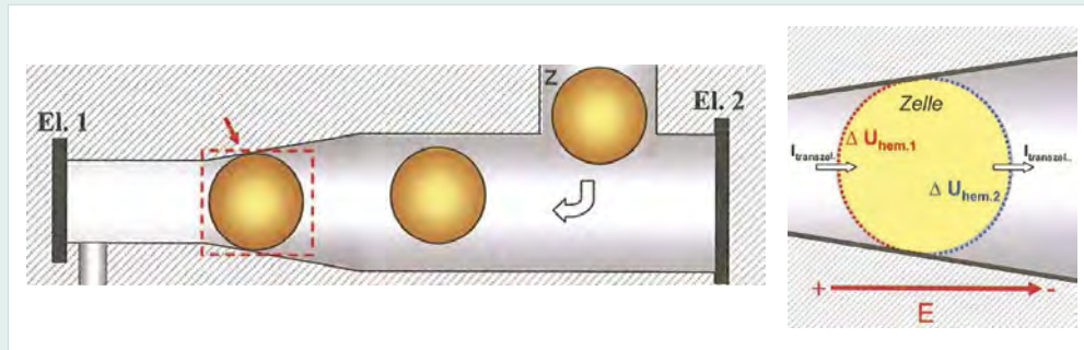
Schematische Darstellung der NIMEP-Technik: Positionierung der Zelle in einem mikrofluidischen System (Abb. links) mit einer vergrößerten Darstellung beim Anlegen eines elektrischen Feldes (Abb. rechts).
