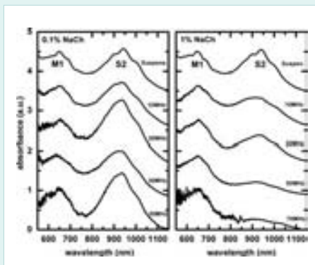
Optische Absorptionsspektren von Kohlenstoff-Nanoröhren-Filmen, hergestellt bei verschiedenen Wechselfeldfrequenzen und Tensidkonzentrationen. Metallische Röhren absorbieren bei M1, halbleitende bei S2.
