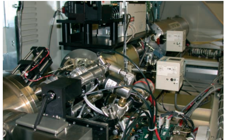
Blick auf das Innenleben des MALDI-Flugzeitmassenspektrometers 4700 Proteomics Analyzer; im Vordergrund ist der Laser und die Ionenquelle für die MALDI-Ionisation zu sehen
