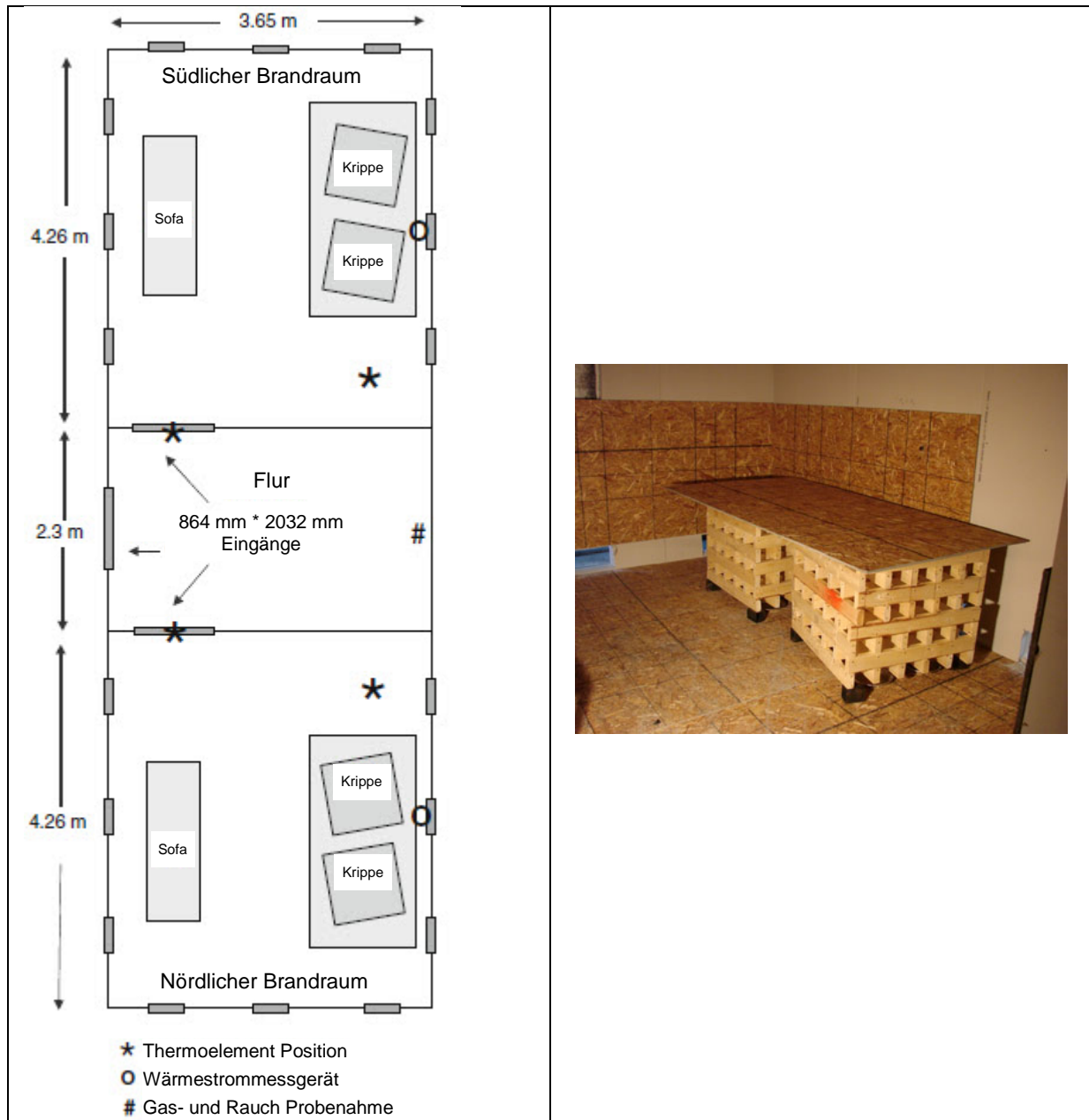
Abbildung 20: Bild links: Brandräume mit Flur (Bild links), Bild rechts: Brandlast (Holzkrippen und OSB-Platte) [Kim und Crampton /2009/, /69/]
