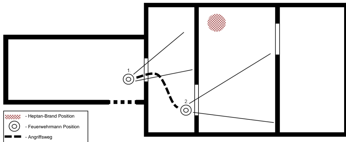
Abbildung 8: Lage des Wannenbrandes in der Versuchsanlage und Bewegung der Feuerwehreinsatzkraft beim Löscheinsatz [Lyckeback und Öhrn /2012/, /63/]
