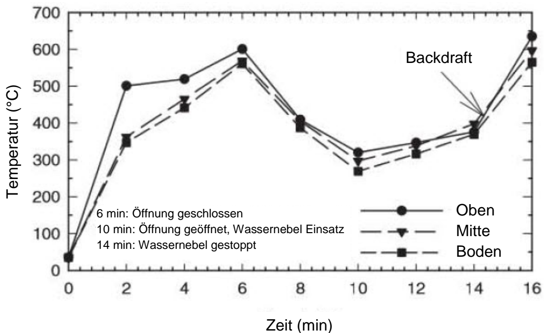
Abbildung 18: Vergleich der Temperaturverläufe bei den ventilationsgesteuerten Bränden unter Einsatz von Wassernebel (Brandszenarium 2) [Zhang, J. et al. /2011/, /64/]
