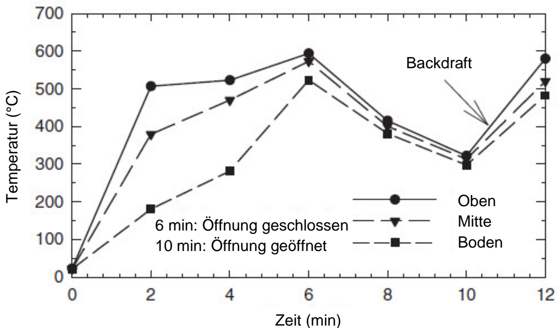
Abbildung 17: Vergleich der Temperaturverläufe bei den ventilationsgesteuerten Bränden ohne Löschmaßnahmen (Brandszenarium 1) [Zhang, J. et al. /2011/, /64/]
