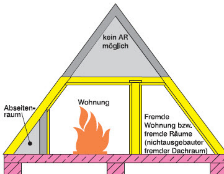
Abbildung 3: Feuerwiderstandsfähiger Dachausbau ohne Brandbrücken [Mayr und Battran /2013/, /15/]
