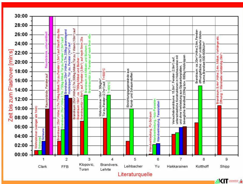
Abbildung 4: Zeit bis zur Entstehung eines Flashovers [Kunkelmann /2003/, /6/]
