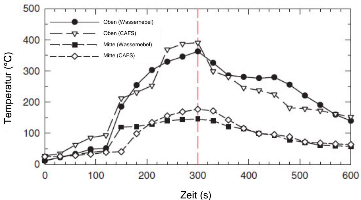
Abbildung 16: Vergleich der Temperaturentwicklung der oberen (Höhe: 1,5 m) und mittleren (Höhe: 1,0 m) Temperaturmessstellen bei den brandlastgesteuerten Brandversuchen mit Einsatz von Wassernebel und DLS [Zhang, J. et al. /2011/, /64/]
