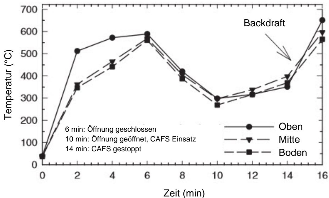
Abbildung 19: Vergleich der Temperaturverläufe bei den ventilationsgesteuerten Bränden unter Einsatz von Druckluftschaum (Brandszenarium 3) [Zhang, J. et al. /2011/, /64/]
