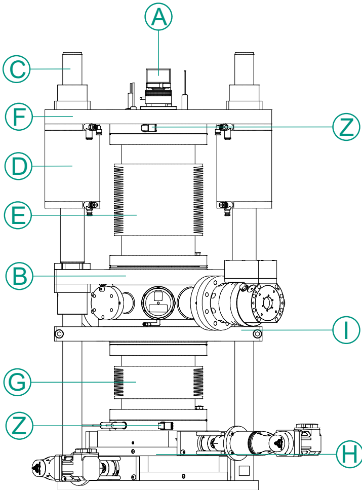
Abbildung C.1: Frontale Ansicht der Hochtemperatur-Vakuumpfchammer. Die Bezeichnung der Komponenten findet sich in Tab. D.11.
