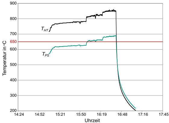
Abbildung 6.15: Heizversuch bis 650^{\circ}\text{C} an der Probe
