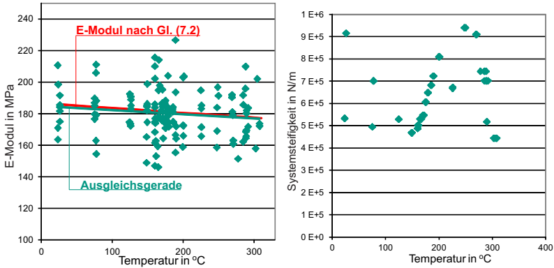
(a) Für die Indentationsversuche in Tantal angepasster E-Modul in Abhängigkeit der Prüftemperatur
