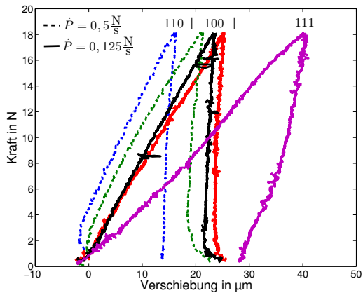
Abbildung 7.21: Vergleich von Indentationskurven für W-Einkristalle unterschiedlicher Orientierung bei 500°C. Die unterbrochenen Linien stellen Versuche mit einer Lastrate von 0,5 \text{ N/s} dar, für die restlichen Indentationskurven gilt eine Lastrate von 0,125 \text{ N/s} . Die deutlich geringere Entlastungssteifigkeit der Indentationskurve im (111)-Kristall wird einem Messfehler zugeschrieben.
