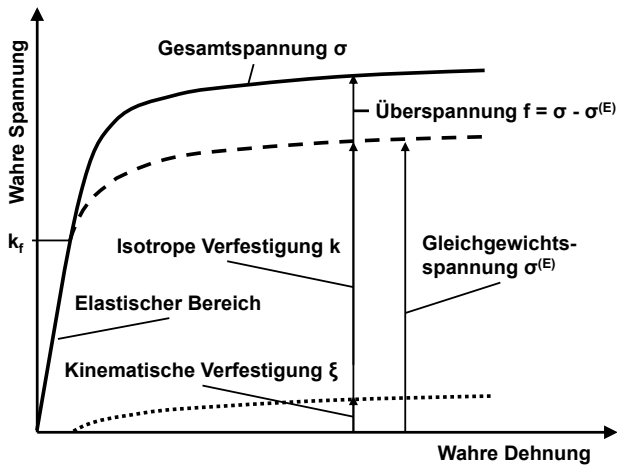
Abbildung 3.15: Zusammenhang zwischen den konstitutiven Größen, die mittels neuronaler Netze ermittelt werden, nach [71]
