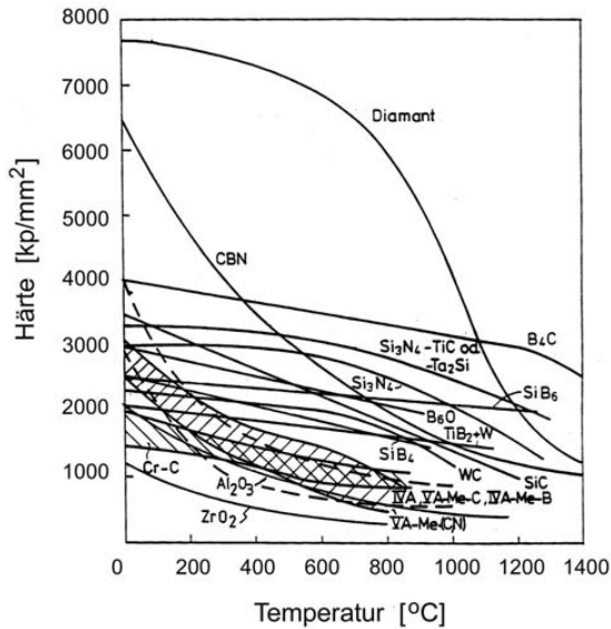
Abbildung 5.5: Hochtemperaturhärte einiger keramischer Werkstoffe nach [90, Kap. 5]
