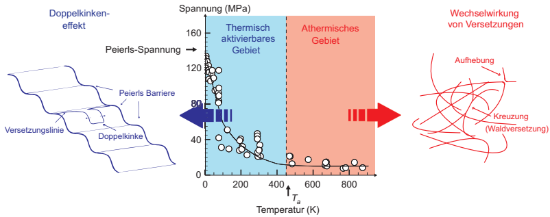
Abbildung 7.6: Abhängigkeit der kritischen Schubspannung von der Temperatur und dominierende Effekte der Versetzungsbewegung für MgO nach [111]
