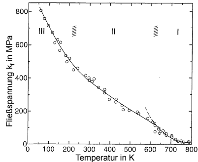
Abbildung 7.20: Temperaturabhängigkeit der Fließspannung k_f von Wolfram nach [122]
