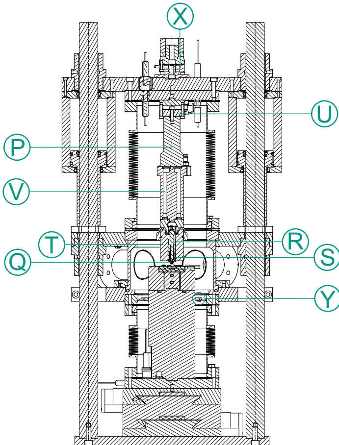
Abbildung C.4: Vertikale Schnittansicht der Hochtemperatur-Vakuumpfchkammer. Die Bezeichnung der Komponenten findet sich in Tab. D.11.
