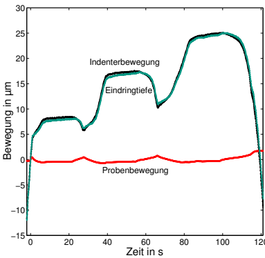
(c) Aus der Relativbewegung resultierende Eindringtiefe
