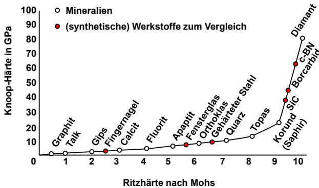
Abbildung 5.4: Korrelation zwischen Mohsscher Ritzhärte und Knoophärte nach [90, Kap. 5]
