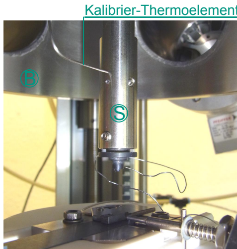
Abbildung 6.10: Temperaturmessung an der Heizpatrone. Die Isolationskeramik ① ist entfernt.
