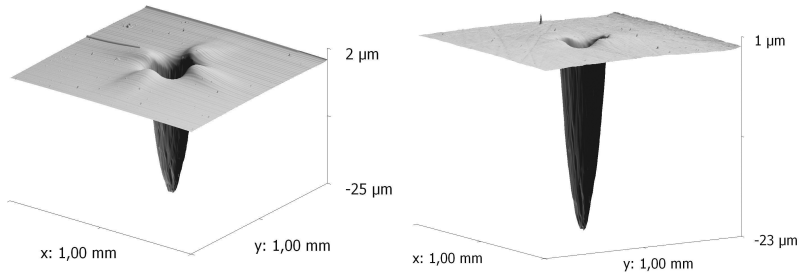
(a) Aufwurfmuster auf der (100)-Ebene
