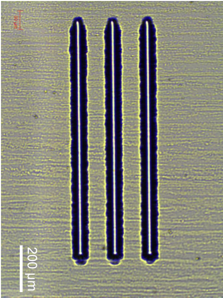
(a) In TZM geritzte Markierungen
