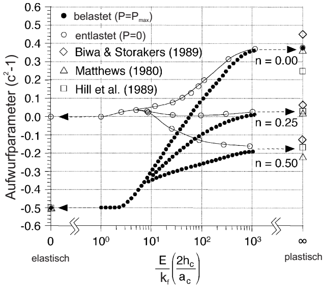
Abbildung 3.6: Abhängigkeit des Aufwurf factors c^2 von Materialparametern und Eindringtiefe nach [57]
