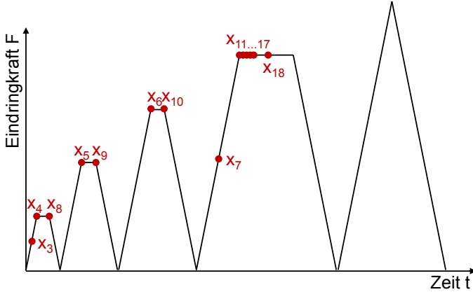
Abbildung 3.14: Für Eingangsneuronen verwendete Datenpunkte der multi-zyklischen Indentationskurve nach [68]
