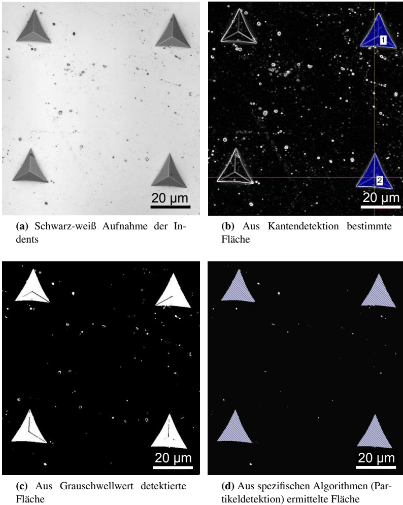
Abbildung C.16: Bestimmung der Indentfläche mit unterschiedlichen Methoden der Bildverarbeitung
