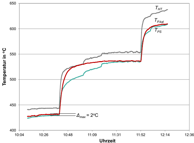
Abbildung 6.14: Darstellung der Temperaturen der Heizplatte T_{HT} , der Kalibrierprobe T_{P,kal} und des Thermoelements an der Seitenfläche der Probe T_{PS} während des Aufheizens
