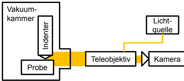
Abbildung 5.16: Schematische Darstellung des optischen Aufbaus zur Messung der Eindringtiefe
