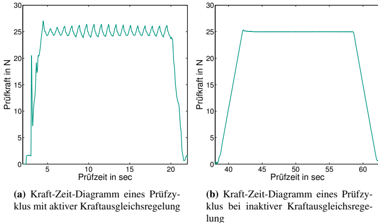
Abbildung 6.4: Einfluss der aktiven Kraftausgleichsregelung auf die Indentationsprüfung bei Normalatmosphäre
