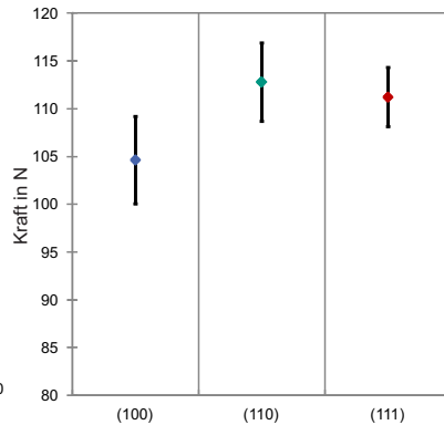
Abbildung 7.18: Mittelwerte und Standardabweichungen der für den Indentationszyklus nach Abb. 7.17 benötigten Kräfte
