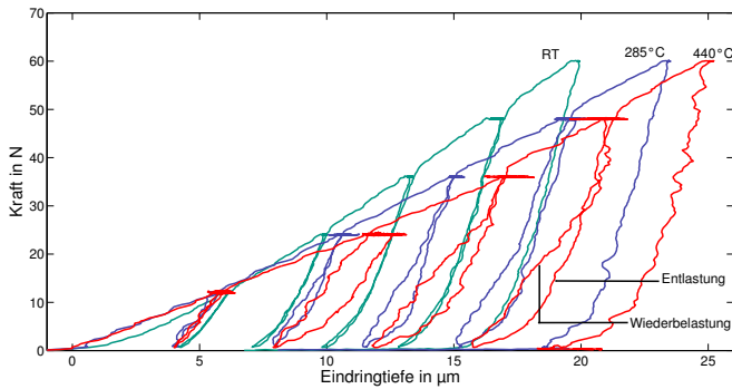
Abbildung 7.5: Last-Eindringtiefe-Kurven fünfzyklischer Indentationsversuche bei unterschiedlichen Temperaturen
