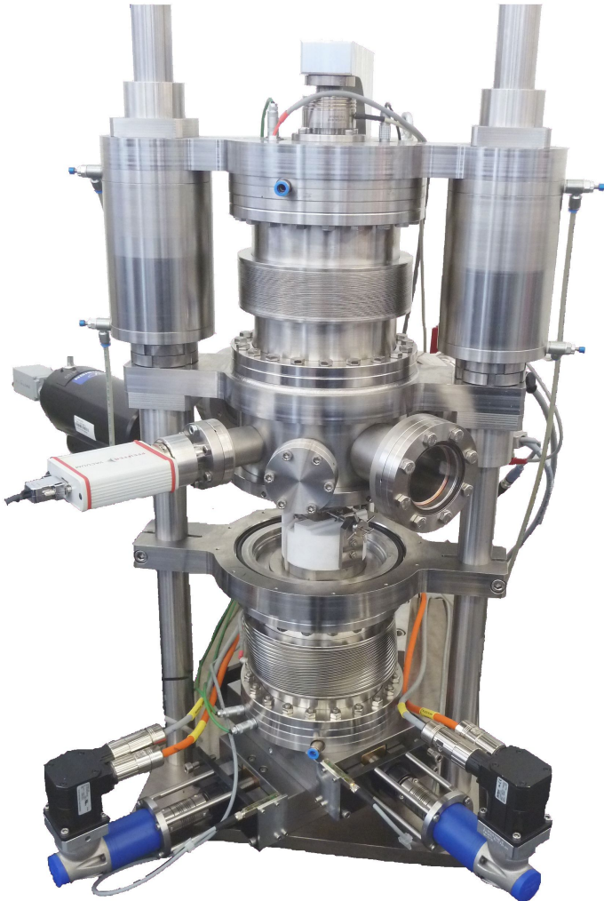
Abbildung 5.27: Karlsruher Hochtemperatur-Indentationsanlage KAHTI
