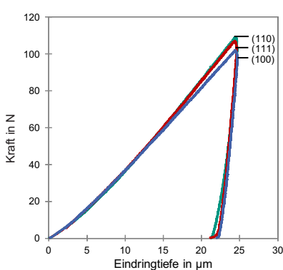
Abbildung 7.17: Indentationskurven für W-Einkristalle unterschiedlicher Orientierung
