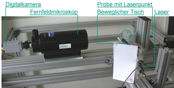
Abbildung 5.8: Versuchsaufbau zur Entwicklung eines optischen Verfahrens zur Messung der Eindringtiefe
