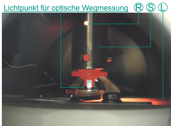
Abbildung 6.9: Heizung von Probe und TZM-Indentermodell auf T \geq 650^\circ\text{C} . Die Isolationskeramik \text{\textcircled{T}} ist entfernt.
