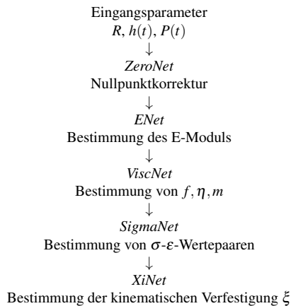
Abbildung 3.13: Ablauf der Berechnung mittels neuronaler Netze nach [69]
