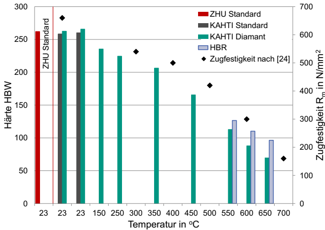
Abbildung 7.3: Temperaturabhängige Härte­werte der Eurofer-Probe E-FML-5 im Vergleich zur Zugfestigkeit von Eurofer nach [24]. Die einzelnen Werte sind nach verwendeter Prüfmaschine und eingesetztem Indenter unterteilt. Die mit „HBR“ gekennzeichneten Werte stellen die mit korrigierter Kontaktfläche bestimmten Härte­werte gemäß Anhang B.4 dar.
