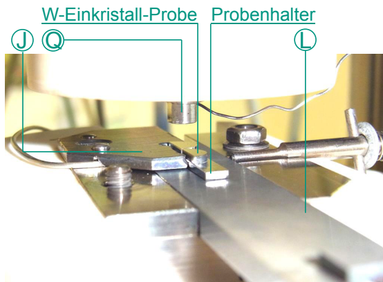
Abbildung 7.16: Positionierung halbiertter W-Einkristall-Proben mit geschliffener Trennfläche innerhalb KAHTI
