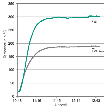
Abbildung 6.12: Vergleich der Temperaturmessungen an Indenterschaft und Eindring Spitze
