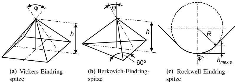
Abbildung 3.2: Nach DIN-EN-ISO 14577 [35, 36] empfohlene Eindringkörper
