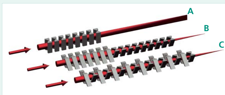
Fokussieren mit refraktiven Röntgenlinsen: Die senkrechten Linsen ergeben einen Linienfokus (Typ A), unter 90 Grad gekreuzte Linsen einen Punktfokus (Typ B und Typ C).
