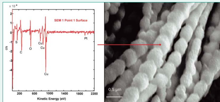
Quantitative Oberflächenanalyse an einem Kupfernanodraht.
