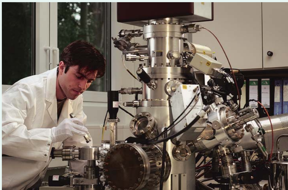
Eine Probe wird in die Scanning-Auger-Nanoprobe PHI 680 eingeschleust.
