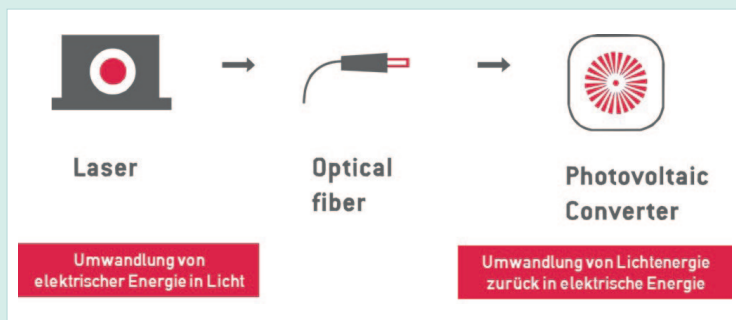
Ein rein optisches Konzept zur Energieversorgung elektrisch betriebener Sensoren.
