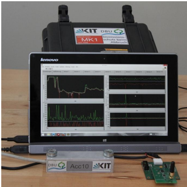
Abbildung 26: Messgraphen auf Tablett-PC, Beschleunigungssensor und Koordinator (ZigBee-Empfänger)
