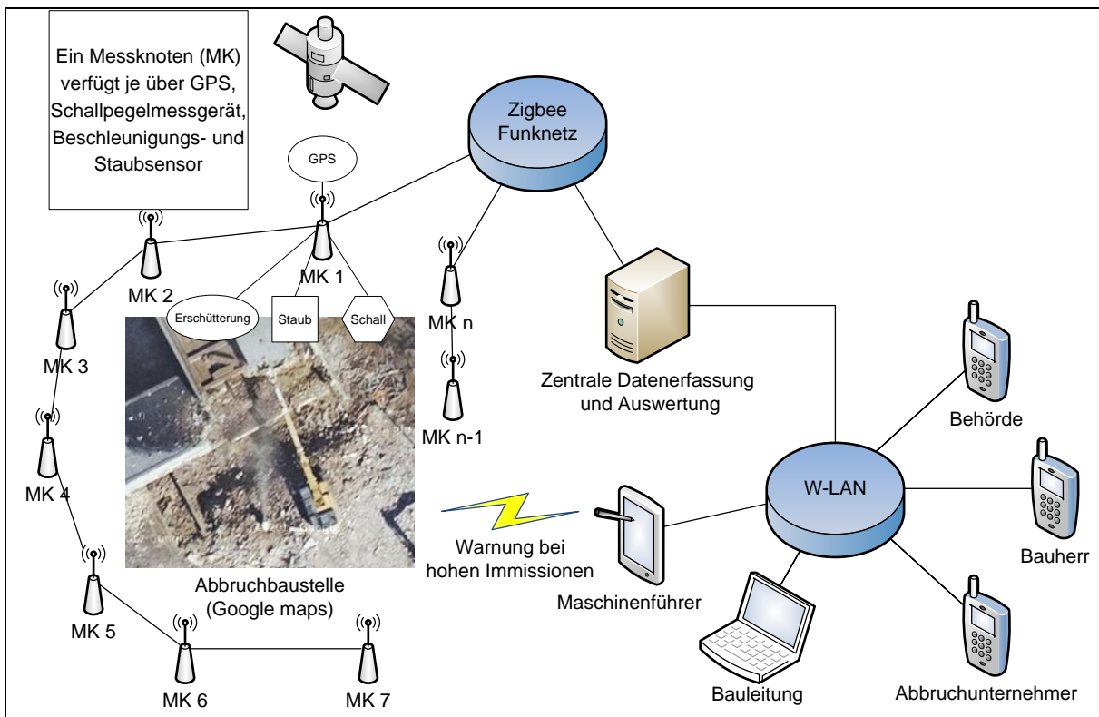
Abbildung 27: Aufbau des Immissionserfassungsystems
