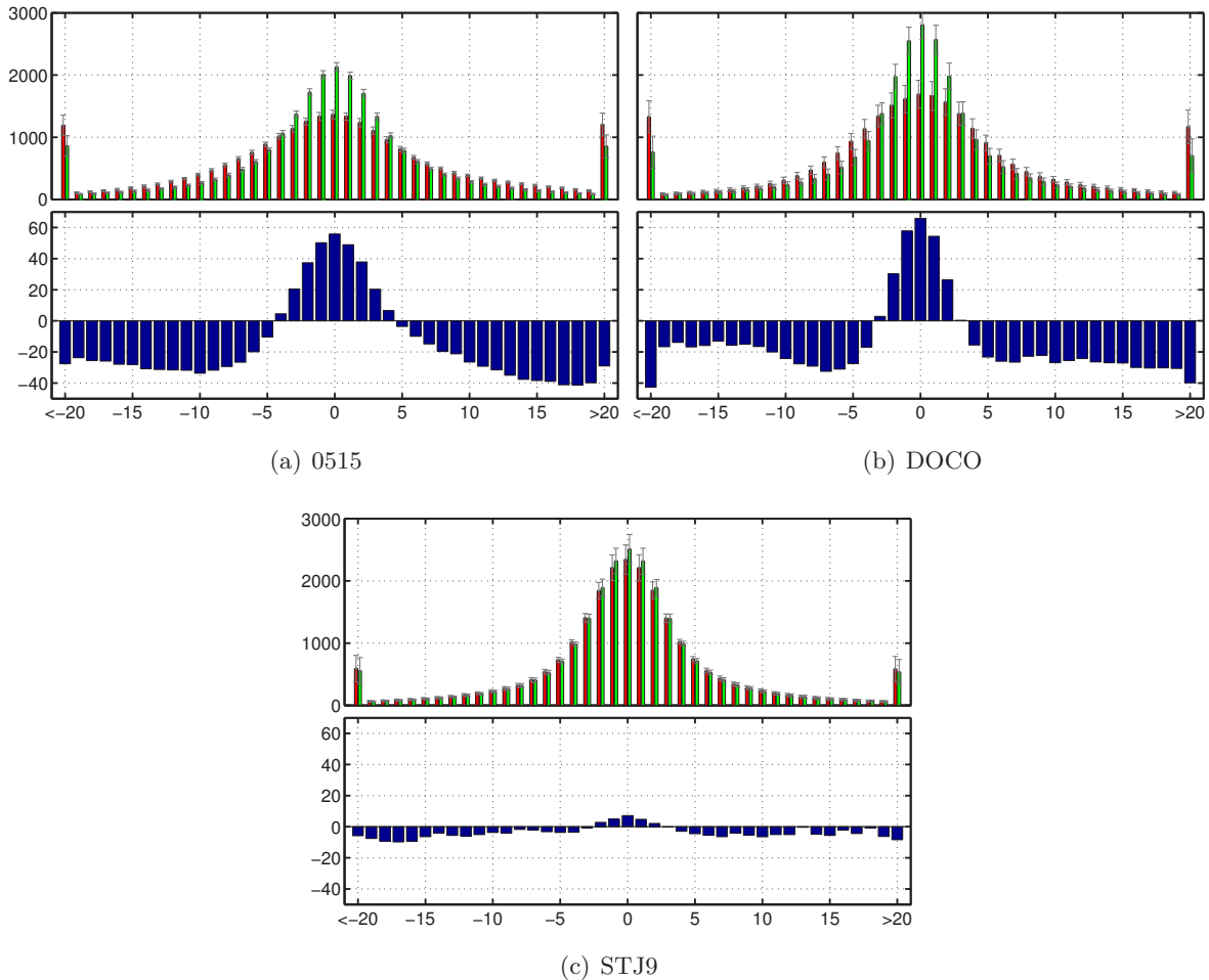
Abb. 6-17: obere Plots: Histogramm der Mediane der Residuenanzahl im Zeitraum DoY 131 bis 240 2013 über Residuenwerte; rot/grün ohne/mit Einführung gestackter Information; graue Balken: Standardabweichung der Residuenanzahl; Rechtsachse: Klassen der Residuenwerte [mm], Hochachse: Anzahl der Residuen einer Klasse; untere Plots: Prozentuale Zu-/Abnahme des Medians gestackt vs. roh nach Residuenklasse; Rechtsachse: Klassen der Residuenwerte [mm], Hochachse: Zunahme der Residuenanzahl [%]
