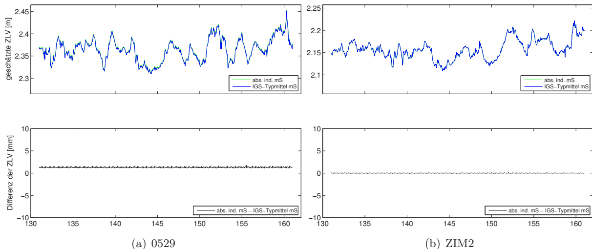
Abb. 7-6: Zenitale troposphärische Laufzeitverzögerungen für Zeitraum DoY 131 bis 160 2013; oben: Absolutwert für Varianten mit abs. ind. Kalibrierwerten und IGS-Typmittelwerten mit Einführung gestackter Information [m]; unten: Differenz abs. ind. minus IGS-Typmittel [mm]
