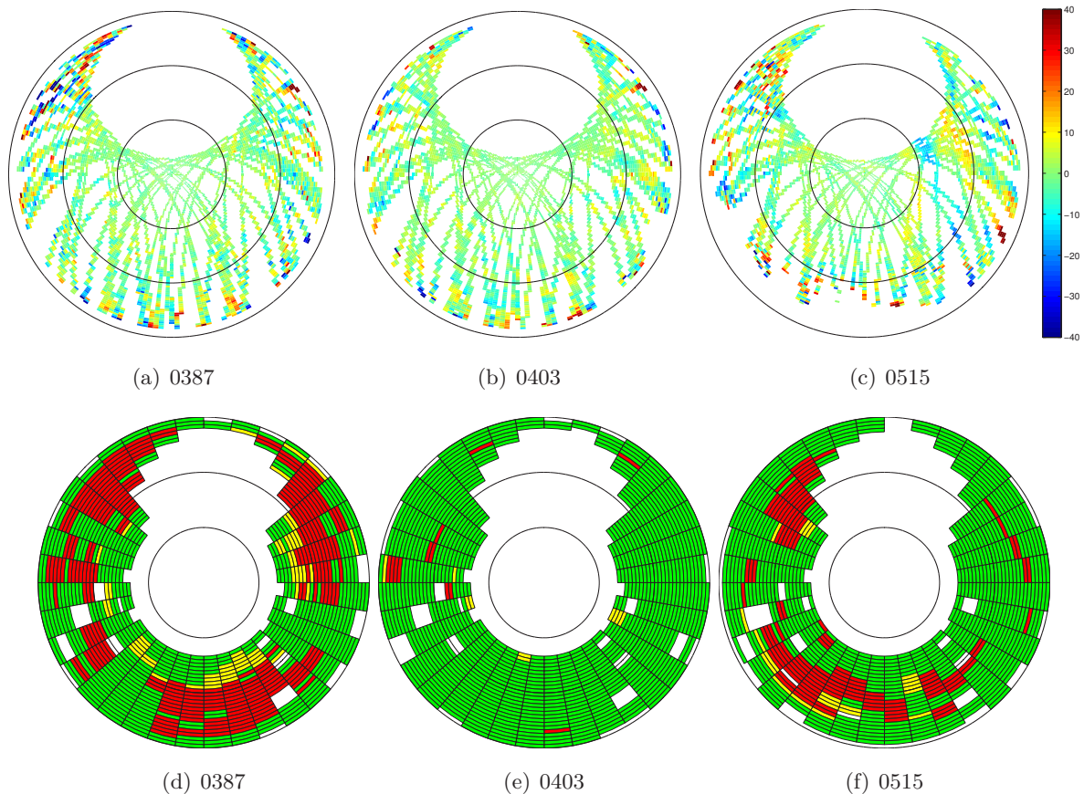
Abb. 6-11: oben: SMs des Zeitraums DoY 158 bis 167 2013; gestackte Werte in [mm]; unten: Mehrwegeanalyse in SAPOS ® Baden-Württemberg und SAPOS ® Rheinland-Pfalz für Zeitraum DoY 160-166 2013; Darstellung in Form von Skyplots; grün/gelb/rot: Daten vorhanden und geringer/mittlerer/starker Mehrwegeeinfluss für diese Zelle; konzentrische Kreise (von aussen nach innen): Elevationen 0°, 30°, 60°
