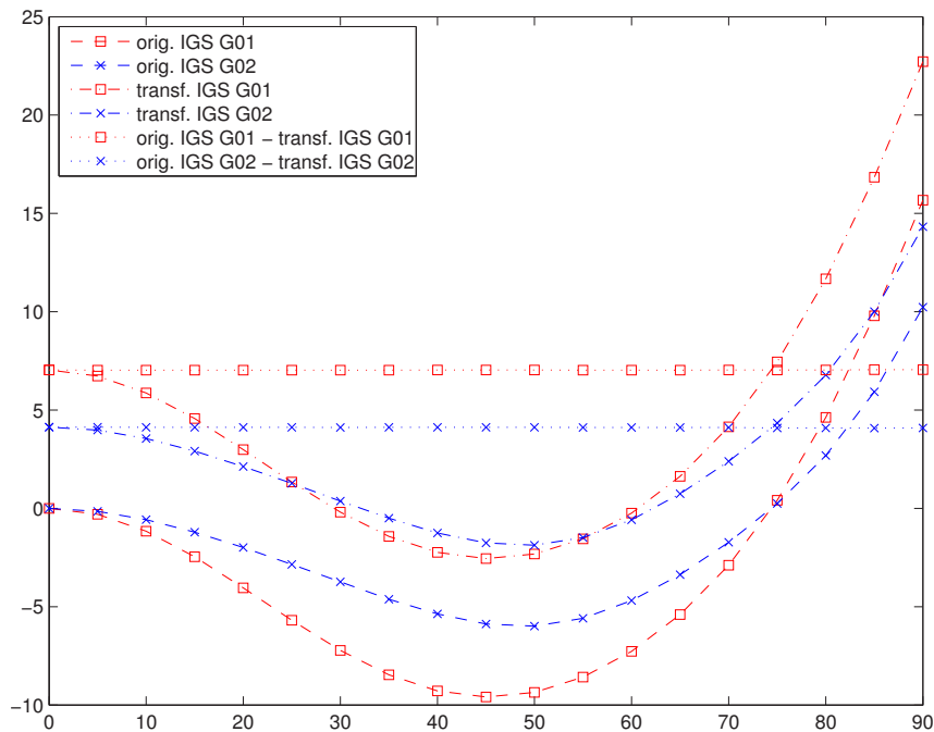
Abb. 7-1: Zenitdistanzabhängige originäre (---) und transformierte (- · -, mit CCANTEX auf IGS-PZO dieser Antenne umgerechnet) PZV der IGS-Typmittelwerte einer Antenne des Typs LEIAT504GG LEIS sowie deren Differenzen (···) für G01 (rot) und G02 (blau); Rechtsachse: Zenitdistanz [°], Hochachse: PZV-Wert bzw. Differenz [mm]
