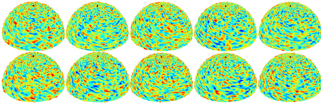
Abb. 4-4: Schematische Darstellung zufälliger und systematischer Fehler auf der Antennenhemisphäre für zehn aufeinanderfolgende Tage, korrigiert um systematische Anteile; schwarzer Punkt: lokaler Zenit
