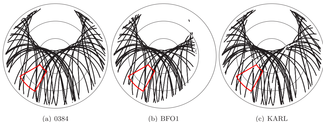
Abb. 6-4: Plot der Residuen für DoY 200 2013 mit originären PZV ohne Modifikation; rot-umrandeter Bereich: PZV-Sektor, der in anderen Versionen modifiziert wurde; konzentrische Kreise (von innen nach aussen): Zenitdistanz 30^\circ , 60^\circ , 90^\circ
