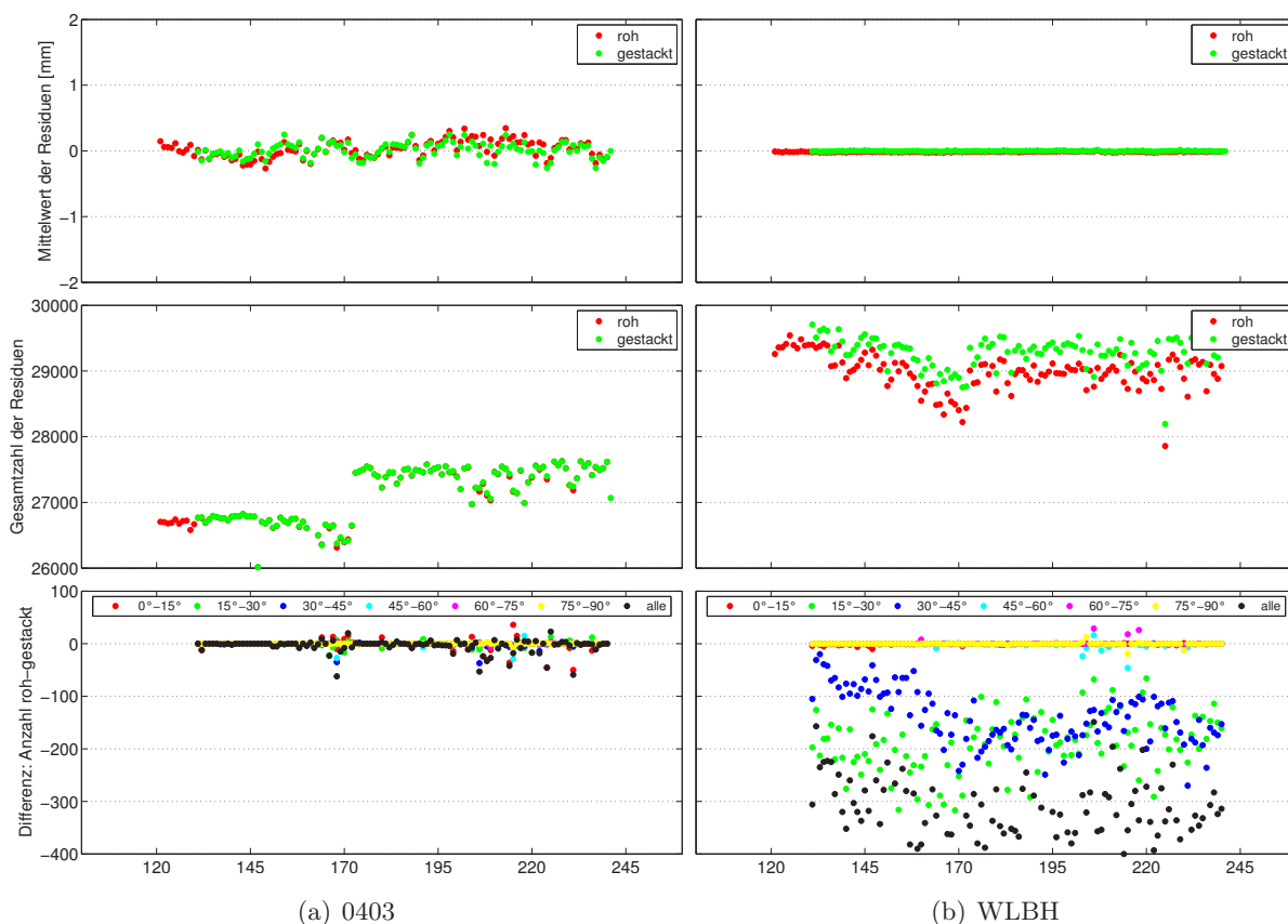
Abb. 6-13: Residuenanalyse ohne/mit Einführung gestackter Information im Zeitraum DoY 121-240 2013; oben: gemittelter Wert über alle Residuen [mm]; Mitte: Gesamtzahl der Residuen; unten: Differenz der Residuenanzahl: roh minus gestackt, nach Elevationsstufen (farbliche Codierung siehe Grafik in unterster Zeile) und für alle Residuen (schwarz)
