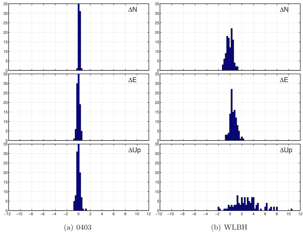
Abb. 6-19: Histogramme der Differenz der Koordinatenzeitreihen ohne minus mit Einführung gestackter Information im Zeitraum DoY 131-240 2013 im topozentrischen Koordinatensystem; Rechtsachse: Differenz [mm], Hochachse: [Anzahl d], Balkenbreite 0.25 mm
