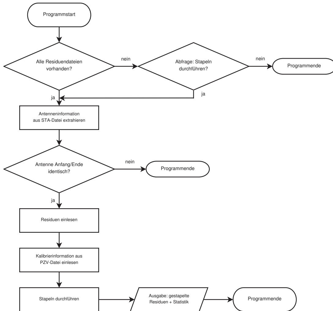
Abb. 4-7: Übersicht des Stacking-Ablaufes
