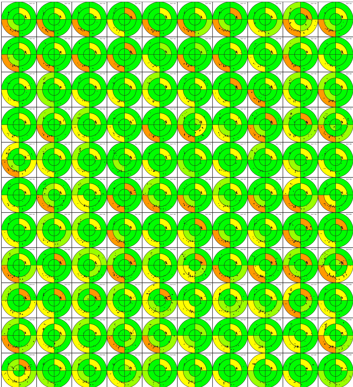
Abb. B-3: Station 0515: nach Sektoren unterteilte Zunahme der Residuenanzahl nach Einführung gestackter Information gegenüber roher Prozessierung im Zeitraum DoY 131 bis 240 2013; grün/hellgrün/gelb/orange/rot: Zunahme um 0–1%/1–2%/2–5%/5–10%/>10%; azimuthale Aufteilung: 0°–90°, 90°–180°, 180°–270° und 270°–360°; Elevationsstufen: 0°–30°, 30°–60° und 60°–90°; schwarze Punkte: durch Stacking in die Auswertung hinzugekommene Residuen
