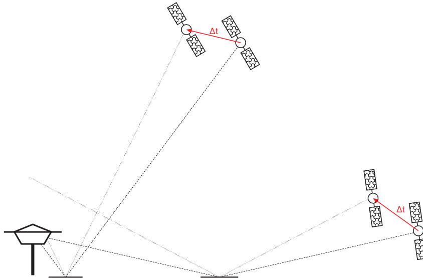
Abb. 3-1: Änderung der Reflexionsgeometrie naher und entfernter Reflektoren durch geänderte Satellitengeometrie
