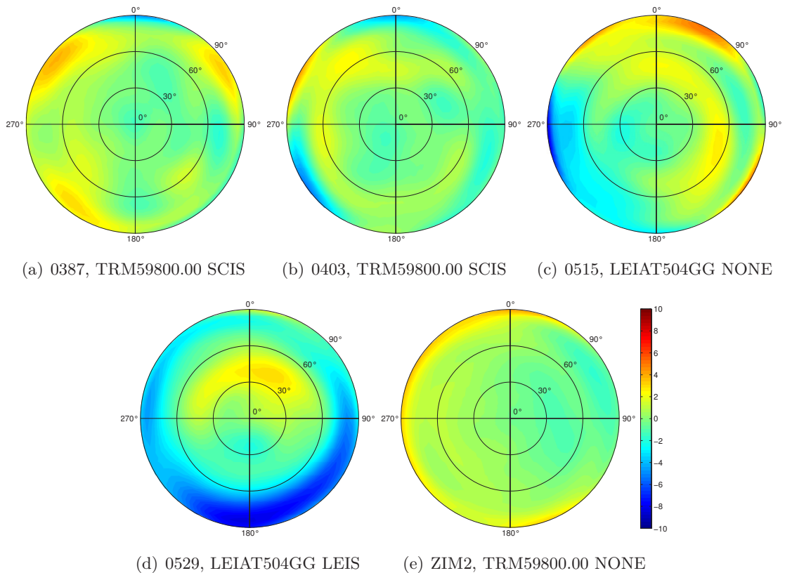
Abb. 7-2: Differenz der auf den IGS-PZO der jeweiligen Antenne umgerechneten individuellen PZV-Werte zum IGS-Typmittel auf L_3 -Niveau der einzelnen Stationen mit den dort genutzten Antennentypen; Werte der Farbskala in [mm]; konzentrische Kreise (von innen nach aussen): Zenitdistanz 30°, 60°, 90°
