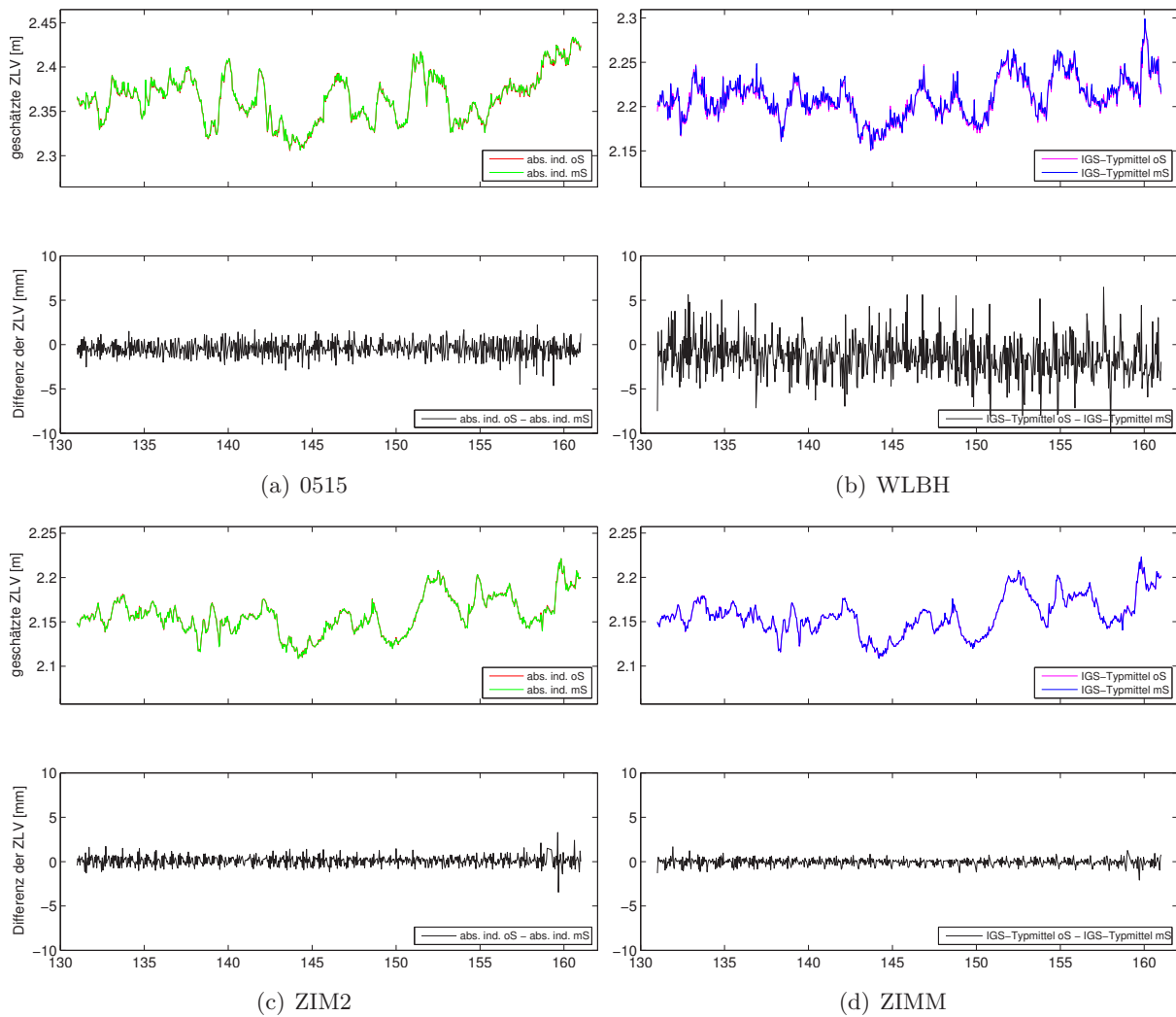
Abb. 6-21: Zenitale troposphärische Laufzeitverzögerungen für Zeitraum DoY 131 bis 160 2013; oben: Absolutwert für Varianten ohne (oS) und mit (mS) Einführung gestackter Information; unten: Differenz oS minus mS
