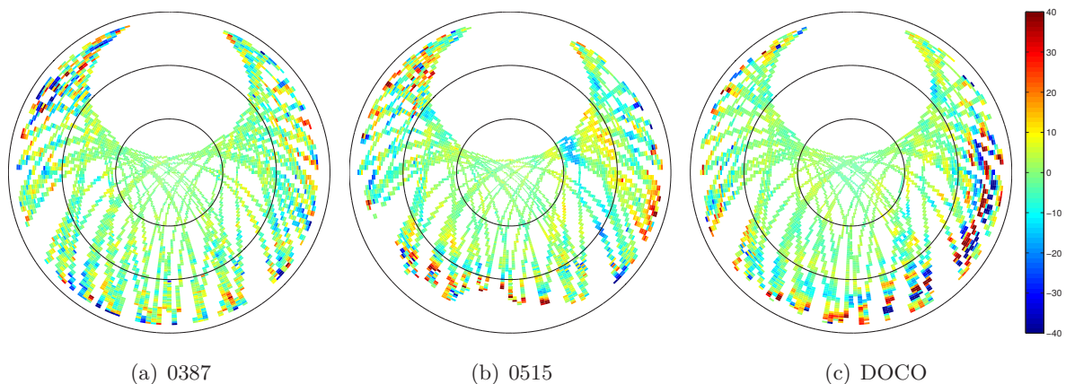
Abb. 6-8: SMs für den Zeitraum DoY 121 bis 130 2013; farbliche Skalierung: Wert des gestackten L_3 -Residuums in [mm]; konzentrische Kreise (von aussen nach innen): Elevationen 0^\circ , 30^\circ , 60^\circ ; Farbskalierung gegenüber Abb. 6-7 modifiziert
