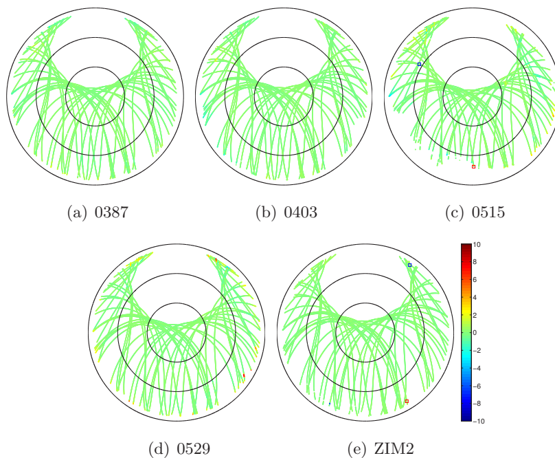
Abb. 7-4: Differenz der L_3 -Residuen für DoY 131 2013: Prozessierung mit individuellen Kalibrierwerten minus Prozessierung mit IGS-Typmittel (jeweils Absolutniveau), in beiden Fällen mit Einführung der gestapelten Residueninformation; Werte der Farbskala in [mm]; rote/blau Quadrare: Residuen treten nur in Prozessierung mit Individualkalibrierung/IGS-Typmittel auf; konzentrische Kreise (von innen nach aussen): Zenitdistanz 30°, 60°, 90°
