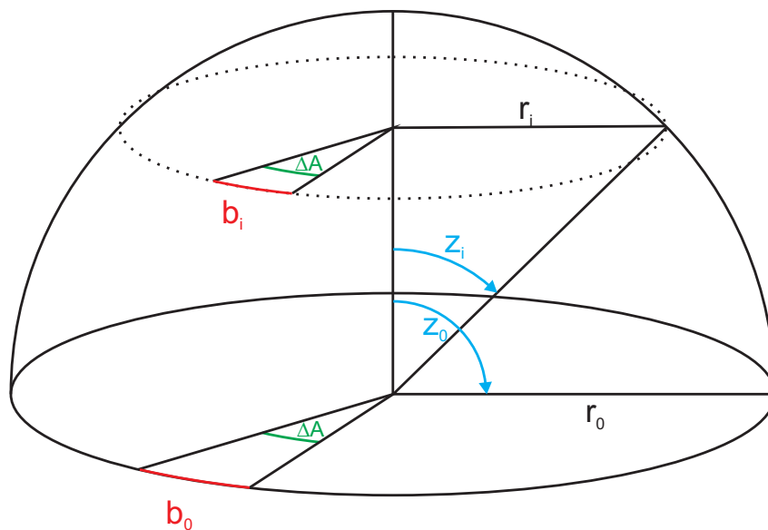
Abb. 8-1: Schematische Darstellung der Änderung der Bogenlänge mit abnehmender Zenitdistanz z
