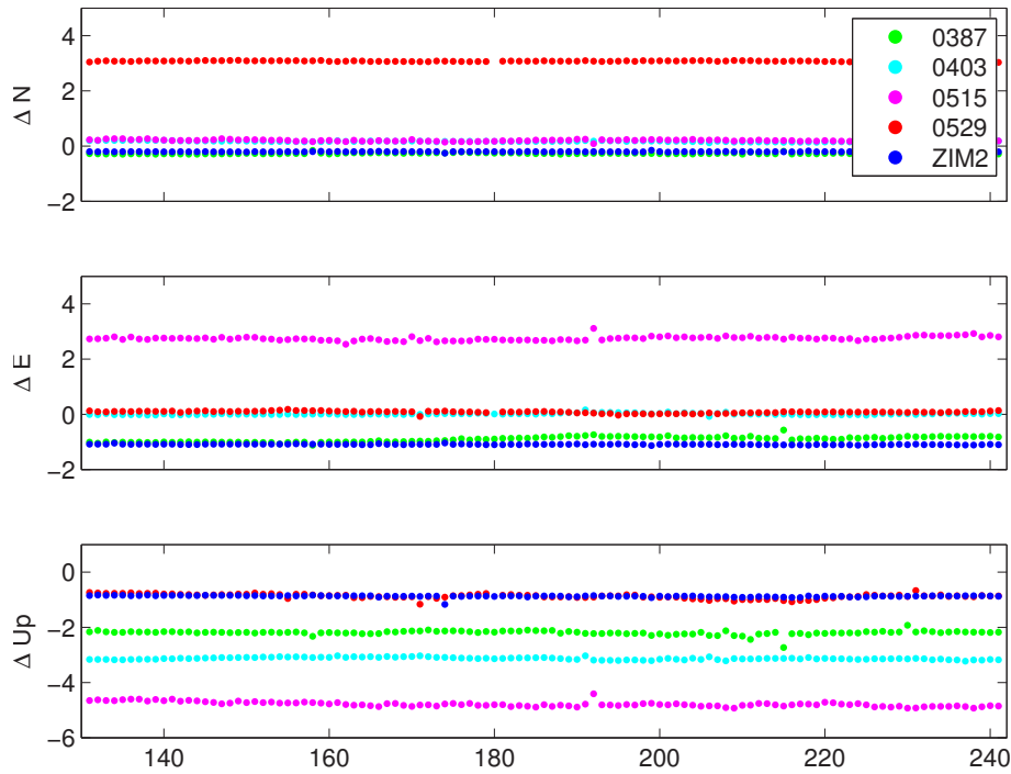
Abb. 7-5: Differenzen der einzelnen Koordinatenkomponenten \Delta N , \Delta E , \Delta Up ; Variante mit abs. ind. Kalibrierwerte minus Variante mit IGS-Typmittelwerten jeweils inklusive gestapelte Residueninformation; Rechtsachse: DoY des Jahres 2013, Hochachse: Differenz [mm]
