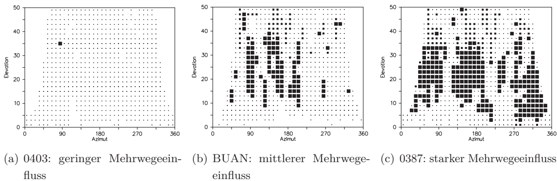
Abb. 6-5: Mehrwegeanalyse im GURN für Zeitraum DoY 127 bis 133 2012; kleines/mittleres/großes Quadrat: Daten vorhanden und geringer/mittlerer/starker Mehrwegeeinfluss für dieses Pixel
