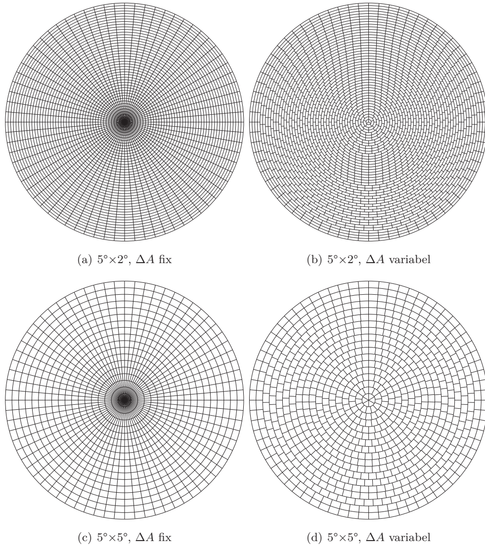
Abb. 8-2: Darstellungen verschiedener Zellgrößen bei festem Azimutinkrement über alle Zenitdistanzbereiche (links) und variablem Azimutinkrement in Abhängigkeit von der Zenitdistanz (rechts) in Form einer mittabstandstreu azimutalen Abbildung der Halbkugel; Zellgröße: \Delta A_0 \times \Delta z
