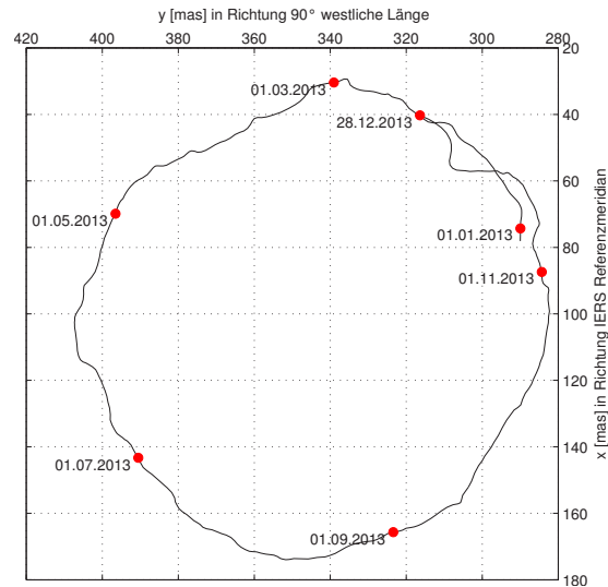
Abb. 2-2: Darstellung der Polbewegung zwischen 30.12.2012 und 28.12.2013 aus Erdrotationsparametern der finalen CODE-Lösungen für die GPS-Wochen 1721 bis 1772
