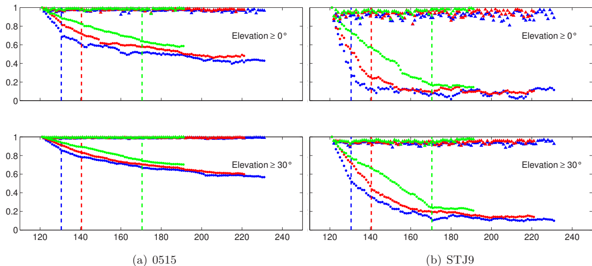
Abb. 6-10: Korrelationskoeffizienten (KK) der Stackingmaps (SMs) verschiedener Stackingzeiträume: 10/20/50 d in blau/rot/grün; Symbole: Dreieck: KK der SM aufeinanderfolgender Tage, Kreis: KK zur ersten SM, jeweils am ersten Tag der SM eingetragen; senkrechte gestrichelte Linien: Ende des Zeitraums der ersten SM; oben: komplette SM, unten: nur Bereiche der SM mit Elevationen \geq 30^\circ ; Rechtsachse: DoY 2013, Hochachse: Korrelationskoeffizient
