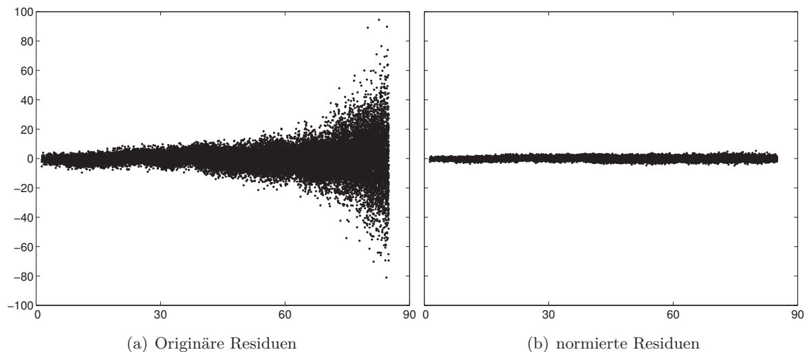
Abb. 8-5: Originäre und normierte Residuen für die Station ZIM2 aus PPP-Prozessierung von DoY 131 2013; Rechtsachse: Zenitdistanz [°], Hochachse: Residuenwert [mm]
