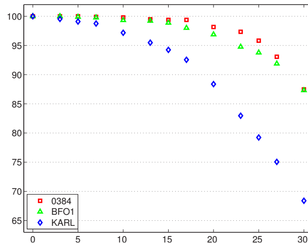
Abb. 6-3: Entwicklung der Residuenanzahl im modifizierten Sektor in Abhängigkeit vom addierten Wert auf L_3 -PZV; Rechtsachse: auf L_3 addierter Wert [mm], Hochachse: Verhältnis des Mittelwerts der Residuenanzahl mit veränderten PZV zu unveränderten PZV des modifizierten Sektors [%] im Zeitraum DoY 199 bis 208 2013
