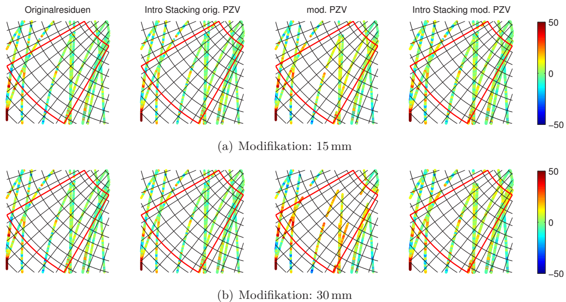
Abb. 6-2: Residuenplots der Station KARL für DoY 199 2013 aus Prozessierungen verschiedener Varianten; rot-umrandeter Bereich: modifizierter PZV-Sektor; Farbskala: Residuenwerte in [mm]; schwarze Gitterlinien: gewähltes Stackingraster (Azimut \times Zenitdistanz = 5^\circ \times 5^\circ )
