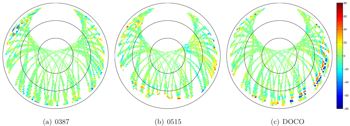
Abb. 6-7: SMs für den Zeitraum DoY 121 bis 130 2013; farbliche Skalierung: Wert des gestackten L_3 -Residuums in [mm]; konzentrische Kreise (von aussen nach innen): Elevationen 0^\circ , 30^\circ , 60^\circ
