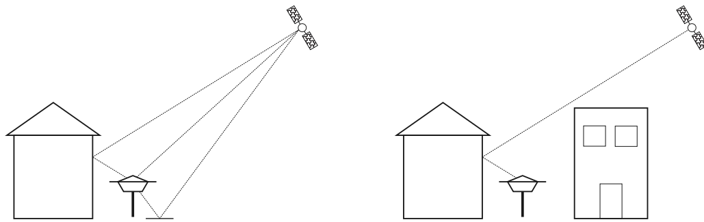
Abb. 2-3: Prinzipskizze zu Mehrwegeeffekten nach [Seeber, 2003, S. 316]
