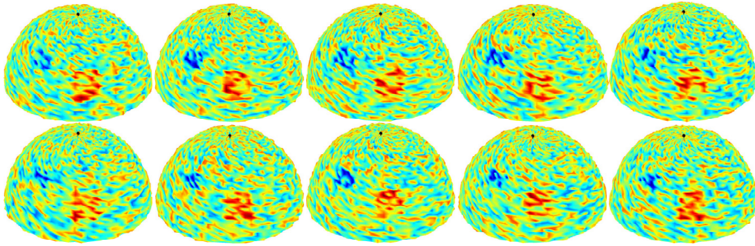
Abb. 4-2: Schematische Darstellung zufälliger und systematischer Fehler auf der Antennenhemisphäre für zehn aufeinanderfolgende Tage; schwarzer Punkt: lokaler Zenit
