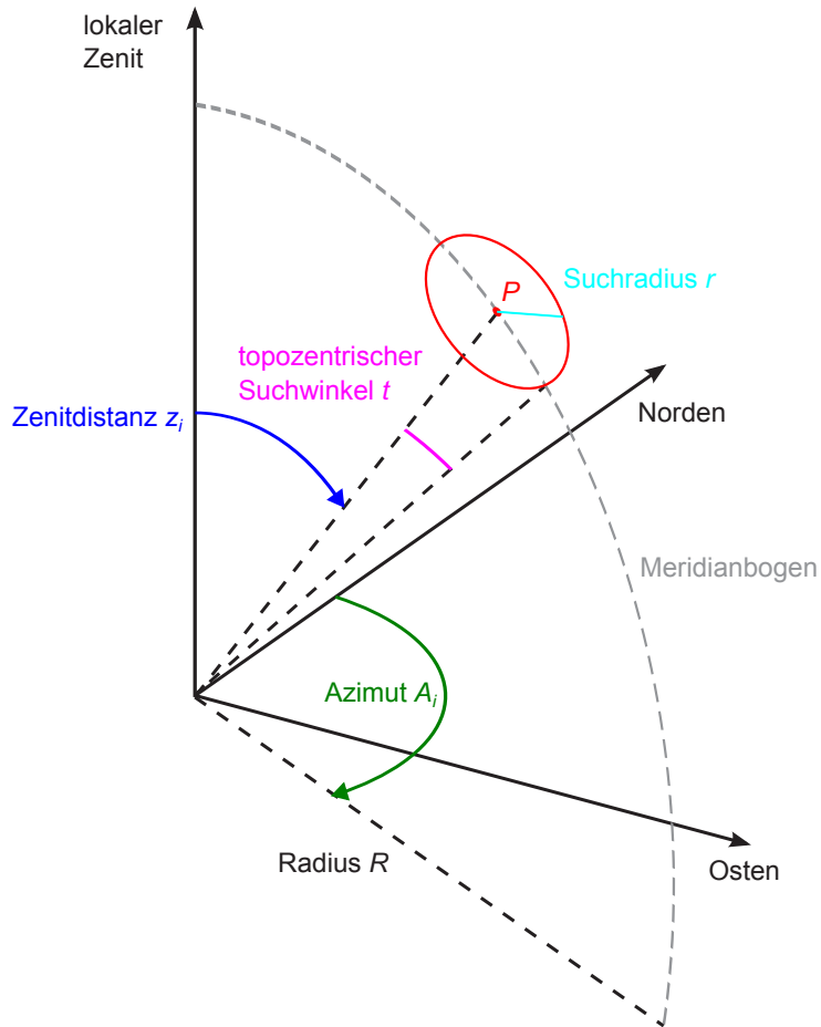
Abb. 8-7: Schematische Darstellung der Definition eines topozentrischen Suchwinkels
