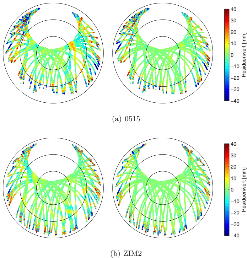
Abb. 6-12: Vergleich der Residuen aus einer Auswertung ohne (links) und mit (rechts) Einführung gestackter Information für DoY 131 2013 für die Stationen 0515 (oben) und ZIM2 (unten)
