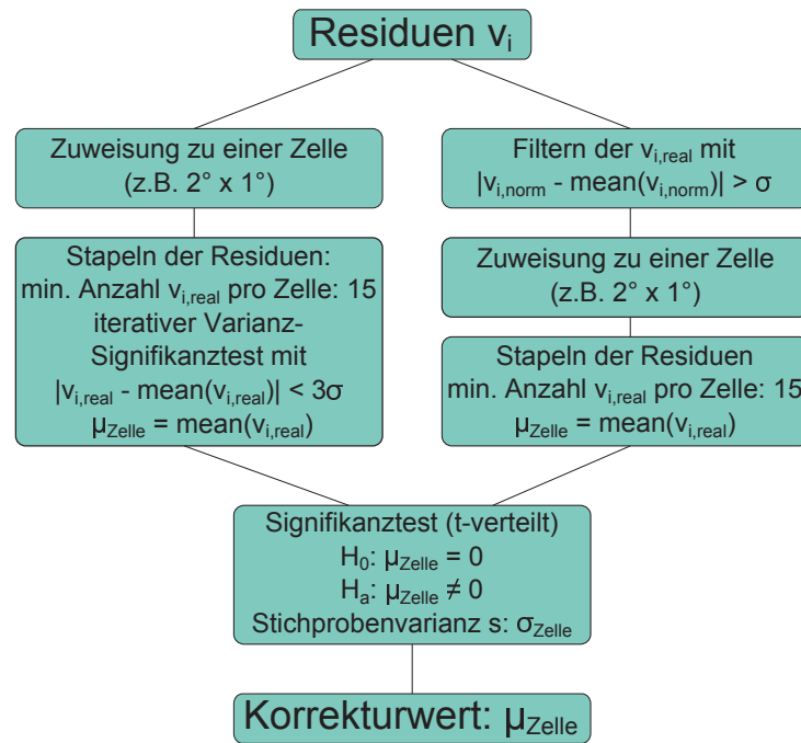
Abb. 8-4: Schematische Darstellung der zwei Varianten des Stackingablaufs mit statistischem Test der Residuen nach [Fuhrmann u. a., 2010, S. 83]; v_{i,real} : originäre Residuen, v_{i,norm} : normierte Residuen
