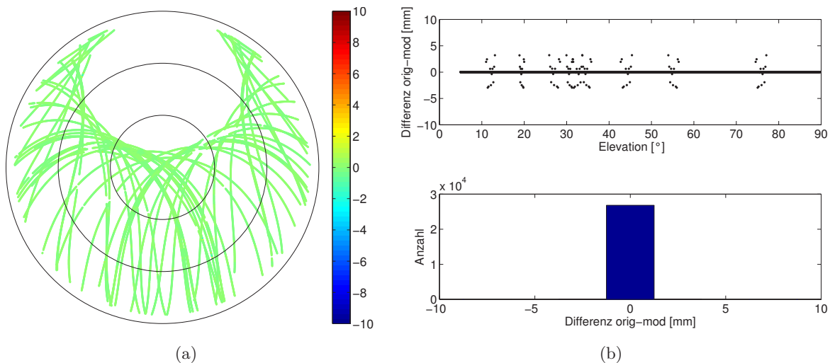
Abb. 4-6: Unterschiede der Rohresiduen aus den Prozessierungen mit originären und auf L_3 umgerechneten PZV für Station KARL, DoY 199 2013; Differenzen: originäre minus modifizierte PZV
