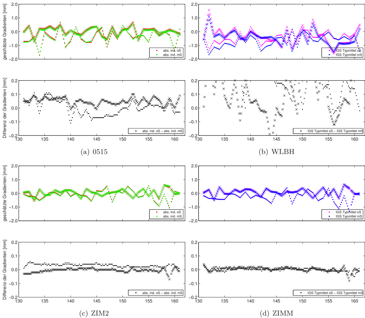
Abb. 6-22: Horizontale Gradienten der zenitalen troposphärischen Laufzeitverzögerungen für Zeitraum DoY 131 bis 160 2013; oben: Absolutwert für Varianten ohne (oS) und mit (mS) Einführung gestackter Information; unten: Differenz oS minus mS; Punkt: Nordkomponente, Kreuz: Ostkomponente; nur jeder vierte Datenpunkt dargestellt
