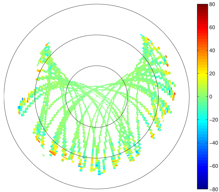
Abb. B-6: Stackingmap der Station WLBH für Zeitraum DoY 121 bis 130 2013; farbliche Skalierung: Wert des gestackten L_3 -Residuums in [mm]; konzentrische Kreise (von aussen nach innen): Elevationen 0^\circ , 30^\circ , 60^\circ
