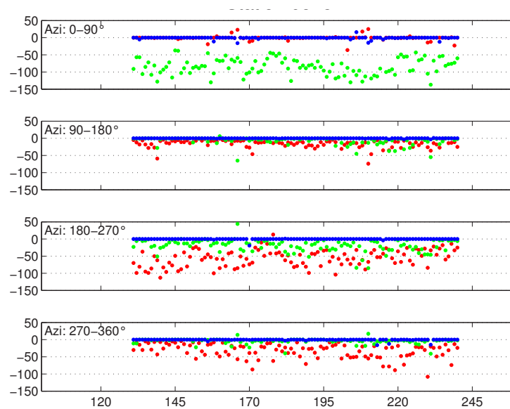
Abb. B-2: Station 0515: Differenz der Residuenanzahl ohne minus mit Einführung gestackter Information im Zeitraum DoY 131-240 2013; Unterteilung in Azimutbereiche (Zeilen der Grafik) und Elevationsbereiche (farbliche Codierung) mit 0°–30° (rot), 30°–60° (grün), 60°–90° (blau)
