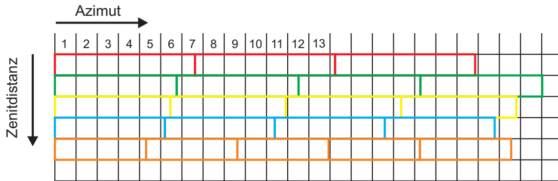
Abb. 8-3: Schematische Darstellung der Abbildung von Zellen mit variablem Azimutinkrement in einer Matrix; die Breite der buntumrandeten Rechtecke steht für das entsprechende Azimutinkrement, die schwarzumrandeten Zellen für die einzelnen Elemente der Matrix
