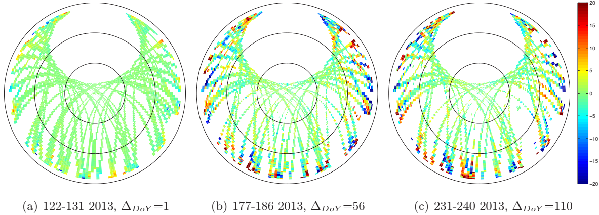
Abb. 6-9: Differenzen der SMs der Station 0403 für drei ausgewählte Stackingzeiträume zur SM für Zeitraum DoY 121 bis 130 2013; farbliche Skalierung: Wert des gestackten L_3 -Residuums in [mm]; konzentrische Kreise (von aussen nach innen): Elevationen 0°, 30°, 60°
