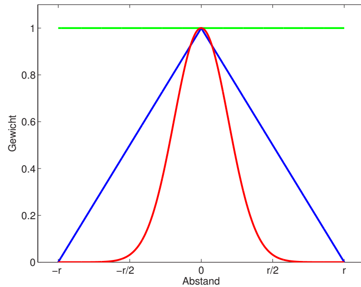
Abb. 8-8: Mögliche Varianten für abstandsabhängige Gewichtung: Gleichgewichtung (grün), lineare Gewichtung (blau), Gauß'sche Glockenkurve (rot)
