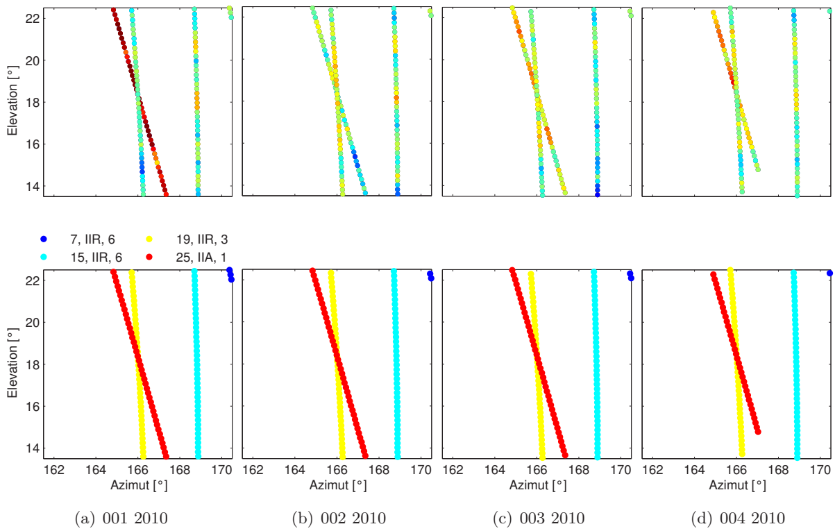
Abb. B-7: Plots der Rohresiduen der Station DILL für einen Ausschnitt der Antennenhemisphäre im Zeitraum DoY 001 bis 010 2010; oben: Residuenwert farblich codiert, unten: einzelne Satelliten mit PRN, Baureihe (Block) und Bahnebene
