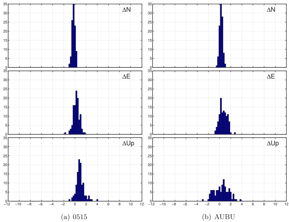
Abb. B-1: Histogramme der Differenz der Koordinatenzeitreihen ohne minus mit Einführung gestackter Information im Zeitraum DoY 131-240 2013 in topozentrischem Koordinatensystem; Rechtsachse: Differenz [mm], Hochachse [Anzahl], Balkenbreite 0.25 mm
