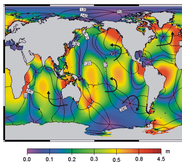
Abb. 2-1: Ozeangezeiten für die Komponente M_2 mit einer Periode von 12 h und 25 min; auftretende Amplitude farblich codiert, schwarze Linien: Phasenlage der Gezeiten; Quelle: http://holt.oso.chalmers.se/loading/loadingprimer.html , Stand: 10.07.2014
