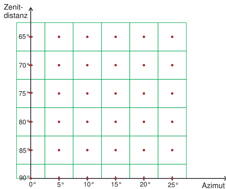
Abb. 6-1: Schema der Stacking-Zellen für einfache Stacking-Variante mit Zellengröße 5°×5° (Azimut × Elevation)
