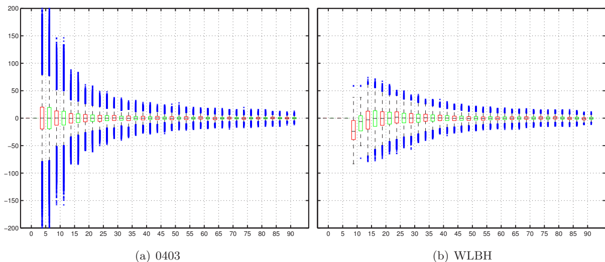
Abb. 6-18: Boxplot der Residuenwerte nach Elevationsbereichen; rot/grün Prozessierung ohne/mit Verwendung gestackter Information; blaue Kreuze: Ausreißer; Rechtsachse: Mittelpunkte der Elevationsbereiche [ ^\circ ]; Hochachse: Residuenwert [mm]
