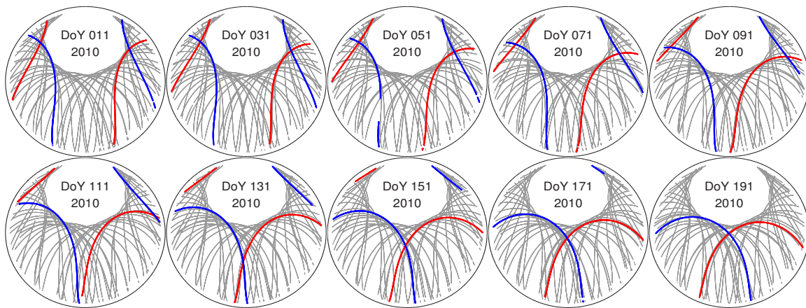
Abb. 8-11: Skyplots der Satellitenspuren der Station DOCO im Zeitraum DoY 011 bis 191 2010; rot: PRN24, blau: PRN26
