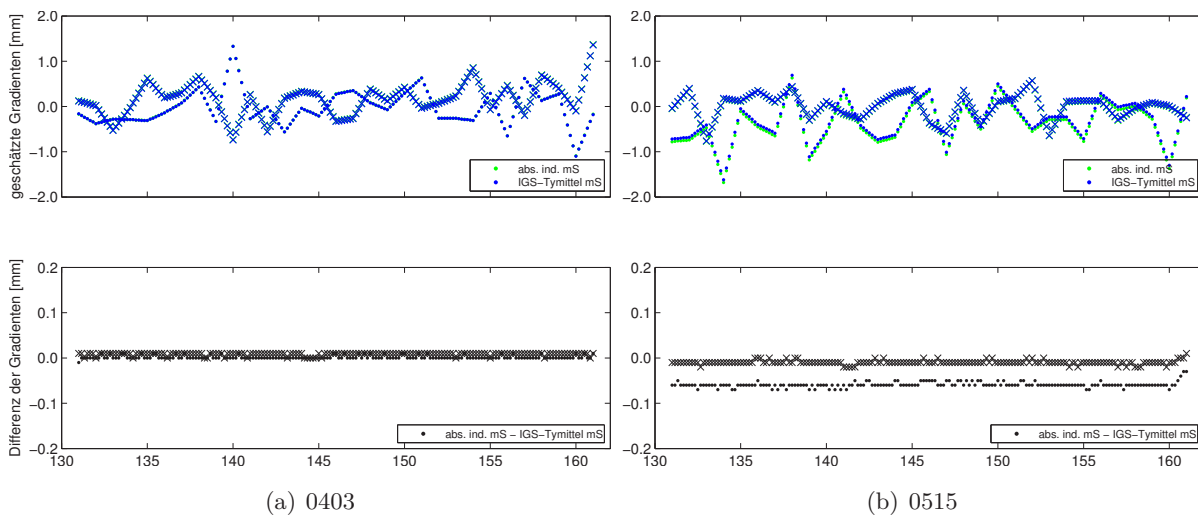
Abb. 7-7: Horizontale Gradienten der zenitalen troposphärischen Laufzeitverzögerungen für Zeitraum DoY 131 bis 160 2013; oben: Absolutwert für Varianten mit abs. ind. Kalibrierwerten und IGS-Typmittelwerten mit Einführung gestackter Information; unten: Differenz abs. ind. minus IGS-Typmittel; Punkt: Nordkomponente, Kreuz: Ostkomponente; nur jeder vierte Datenpunkt dargestellt
