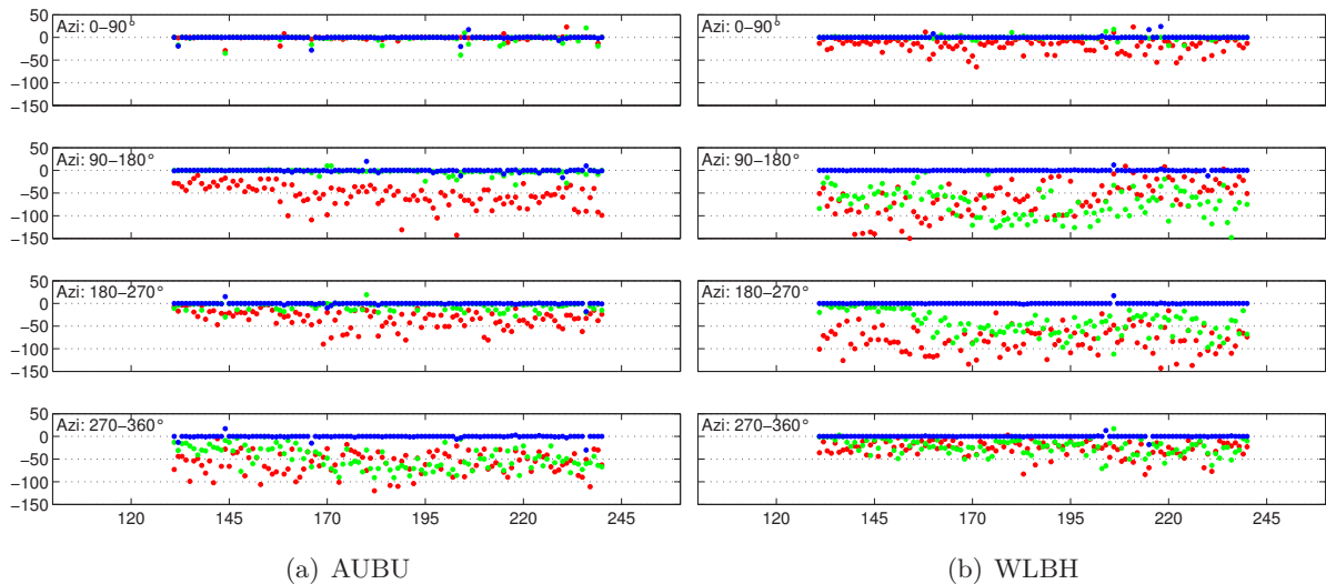
Abb. 6-14: Differenz der Residuenanzahl ohne minus mit Einführung gestackter Information im Zeitraum DoY 131-240 2013; Unterteilung in Azimutbereiche (Zeilen der Grafik) und Elevationsbereiche (farbliche Codierung) mit 0^{\circ} – 30^{\circ} (rot), 30^{\circ} – 60^{\circ} (grün), 60^{\circ} – 90^{\circ} (blau)
