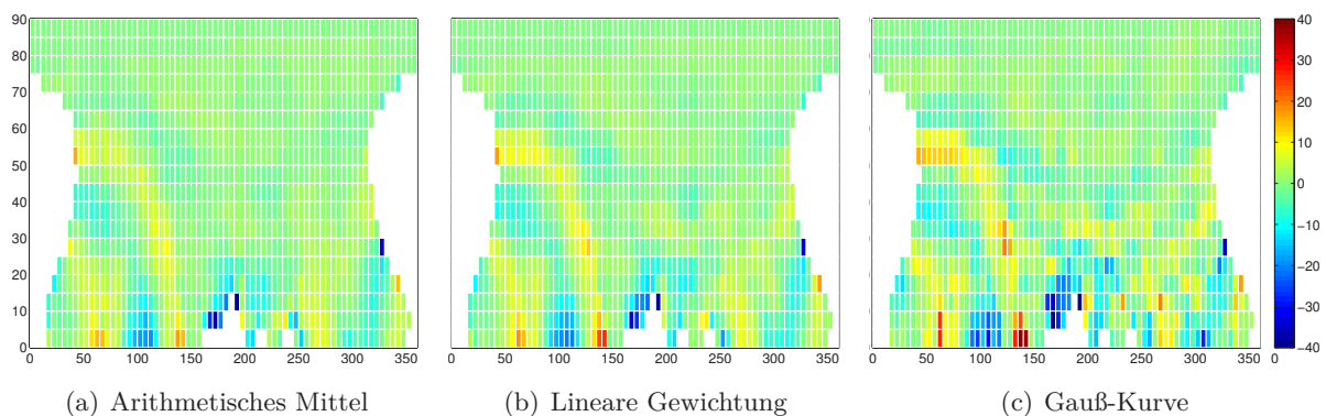
Abb. 8-9: Stackingmaps für Station 0515 im Zeitraum DoY 121 bis 130 2013 mit alternativer Zellfestlegung (topozentrischer Suchradius: 10^\circ ); Rasterabstand: 5^\circ \times 5^\circ (Azimut \times Elevation); Korrekturwert farblich codiert in [mm]; Rechtsachse: Azimut [ ^\circ ], Hochachse: Elevation [ ^\circ ]
