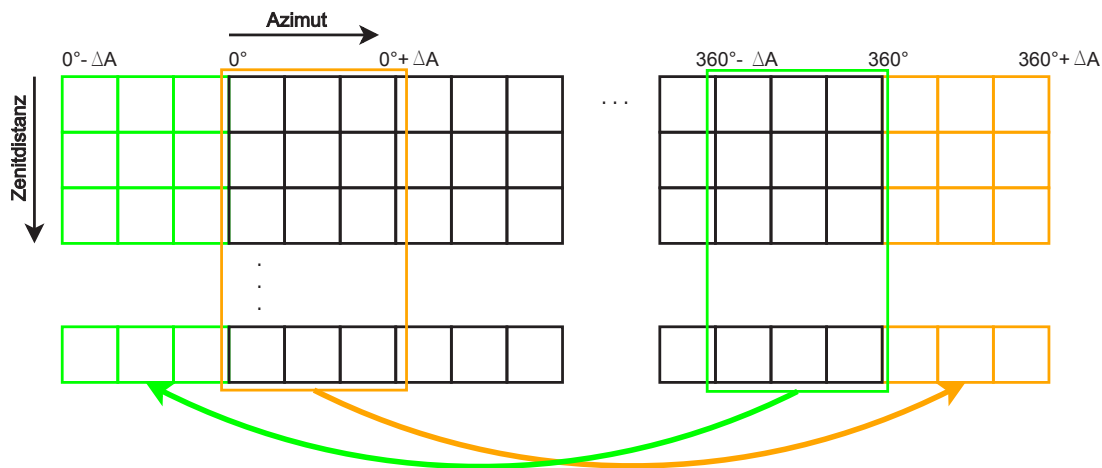
Abb. 4-8: Erweiterungsschema der Residuenmatrix
