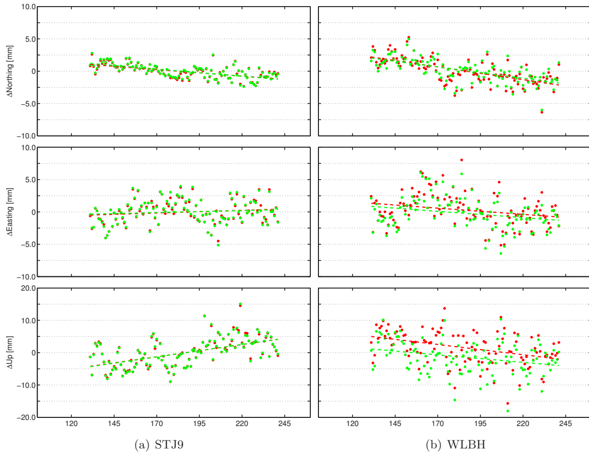
Abb. 6-20: Um den eurasischen Trend bereinigte Koordinatenzeitreihen ohne (rot) und mit (grün) Einführung gestackter Information, reduziert um den gemeinsamen Median der jeweiligen Koordinatenkomponente im Zeitraum DoY 131 bis 240 2013; gestrichelte Linien: geschätzte Regressionsgeraden; Rechtsachse: DoY 2013, Hochachse: Koordinatenkomponente [mm]
