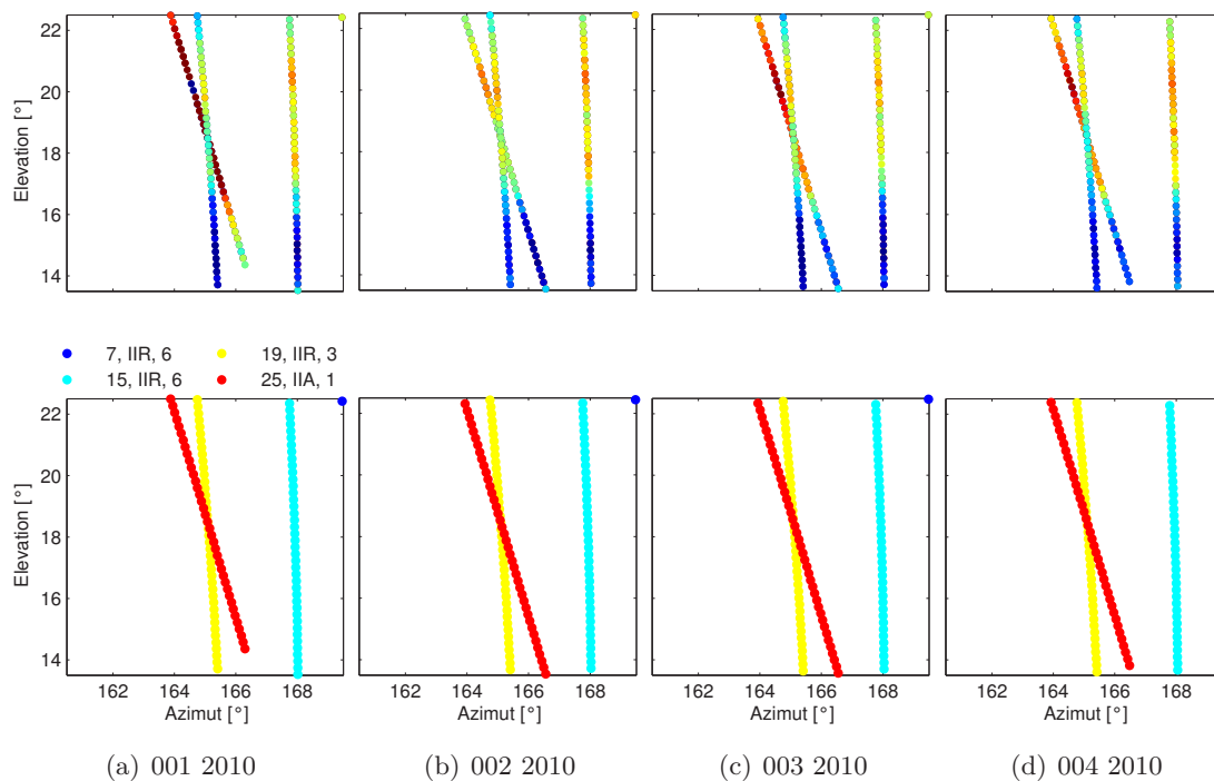
Abb. 8-10: Plots der Real-Residuen der Station DOCO für einen Ausschnitt der Antennenhemisphäre im Zeitraum DoY 001 bis 004 2010; oben: Residuenwert farblich codiert, unten: einzelne Satelliten mit PRN, Baureihe (Block) und Bahnebene
