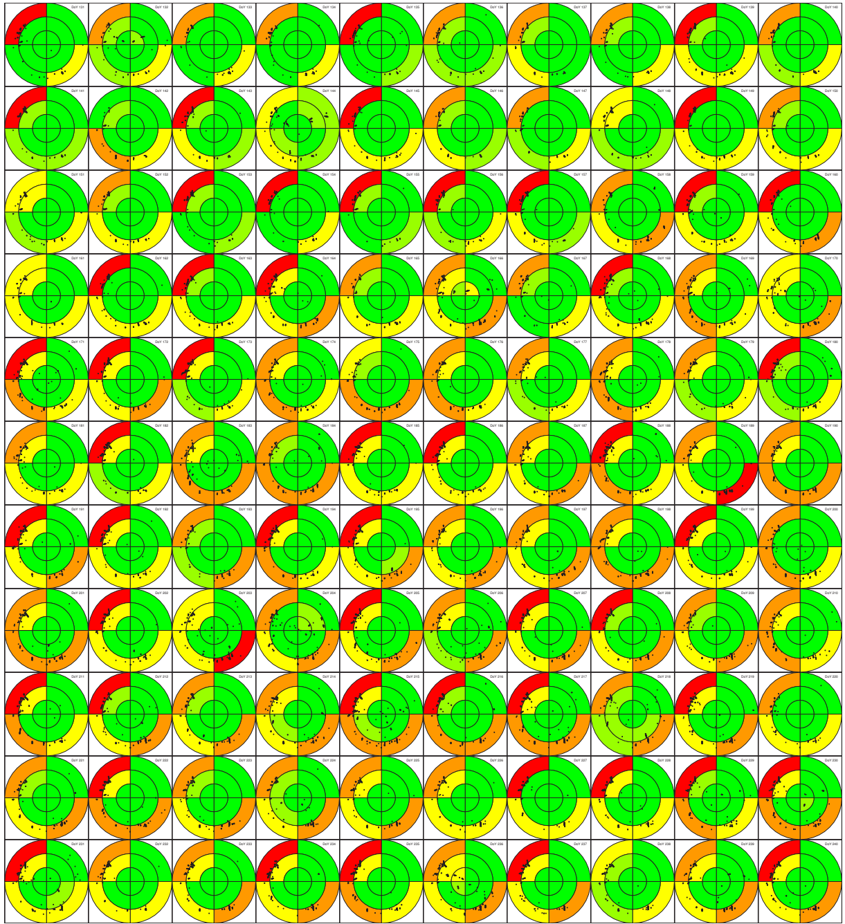
Abb. B-4: Station AUBU: nach Sektoren unterteilte Zunahme der Residuenanzahl nach Einführung gestackter Information gegenüber roher Prozessierung im Zeitraum DoY 131 bis 240 2013; grün/hellgrün/gelb/orange/rot: Zunahme um 0–1 %/1–2 %/2–5 %/5–10 %/>10 %; azimuthale Aufteilung: 0°–90°, 90°–180°, 180°–270° und 270°–360°; Elevationsstufen: 0°–30°, 30°–60° und 60°–90°; schwarze Punkte: durch Stacking in die Auswertung hinzugekommene Residuen
