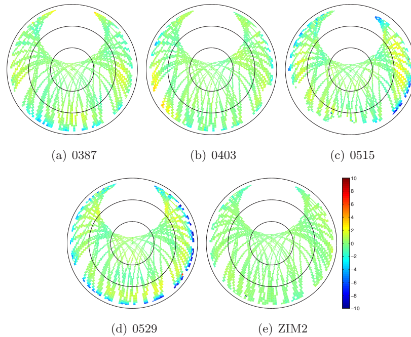
Abb. 7-3: Differenz der Stackingmaps der L_3 -Residuen: Prozessierung mit individuellen Kalibrierwerten minus Prozessierung mit IGS-Typmittelwerten (jeweils Absolutniveau); Stackingzeitraum: DoY 121-130 2013; Werte der Farbskala in [mm]; konzentrische Kreise (von innen nach aussen): Zenitdistanz 30°, 60°, 90°
