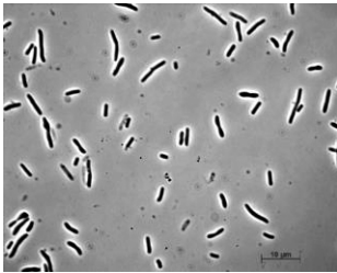
Abb. 2.3: Escherichia coli DSMZ 1103
