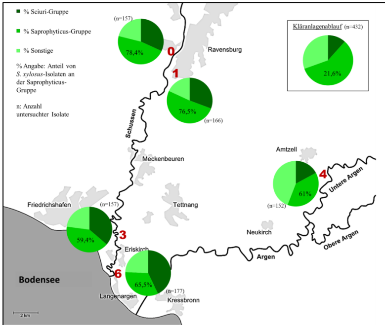
Abb. 8.2: Speziesverteilung der Staphylokokken entlang der Schussen sowie in der Argen und im Kläranlagenablauf
