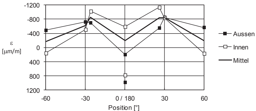
Abbildung 3.20: N6 SW768 T3 V3: Dehnungen in Längsrichtung, Laststufe 3, Probekörperhälfte 2
