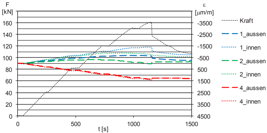
Abbildung 3.26: RUND 850 T3 V3: Dehnungen in Längsrichtung über die Zeit t, Probekörperhälfte 2
