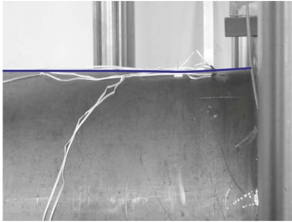
Abbildung 4.43: RUND 850 T3 V3: lokale Vorverformung nahe der Lasteinleitungsplatte
