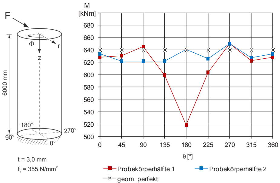
Abbildung 4.41: Berechnungsmodell, Traglast M in Abhängigkeit der Belastungsrichtung \theta
