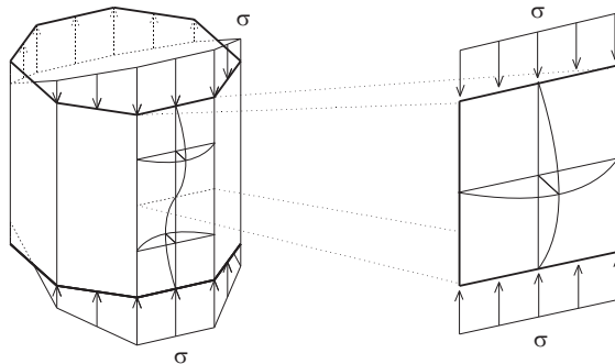
Abbildung 2.1: Tragwerksidealisierung druckbeanspruchter polygonaler Querschnitte
