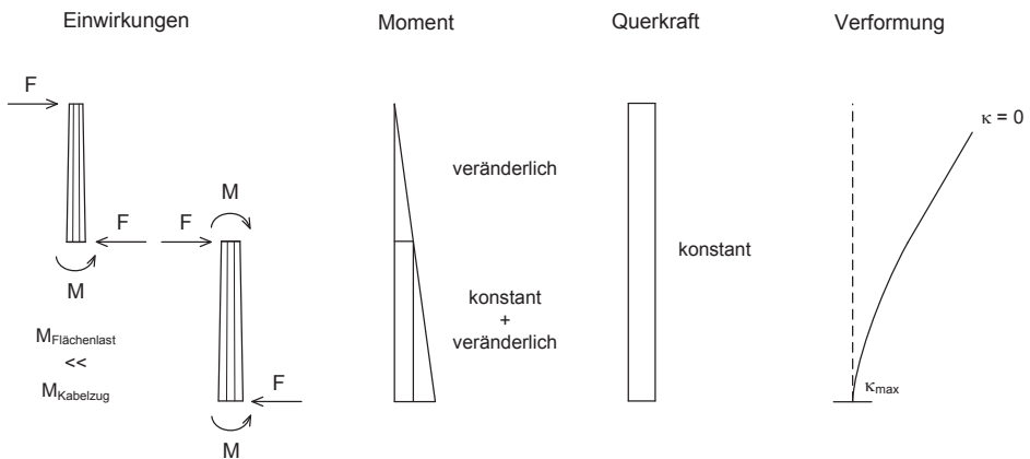
Abbildung 4.10: Segmentbeanspruchungen
