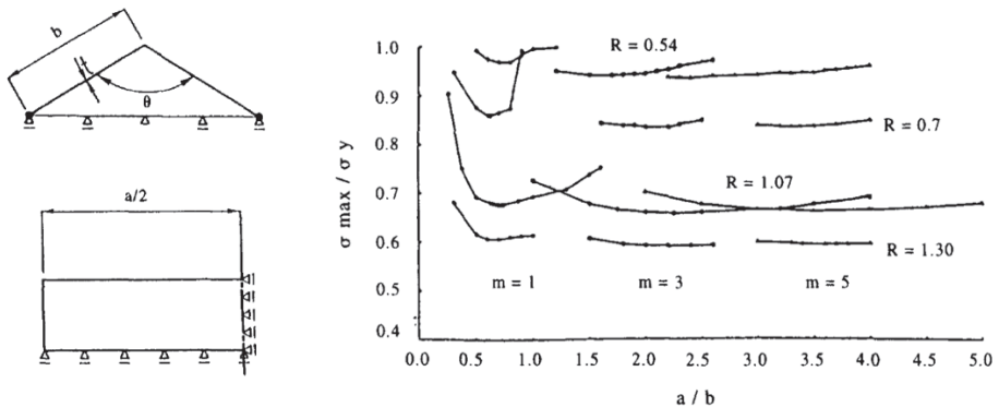
Abbildung 2.29: Berechnungsmodell mit zwei Flächen; Gemittelte Beulspannung bei verschiedenen Seitenverhältnissen a/b , Plattenschlankheiten R und Halbwellen m in Längsrichtung [62]
