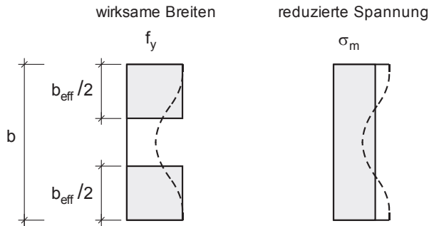
Abbildung 2.7: Methoden zur Berücksichtigung der nichtlinearen Spannungsverteilung
