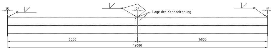
Abbildung A1: Abmessungen N6_SW768_T3
