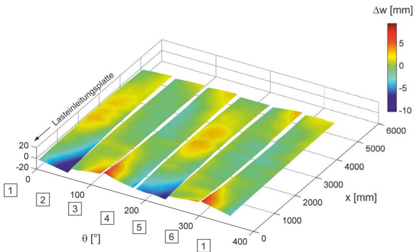
Abbildung 3.9: N6 SW768 T3 V3 Probekörperhälfte 2: \Delta w bez. auf best-fit Polygon
