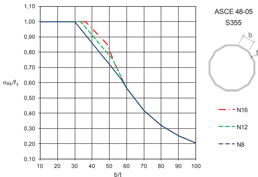
Abbildung 2.18: zulässige bezogene Spannungen \sigma_{Rk}/f_y für biegebeanspruchte, polygonale Querschnitte mit 8, 12 und 16 Kanten nach [4]
