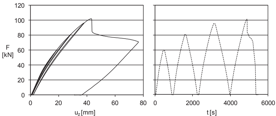
Abbildung 3.19: N6 SW768 T3 V3: links: Kraft-Verformungs-Diagramm, rechts: Last-Zeit-Verlauf
