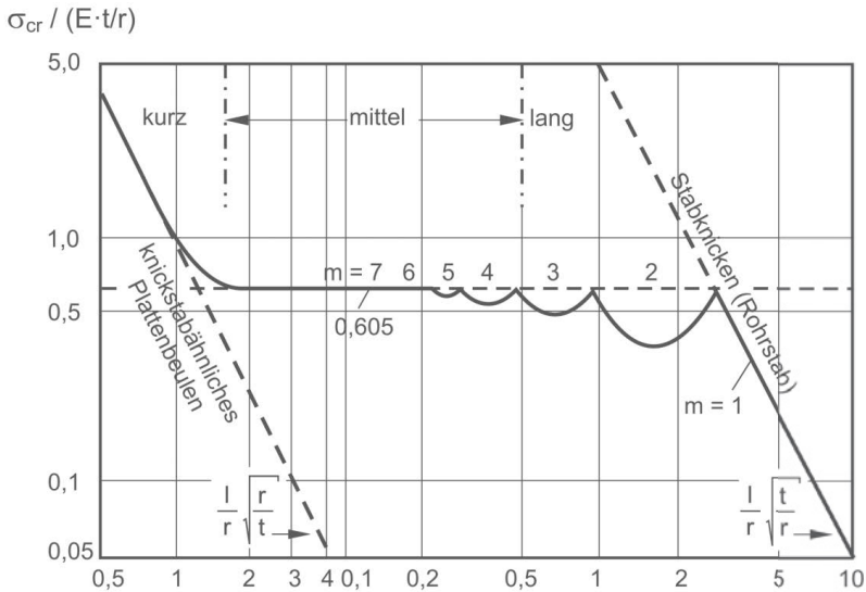
Abbildung 2.12: kritische Axialbeulspannung nach Flügge [57]
