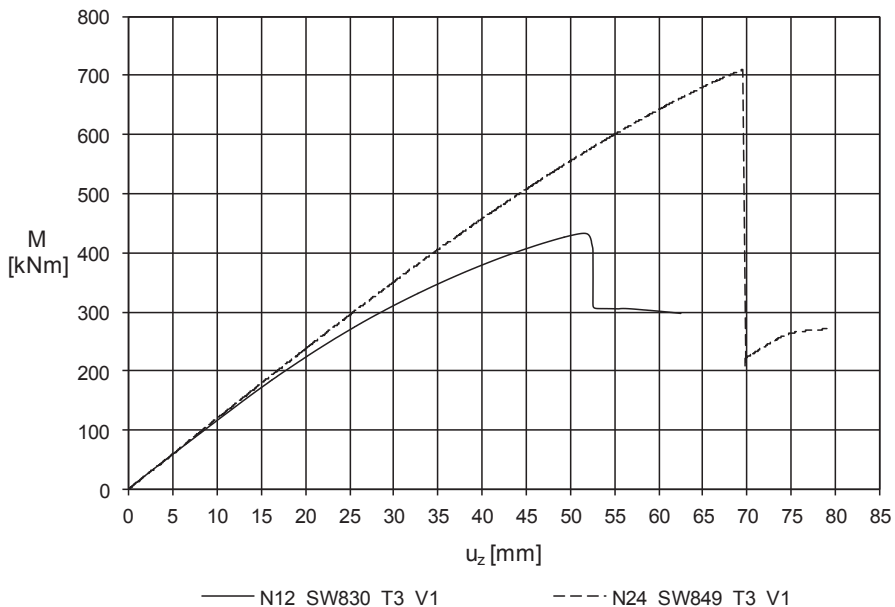
Abbildung 3.29: Last-Verformungsverläufe N12 SW830 T3 V1 u. N24 SW849 T3 V1
