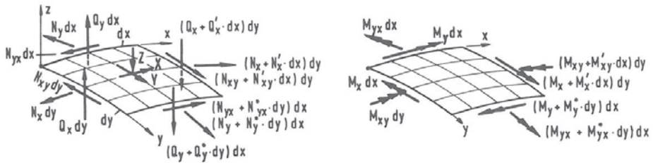
Abbildung 2.3: infinitesimales Mittelflächenelement mit Schnittgrößen und deren Zuwächsen aus [66]
