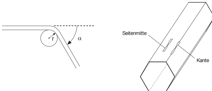
Abbildung 4.35: links: Schwenkbiegen, Kantwinkel \alpha , rechts: Lage der Materialproben
