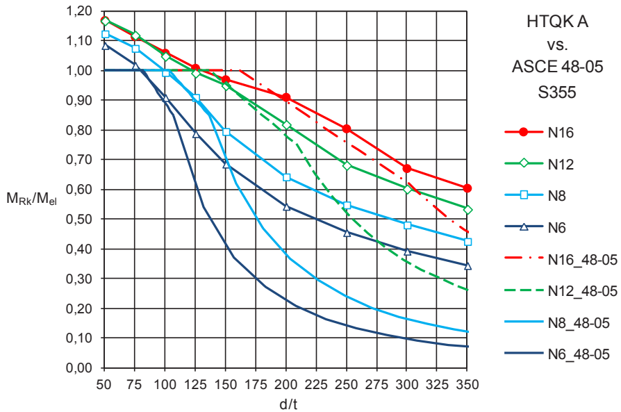
Abbildung 5.17: polygonale Querschnitte: HTQK A vs. ASCE 48-05 [4]
