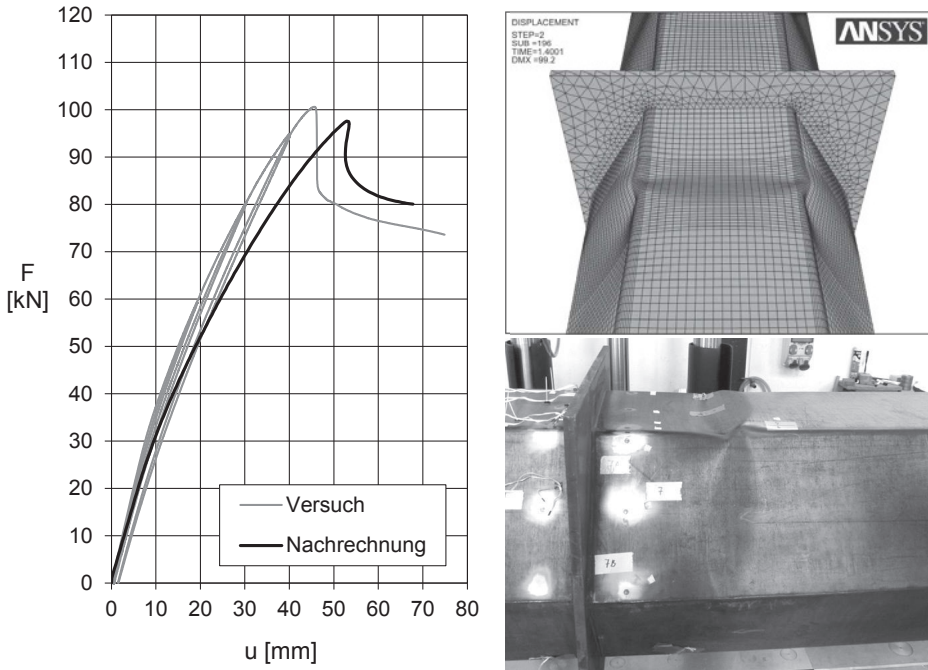
Abbildung 4.5: Berechnungsergebnisse Nachrechnung N6_SW768_T3 Versuch 3, links: Last-Verformungskurven Versuch und Nachrechnung, rechts: Nachbeulformen Nachrechnung (ohne Überhöhung) und Versuch
