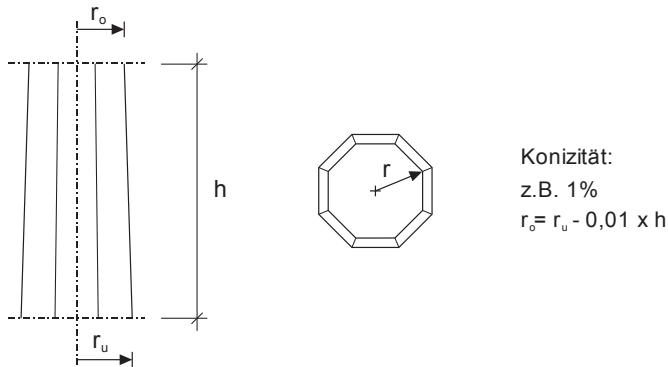
Abbildung 4.27: Konizität
