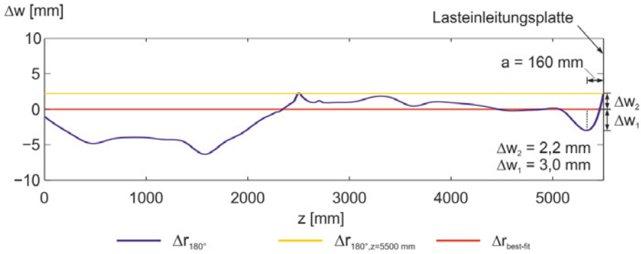
Abbildung 4.46: Bezugsradien zur Bestimmung der Eindringtiefe
