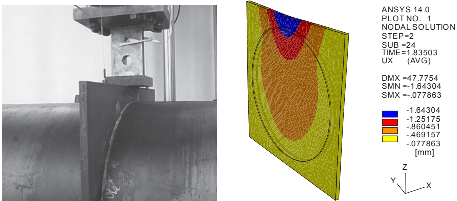
Abbildung 4.8: links: Detail Lasteinleitung, rechts: Lasteinleitungsplatte Nachrechnung RUND bei Erreichen der Traglast
