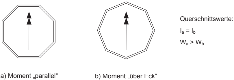
Abbildung 4.13: Belastungsrichtungen
