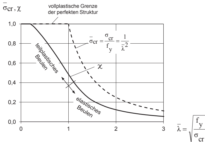
Abbildung 2.9: Beulabminderungsfaktor \chi in Abhängigkeit der bezogenen Schlankheit \bar{\lambda}
