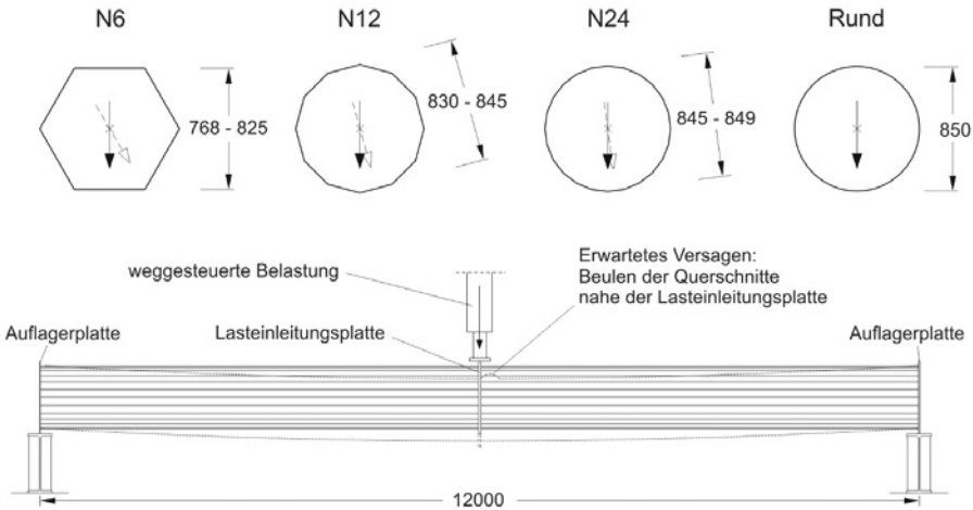
Abbildung 3.1: Probekörpergeometrie und Versuchsaufbau
