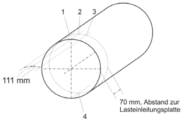
Abbildung 3.24: RUND 850 T3 V3: Messstellen
