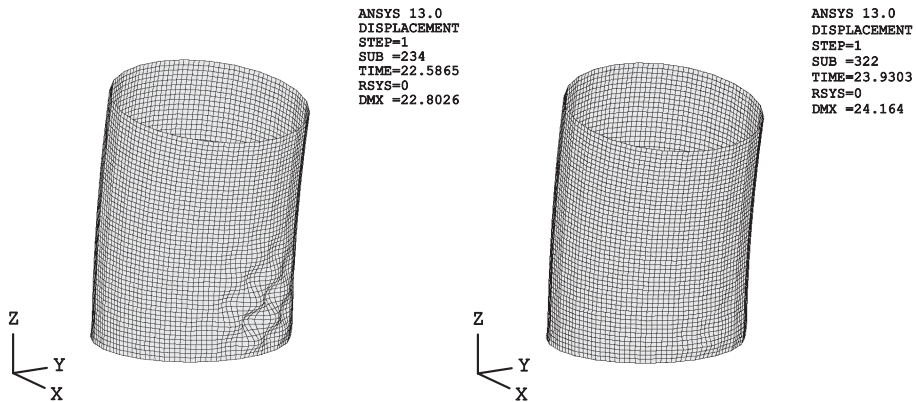
Abbildung 4.17: Vorbeulformen N24 d/t = 400 , links: Moment parallel / Einzelbeulen zwischen den Kanten, rechts: Moment ü. Eck / Vorbeulform des biegebeanspruchten Kreiszyinders, (unterer Mastabschnitt, Verformungen 50-fach überhöht dargestellt)
