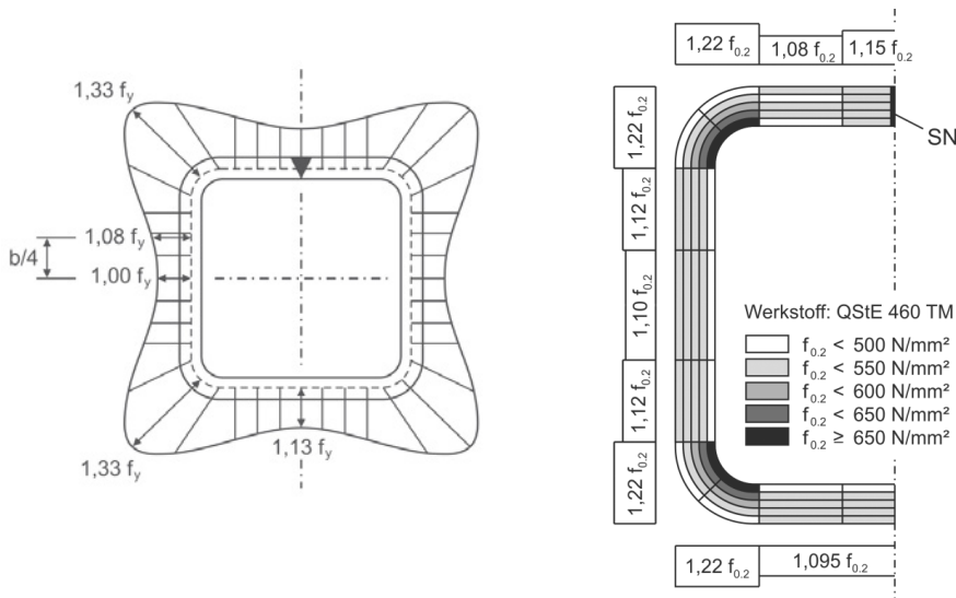
Abbildung 4.36: gemessene Streckgrenzenverteilung an einem kaltgefertigten Quadrat-hohlprofil links aus [84], rechts aus [35]
