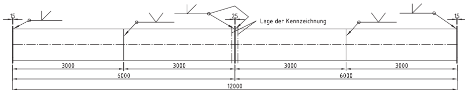
Abbildung A7: Abmessungen RUND_D850_T3
