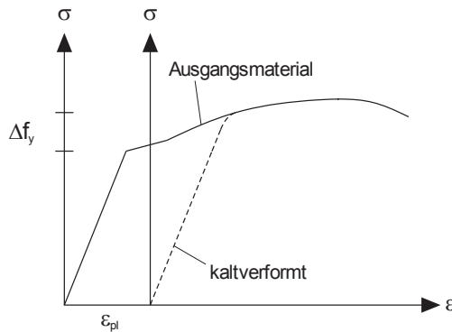
Abbildung 4.34: Spannungs-Dehnungslinie des Ausgangsmaterial bzw. nach Kaltverformung
