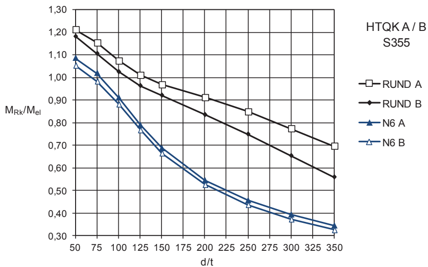
Abbildung 5.10: bezogene Biegetragfähigkeit M_{Rk}/M_{el} : N6 u. RUND, HTQK A u. B, d/t = 50 - 350
