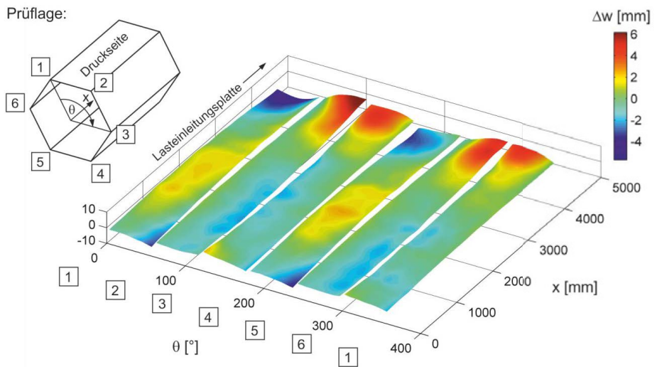
Abbildung 3.8: N6 SW768 T3 V3 Probekörperhälfte 1: \Delta w bez. auf best-fit Polygon
