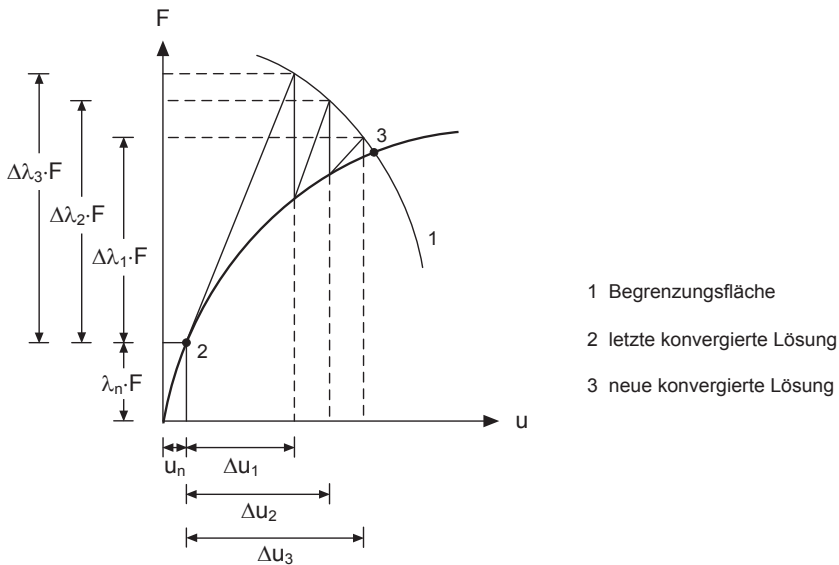
Abbildung 2.21: das Bogenlängenverfahren für einen Lastschritt [60]
