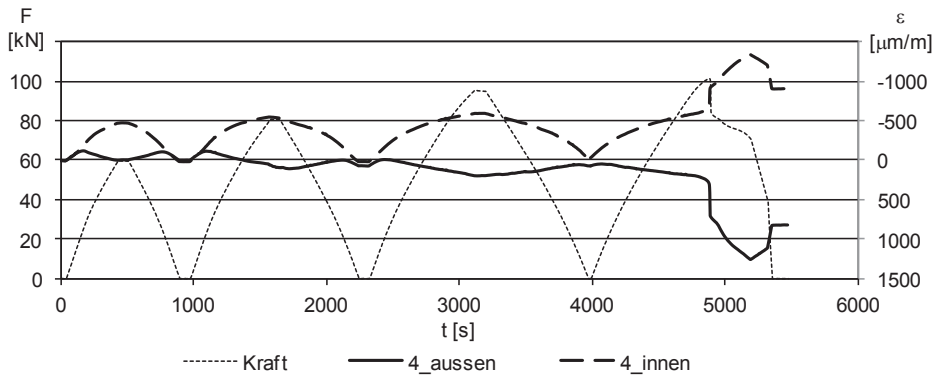
Abbildung 3.22: N6 SW768 T3 V3: Dehnungen in Längsrichtung über die Zeit t , Messstelle Nr. 4, Probekörperhälfte 2
