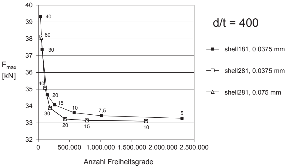
Abbildung 4.3: Konvergenzstudien: Variation der Elementtypen und Lastschrittweiten, oben: Schlankheit d/t 200, unten Schlankheit d/t = 400, Angaben im Diagramm: Elementgrößen in mm
