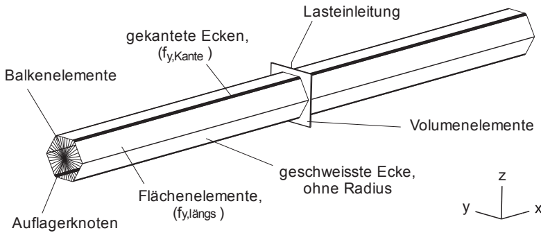
Abbildung 4.4: Übersicht Berechnungsmodell N6
