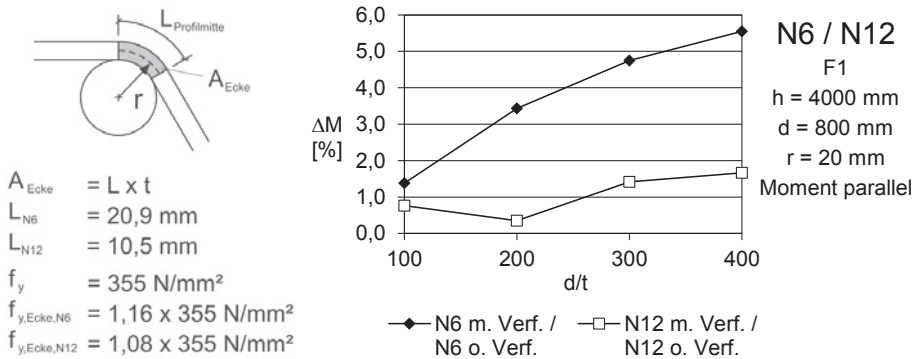
Abbildung 4.37: Einfluss der Kaltverfestigung infolge des Kantens auf die Biegetragfähigkeit polygonaler Querschnitte am Beispiel N6 und N12 (Biegung parallel)
