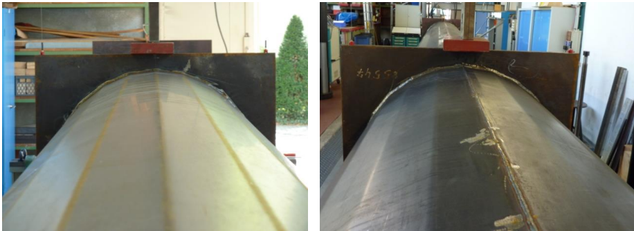
Abbildung 5.13: links: N24 SW849 T3 V1, ohne Schweißnaht im Druckbereich; rechts: N24 SW849 T3 V2: Schweißnaht an der am höchsten druckbeanspruchten Kante
