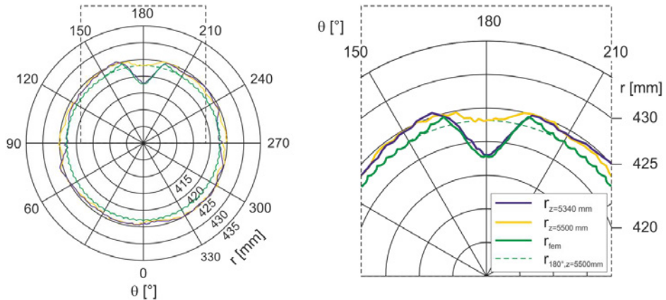
Abbildung 4.49: Querschnitt durch die gemessene Vorbeule und die berechnete Vorbeule ( z = 5340 mm), Querschnitt am Mastfuß ( z = 5500 mm)
