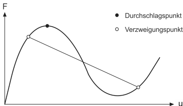
Abbildung 2.22: Durchschlags- und Verzweigungspunkte eines Last-Verformungspfades
