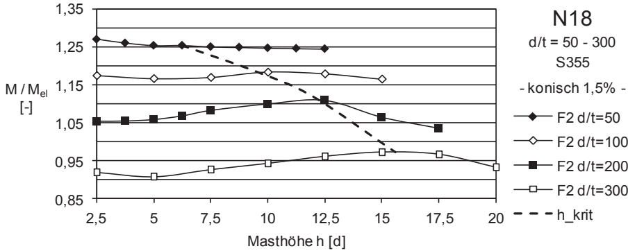
Abbildung 4.30: N18: Biegetragfähigkeit (Masttyp F2) in Abhängigkeit der Masthöhe für verschiedene Bauteilschlankheiten d/t , Konizität r = 1,5\%
