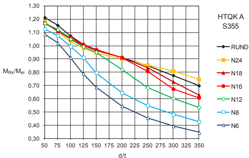
Abbildung 5.9: bezogene Biegetragfähigkeit M_{Rk}/M_{el} : N6 – RUND, HTQK A, d/t = 50 - 350
