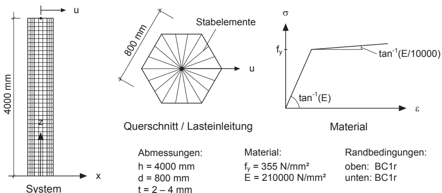
Abbildung 4.1: FE-Modell für Parameterstudien
