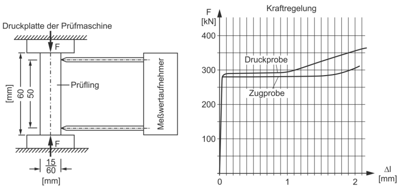
Abbildung 4.33: links: Druckversuch Aufbau und Abmessungen Materialprobe, rechts: Gegenüberstellung der Ergebnisse aus Zug- und Druckversuch aus [65]
