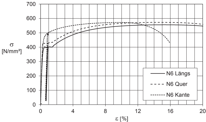
Abbildung 3.4: Zugproben in Längs- und Querrichtung sowie aus dem Kantenbereich des Materials des Probekörper N6 SW768 T3 V1
