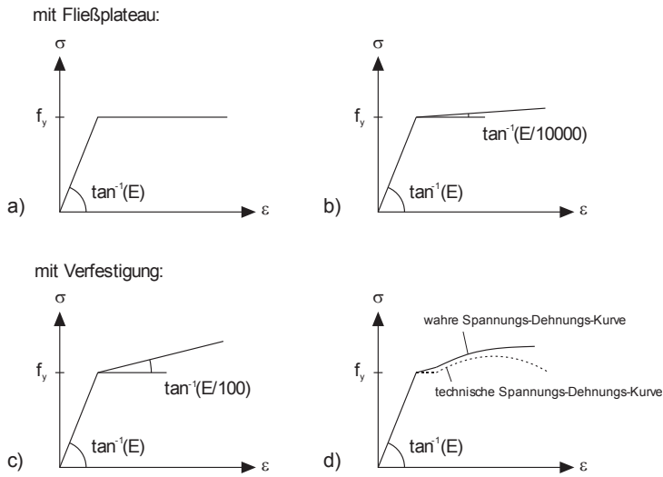
Abbildung 4.32: Modellierung des Werkstoffverhaltens aus [23]
