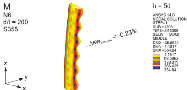
Abbildung 4.23: Vorbeulform des Masttyp M im GZT
