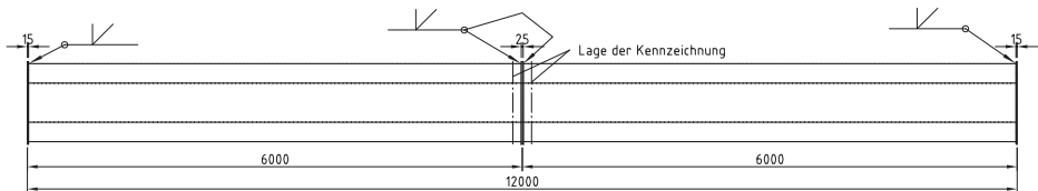
Abbildung A2: Abmessungen N6_SW825_T3
