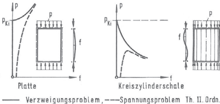
Abbildung 2.2: Stabilitätsfälle Platte und Kreiszyinderschale aus [66]
