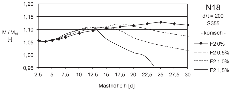
Abbildung 4.29: N18: Biegetragfähigkeit (Masttyp F2) in Abhängigkeit der Masthöhe für verschiedene Konizitäten
