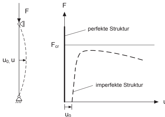
Abbildung 2.23: Minimalbeispiel druckbeanspruchte Pendelstütze
