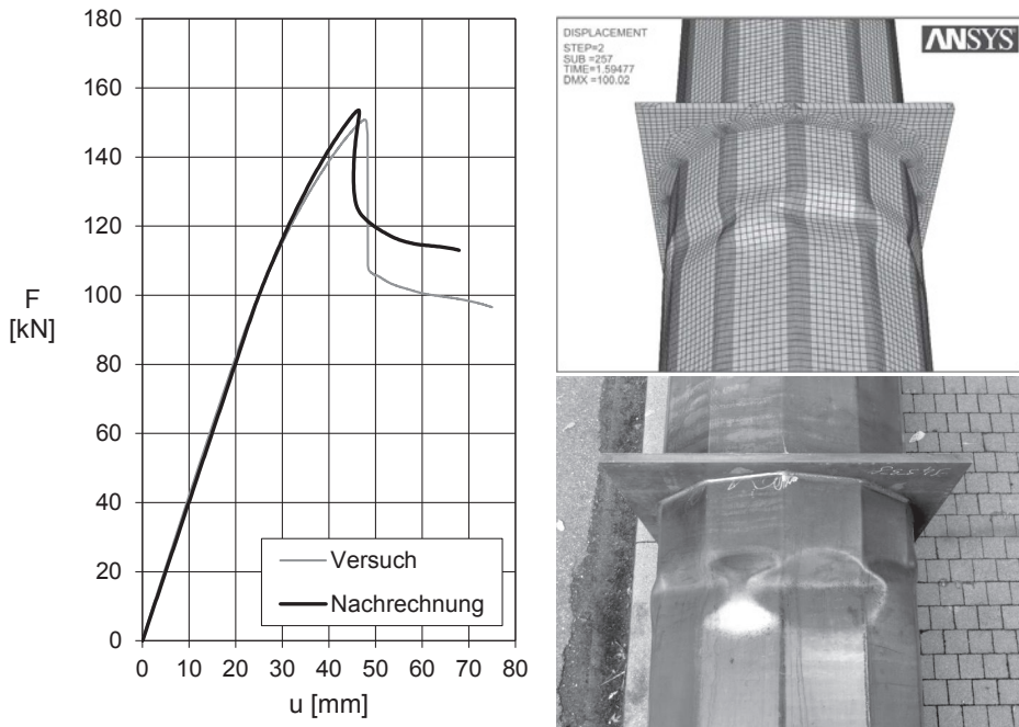
Abbildung 4.6: Berechnungsergebnisse Nachrechnung N12_SW845_T3 Versuch 3, links: Last-Verformungskurven Versuch und Nachrechnung, rechts: Nachbeulformen Nachrechnung (ohne Überhöhung) und Versuch
