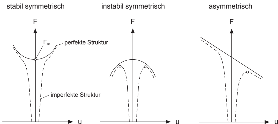
Abbildung 2.24: Klassifizierung der Verzweigungsarten nach Koiter
