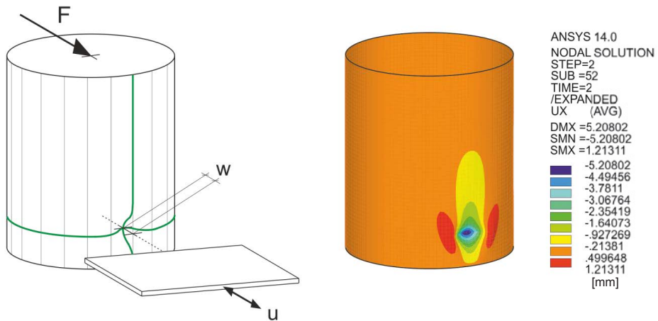
Abbildung 4.45: Simulation der Entstehung einer Vorverformung: Anprall
