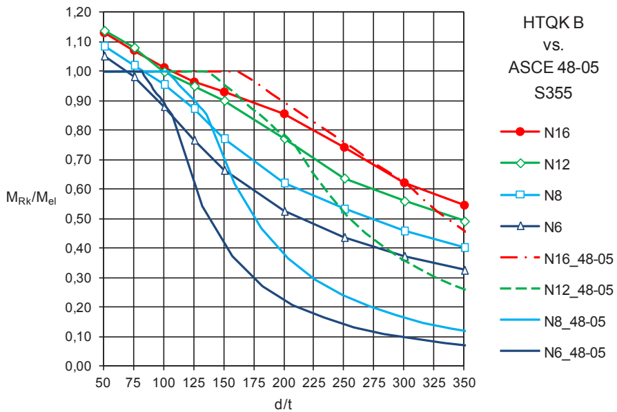
Abbildung 5.18: polygonale Querschnitte: HTQK B vs. ASCE 48-05 [4]
