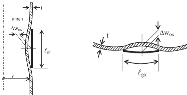
Abbildung 2.14: Messung von Vorbeultiefen (Amplituden) aus [25]
