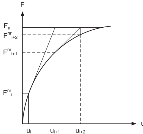
Abbildung 2.20: Gleichgewichtsiterationen des Newton-Raphson-Verfahrens [2]
