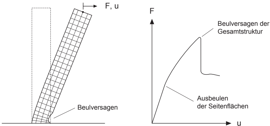
Abbildung 2.25: Berechnungsmodell, typischer Last-Verformungsverlauf eines polygonalen Querschnitts mit 12 Kanten
