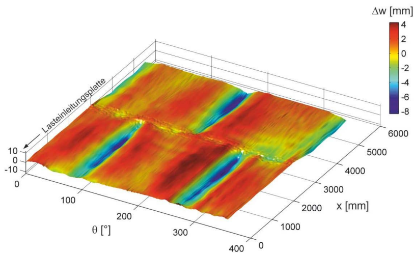
Abbildung 3.15: RUND 850 T3 V3 Probekörperhälfte 2: \Delta w bez. auf best-fit Zylinder
