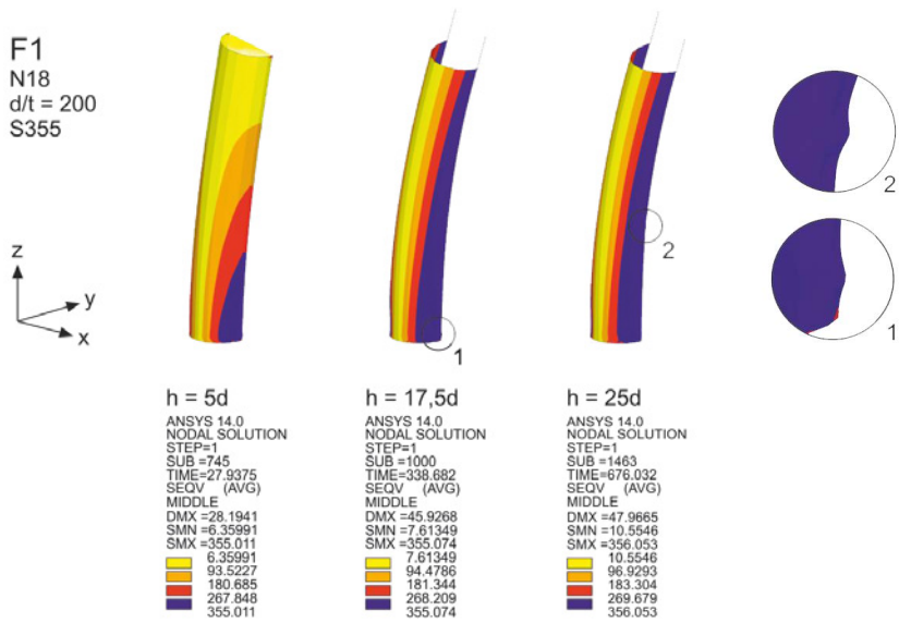
Abbildung 4.25: Vorbeulformen des Masttyps F1 im GZT: h = 4 m, 14 m und 20 m (Darstellung der ersten 4 m oberhalb des Mastfußes, halbes System, Verformungen 20-fach überhöht) und Vergleichsspannungen in Elementmitte
