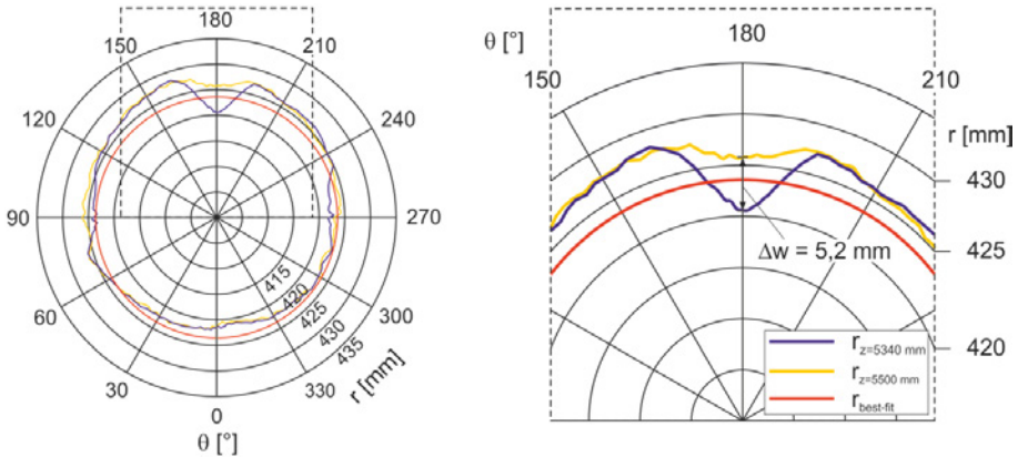
Abbildung 4.47: Querschnitt durch die Vorbeule ( z = 5340 \text{ mm} ) und Querschnitt am Mastfuß ( z = 5500 \text{ mm} ), r_{\text{best-fit}} , Probekörperhälfte 1
