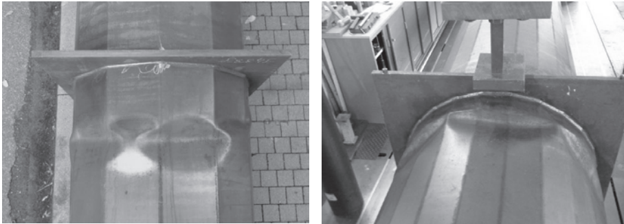
Abbildung 1.3: Probekörper nach Erreichen der Traglast, links: eine Beule je Seitenfläche, rechts: Beulen über mehrere Kanten hinweg
