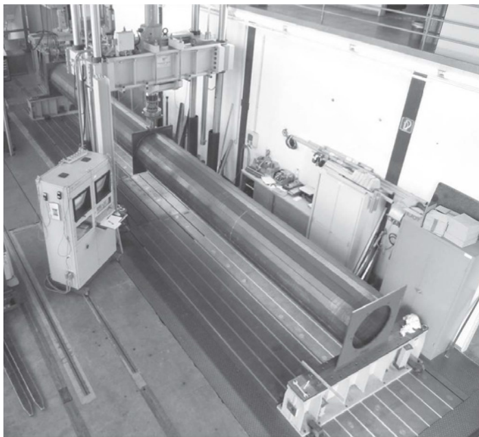
Abbildung 3.2: Versuchsaufbau, Probekörper N24 SW845 T3 V1
