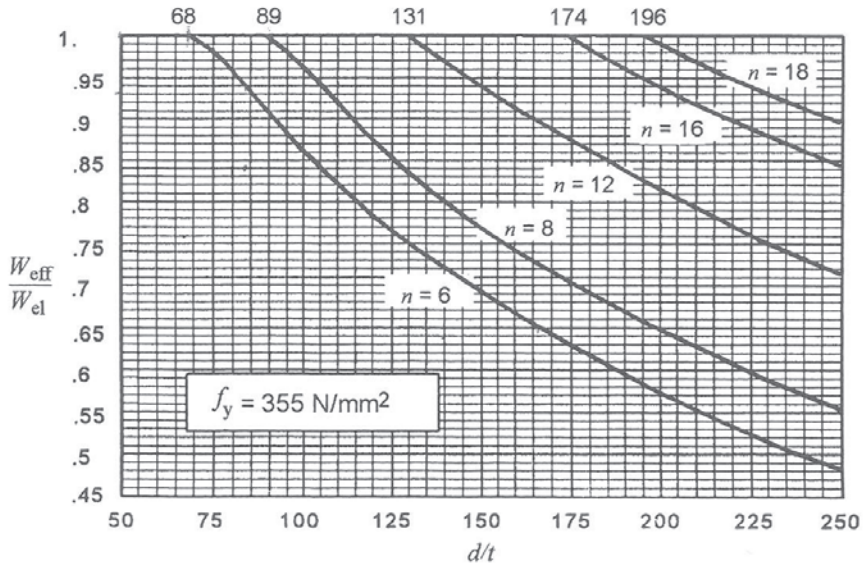
Abbildung 2.17: wirksames Widerstandsmoment W_{\text{eff}} für polygonale Querschnitte nach [27]
