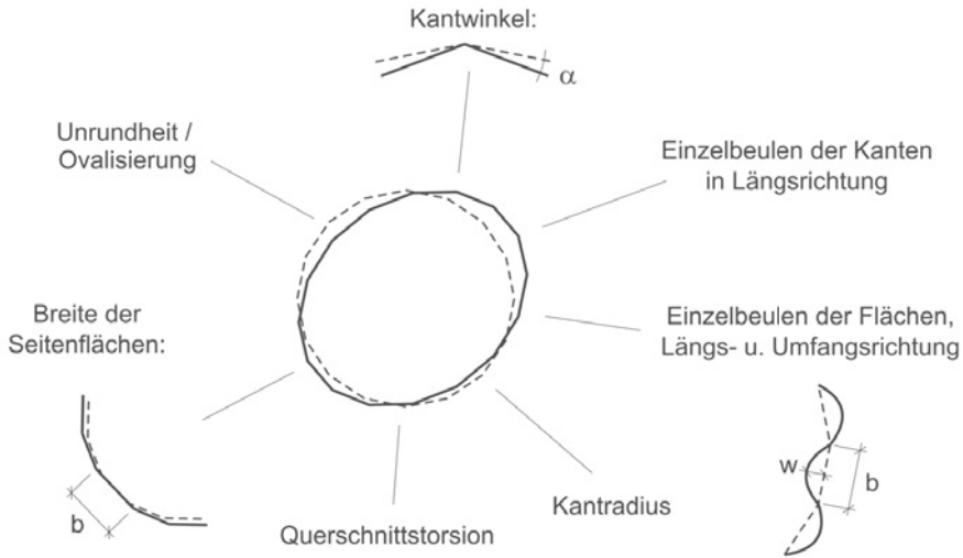
Abbildung 2.15: mögliche Vorverformungen polygonaler Querschnitte
