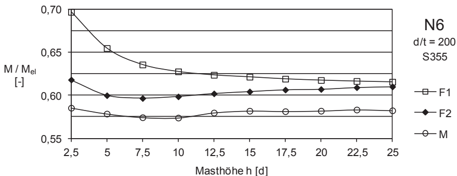
Abbildung 4.21: Biegetragfähigkeit M in Abhängigkeit der Masthöhe h (N6, d/t = 200 ) für die Masttypen F1, F2 und M
