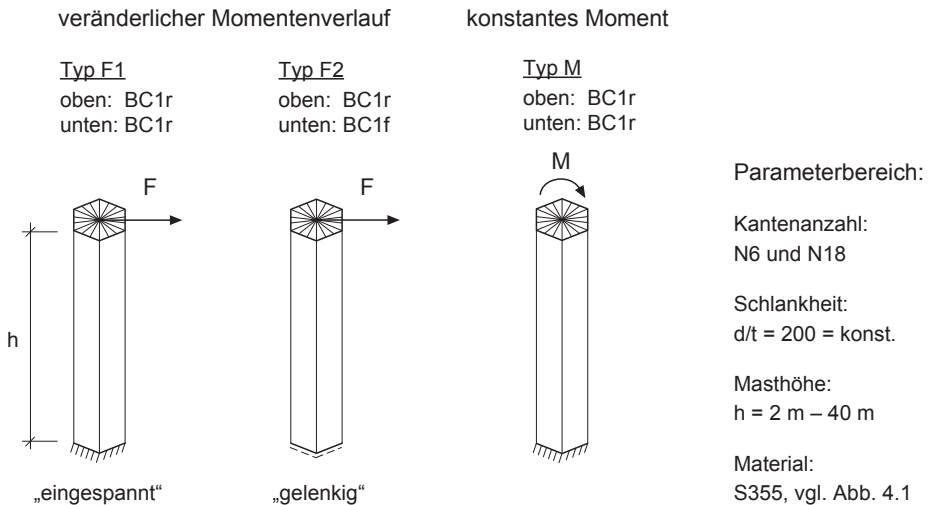
Abbildung 4.20: Berechnungsmodelle für die Untersuchungen zum Einfluss der Masthöhe
