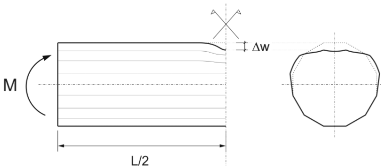
Abbildung 5.1: numerisches Berechnungsmodell
