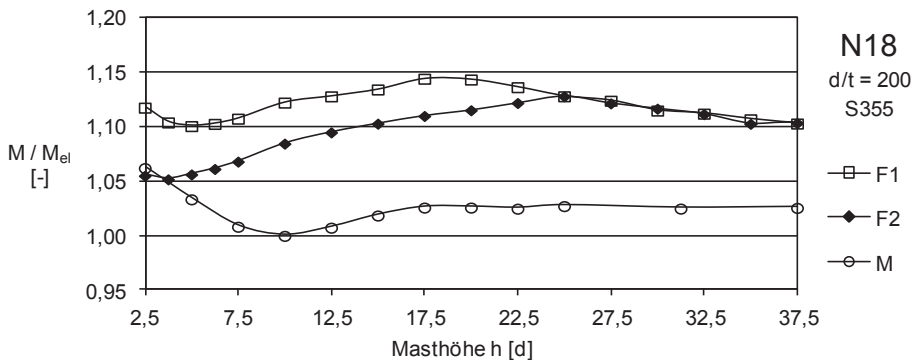
Abbildung 4.24: Biegetragfähigkeit M in Abhängigkeit der Masthöhe h (N18, d/t = 200 ) für die Masttypen F1, F2 und M
