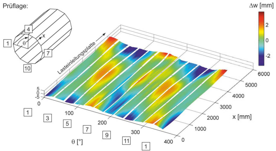
Abbildung 3.11: N12 SW845 T3 V3 Probekörperhälfte 1: \Delta w bez. auf best-fit Polygon
