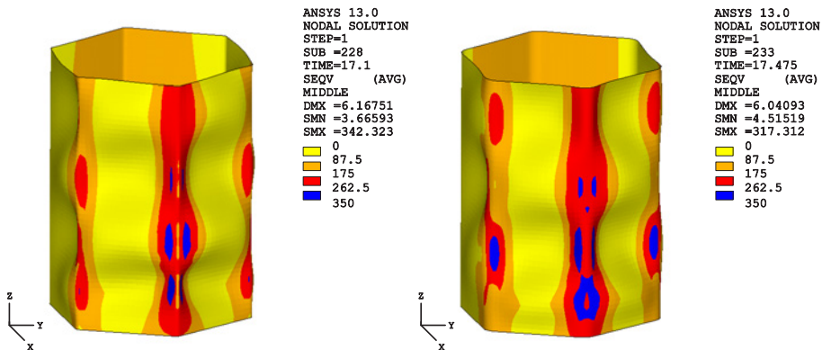
Abbildung 4.19: Vergleichspannungsverteilung in Elementmitte und Vorbeulformen bei verschiedenen Biegerollenradien, links: r = 20 mm, rechts: r = 60 mm (unterer Mastabschnitt, Polygon N6, d/t = 400 , Moment ü. Eck)
