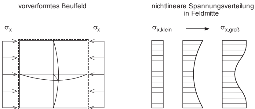
Abbildung 2.6: Entwicklung der Spannungsverteilung einer durchbeanspruchten, vorverformten Platte
