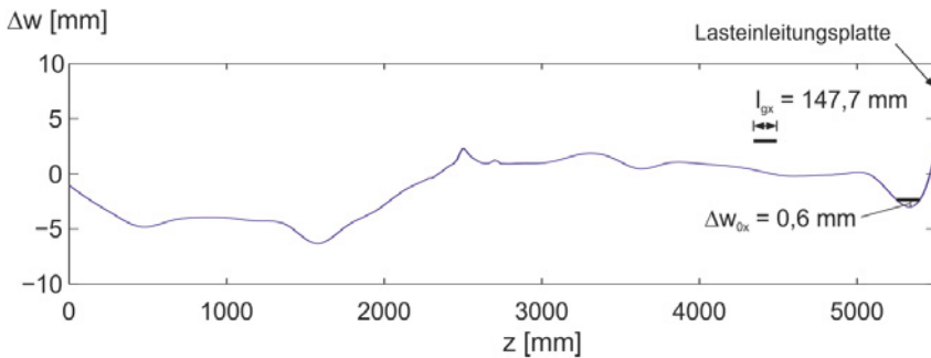
Abbildung 3.16: RUND 850 T3 V3 Probekörperhälfte 1: Längsschnitt \theta=180^\circ
