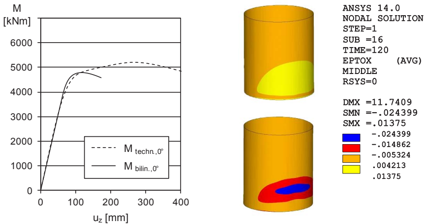
Abbildung 4.39: links: Last-Verformungskurven für d/t = 50 , Druckbeanspruchung bei 0^\circ , rechts: Dehnungen \epsilon_{x,min/max} in Elementmitte im GZT für M_{bilin,0^\circ}
