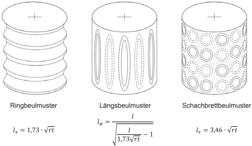
Abbildung 2.11: Beulmuster eines mittellangen Kreiszyinders unter Axialdruck nach [57]
