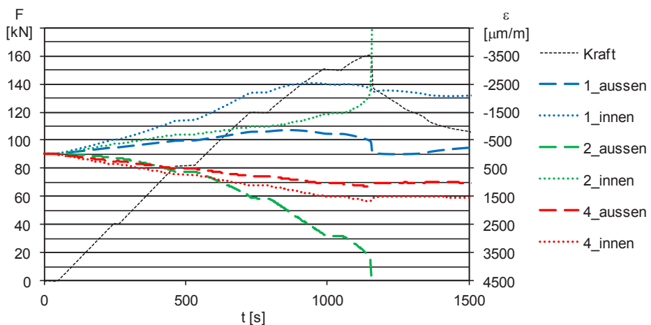
Abbildung 3.25: RUND 850 T3 V3: Dehnungen in Längsrichtung über die Zeit t , Probekörperhälfte 1
