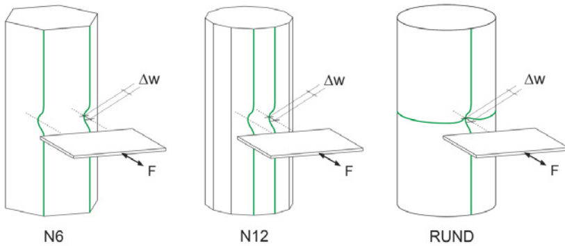
Abbildung 5.4: Übertrag des Imperfektionsansatzes „Anprall“ auf polygonale Querschnitte
