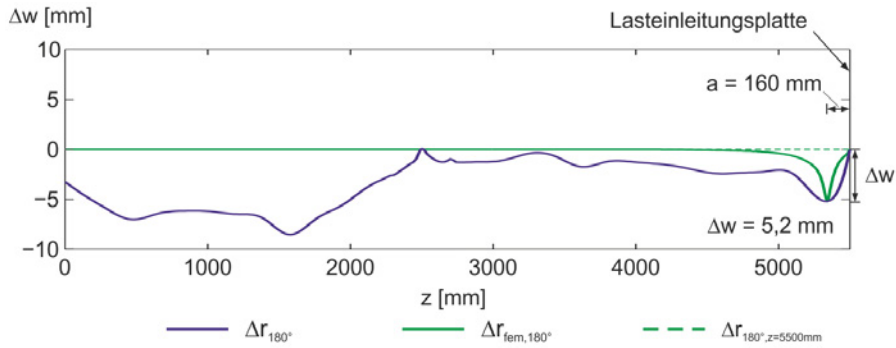
Abbildung 4.48: Längsschnitt durch den 180°-Meridian: Messdaten und berechnete Vorverformung
