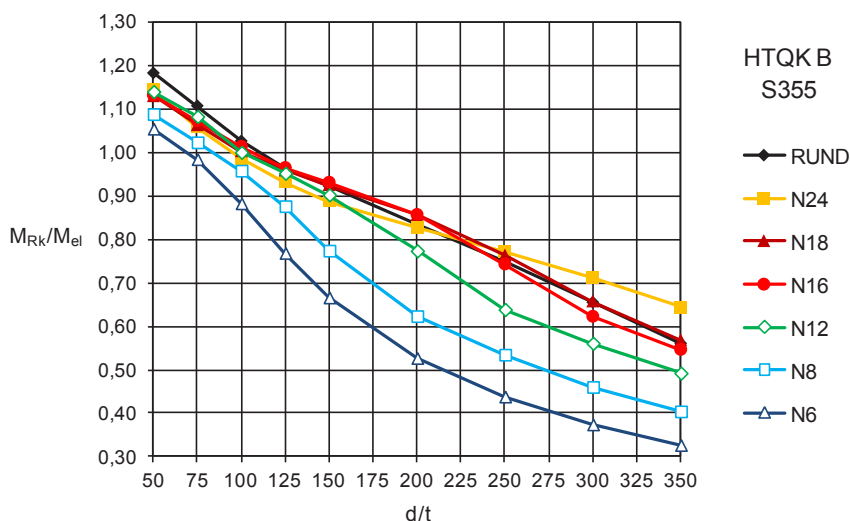
Abbildung 5.7: bezogene Biegetragfähigkeit M_{Rk}/M_{el} : N6 – RUND, HTQK B, d/t = 50 - 350
