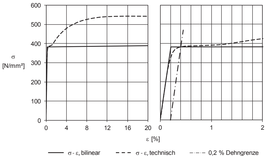
Abbildung 4.38: bilineares Werkstoffmodell und technische Spannungs-Dehnung-Linie
