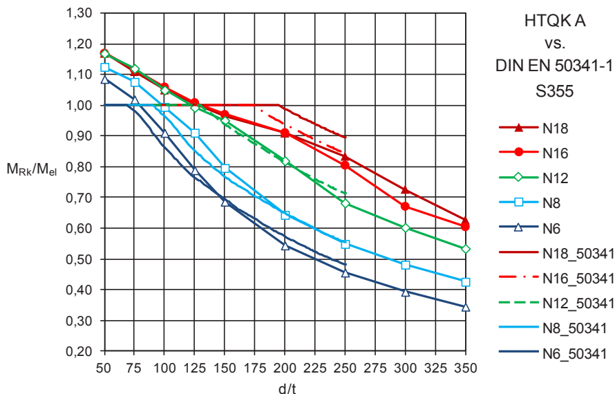
Abbildung 5.15: polygonale Querschnitte: HTQK A vs. DIN EN 50341-1 [27]
