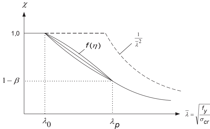
Abbildung 2.13: allgemeine Funktion für den Beulabminderungsfaktor \chi [69]
