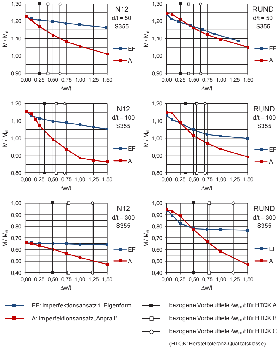
Abbildung 5.6: Vergleich der Imperfektionsansätze Eigenform und Anprall: bezogene Biegetragfähigkeiten in Abhängigkeit von \Delta w/t
