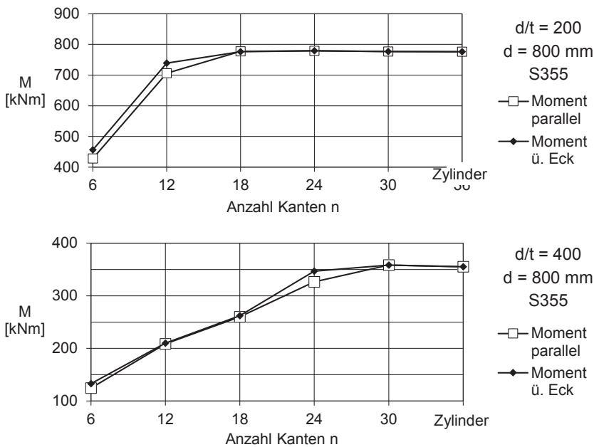
Abbildung 4.16: Traglast für verschiedene Kantenanzahlen in Abhängigkeit der Belastungsrichtung
