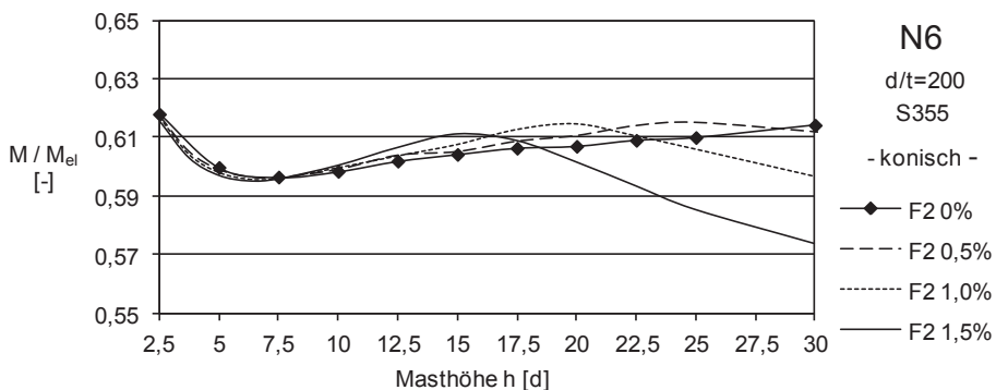
Abbildung 4.28: N6: Biegetragfähigkeit (Masttyp F2) in Abhängigkeit der Masthöhe für verschiedene Konizitäten
