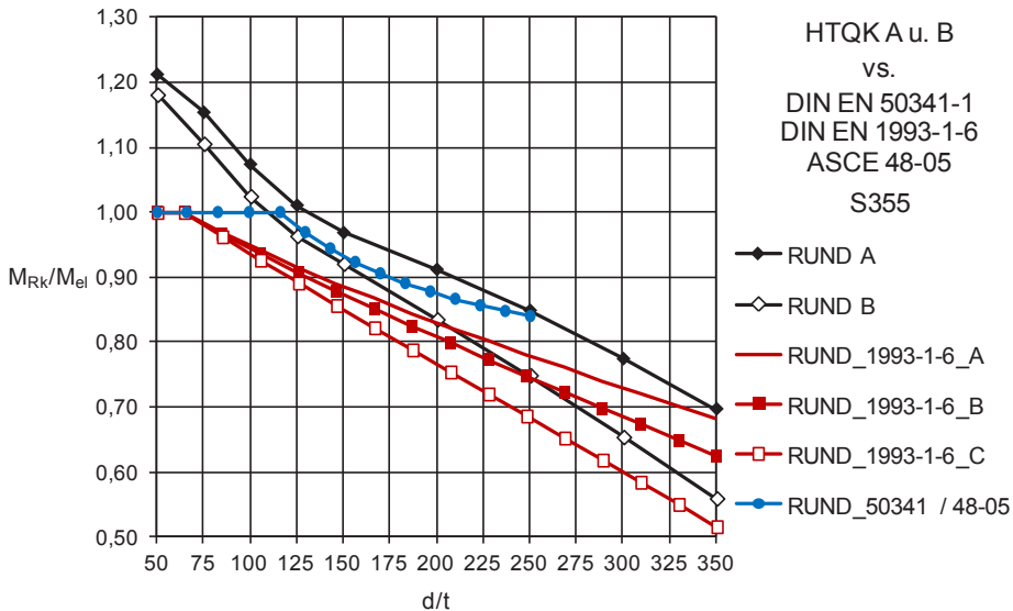
Abbildung 5.19: runde Querschnitte: HTQK A u. B vs. DIN EN 1993-1-6 [25], DIN EN 50341-1 [27] u. ASCE 48-05 [4]
