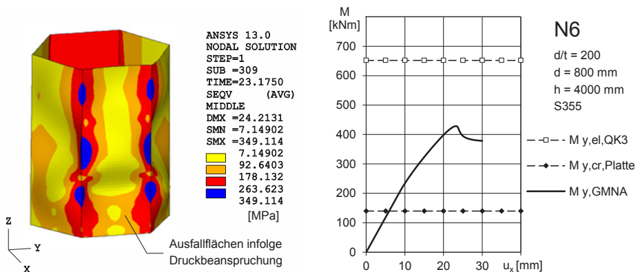
Abbildung 4.14: links: Vergleichsspannungsverteilung in Elementmitte unter Biegebeanspruchung „Moment parallel“ bei Erreichen der Traglast (unterer Mastabschnitt), rechts: zugehöriges Last-Verformungsdiagramm
