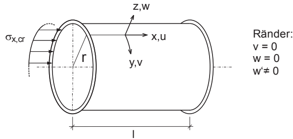
Abbildung 2.10: axialdruckbeanspruchte Kreiszyinderschale, Randbedingungen
