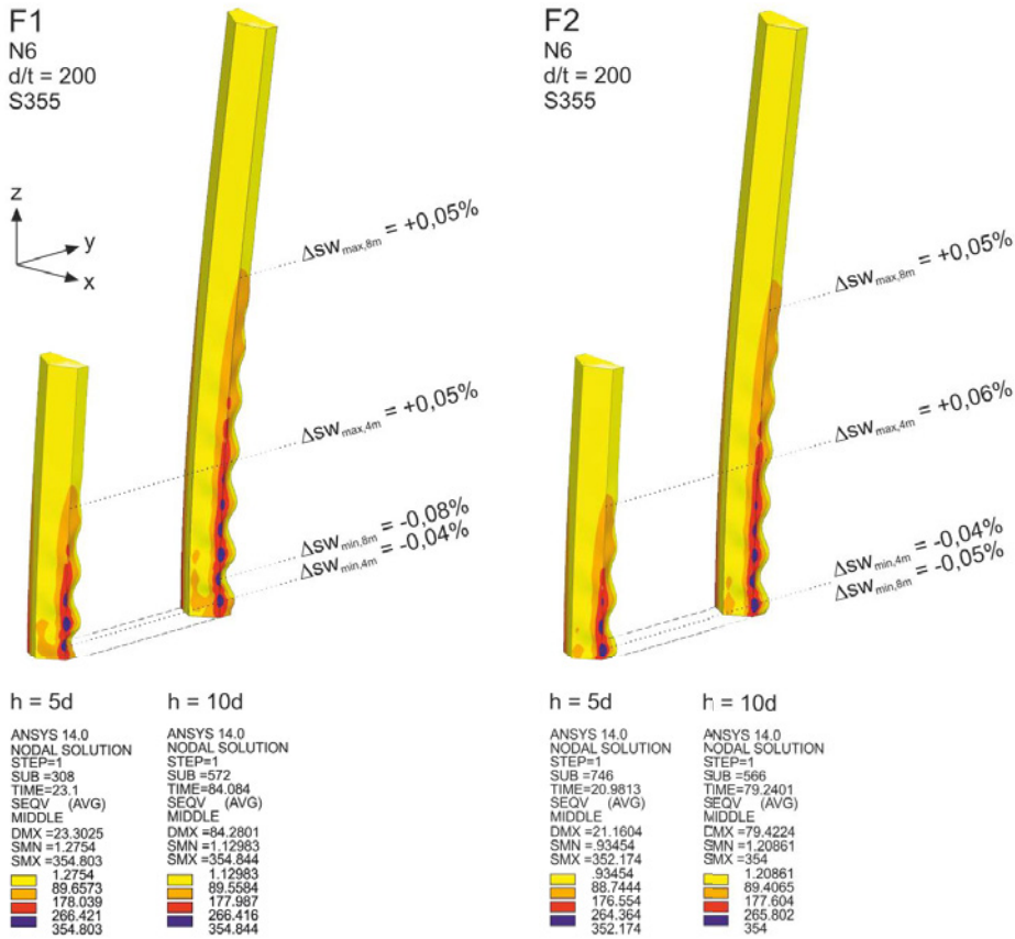
Abbildung 4.22: Vorbeulform der Masttypen F1 und F2 im GZT (halbes System, h = 5 d u. 10 d, 10-fach überhöht), Vergleichsspannungen in Elementmitte sowie Lage und Größe der min. und max. „Querschnittsovalisierung“
