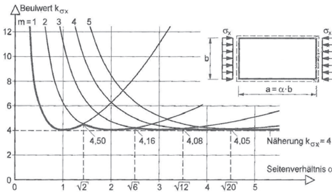
Abbildung 2.5: Beulwerte k_{\sigma_x} für rechteckige Platten mit konstanten Randspannungen aus [48]
