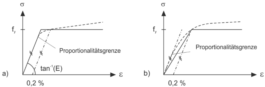
Abbildung 4.40: elastisch-ideal plastische Materialgesetze: links: konventioneller Ansatz, rechts: alternativer Ansatz für Werkstoffe mit niedriger Proportionalitätsgrenze
