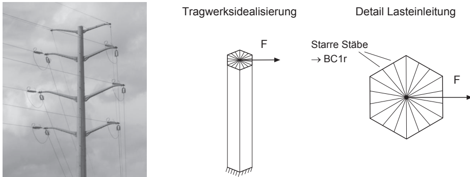
Abbildung 4.11: links: Beispiel Lasteinleitung, Mitte und rechts: Tragwerksidealisierung und zugehöriges Lasteinleitungsdetail
