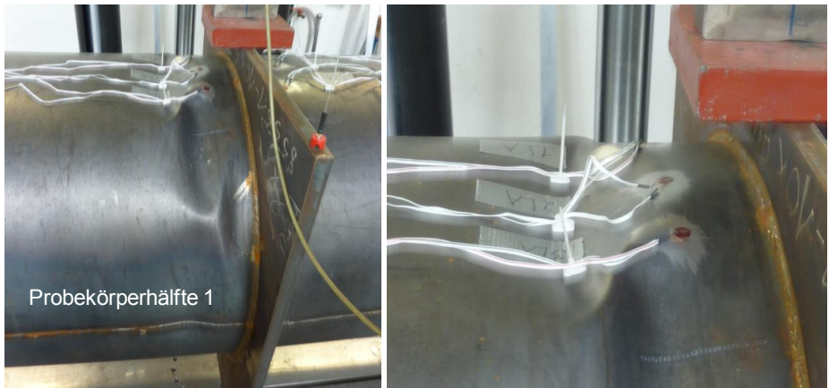
Abbildung 3.27: RUND 850 T3 V3: Beulen nach dem Versagen, Positionen der DMS auf der Probekörperoberseite
