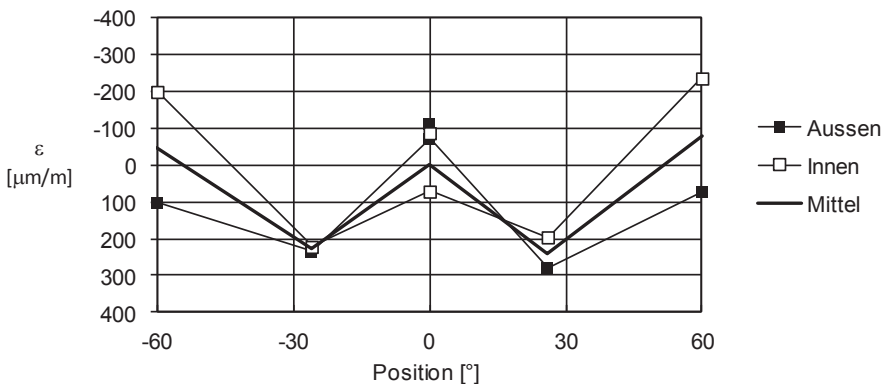
Abbildung 3.21: N6 SW768 T3 V3: Dehnungen in Umfangsrichtung, Laststufe 3, Probekörperhälfte 2
