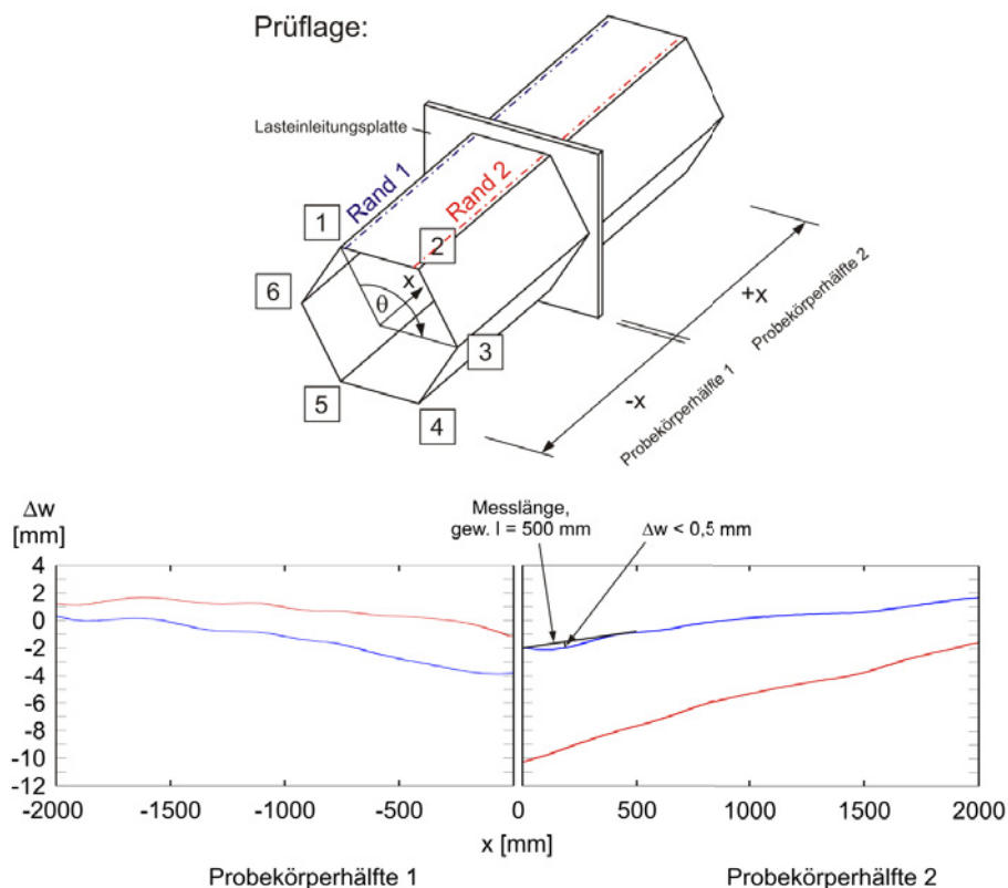
Abbildung 5.12: N6 SW768 T3 V3: Vorverformungen \Delta w der Ränder der am höchsten druckbeanspruchte Seitenfläche
