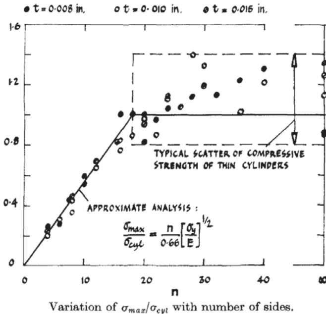
Abbildung 2.26: bezogene Beulspannung polygonaler Querschnitte nach Bulson [12]
