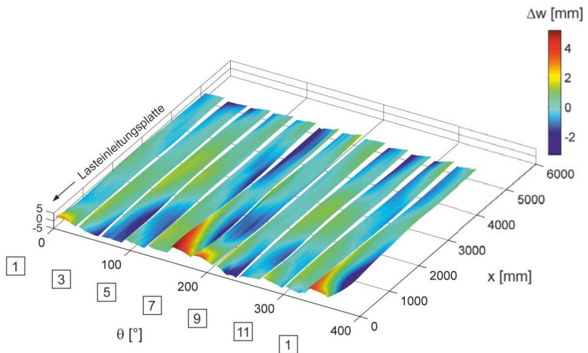
Abbildung 3.12: N12 SW845 T3 V3 Probekörperhälfte 2: \Delta w bez. auf best-fit Polygon
