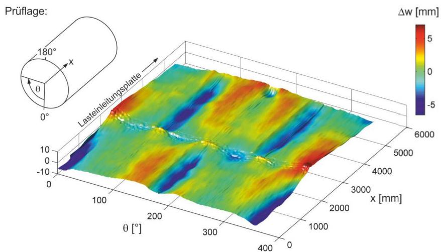
Abbildung 3.14: RUND 850 T3 V3 Probekörperhälfte 1: \Delta w bez. auf best-fit Zylinder
