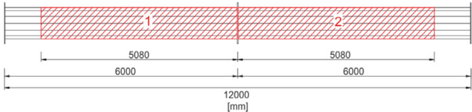
Abbildung 3.10: N12 SW845 T3 V3: Messbereiche
