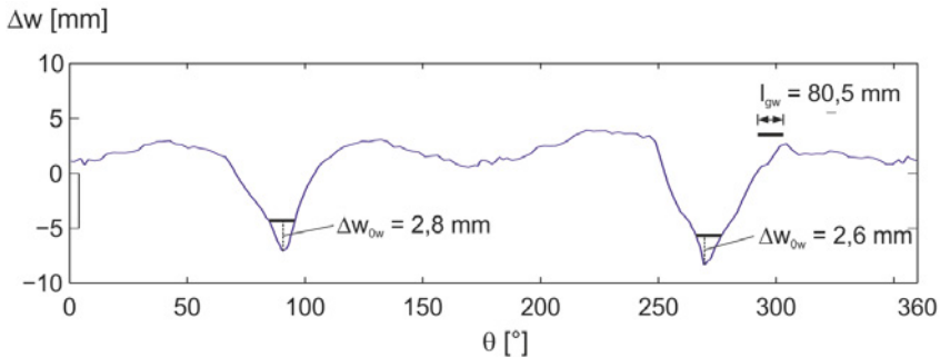
Abbildung 3.17: RUND 850 T3 V3 Probekörperhälfte 2: Querschnitt z=2120 mm
