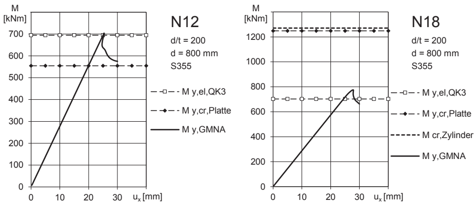
Abbildung 4.15: Last-Verformungsdiagramme N12 und N18 mit zugehörigen M_{el,QK3} und M_{cr}
