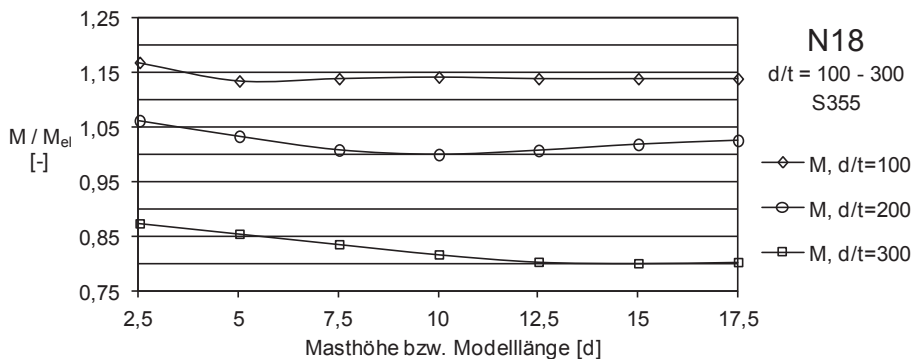
Abbildung 5.2: Biegetragfähigkeit M in Abhängigkeit der Masthöhe h (N18, d/t = 100 , 200 u. 300 ) bei konstanter Momentenbeanspruchung
