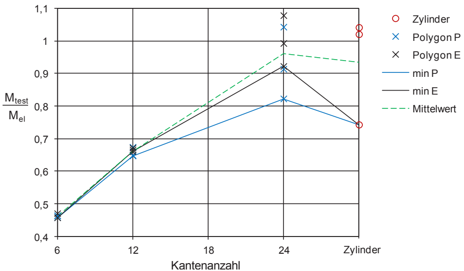
Abbildung 3.28: bezogene Biegetragfähigkeiten in Abhängigkeit der Kantenanzahl
