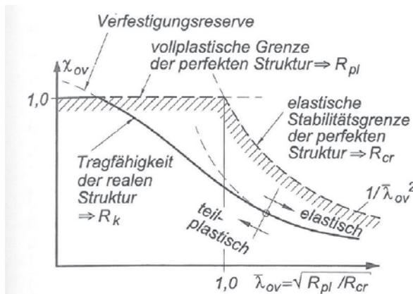
Abbildung 2.19: Beulabminderungsfaktor des MNA / LBA-Beulsicherheitsnachweises aus [76]
