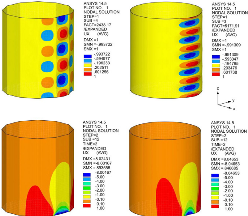
Abbildung 5.3: Imperfektionsansatz Eigenform (oben) und Imperfektionsansatz Anprall (unten) am Beispiel N12 und RUND ( d/t = 100 , d = 800 )
