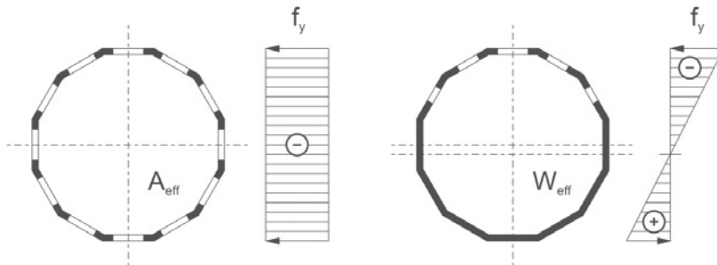
Abbildung 2.16: wirksame Querschnittsanteile (QK 4) [27]
