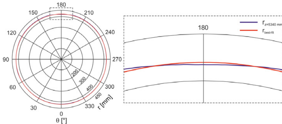
Abbildung 4.44: RUND 850 T3 V3: Umfangsschnitt durch die lokale Vorverformung nahe der Lasteinleitungsplatte ( z = 5340 mm)
