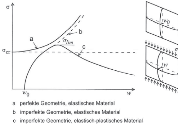
Abbildung 2.4: Überkritisches Tragverhalten schlanker, druckbeanspruchter Platten aus [7]
