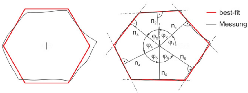
Abbildung 3.5: links: best-fit mit regelmäßigem Polygon, rechts: best-fit mit unregelmäßigem Polygon
