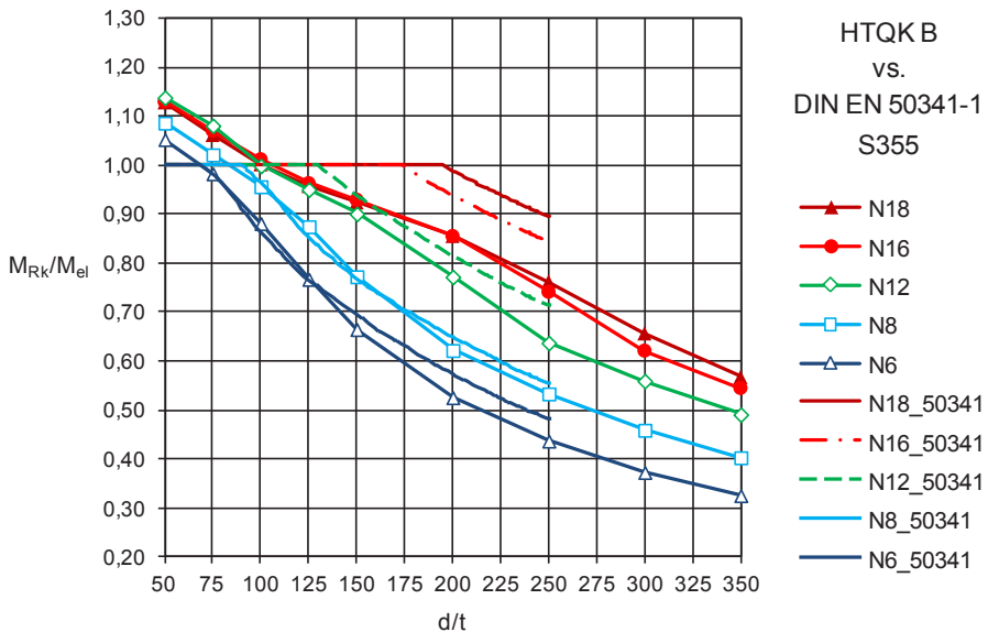
Abbildung 5.16: polygonale Querschnitte: HTQK B vs. DIN EN 50341-1 [27]
