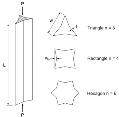
Abbildung 2.28: Vorverformungen der Seitenflächen [54]
