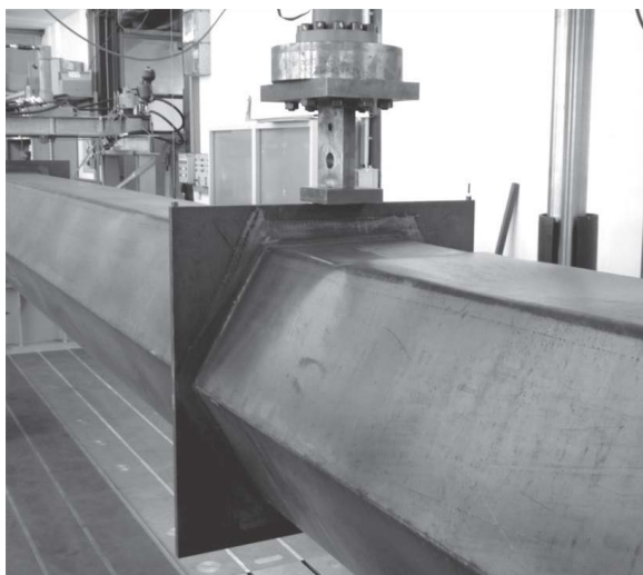
Abbildung 3.3: Detail Lasteinleitungsplatte, Probekörper N6 SW768 T3 V1
