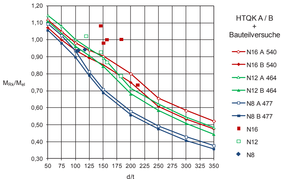
Abbildung 5.14: bezogene Biegetragfähigkeit M_{Rk}/M_{El} : N8, N12 u. N16, HTQK A u. B zusammen mit den Ergebnissen der Bauteilversuche aus [13]
