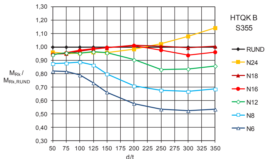
Abbildung 5.8: bezogene Biegetragfähigkeit M_{Rk}/M_{Rk,RUND} : N6 – RUND, HTQK B, d/t = 50 - 350
