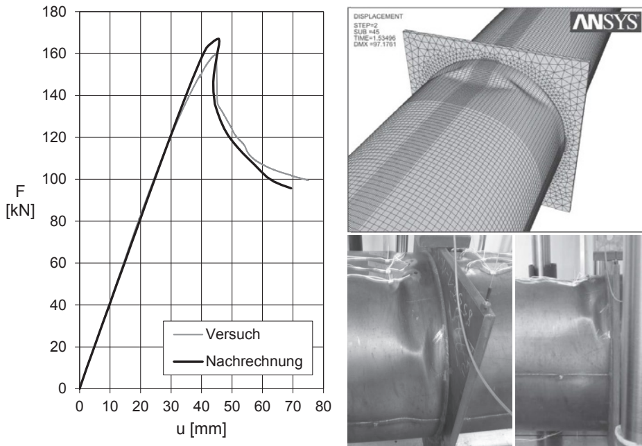
Abbildung 4.7: Berechnungsergebnisse Nachrechnung RUND_850_T3 Versuch 3, links: Last-Verformungskurven Versuch und Nachrechnung, rechts: Nachbeulformen Nachrechnung (ohne Überhöhung) und Versuch
