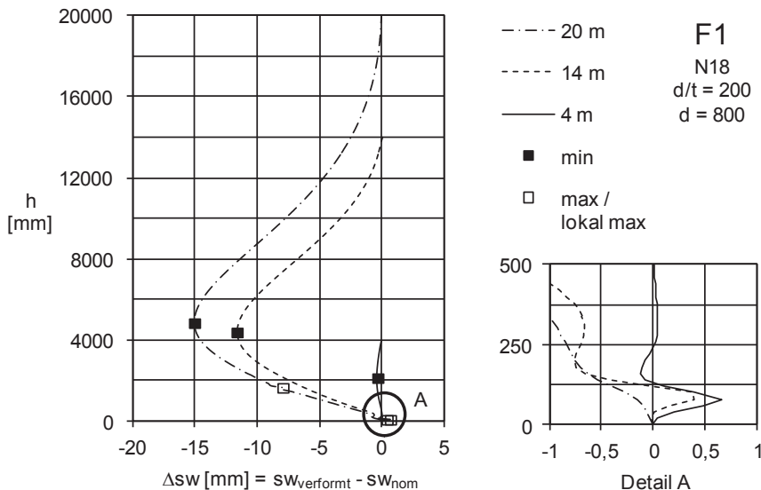
Abbildung 4.26: Entwicklung der Schlüsselweite (Ovalisierung) in Krafrichtung im GZT: h = 4 \text{ m} / 5 d , 14 \text{ m} / 17,5 d und 20 \text{ m} / 25 d (N18, F1, d/t = 200 )
