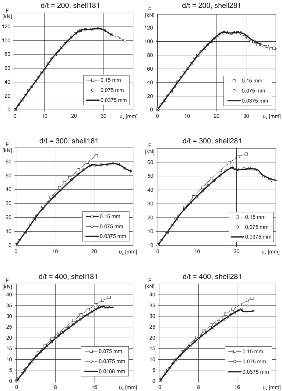
Abbildung 4.2: Variation der maximalen Lastschrittweite bei verschiedenen Schlankheiten, Elementgröße ca. 20 mm
