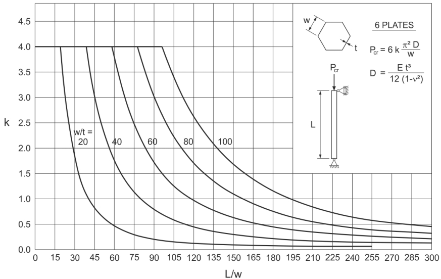
Abbildung 2.27: Beulwerte k für Pendelstützen mit hexagonalem Querschnitt aus [5]
