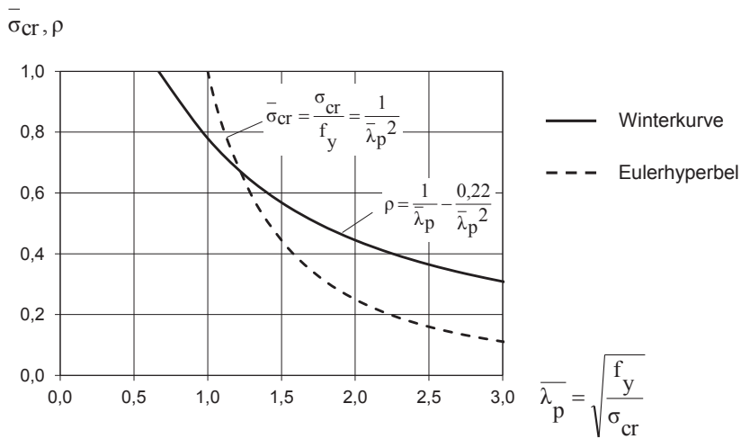
Abbildung 2.8: Winterkurve für eine allseitig gelagerte, gleichförmig druckbeanspruchte Platte und Eulerhyperbel
