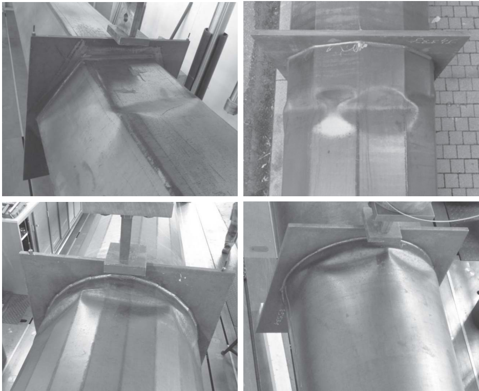
Abbildung 3.30: Beulformen: N6 SW768 T3 V1, N12 SW845 T3 V3, N24 SW845 T3 V1, RUND D850 T3 V1
