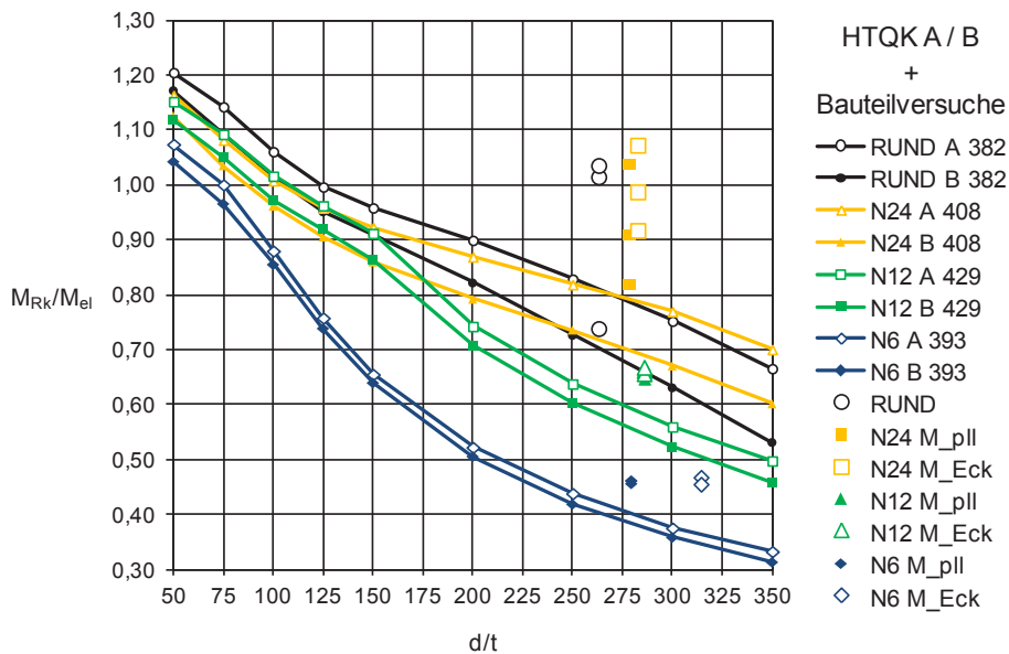
Abbildung 5.11: bezogene Biegetragfähigkeit M_{Rk}/M_{ei} : N6, N12, N24 u. RUND, HTQK A u. B zusammen mit den Ergebnissen der eigenen Bauteilversuche
