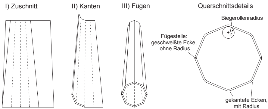
Abbildung 4.18: Herstellprozess eines polygonalen Masts, Querschnittsdetails
