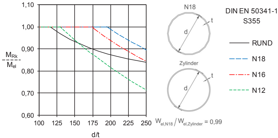
Abbildung 1.4: bezogene Biegetragfähigkeit M_{Rk}/M_{el} für polygonale und runde Querschnitte nach DIN EN 50341-1 [27]
