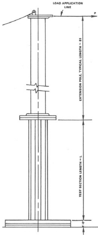
Abbildung 2.31: links: Versuchsaufbau, rechts: Bemessungsgleichungen [13], [4]
