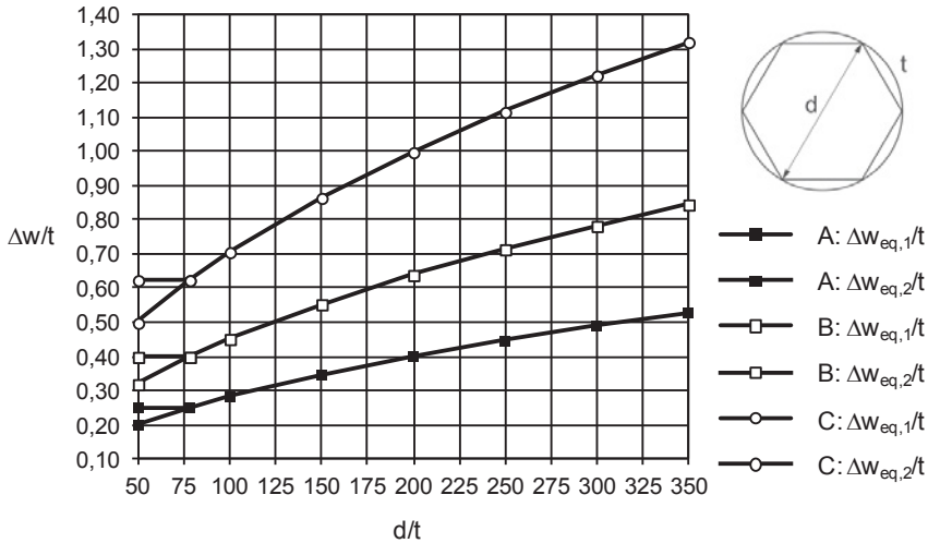
Abbildung 5.5: Amplituden der Ersatzimperfection \Delta w_{0,eq} für die Herstelltoleranz-Qualitätsklassen C: normal, B: hoch und A: exzellent
