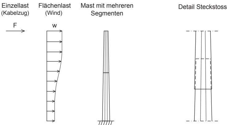
Abbildung 4.9: links: Tragwerk und Beanspruchungen, rechts: Detail Steckstoß
