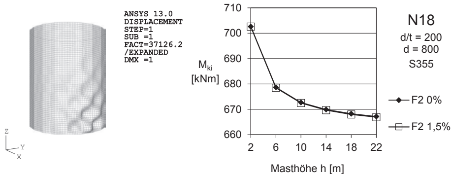
Abbildung 4.31: links: 1. Eigenform h = 18 m, rechts: M_{ki} in Abhängigkeit der Masthöhe für verschiedene Konizitäten
