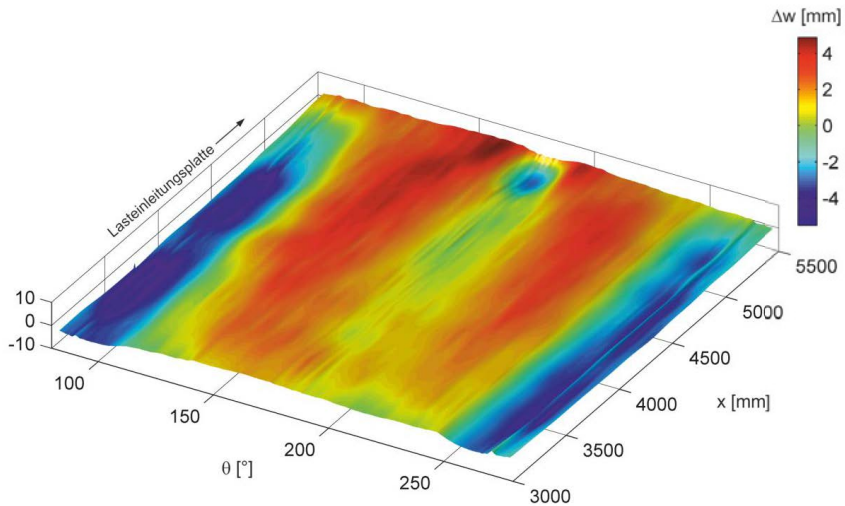
Abbildung 4.42: RUND 850 T3 V3: lokale Vorverformung (Ausschnitt aus Abbildung 3.14)
