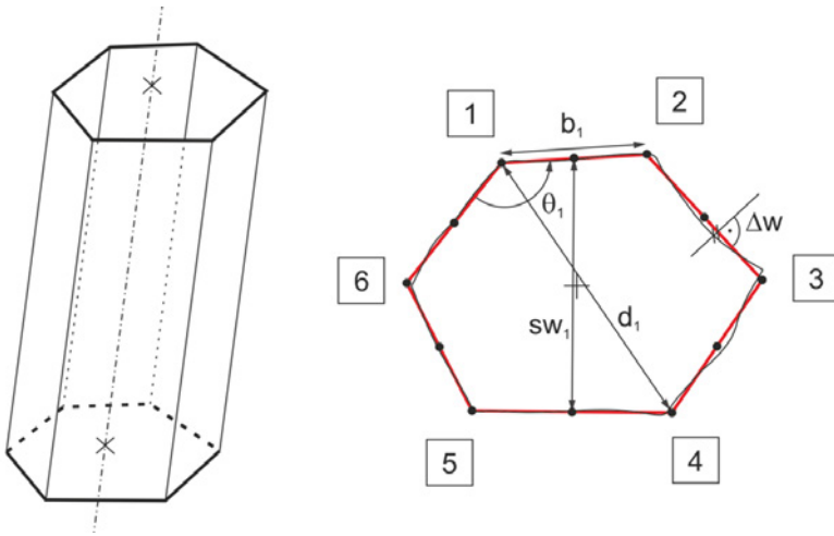
Abbildung 3.6: links: best-fit mit unregelmäßigem Polygon, rechts: abgeleitete Größen
