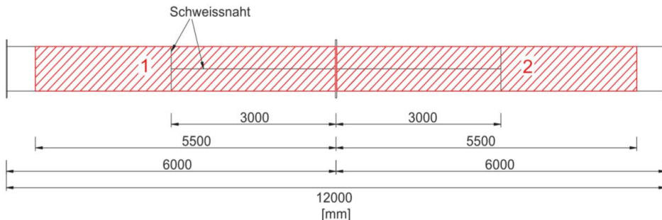
Abbildung 3.13: RUND 850 T3 V3: Messbereiche
