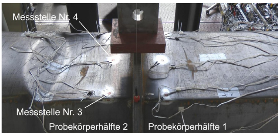
Abbildung 3.23: N6 SW768 T3 V3: Position der DMS auf der Oberseite, Lage der Beule nach dem Versagen
