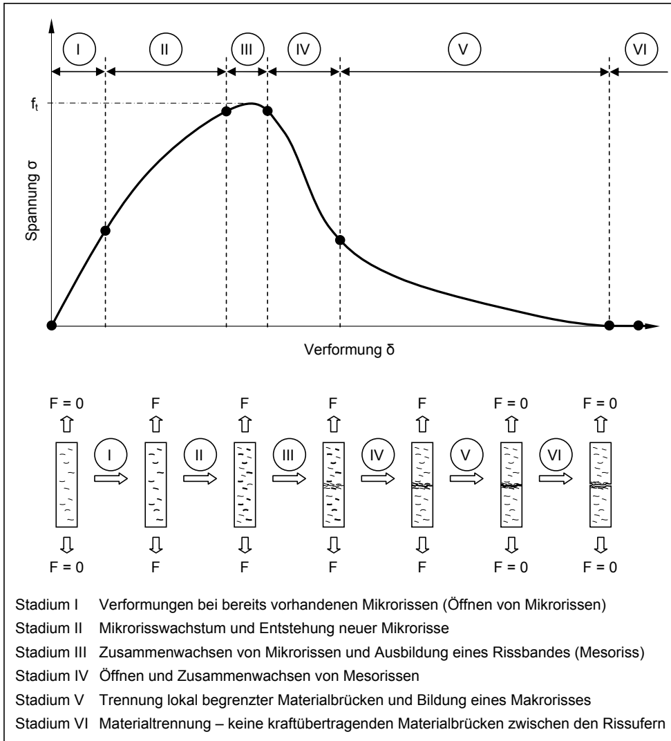
Abb. 2.10: Schematische Darstellung der Spannungs-Verformungskurve und des Bruchverlaufs einer zentrisch auf Zug beanspruchten Sandsteinprobe, in Anlehnung an [1, 33, 93]
