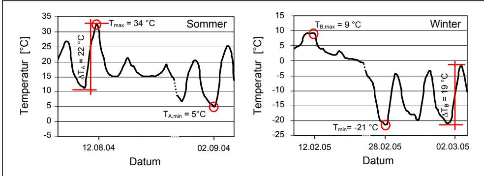
Abb. 4.12: Größte Temperaturänderungen innerhalb von 24 h sowie Minimal- und Maximaltemperaturen an der Gesteinsoberfläche im Sommer (links, Detail A aus Abbildung 4.11) und im Winter (rechts, Detail B aus Abbildung 4.11)
