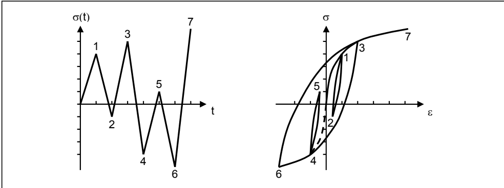
Abb. 2.16: Schematische Darstellung eines Spannungs-Zeit-Diagramms (links) und des entsprechenden Spannungs-Dehnungsdiagramms [78]
