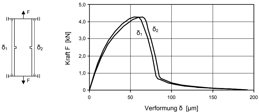
Abb. 3.17: Charakteristische Kraft-Verformungsverläufe für die beiden Wegaufnehmer in einem Zugversuch mit Behinderung der Prüfkörperverdrehung
