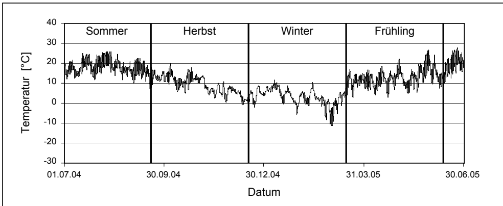
Abb. 4.13: Jahreszeitlicher Temperaturverlauf in einer Gesteinstiefe von 10 cm
