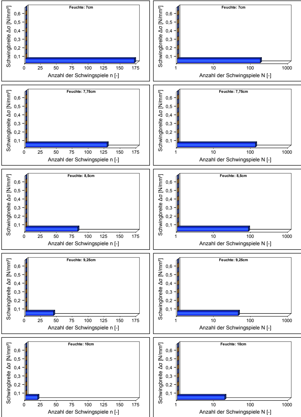
Abb. A-5.10: Stufendiagramme (links) und Spannungskollektive (rechts) der Beanspruchungen in- folge hygrischer Einwirkungen in unterschiedlichen Gesteinstiefen
