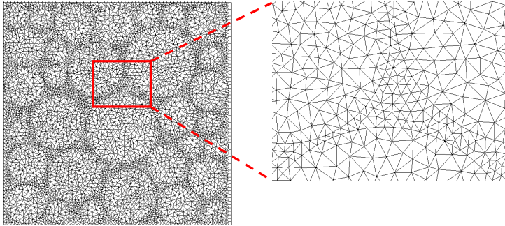
Abb. 4.29: FE-Netz des Gesamtmodells (links) sowie ein repräsentativer Ausschnitt für den Bereich zwischen den Einzelkörnern (rechts)
