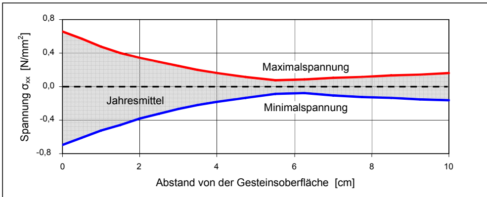
Abb. 4.21: Verteilung der thermisch induzierten Spannung bis in eine Gesteinstiefe von 10 cm
