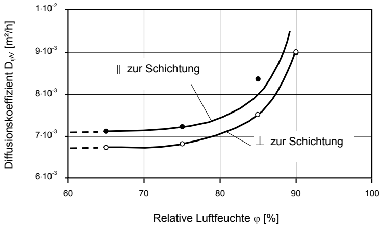
Abb. A-3.4: Gemessene Diffusionskoeffizienten D_{\phi,v} (Mittelwerte aus je 3 Einzelmessungen) in Abhängigkeit von der relativen Luftfeuchte und der Schichtorientierung (parallel bzw. senkrecht zur Schichtung) [67]
