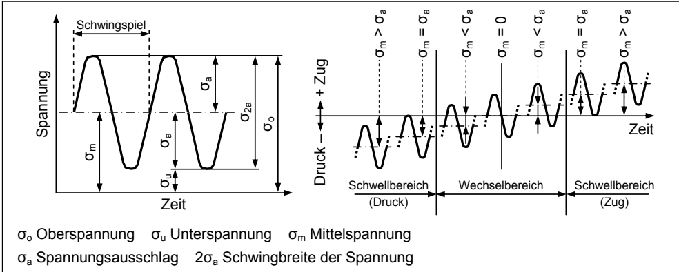
Abb. 2.14: Kenngrößen (links) und Beanspruchungsfälle (rechts) beim Wöhlerversuch [17]
