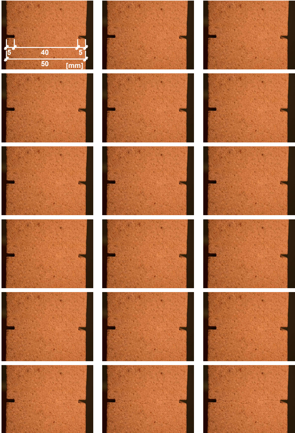
Abb. A-3.7: Durchtrennung eines Prüfkörpers im zentrischen Zugversuch
