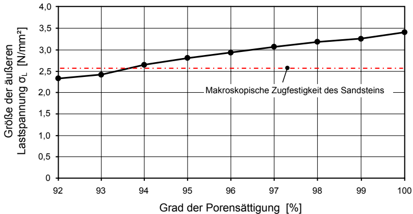
Abb. 4.39: Transformation der vom Porenfüllgrad abhängigen inneren Drücke durch Eisbildung in äußere Lastspannungen
