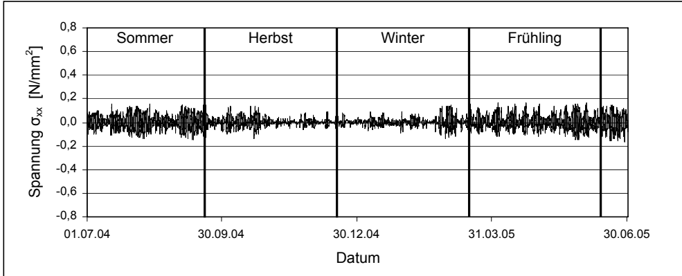
Abb. 4.20: Jahreszeitlicher Verlauf der thermisch induzierten Spannungen in einer Gesteinstiefe von 10 cm
