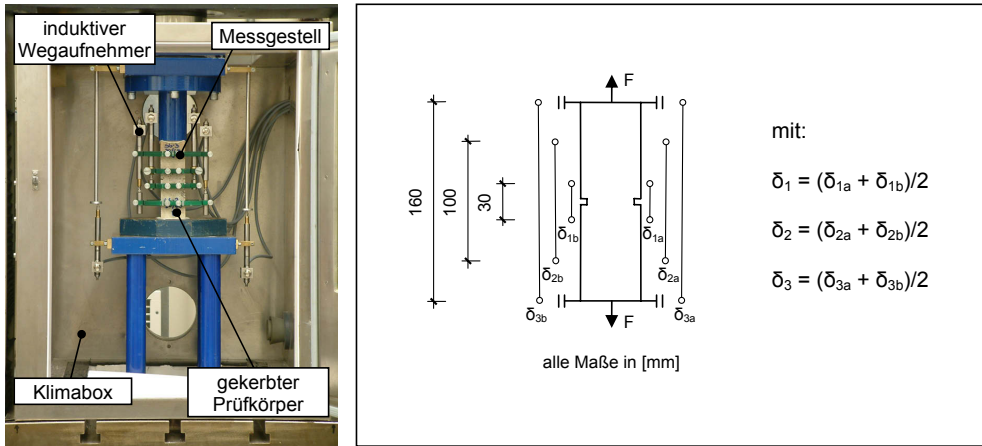
Abb. 3.20: Versuchsaufbau für die Durchführung der bruchmechanischen Untersuchungen (links) und schematische Darstellung der Anordnung der Wegaufnehmer sowie die Bezeichnung der jeweiligen Messgrößen (rechts)
