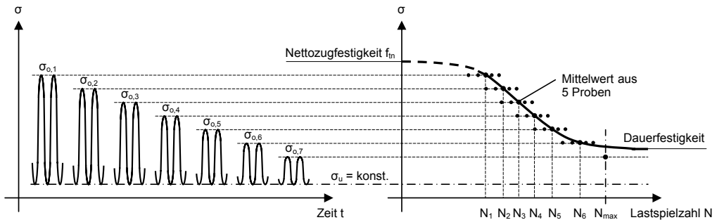
Abb. 3.26: Ermittlung der Wöhlerlinie bei konstanter Unterspannung \sigma_u
