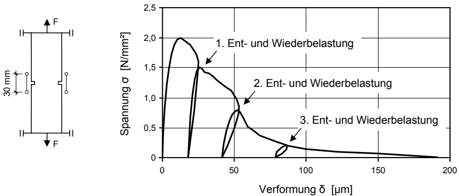
Abb. 3.18: Spannungs-Verformungsverlauf für einen zentrischen Zugversuch mit mehrfacher Entlastung und Wiederbelastung
