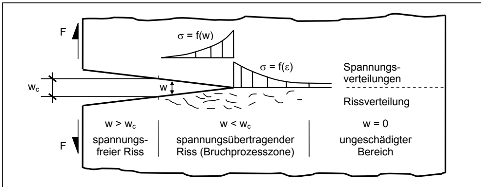
Abb. 2.11: Spannungübertragung über einen Riss nach dem Konzept der Kohäsionsrissmodelle, in Anlehnung an [72]
