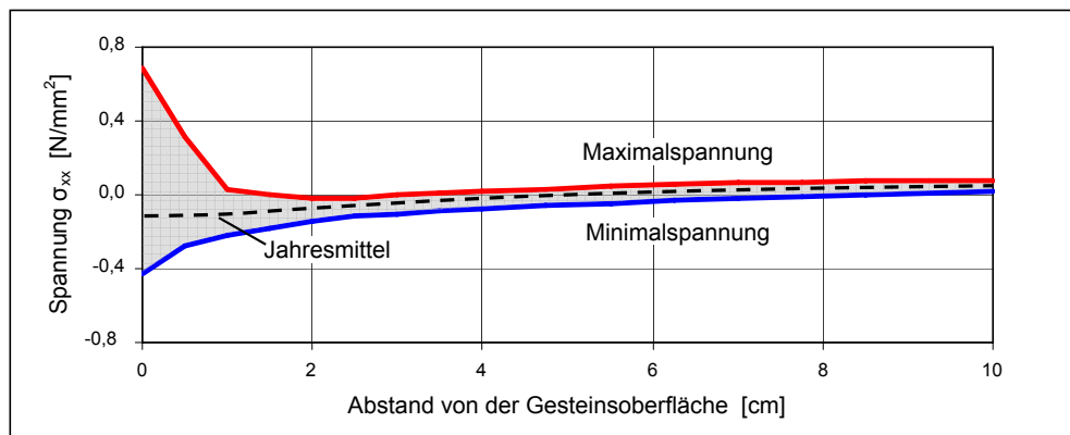
Abb. 4.24: Verteilung der hygrisch induzierten Spannung bis in eine Steintiefe von 10 cm
