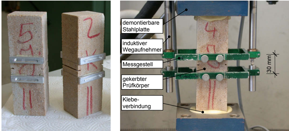
Abb. 3.27: Mit Aluminiumschiene präparierte Prüfkörper (links) sowie der Einbauzustand in die Prüfmaschine zur Durchführung der dynamischen Zugversuche (rechts)
