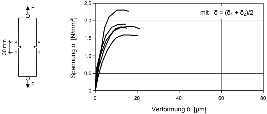
Abb. 3.14: Exemplarische Versuchsergebnisse der Zugversuche an gekerbten Prüfkörpern ohne Behinderung der Prüfkörperverdrehung (gelenkige Lagerung)
