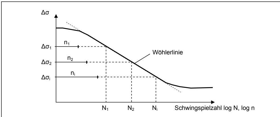
Abb. 2.18: Graphische Darstellung zur Schadensakkumulationshypothese nach Palmgren-Miner
