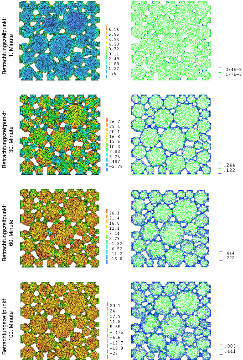
Abb. 4.35: Entwicklung der Hauptzugspannungen \sigma_{11} [ N/mm^2 ] (links) und der Rissdehnungen \epsilon_{cr} [-] infolge einer Eisbildung bei einer Porensättigung von 100 %
