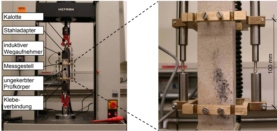
Abb. 3.11: Versuchsaufbau für die Durchführung der Zugversuche an ungekerbten Prüfkörpern ohne Behinderung der Prüfkörperverdrehung (gelenkige Lagerung)
