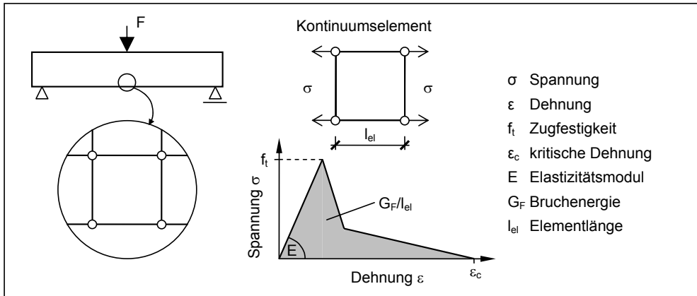
Abb. 2.13: Implementierung des Crack Band Modells zur Beschreibung des Tragverhaltens unter Zugbeanspruchung nach [93]
