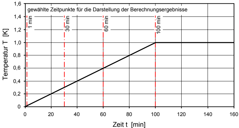
Abb. 4.34: Zeitlicher Verlauf der Temperaturerhöhung um 1 K zur Erzielung einer Expansion des Eismaterials um 9 %
