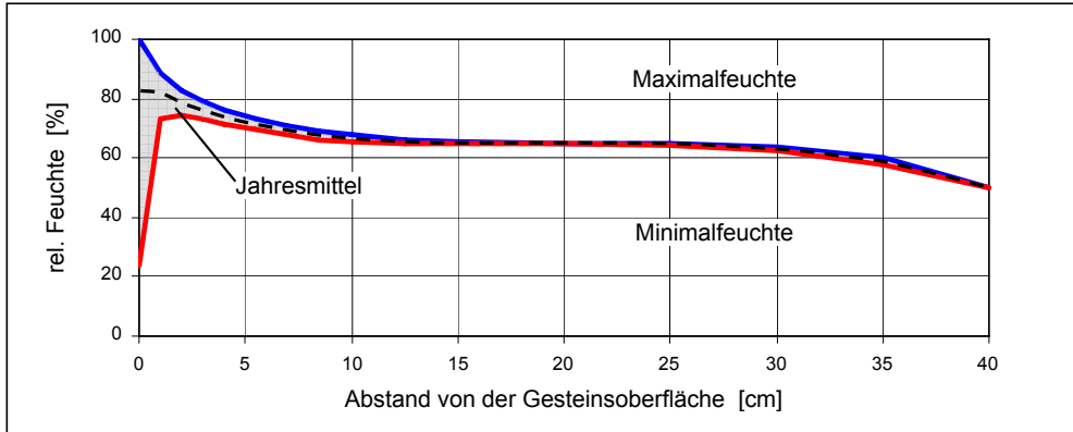
Abb. 4.18: Jahreszeitlicher Feuchteschwankungsbereich über die Gesteinstiefe
