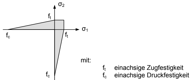
Abb. 4.31: Beschreibung des biaxialen Tragverhaltens vom porenfreien Sandsteinmaterial
