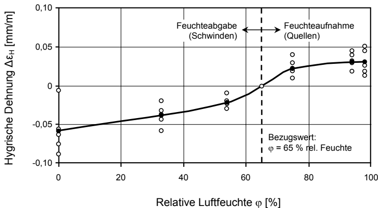
Abb. A-3.5: Messwerte der Sorptionsversuche – hygrische Dehnungen \Delta\epsilon_H im hygrokopischen Feuchtebereich in Abhängigkeit von der relativen Luftfeuchte \phi [67]
