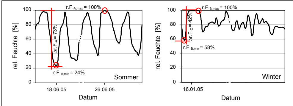
Abb. 4.16: Größte Feuchteänderung innerhalb von 24 h sowie charakteristische Feuchteänderungen an der Gesteinsoberfläche im Sommer (links, Detail A aus Abbildung 4.15) und im Winter (rechts, Detail B aus Abbildung 4.15)
