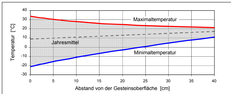
Abb. 4.14: Jahreszeitlicher Temperaturschwankungsbereich über die Gesteinstiefe
