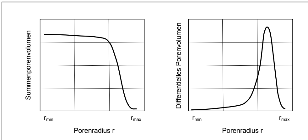
Abb. 2.7: Summenporenvolumenkurve (links) und Porengrößenverteilungskurve (rechts)
