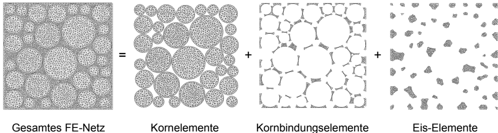
Abb. 4.30: Aufbau des numerischen Modells bestehend aus Körnern, Kornbindungen sowie Porenraum bzw. Eis
