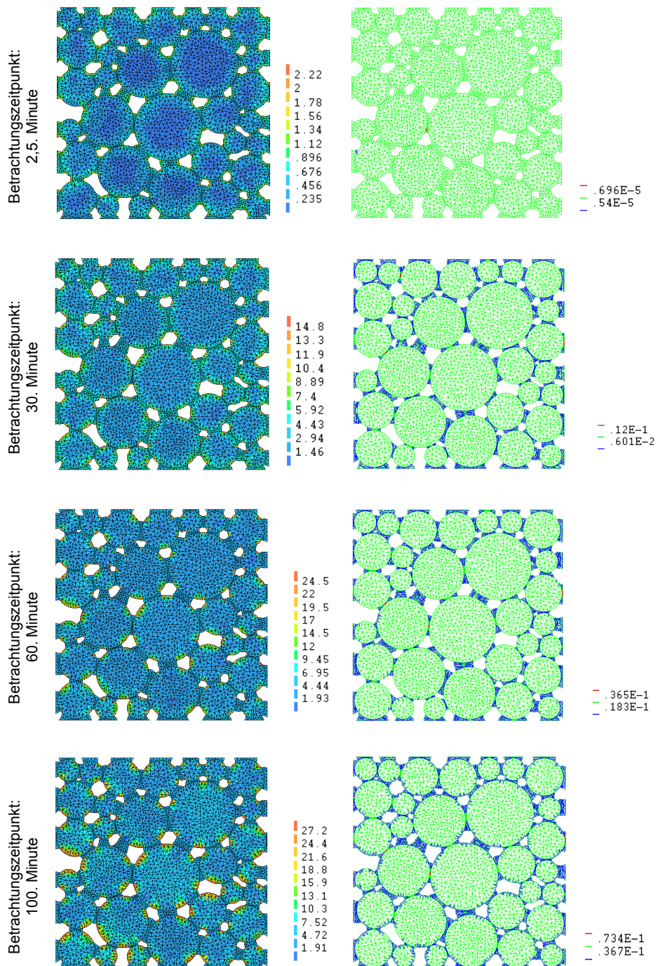
Abb. A-4.5: Entwicklung der Hauptzugspannungen \sigma_{11} [N/mm 2 ] (links) und der Rissdehnungen \epsilon_{cr} [-] infolge einer Eisbildung bei einer Porensättigung von 92 %
