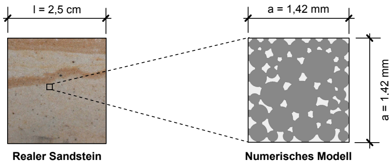
Abb. 4.28: Größe des zweidimensionalen Strukturmodells auf Mesoebene
