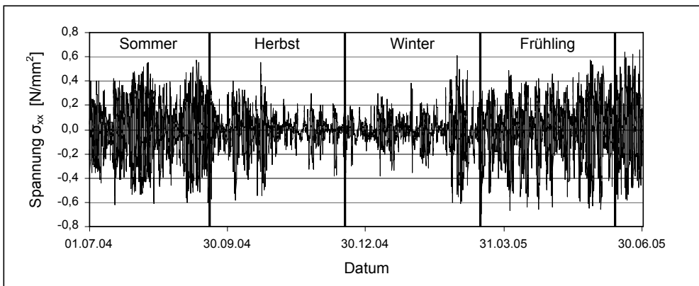
Abb. 4.19: Jahreszeitlicher Verlauf der thermisch induzierten Spannungen an der Gesteinsoberfläche
