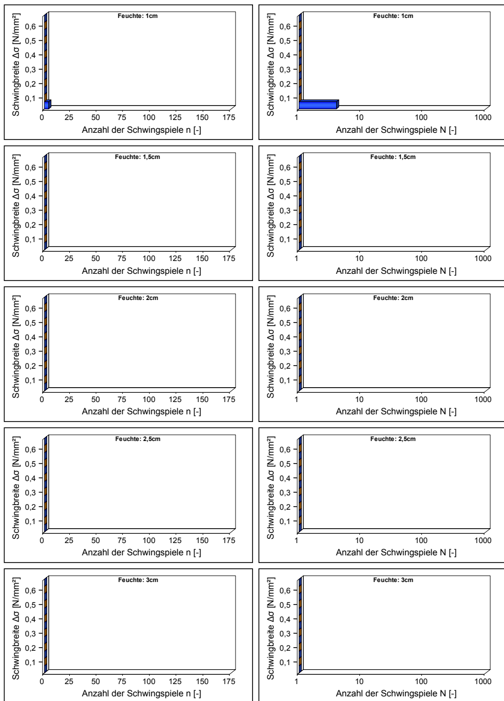
Abb. A-5.8: Stufendiagramme (links) und Spannungskollektive (rechts) der Beanspruchungen in- folge hygrischer Einwirkungen in unterschiedlichen Gesteinstiefen
