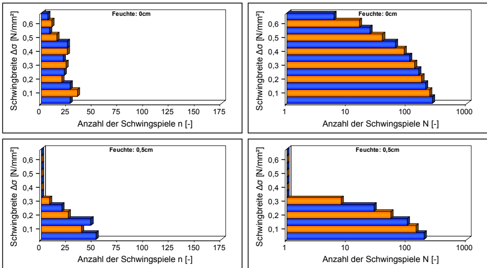
Abb. A-5.7: Stufendiagramme (links) und Spannungskollektive (rechts) der Beanspruchungen infolge hygrischer Einwirkungen in unterschiedlichen Gesteinstiefen
