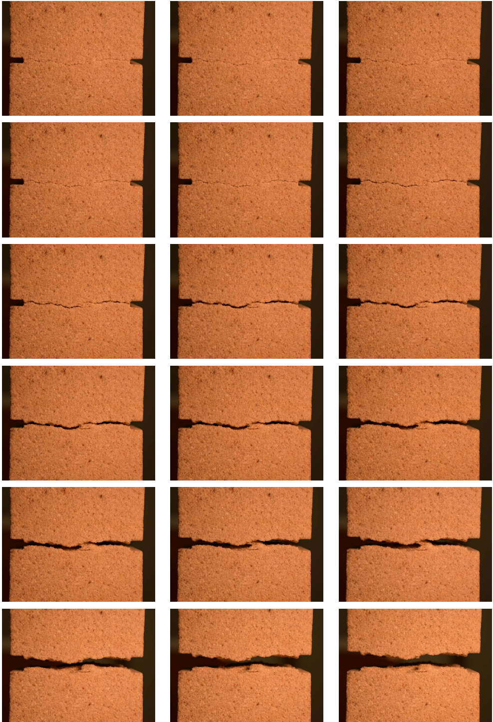
Abb. A-3.7: Durchtrennung eines Prüfkörpers im zentrischen Zugversuch (Fortsetzung)
