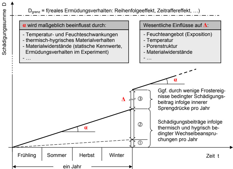
Abb. 5.6: Schematische Darstellung der Schädigungsbeiträge gemäß Gleichung 5.4 für einen Zeitraum von einem Jahr
