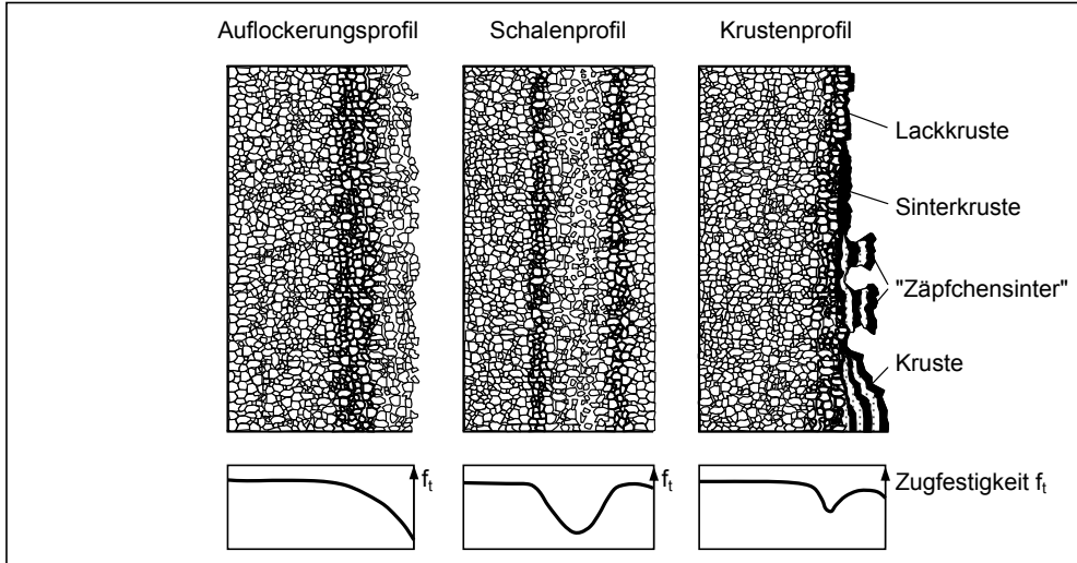
Abb. 2.23: Schematische Darstellung der oberflächlichen Verwitterungsprofile und ihrer Verteilungen der Gesteinszugfestigkeiten (in Anlehnung an [51, 67])
