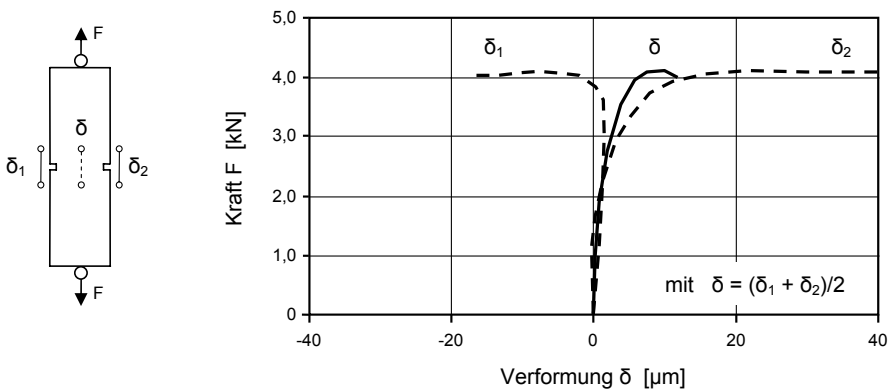
Abb. 3.15: Charakteristische Kraft-Verformungsverläufe für die beiden Wegaufnehmer in einem Zugversuch ohne Behinderung der Prüfkörperverdrehung
