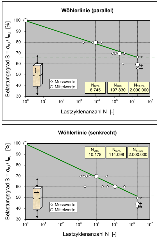
Abb. 3.29: Versuchsergebnisse der dynamischen Zugversuche für eine Belastung parallel zur Schichtungsrichtung (oben) und senkrecht zur Schichtungsrichtung (unten)
