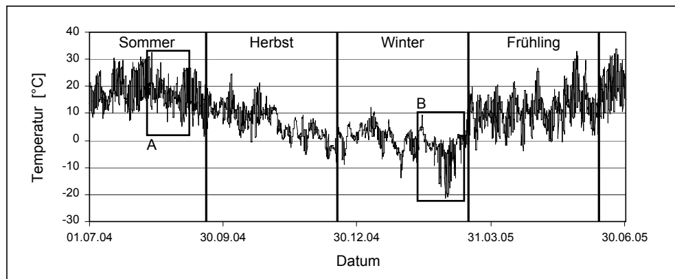
Abb. 4.11: Jahreszeitlicher Temperaturverlauf an der Gesteinsoberfläche
