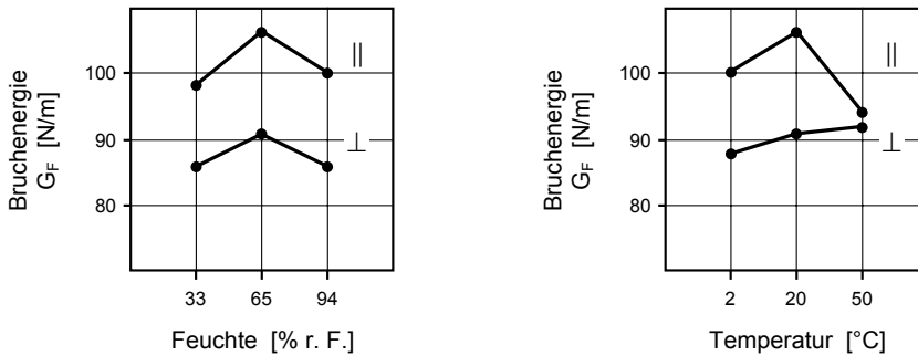
Abb. 3.25: Einfluss der Feuchte- und Temperaturbedingungen auf die Bruchenergie G_F bei einer Beanspruchung parallel (//) bzw. senkrecht (⊥) zur Schichtungsorientierung
