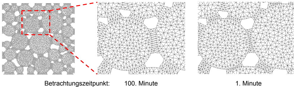
Abb. 4.36: Elementdeformationen infolge einer Eisbildung im Porenraum des Sandsteins
