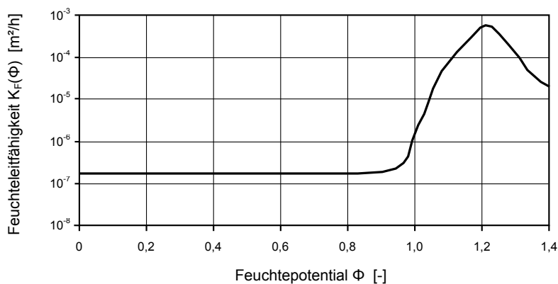
Abb. 4.2: Feuchteleitfähigkeit parallel zur Schichtung des Postaer Sandsteins der Varietät Mühlenteile in Abhängigkeit vom Feuchtepotential [67]
