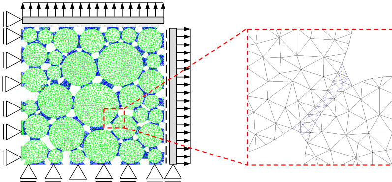
Abb. 4.38: Rissbild infolge einer äußeren Lastspannung von 3,3 \text{ N/mm}^2
