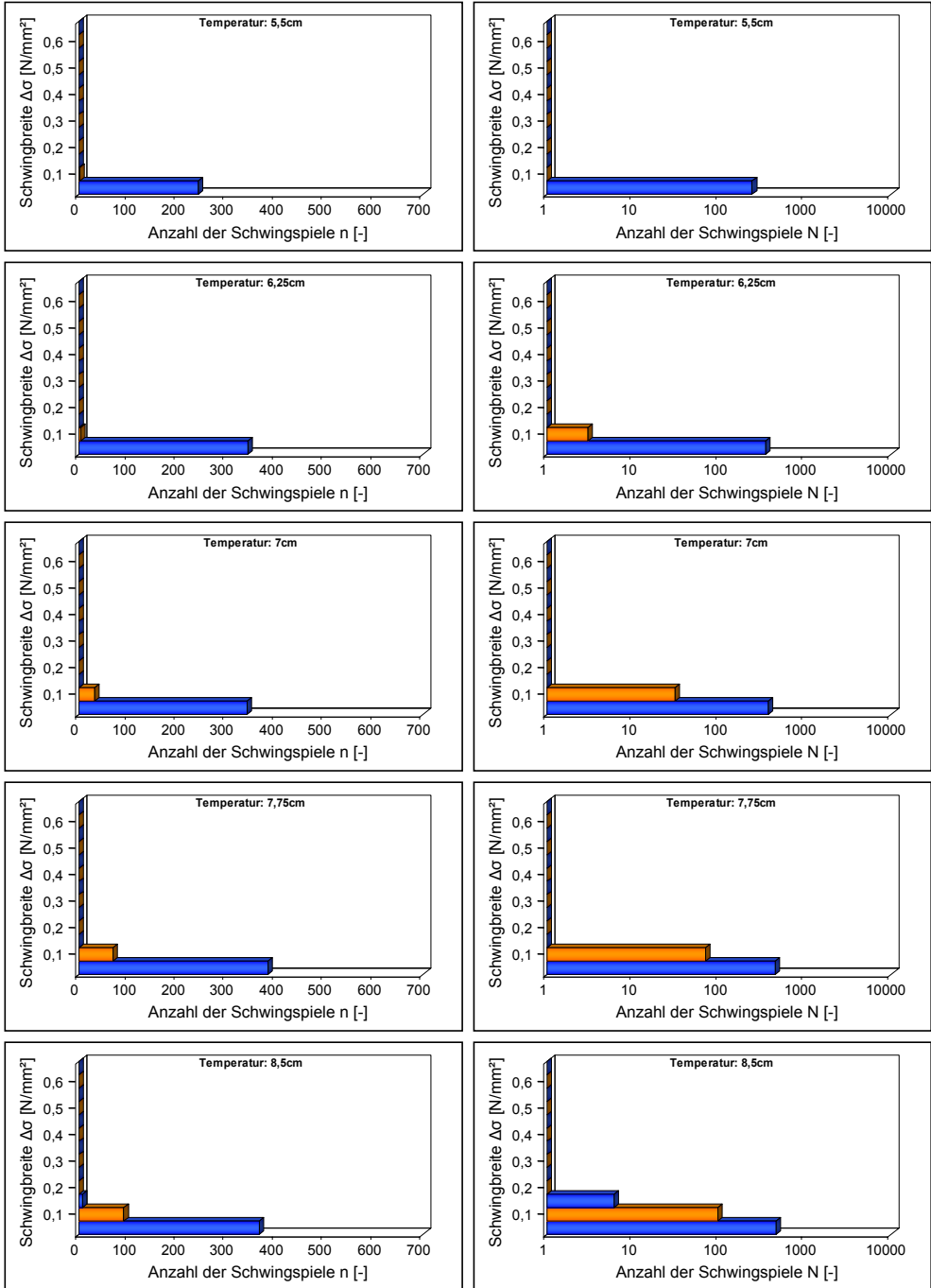
Abb. A-5.5: Stufendiagramme (links) und Spannungskollektive (rechts) der Beanspruchungen in- folge thermischer Einwirkungen in unterschiedlichen Gesteinstiefen
