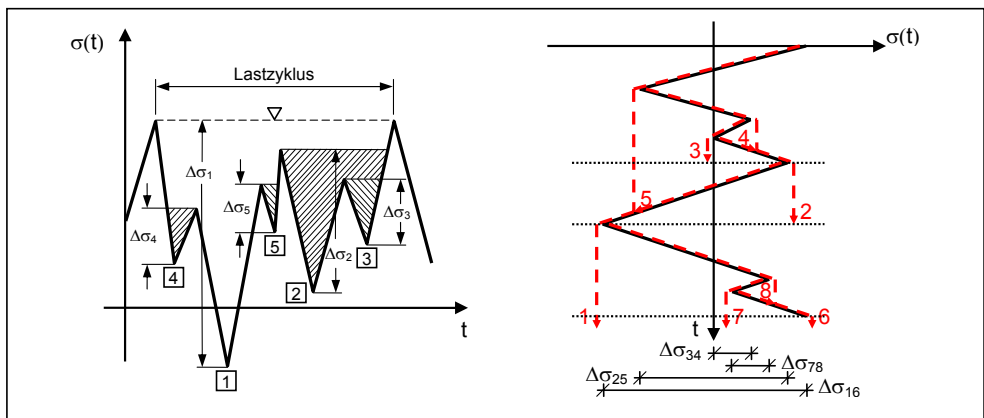
Abb. 2.17: Reservoir-Verfahren (links) und Rainflow-Verfahren (rechts) [78]
