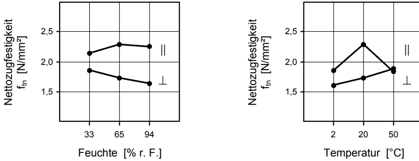
Abb. 3.24: Einfluss der Feuchte- und Temperaturbedingungen auf die Nettozugfestigkeit f_{tn} bei einer Beanspruchung parallel (//) bzw. senkrecht (⊥) zur Schichtungsorientierung
