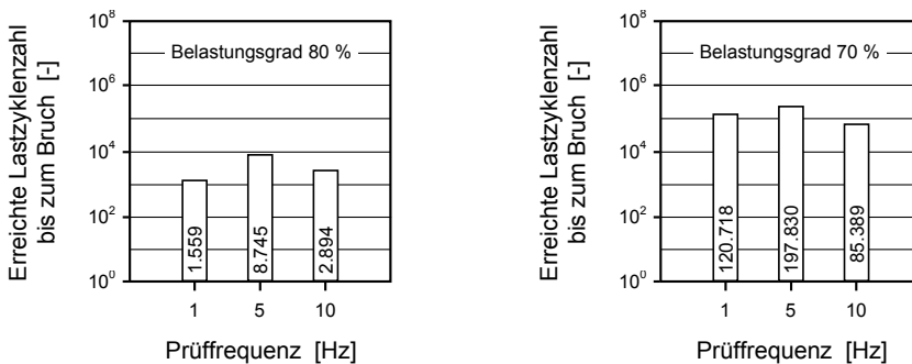
Abb. 3.28: Einfluss der Prüffrequenz auf die erreichte Lastspielzahl bis zum Bruch bei einer Belastungsrichtung parallel zur Schichtungsrichtung (Mittelwerte aus drei Einzelversuchen bei den Prüffrequenzen 1 und 10 Hz; Mittelwerte aus fünf Einzelversuchen bei der Prüffrequenz von 5 Hz)
