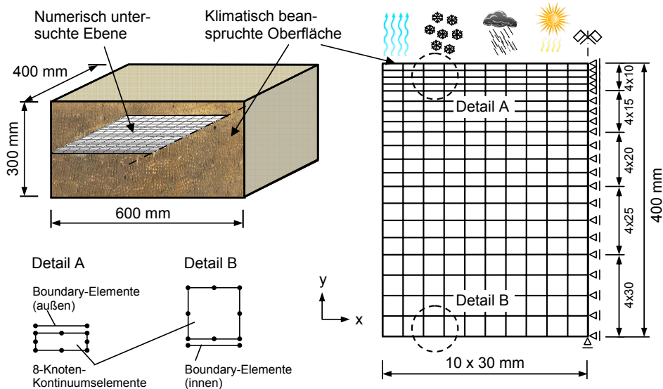
Abb. 4.6: Numerisch untersuchte Ebene eines Sandsteinkontinuums und diskretisiertes System
