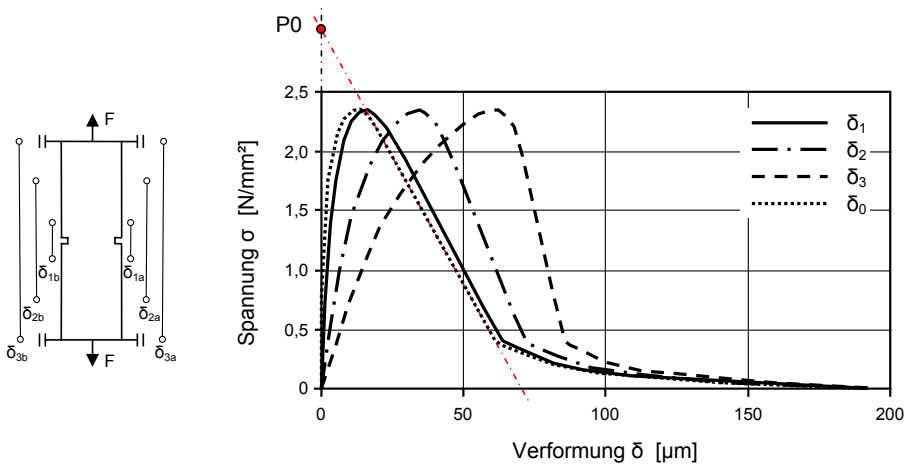
Abb. 3.23: Mögliche Entwicklung der Spannungs-Rissöffnungsbeziehung aus den vorliegenden experimentellen Versuchsergebnissen
