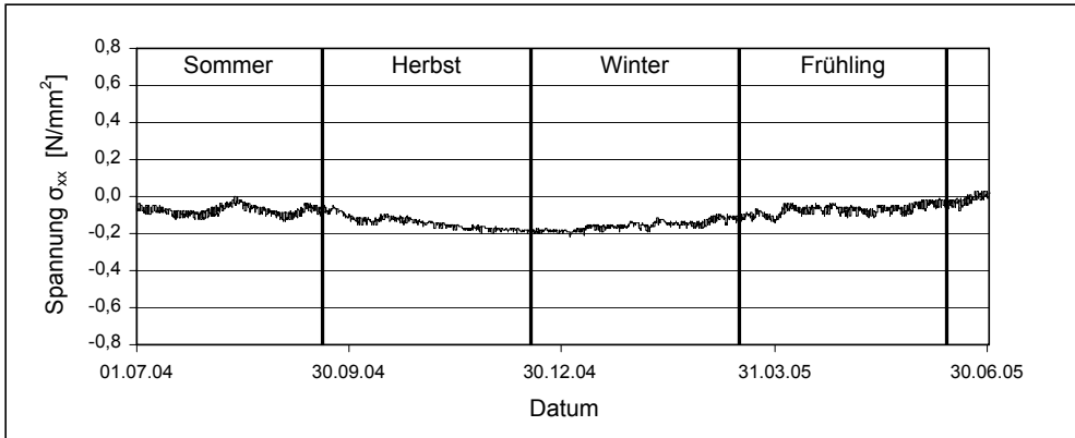
Abb. 4.23: Jahreszeitlicher Verlauf der hygrysch induzierten Spannungen in einer Gesteinstiefe von 1 cm
