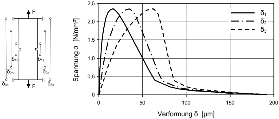
Abb. 3.21: Charakteristische Verläufe der Spannungs-Verformungsbeziehungen für unterschiedlich angeordnete Wegaufnehmer entlang der Prüfkörperlängsachse
