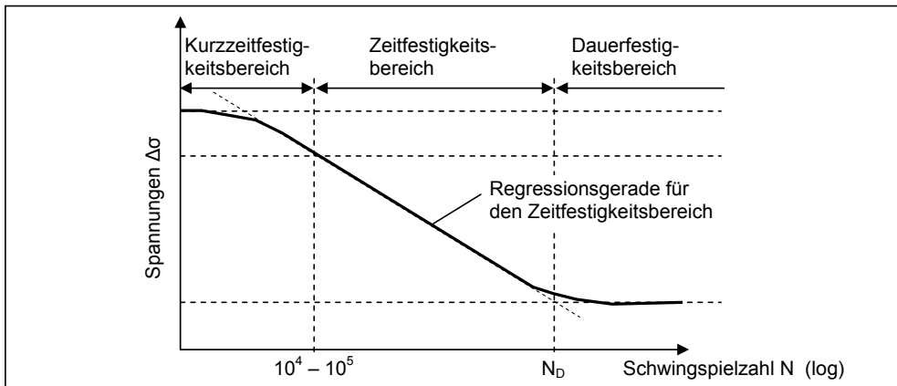
Abb. 2.15: Schematische Darstellung einer Wöhlerlinie mit ihren charakteristischen Festigkeitsbereichen [85, 102]
