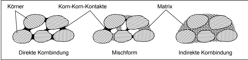
Abb. 2.3: Schematische Darstellung des mikrostrukturellen Aufbaus von Sandsteinen nach [1]
