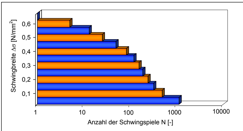
Abb. 5.5: Spannungskollektiv der infolge thermischen Einwirkungen an der Gesteinsoberfläche resultierenden Beanspruchungen (Betrachtungszeitraum: 1 Jahr)
