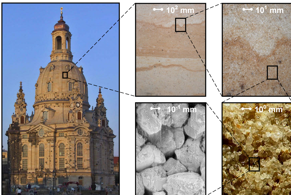
Abb. 3.1: Frauenkirche Dresden und das strukturelle Erscheinungsbild des Postaer Sandsteins in unterschiedlichen Vergrößerungen
