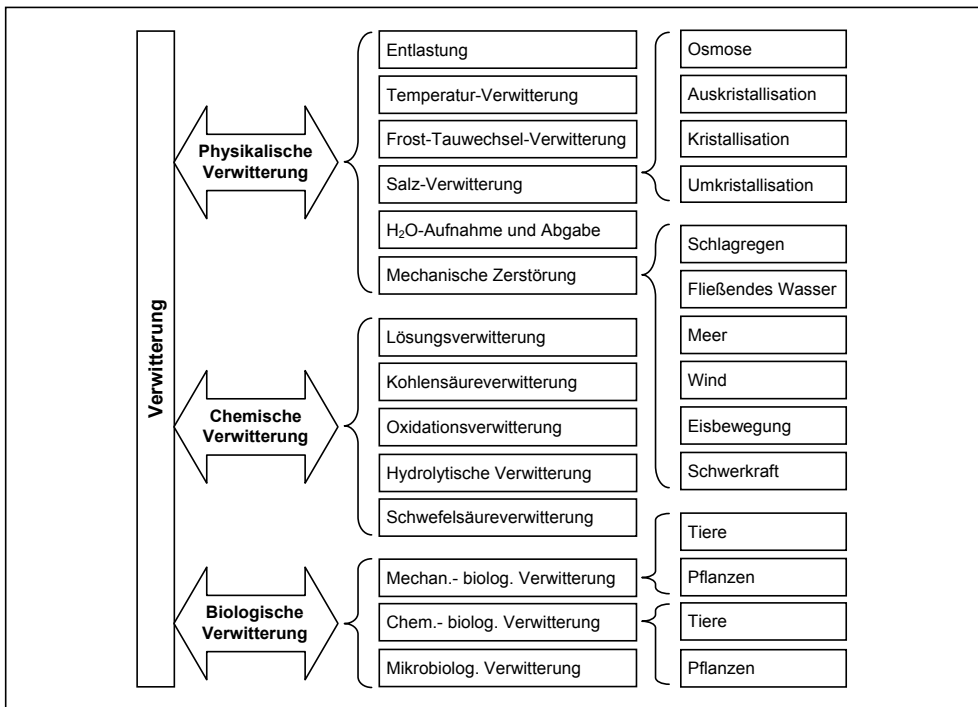
Abb. 2.20: Hauptgruppen der Verwitterung und Klassifikation der Verwitterungsarten nach [41]
