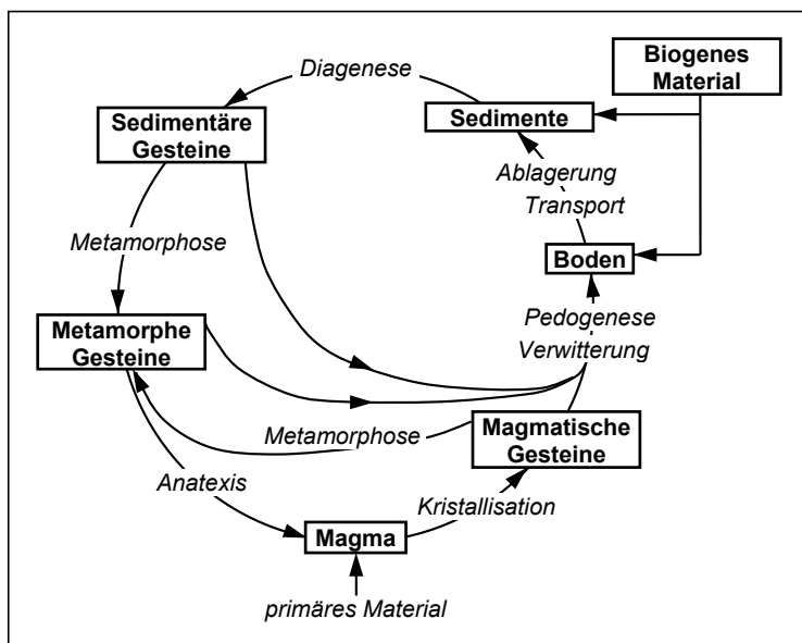
Abb. 2.1: Gesteinskreislauf nach [121]
