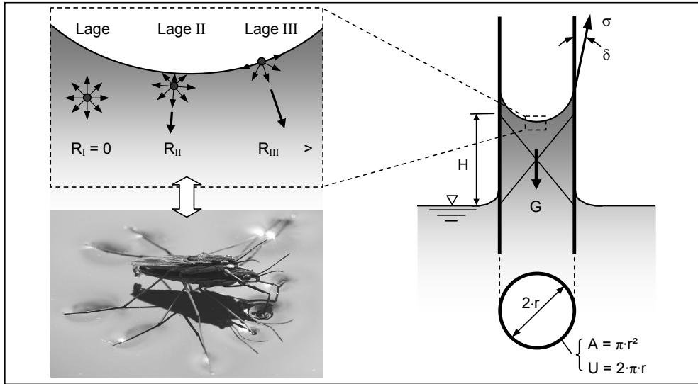
Abb. 2.9: Zustandekommen der Oberflächenspannung (links) und Flüssigkeitssäule in einer zylindrischen Kapillare (rechts)
