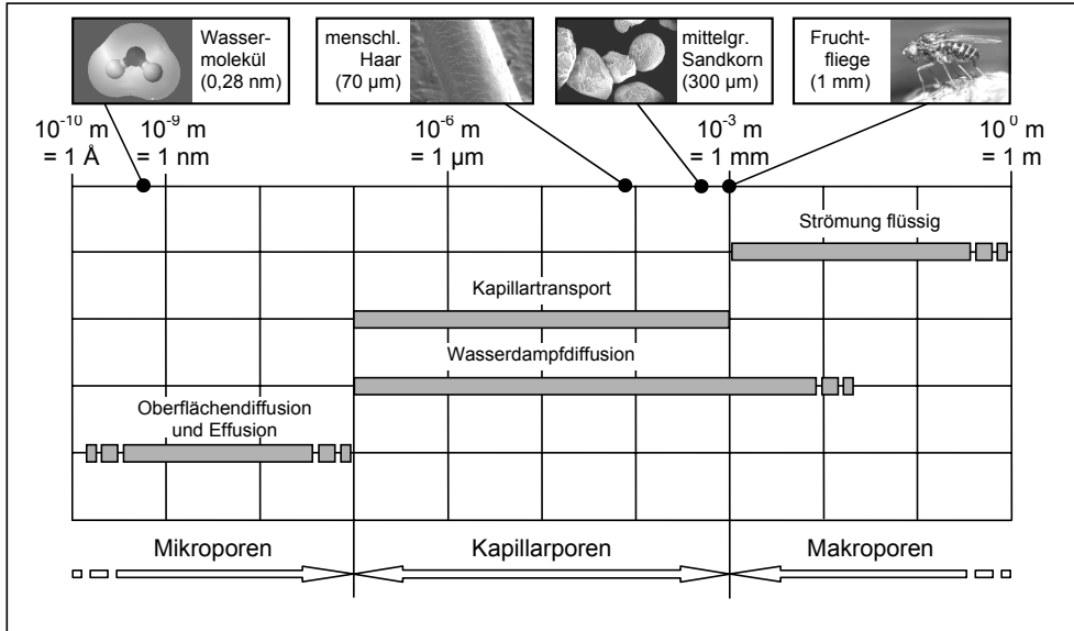
Abb. 2.6: Maßgebende Feuchtetransportmechanismen in Abhängigkeit der Porengröße (in Anlehnung an [90])
