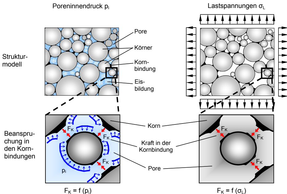
Abb. 4.27: Schematische Darstellung des Strukturmodells unter der Wirkung von Poreninnendrücken aus Eisbildung (links) und Lastspannungen (rechts)
