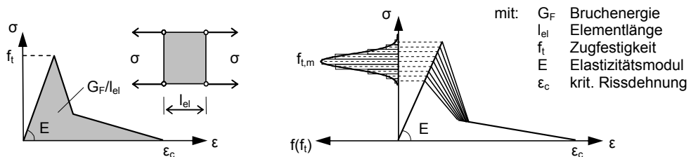
Abb. 4.5: Implementierung des Crack Band Modells (links) und Berücksichtigung der Heterogenität des Sandsteins (rechts)
