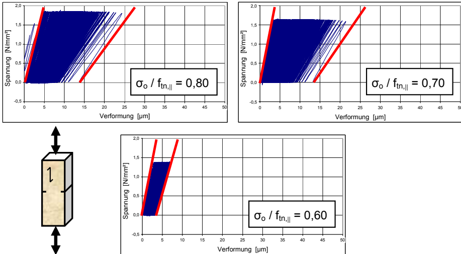
Abb. 3.30: Spannungs-Verformungsverläufe für unterschiedliche Belastungsgrade bei einer dynamischen Belastungsrichtung parallel zur Schichtungsorientierung
