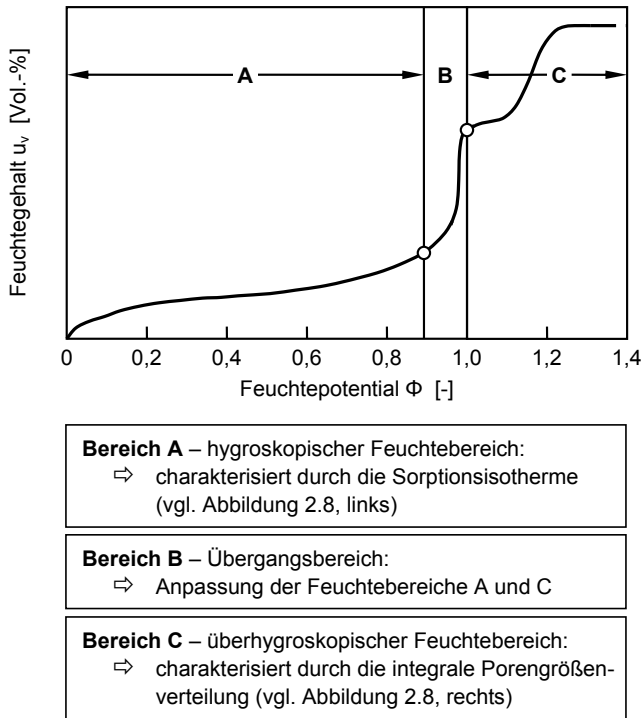
Abb. 4.1: Allgemeines Feuchtepotential nach Kießl (in Anlehnung an [74])
