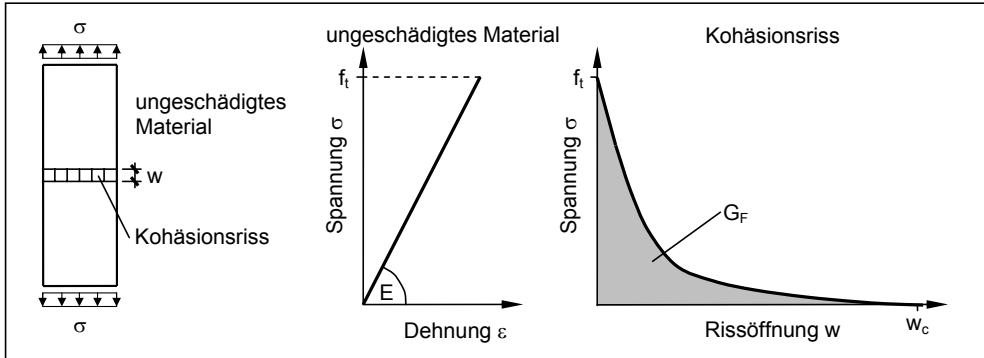
Abb. 2.12: Prinzip der Kohäsionsrissmodelle, in Anlehnung an [93]
