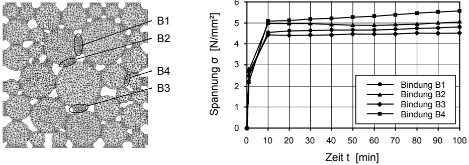
Abb. 4.37: Verlauf der mittleren Spannungen in Richtung der Kornbindungen für vier ausgewählte Kornbrücken B1 bis B4
