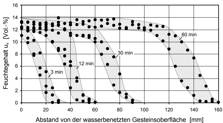
Abb. A-3.2: Mittels NMR-Spektroskopie gemessene Feuchtegehaltsverteilungen während einer einstündigen kapillaren Wasseraufnahme parallel zur Schichtungsrichtung [67]
