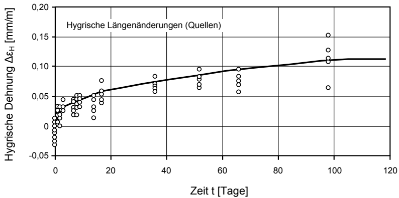
Abb. A-3.6: Messwerte der Quellversuche - hygrische Dehnungen \Delta\epsilon_H im überhygroskopischen Feuchtebereich in Abhängigkeit von der Zeit t [67]
