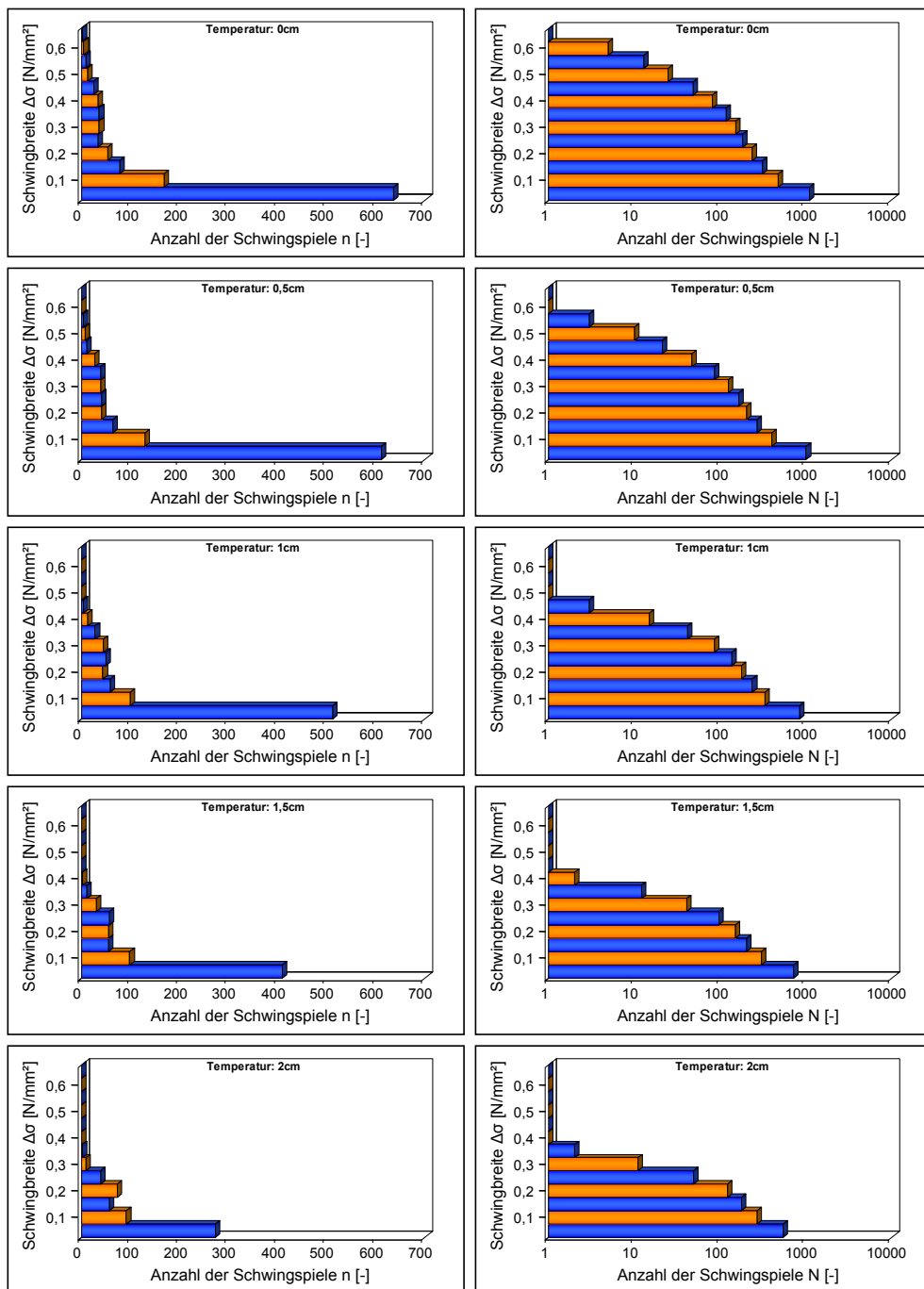
Abb. A-5.3: Stufendiagramme (links) und Spannungskollektive (rechts) der Beanspruchungen in- folge thermischer Einwirkungen in unterschiedlichen Gesteinstiefen
