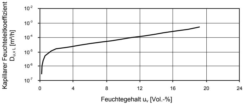
Abb. A-3.3: Experimentell ermittelter Feuchteleitfähigkeitskoeffizient für den kapillaren Flüssigkeitstransport parallel zur Schichtungsrichtung [67]
