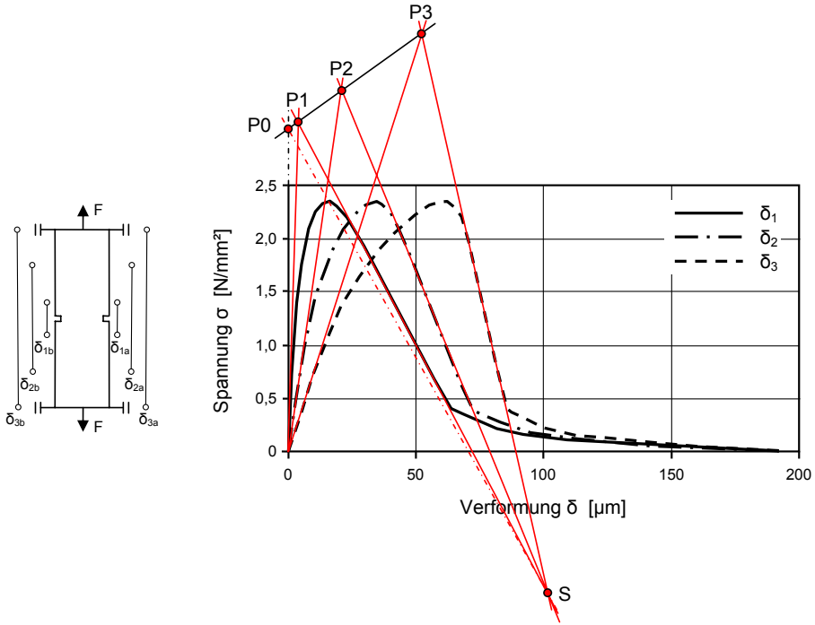
Abb. 3.22: Phänomenologische Erkenntnisse aus den Verläufen der Spannungs-Verformungsbeziehungen für unterschiedlich angeordnete Wegaufnehmer entlang der Prüfkörperlängsachse
