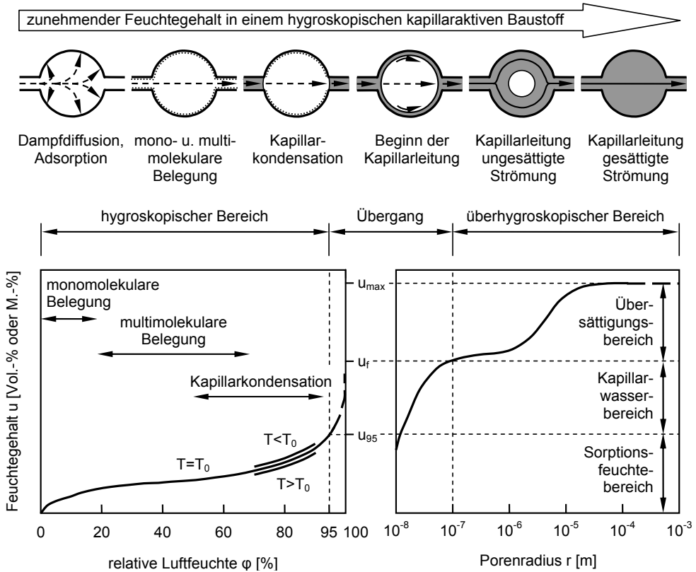
Abb. 2.8: Qualitative Darstellung des Feuchtegehaltes poröser Baustoffe in Abhängigkeit von der relativen Luftfeuchte (links) sowie in Abhängigkeit vom Porenradius (rechts) (in Anlehnung an [74])
