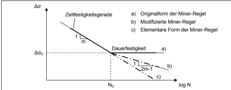
Abb. 2.19: Modifikationen der Wöhlerlinie zur Berücksichtigung von Ermüdungsbeanspruchungen unterhalb der "Dauerfestigkeit"
