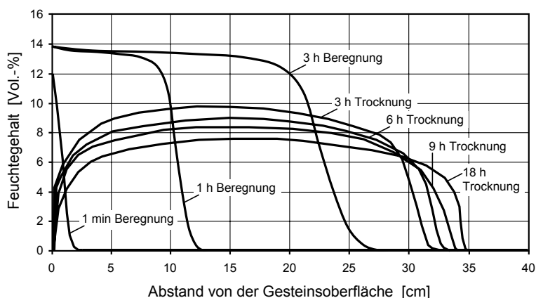
Abb. 4.7: Feuchteverteilung im Stein – 3-stündige Beregnung und daran anschließende 18-stündige Trocknung
