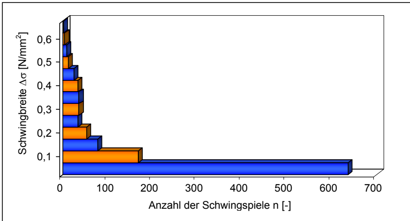
Abb. 5.4: Stufendiagramm mit den Summen der Schwingspiele für die jeweiligen Schwingbreiten an der Gesteinsoberfläche infolge thermischer Einwirkungen (Betrachtungszeitraum: 1 Jahr)
