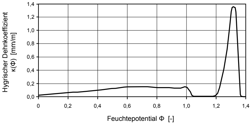
Abb. 4.4: Hygrischer Ausdehnungskoeffizient in Abhängigkeit vom Feuchtepotential für die Feuchtedehnung parallel zur Schichtung des Postaer Sandsteins der Varietät Mühlleite [153]
