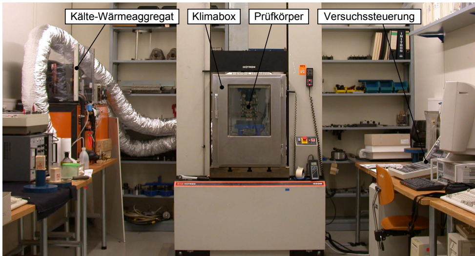
Abb. 3.19: Versuchsaufbau für die Durchführung der bruchmechanischen Untersuchungen in einer Klimabox einschließlich eines Kälte-Wärmeaggregats zur Regulierung des Prüfklimas
