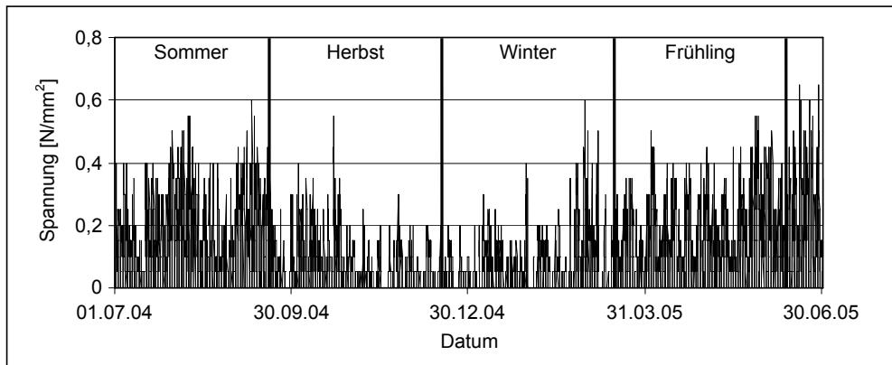
Abb. 5.1: Zugspannungs-Zeitverlauf mit gerundeten Spannungswerten an der Gesteinsoberfläche infolge jahreszeitlich wechselnder thermischer Einwirkungen
