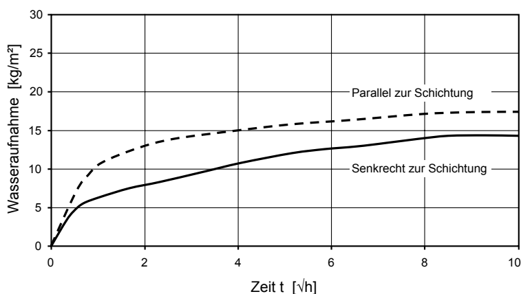
Abb. A-3.1: Untersuchungsergebnisse zur kapillaren Wasseraufnahme in Anlehnung an DIN 52 617 [27]; je Schichtorientierung Mittelwerte aus zehn Einzelmessungen [67]
