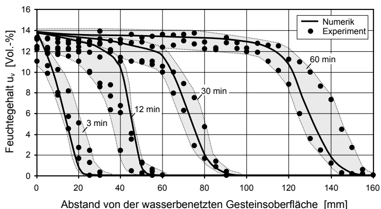
Abb. 4.9: Vergleich der experimentell gemessenen [67] und der berechneten Feuchtegehaltsverteilungen für die kapillare Wasseraufnahme parallel zur Schichtorientierung des Postaer Sandsteins der Varietät Mühlleite
