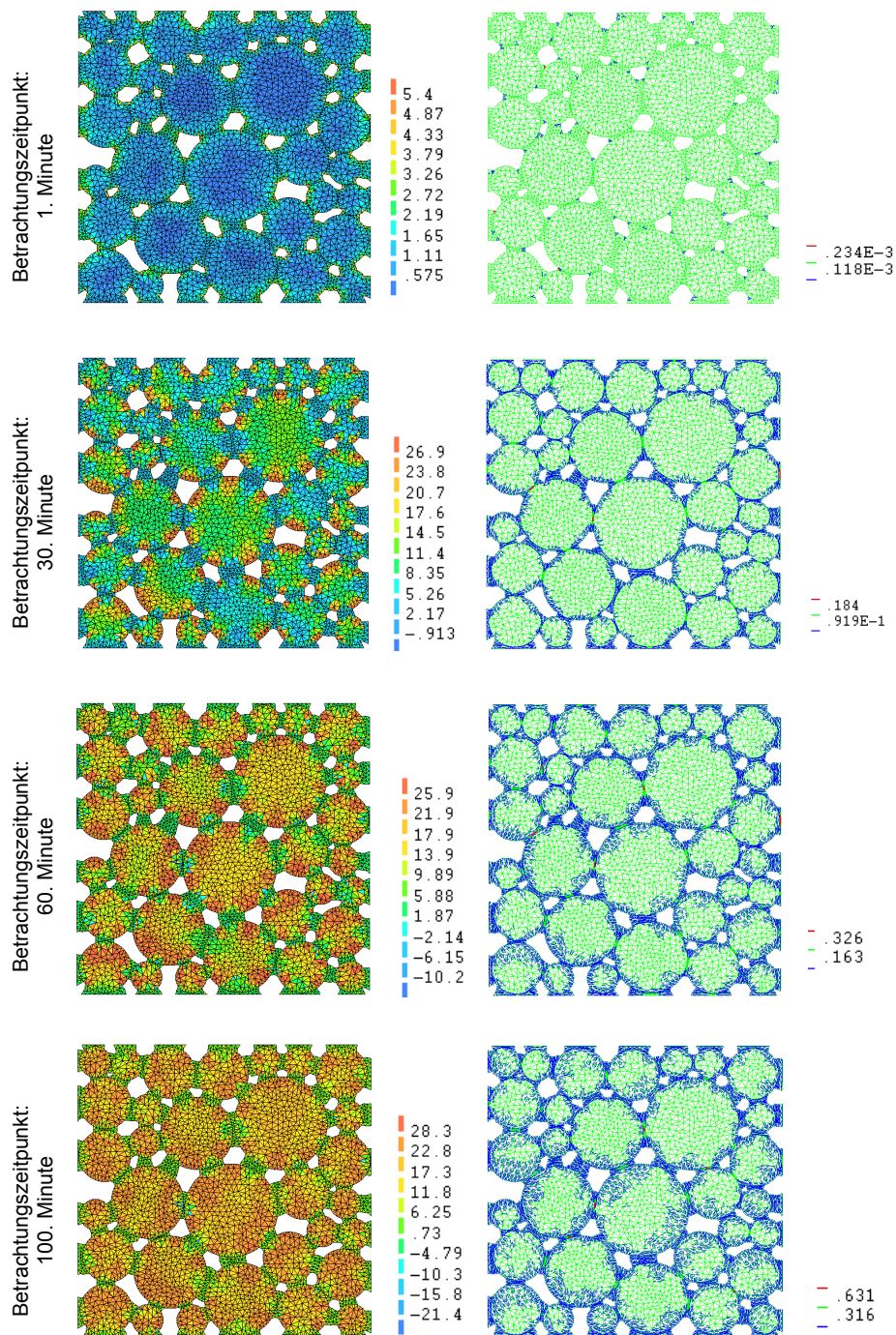
Abb. A-4.3: Entwicklung der Hauptzugspannungen \sigma_{11} [ \text{N/mm}^2 ] (links) und der Rissdehnungen \epsilon_{cr} [-] infolge einer Eisbildung bei einer Porensättigung von 98 %
