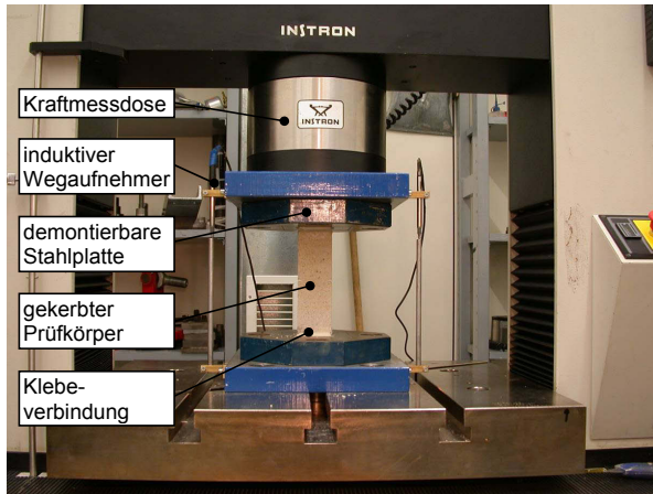
Abb. 3.16: Versuchsaufbau für die Durchführung der Zugversuche an gekerbten Prüfkörpern mit Behinderung der Prüfkörperverdrehung (starre Lagerung)
