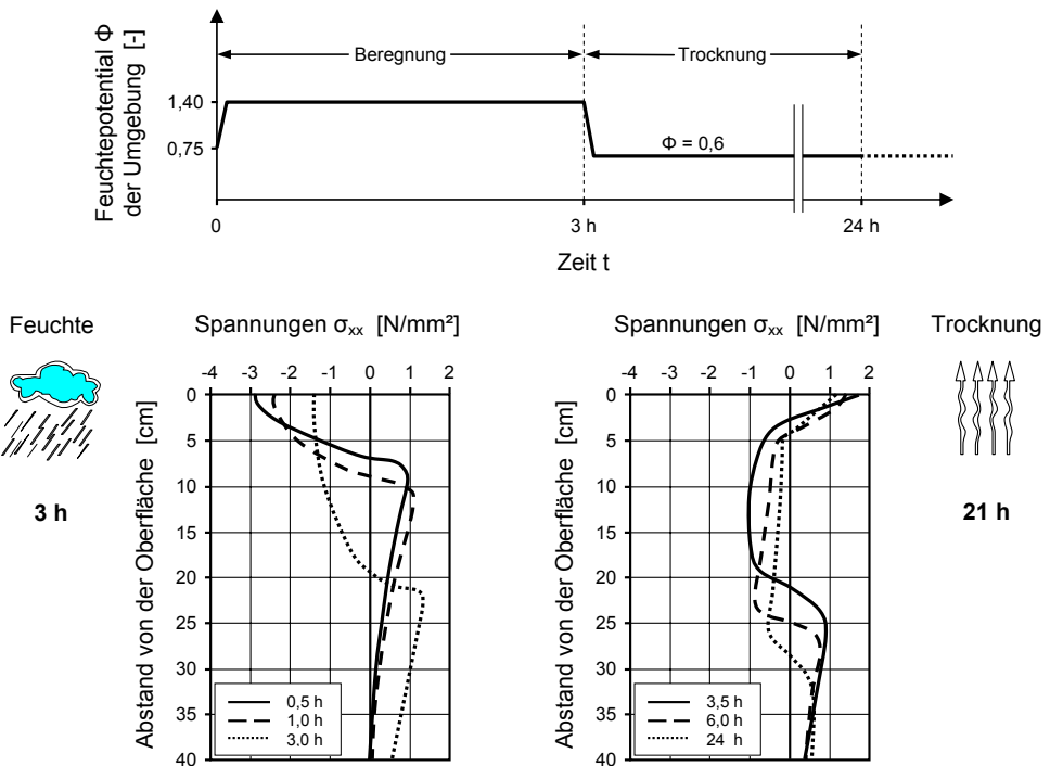
Abb. 4.8: Eigenspannungen infolge hygrischer Beanspruchung (oben); linkes Bild: während 3-stündiger Beregnung; rechtes Bild: während anschließender 21-stündiger Trocknung
