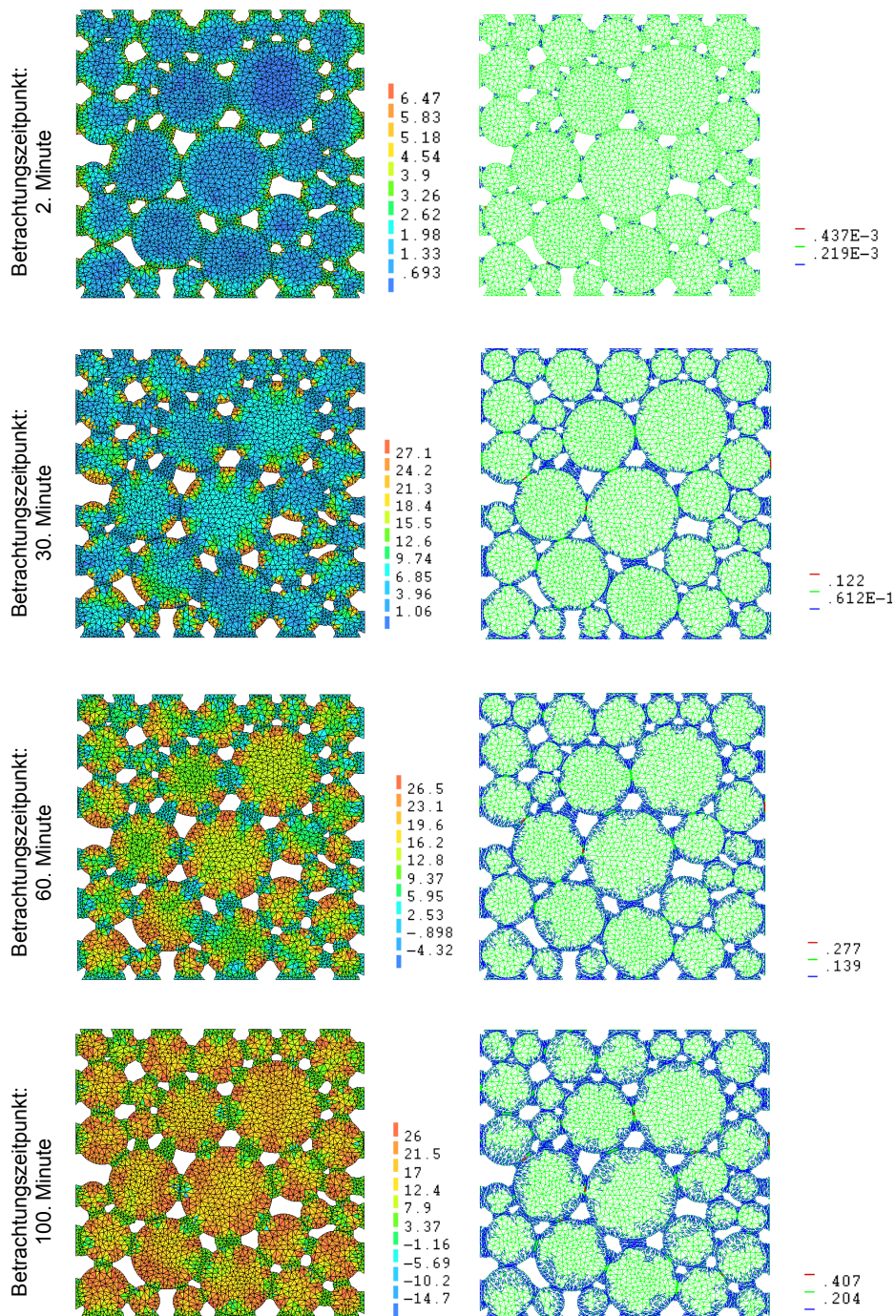
Abb. A-4.4: Entwicklung der Hauptzugspannungen \sigma_{11} [N/mm 2 ] (links) und der Rissdehnungen \varepsilon_{cr} [-] infolge einer Eisbildung bei einer Porensättigung von 96 %
