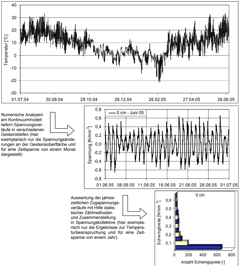
Abb. 4.10: Darstellung exemplarischer Untersuchungsergebnisse am Kontinuummodell
