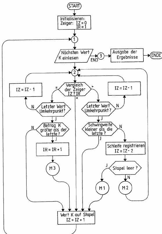
Abb. A-5.1: Ablaufschema des Algorithmus nach [12] zur Auswertung von Beanspruchungs-Zeitverläufen nach dem Rainflow-Zählverfahren
