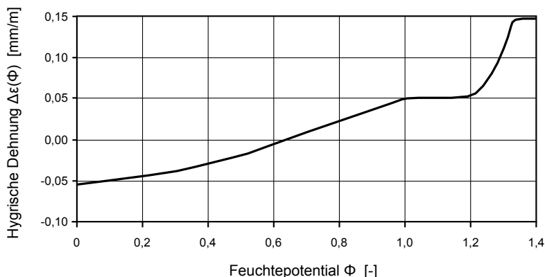
Abb. 4.3: Überlagerte hygri- sche Dehnfunktion in Abhängigkeit vom Feuchtepotential für die Feuchtedehnung parallel zur Schichtung des Postaer Sandsteins der Varietät Mühlleite [67]
