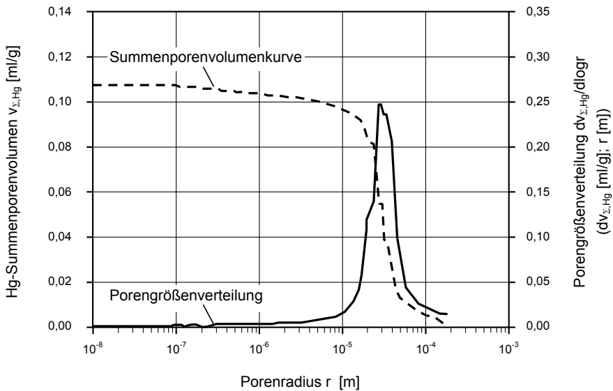
Abb. 3.3: Porengrößenverteilung und Summenporenvolumenkurve für das untersuchte Sandsteinmaterial (Postaer Sandstein der Gesteinsvarietät Mühlleite)
