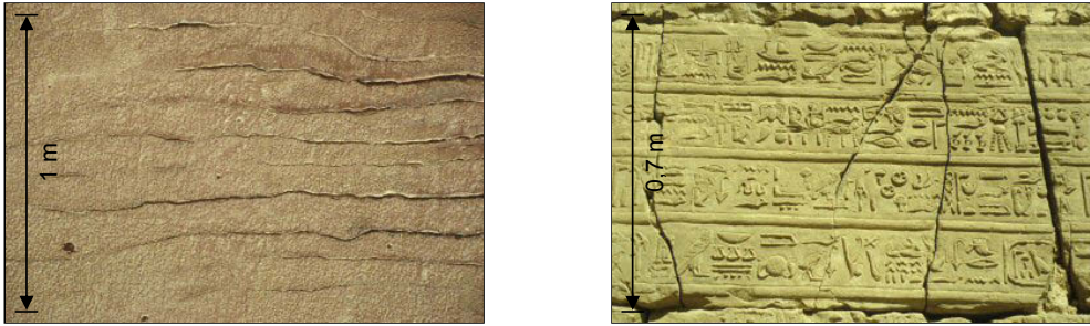
Abb. 2.24: Schichtparallele (links) und ungerichtete Rissbildungen (rechts) in Sandsteinen [44]
