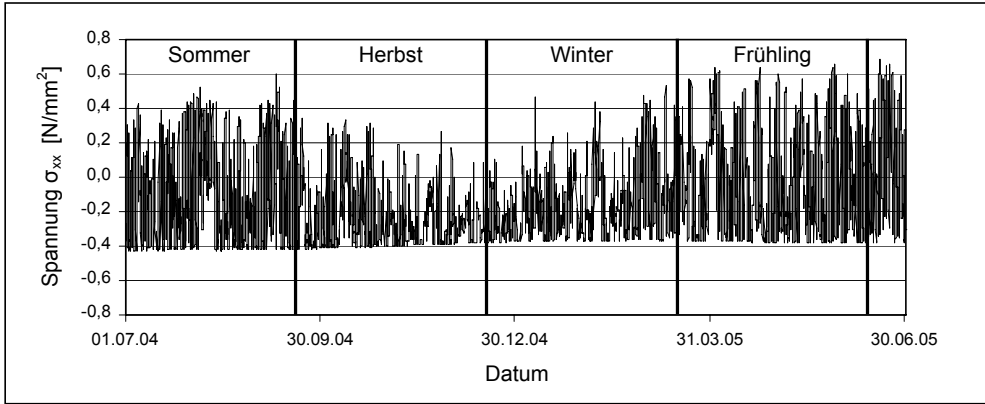
Abb. 4.22: Jahreszeitlicher Verlauf der hygrysch induzierten Spannungen an der Gesteinsoberfläche
