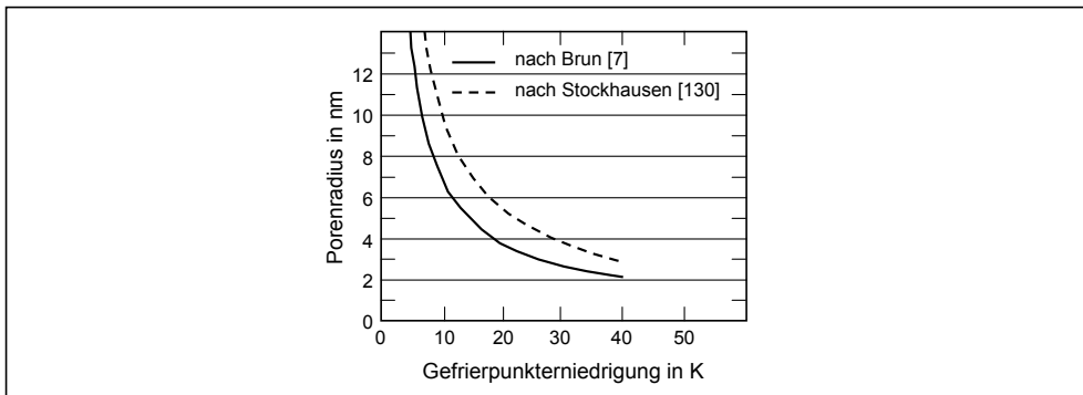
Abb. 2.22: Radiusgefrierpunktbeziehung für zylindrische Poren [137]
