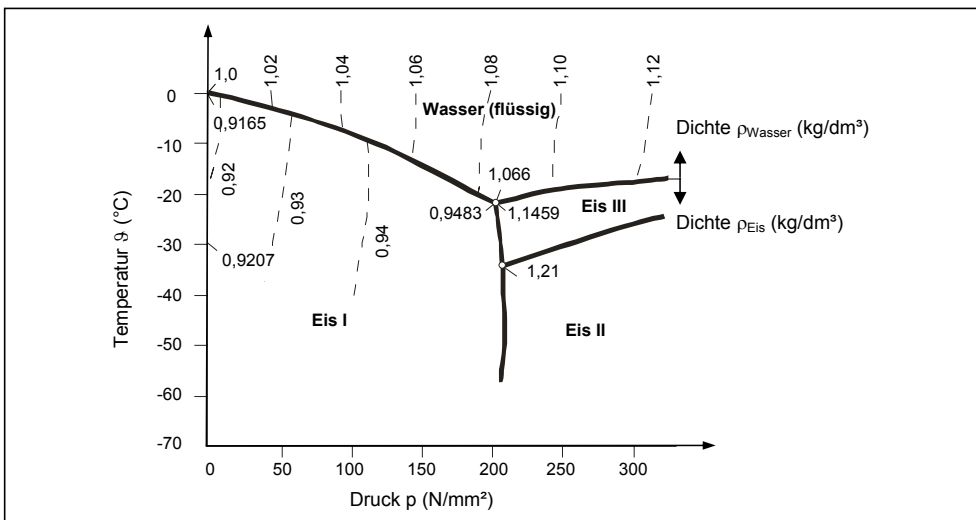
Abb. 2.21: Druck-Temperatur-Dichte-Diagramm der Phasen Wasser und Eis [151]
