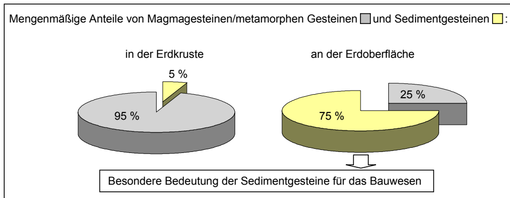
Abb. 2.2: Mengenmäßige Gesteinsvorkommen und die hieraus resultierende Bedeutung für das Bauwesen
