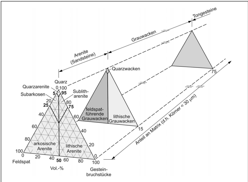
Abb. 2.4: Klassifikation der Sandsteine nach [111], (Angaben in Vol.-%)
