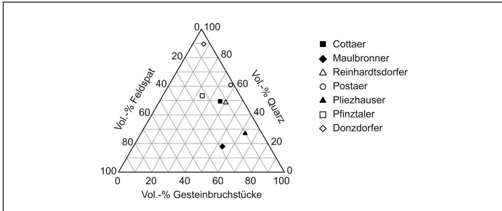
Abb. 2.5: Lage der Sandsteine im Dreistoffdiagramm (Angaben in Vol.-%) [105]
