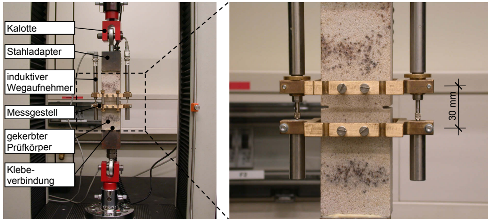
Abb. 3.13: Versuchsaufbau für die Durchführung der Zugversuche an gekerbten Prüfkörpern ohne Behinderung der Prüfkörperverdrehung (gelenkige Lagerung)
