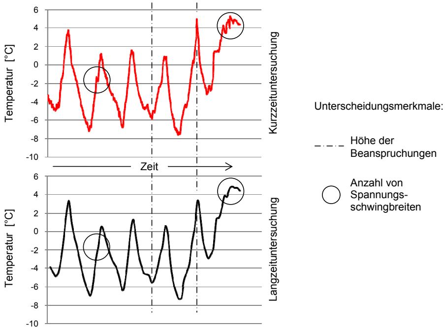
Abb. 4.25: Qualitativer Vergleich der Temperaturverläufe an der Gesteinsoberfläche; oben: aus Kurzzeituntersuchung, unten: aus Langzeituntersuchung
