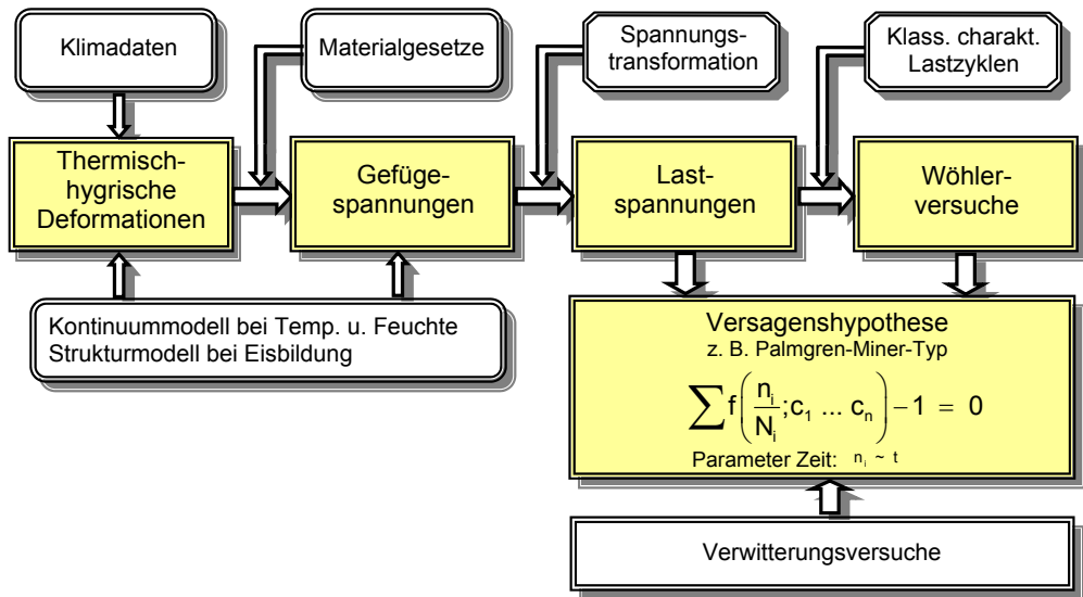
Abb. 1.1: Konzept zur Entwicklung eines Prognosemodells
