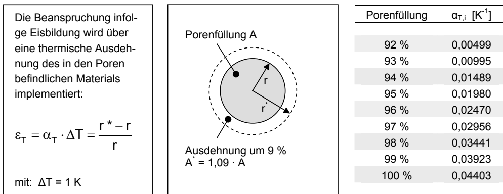
Abb. 4.32: Implementierung der Beanspruchung infolge Eisbildung unter Berücksichtigung unterschiedlicher Porenfüllgrade (in Anlehnung an [30, 146])
