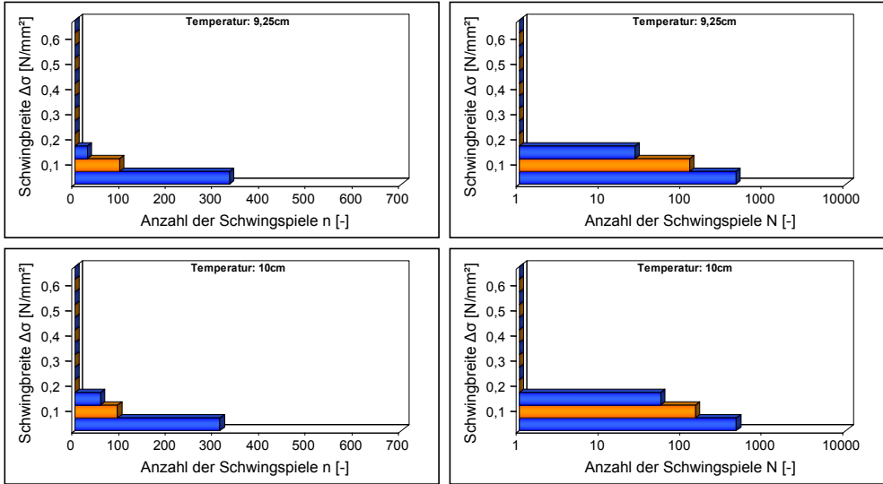
Abb. A-5.6: Stufendiagramme (links) und Spannungskollektive (rechts) der Beanspruchungen infolge thermischer Einwirkungen in unterschiedlichen Gesteinstiefen
