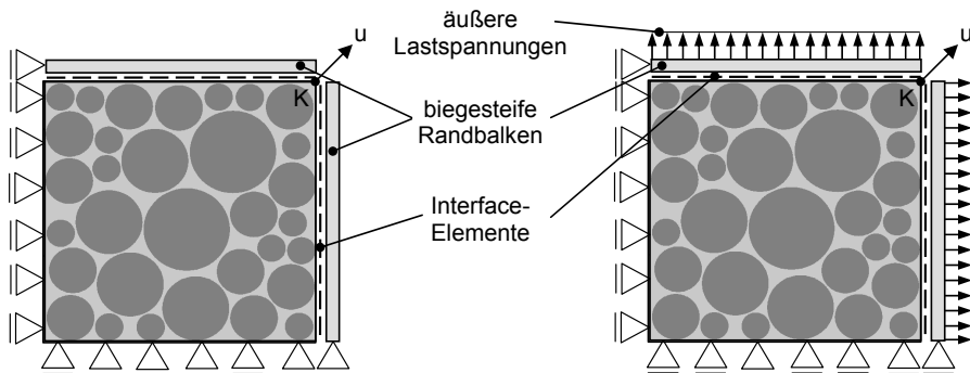
Abb. 4.33: Aufbau des Strukturmodells zur Modellierung der Eisbildung im Porenraum (links) sowie zur Modellierung der äußeren Lastspannungen (rechts)
