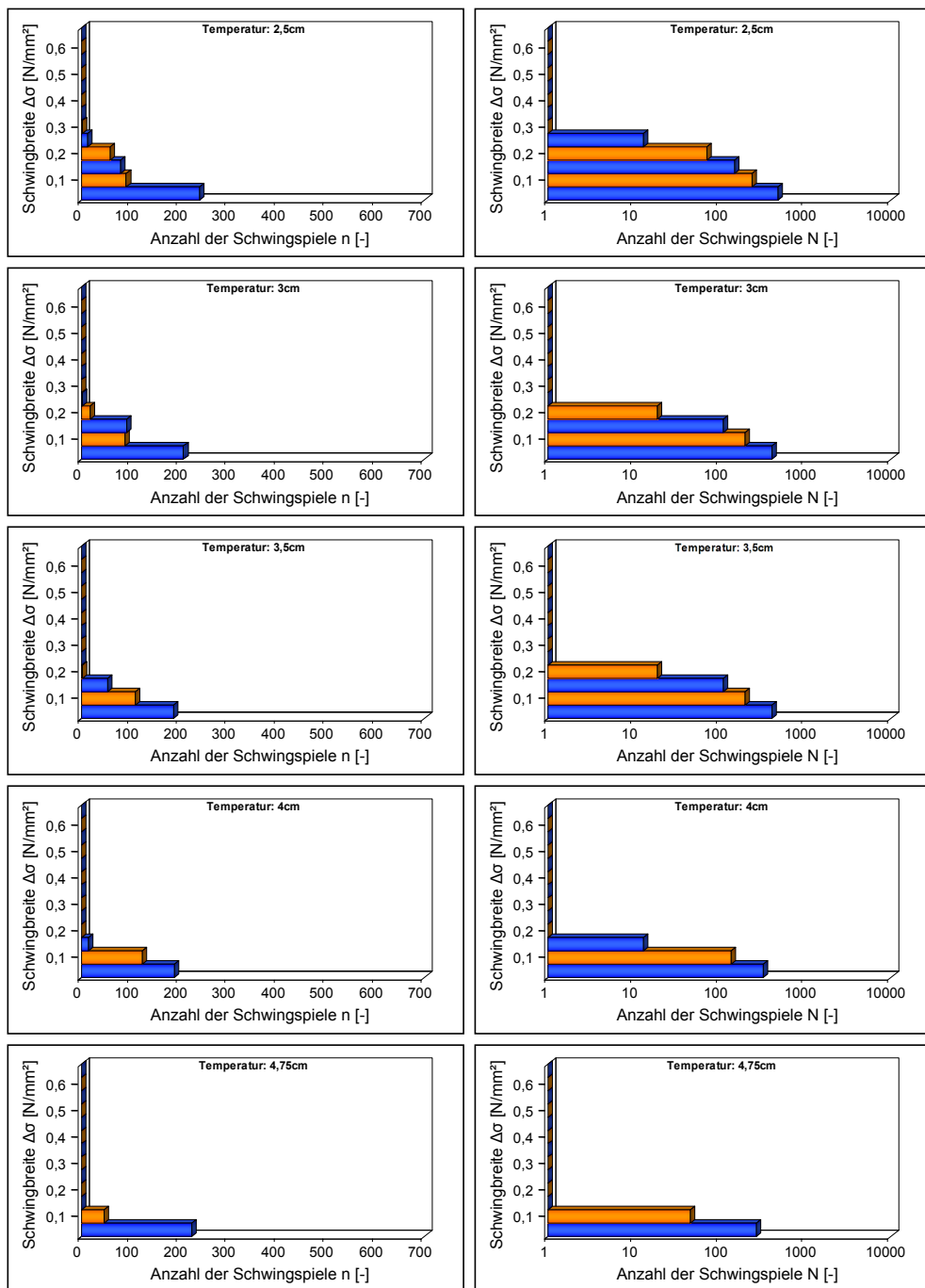
Abb. A-5.4: Stufendiagramme (links) und Spannungskollektive (rechts) der Beanspruchungen in- folge thermischer Einwirkungen in unterschiedlichen Gesteinstiefen
