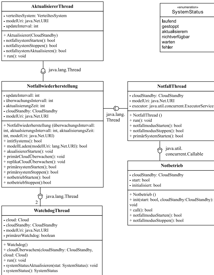
Abbildung 72: Klassendiagramm der Notfallwiederherstellungskomponente
