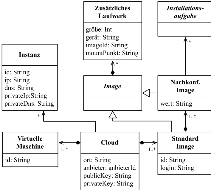
Abbildung 117: MOF Klassendiagramm des Infrastruktur-Pakets (vgl. [84])
