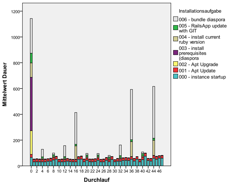
Abbildung 93: Applikationsserver Deploymentzeiten (mit Cloud Standby)
