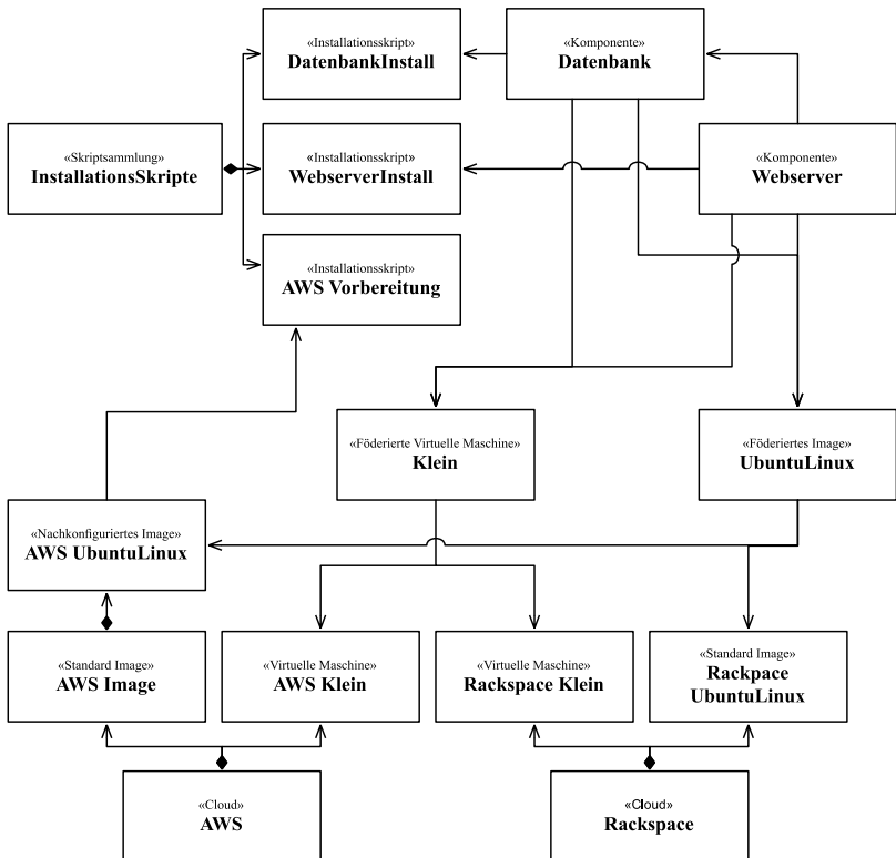
Abbildung 56: Beispielmodell für die föderierte Infrastruktur-Beschreibung basierend auf der Cloud Standby Beschreibungssprache
