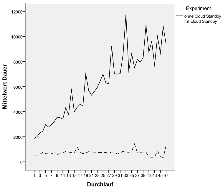
Abbildung 105: Vergleich der Deploymentzeiten über die Zeit (vgl. [86])
