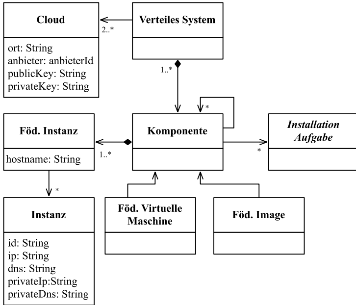
Abbildung 119: MOF Klassendiagramm des Verteiltes-System-Pakets (vgl. [84])
