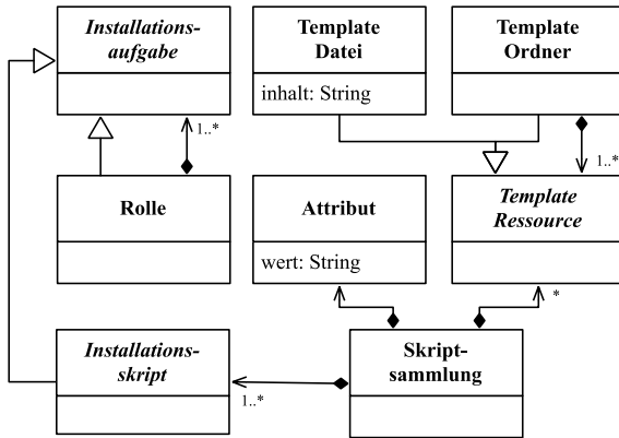
Abbildung 51: MOF Classendiagramm des Software-Paketes
