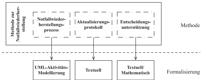
Abbildung 30: Formalisierung der Notfallwiederherstellungsmethode
