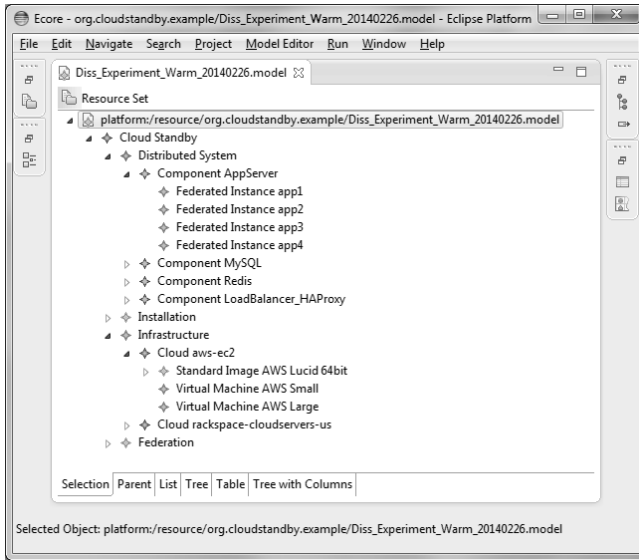
Abbildung 67: Beispielhafte Darstellung eines Modells im Cloud Standby Modell Editor
