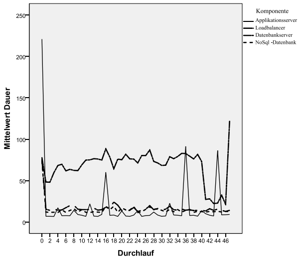
Abbildung 91: Vergleich der Deploymentzeiten nach Komponente
