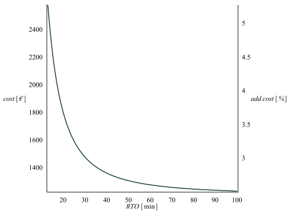
Abbildung 100: Absolute Kosten und prozentuale zusätzliche Kosten für Cloud Standby in Bezug auf das RTO
