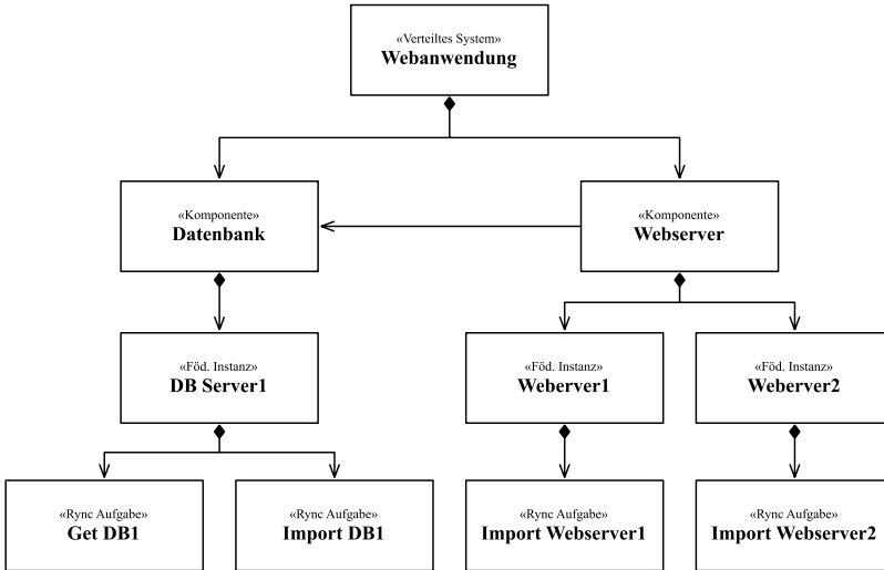
Abbildung 57: Beispielmodell für die Verteiltes System Beschreibung basierend auf der Cloud Standby Beschreibungssprache
