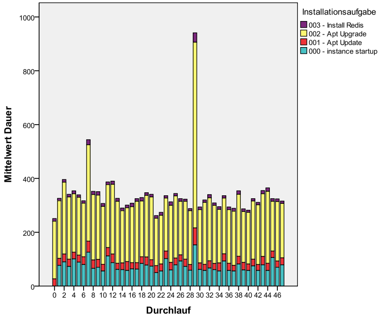
Abbildung 85: NoSQL Datenbankservers Deploymentzeiten (ohne Cloud Standby)
