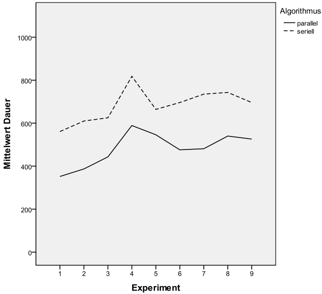
Abbildung 96: Einfluss des parallelen Deployments auf das RTO
