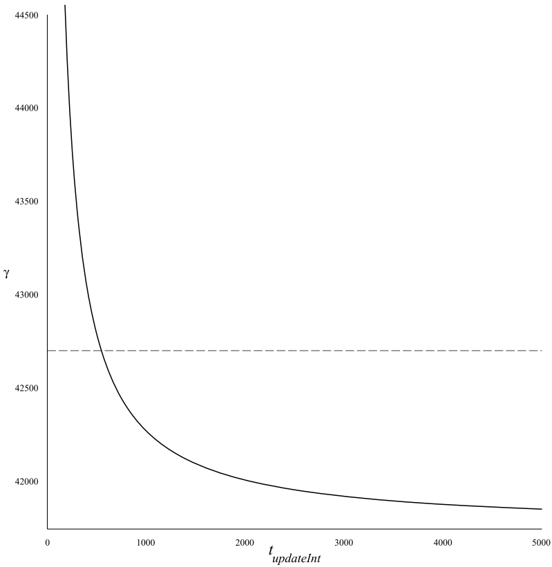
Abbildung 104: Kostenentwicklung bei steigendem Backup-Intervall (schwarze Kurve: \gamma_{1,400} , graue gestrichelte Gerade: \gamma_{2,400} , vgl [84], [85])
