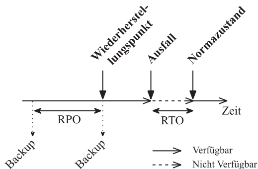
Abbildung 11: RPO und RTO im IT-Kontext (vgl. [86])
