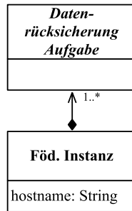
Abbildung 120: Metamodell des Datenrücksicherung-Pakets
