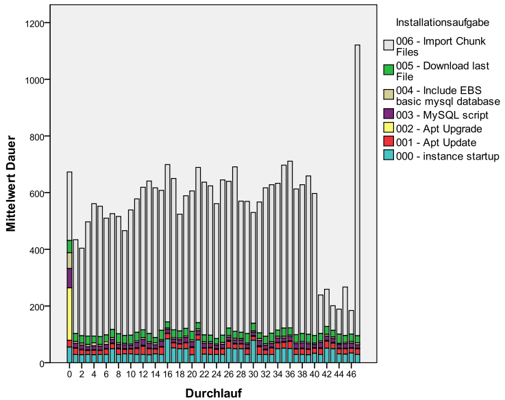
Abbildung 92: Datenbankserver Deploymentzeiten (mit Cloud Standby)
