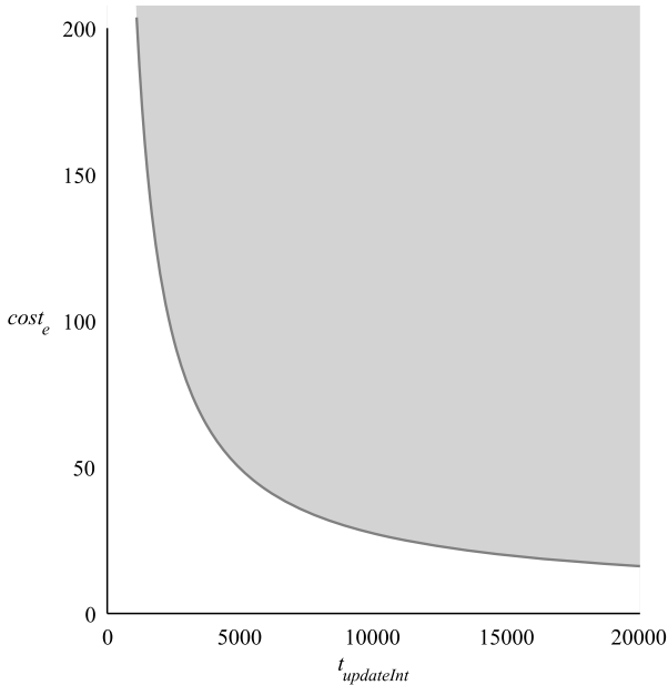
Abbildung 109: t_{updateInt} und cost_e Kombinationen, in denen das Replikationssystem günstiger (grauer Bereich) ist, gleich viel kostet (graue Linie) und teurer ist (weißer Bereich) (vgl. [84]–[86])
