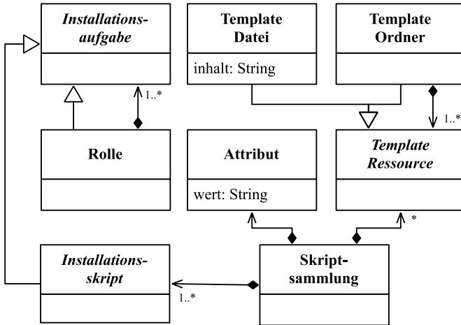
Abbildung 115: MOF Klassendiagramm des Software-Pakets
