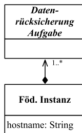
Abbildung 55: Metamodell des Datenrücksicherung-Paketes
