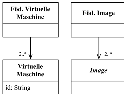
Abbildung 118: MOF Klassendiagramm des Föderation-Pakets (vgl. [84])
