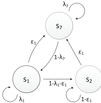
Abbildung 43: Markov-Kette ohne Cloud Standby ( MK_2 ) [84], [85]
