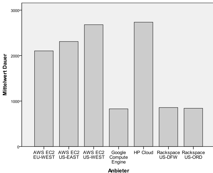
Abbildung 107: Vergleich der Deploymentzeiten des initialen Deployments bei verschiedenen Anbietern
