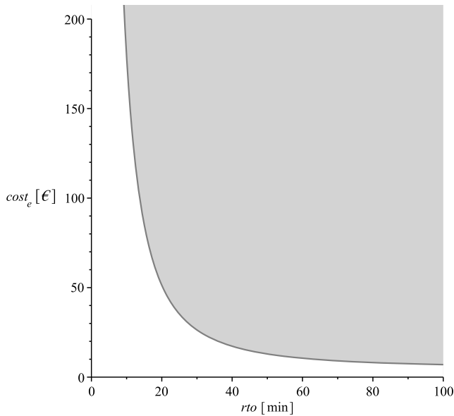
Abbildung 110: Vergleich von RTO und Ausfallkosten ( cost_e ) mit Kombinationen, in denen sich der Einsatz von Cloud Standby lohnt (grau)
