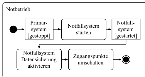
Abbildung 32: Aktivität „Notbetrieb starten“ (vgl. [86])
