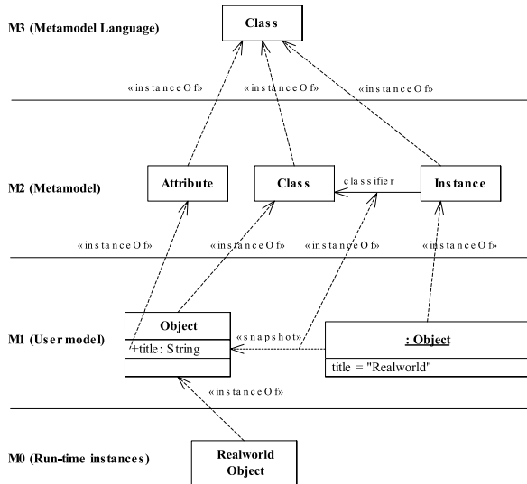
Abbildung 20: MaOF Metamodellierungshierarchie [108]
