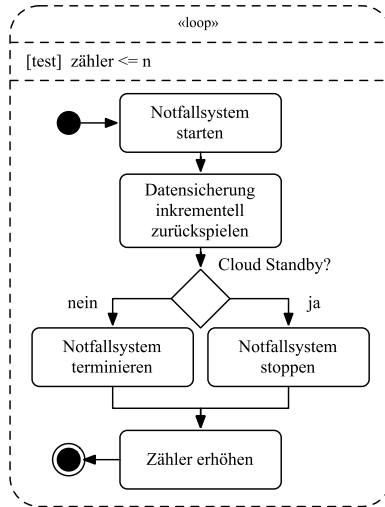
Abbildung 77: Experimentablauf
