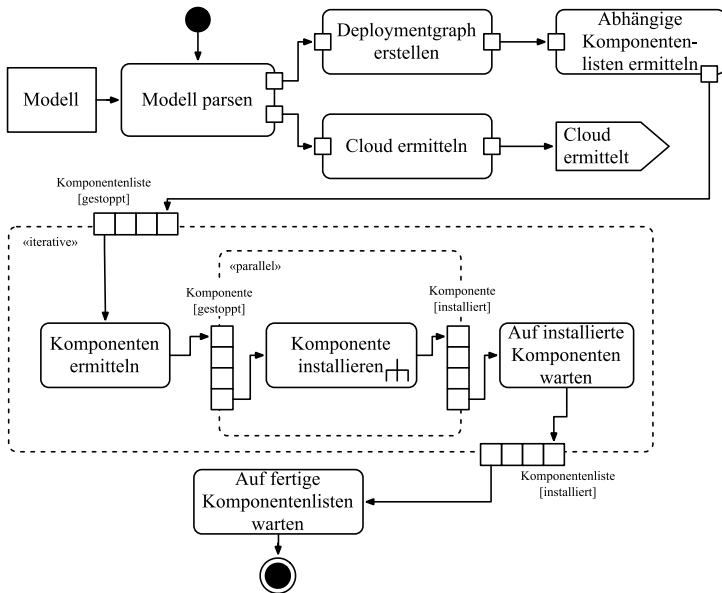
Abbildung 58: Gesamter Deploymentprozess
