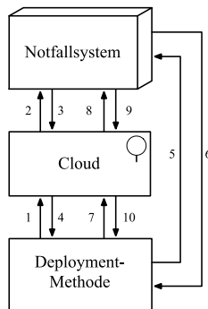
Abbildung 62: Deployment Protokoll
