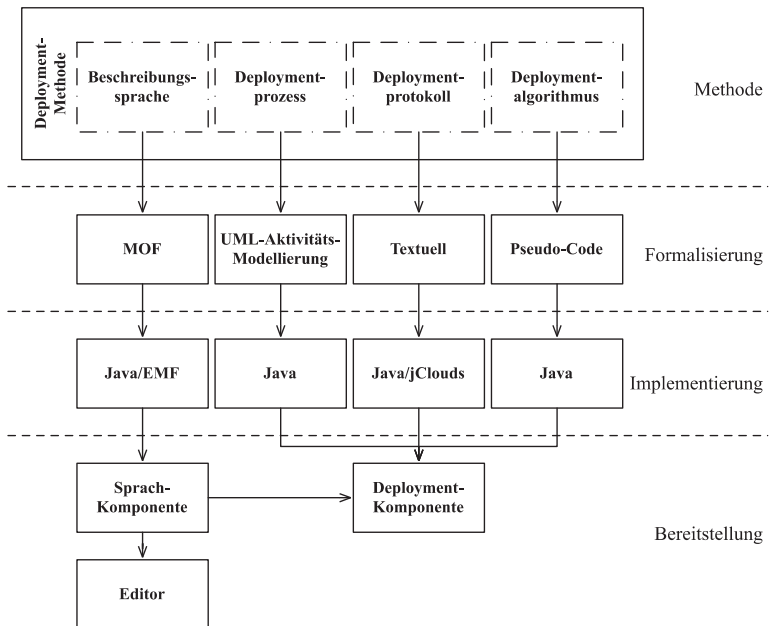
Abbildung 6: Übersicht über die Deployment-Methode und deren Umsetzung in dieser Arbeit
