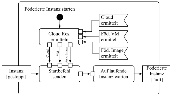
Abbildung 60: Subprozess Föderierte Instanz starten
