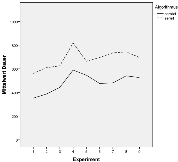
Abbildung 106: Einfluss des parallelen Deployments auf das RTO
