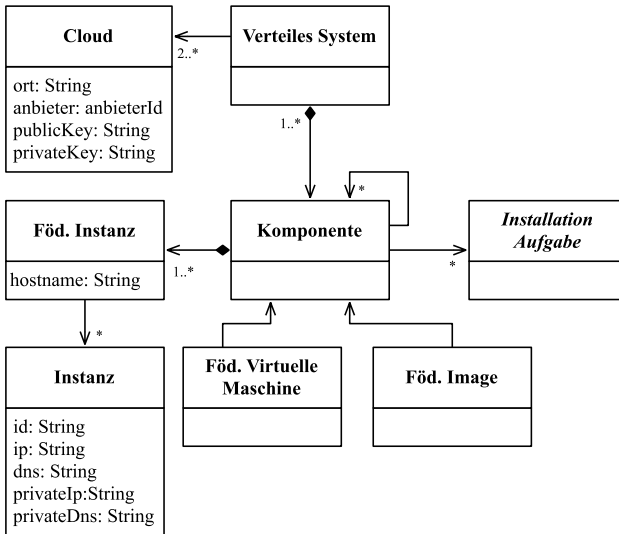
Abbildung 54: MOF Klassendiagramm des Verteiltes-System-Pakets (vgl. [84])
