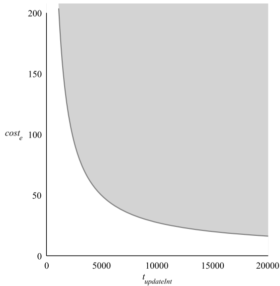
Abbildung 103: t_{updateInt} und cost_e Kombinationen, in denen das Replikationssystem günstiger (grauer Bereich) ist, gleich viel kostet (graue Linie) und teurer ist (weißer Bereich) (vgl. [84]–[86])
