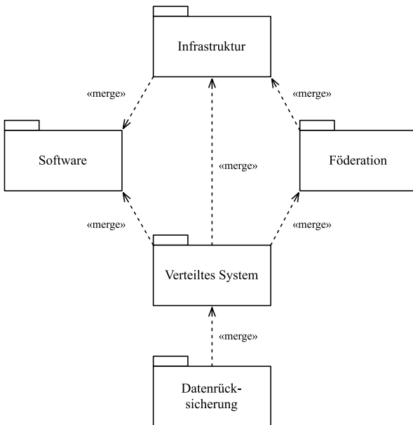
Abbildung 50: Die Beschreibungssprache als Paketdiagramm
