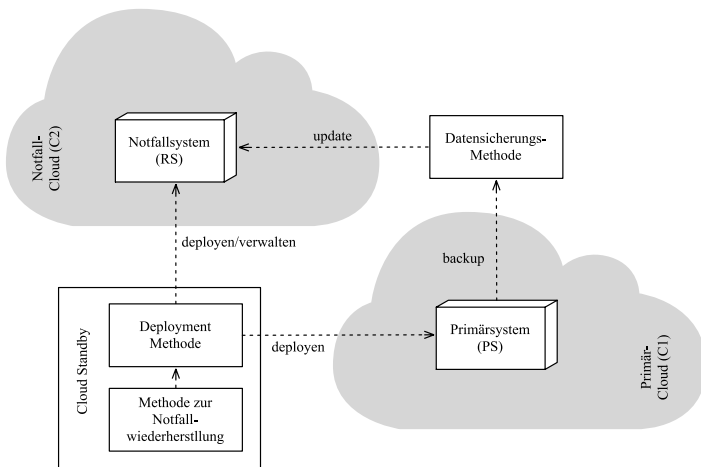
Abbildung 45: Deployment-Methode im Zusammenspiel der Methoden (vgl. [86])
