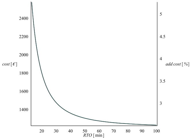
Abbildung 108: Absolute Kosten (cost) und prozentuale zusätzliche Kosten (add cost) für Cloud Standby in Bezug auf das RTO
