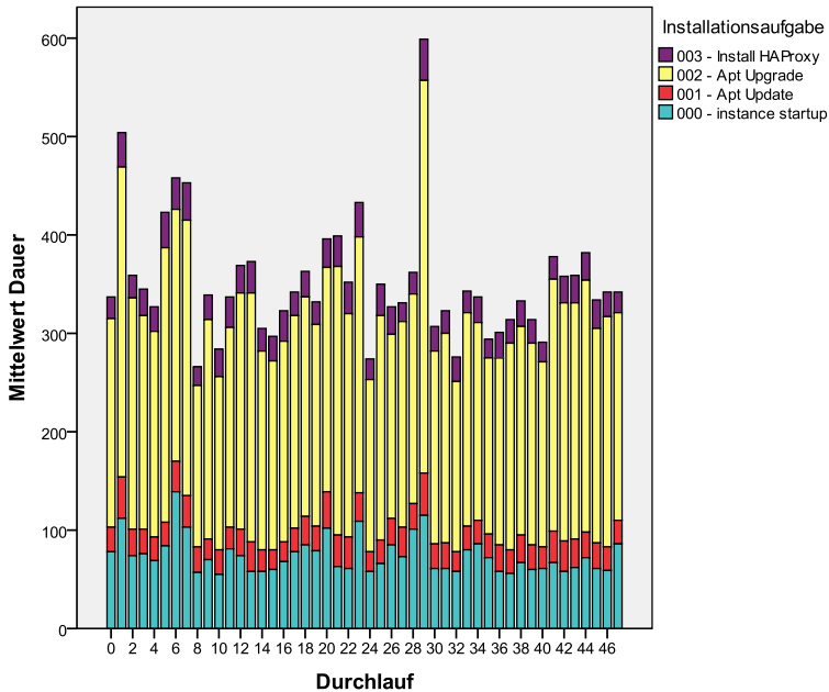
Abbildung 84: Loadbalancer Deploymentzeiten (ohne Cloud Standby)
