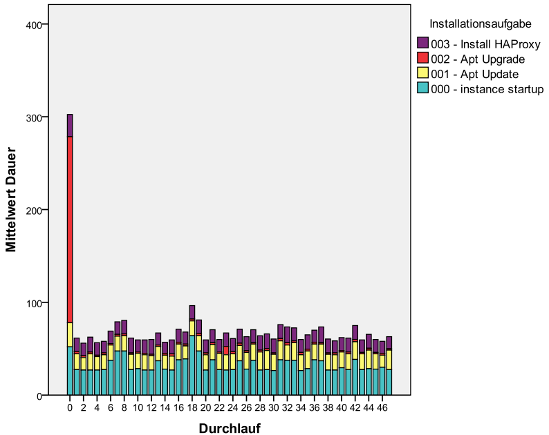
Abbildung 94: Loadbalancer Deploymentzeiten (mit Cloud Standby)
