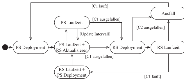
Abbildung 28: Cloud Standby Systemzustände (vgl. [86])
