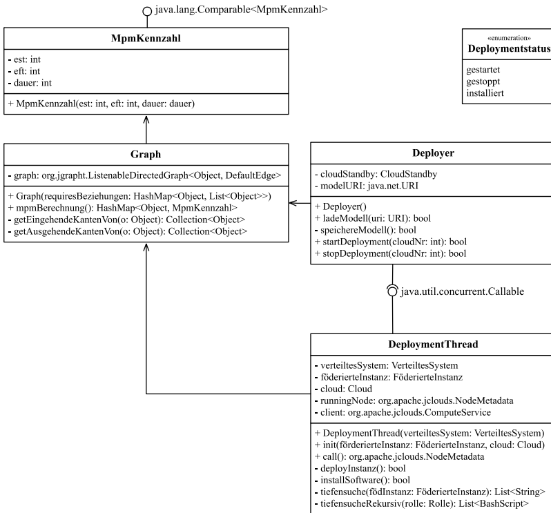
Abbildung 71: Klassendiagramm der Deploymentsteuerung
