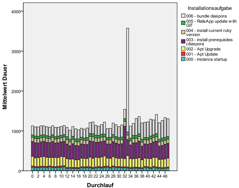
Abbildung 83: Applikationsserver Deploymentzeiten (ohne Cloud Standby)
