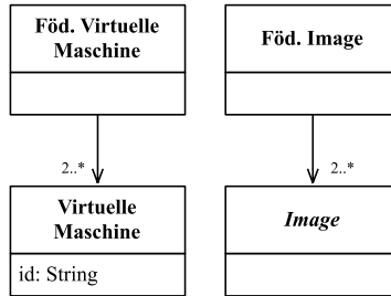
Abbildung 53: MOF Klassendiagramm des Föderation-Pakets (vgl. [84])
