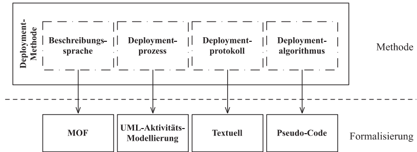
Abbildung 46: Formalisierung der Modellbasierten Deployment-Methode
