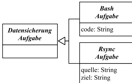
Abbildung 121: Konkretisierung der abstrakten Datensicherung Aufgabe in der Implementierung
