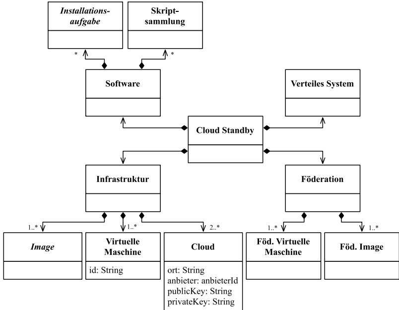
Abbildung 68: Sprach-Erweiterungen für den Editor
