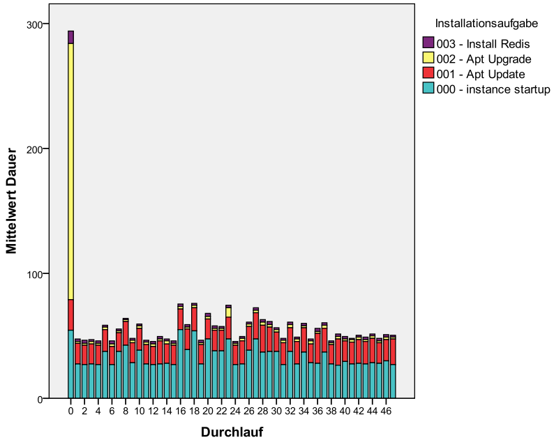
Abbildung 95: NoSQL Datenbankserver Deploymentzeiten (mit Cloud Standby)
