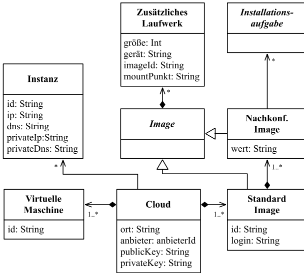
Abbildung 52: MOF Klassendiagramm des Infrastruktur-Pakets (vgl. [84])
