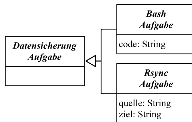
Abbildung 70: Konkretisierung der abstrakten Datensicherung Aufgabe in der Implementierung
