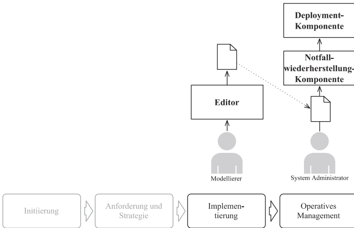
Abbildung 7: Erstellung und Nutzung der Deploymentbeschreibung
