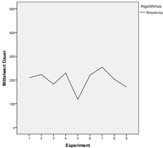
Abbildung 97: Einsparungen in der Deploymentzeit durch die Modellierung
