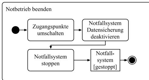
Abbildung 33: Aktivität „Notbetrieb beenden“
