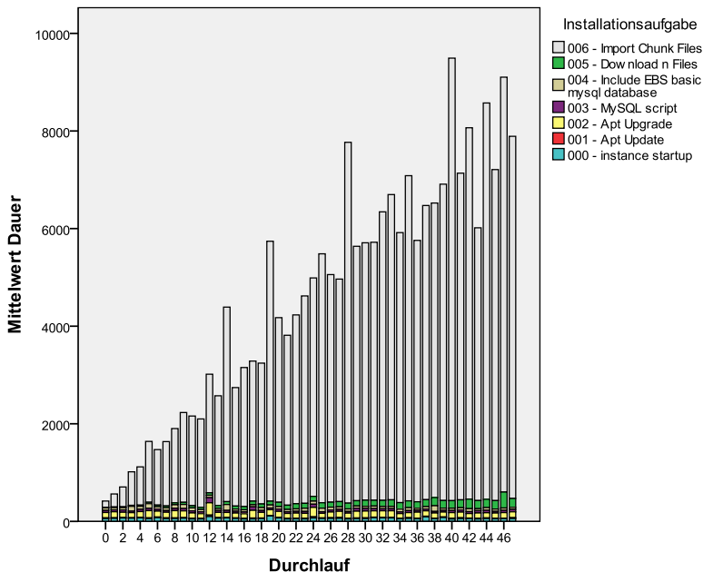
Abbildung 82: Datenbankserver Deploymentzeiten (ohne Cloud Standby)
