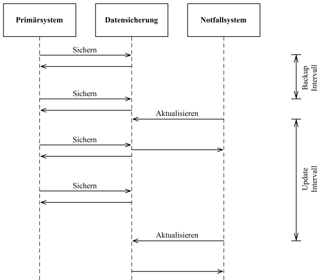
Abbildung 29: Exemplarische Darstellung des Nicht-Zusammenhangs des Update- und Backup-Intervalls als UML Sequenzdiagramm (vgl. [86])
