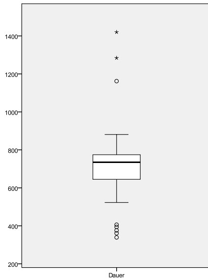
Abbildung 87: Verteilung der Deploymentzeiten mit Cloud Standby
