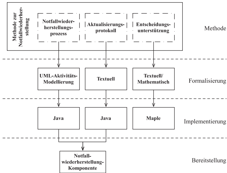
Abbildung 5: Übersicht über die Methode zur Notfallwiederherstellung und die Umsetzung in dieser Arbeit
