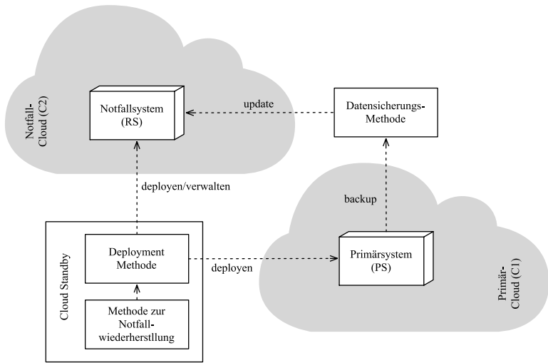
Abbildung 3: Zusammenspiel der Komponenten und Methoden (vgl. [86])
