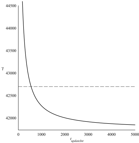
Abbildung 40: Beispielhafte Darstellung der Gesamtkosten mit (durchgezogene Linie) und ohne Absicherung (gestrichelte Linie) und dem kostenneutralen Update-Intervall im Schnittpunkt
