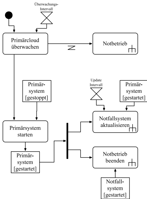
Abbildung 31: Notfallwiederherstellungsprozess (vgl. [86])
