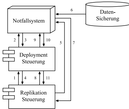
Abbildung 35: Aktualisierungsprotokoll
