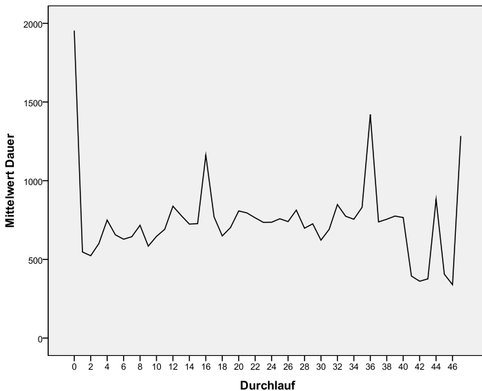
Abbildung 86: Entwicklung der Deploymentzeit mit Cloud Standby bei voranschreitender Alterung der Daten
