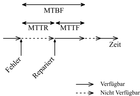
Abbildung 14: Übersicht über MTBF, MTTR und MTTF
