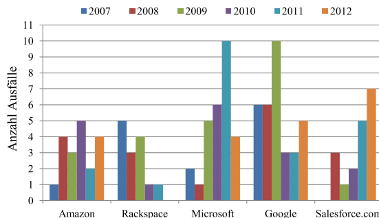
Abbildung 19: Ausfallverteilung über Anbieter und Jahre [88]
