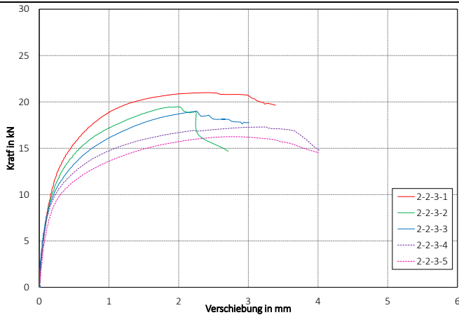
Bild A-11 Last-Verformungsdiagramm Reihe 2-2-3
