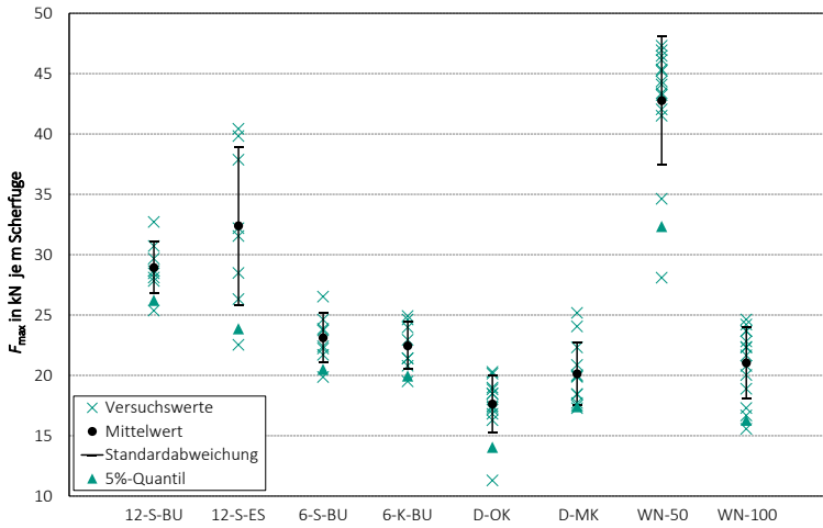
Bild 5-13 Versuchswerte und statistische Kennwerte der Höchstlast F_{max}
