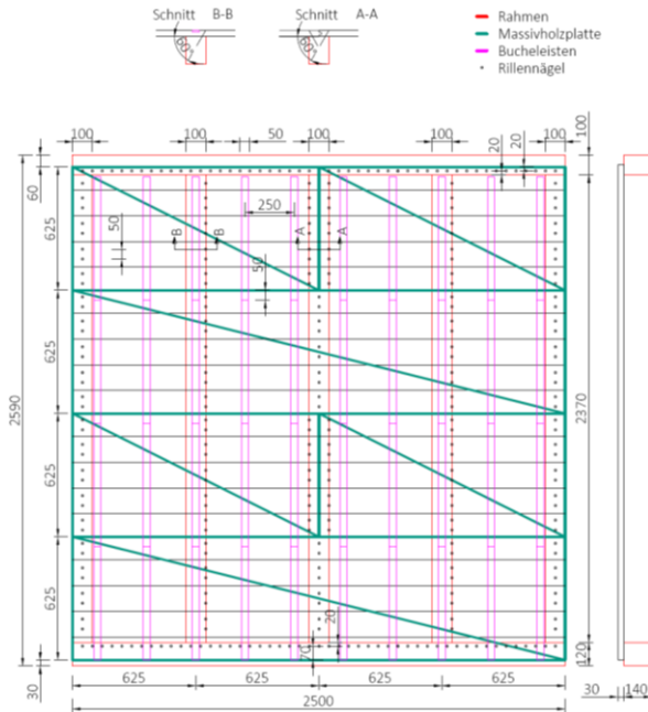
Bild 7-1 Konstruktionszeichnung Tafелеlement Reihe BLH; Maße in mm
