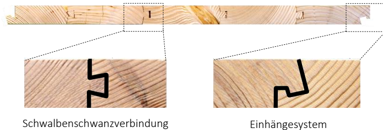
Bild 1-3 Klebstofffreie Massivholzplatte und Details
