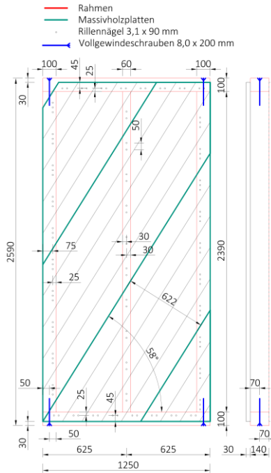
Bild 7-4 Konstruktionszeichnung Tafelement Reihe OVDS-Z, OVDS-D bzw. OVDS-DZ; Maße in mm
