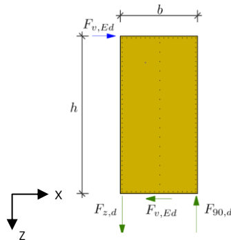
Bild 8-5 Kräfte bei horizontaler Belastung; Quelle: Vogt und Seim (2014)
