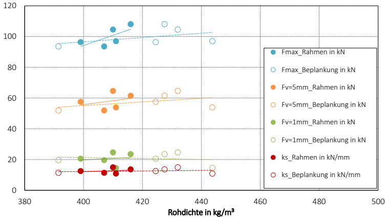
Bild 6-14 Versuchsergebnisse der Reihe Z2 in Abhängigkeit der Rohdichte
