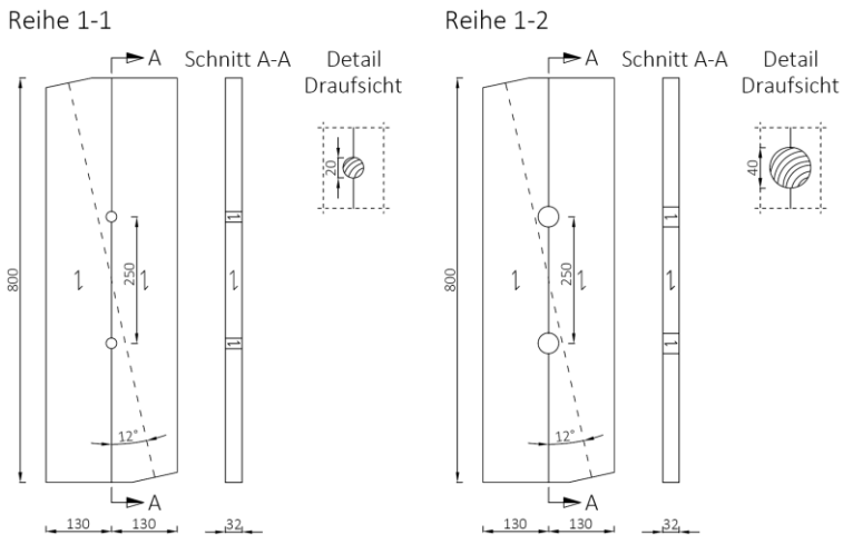
Bild 4-4 Prüfkörpergeometrie und Details für die Reihe 1
