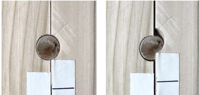
Bild 5-8 Dübelverbindung mit ausmittiger Anordnung vor und nach Versuchsdurchführung
