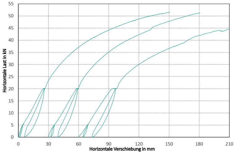
Bild A-22 Last-Verformungsdiagramme Reihe BLH
