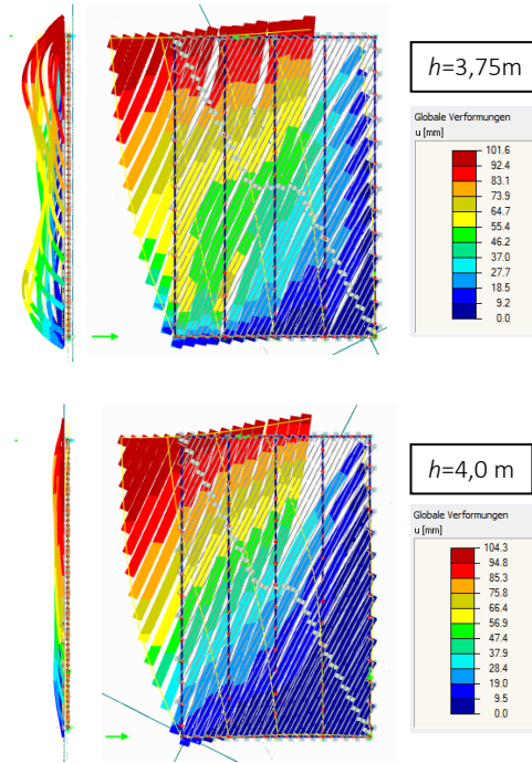
Bild 8-42 Verformungsfiguren bei v=100\text{ mm} der Modelle h=3,75\text{ m} (oben) und h=4,0\text{ m} (unten), Ansichten jeweils in x -Richtung (links) und y -Richtung (rechts), 8-fache Überhöhung
