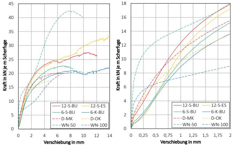
Bild 5-11 Last-Verformungskurven aller Reihen für gesamten Lastbereich (links) und für Anfangslastbereich (rechts)
