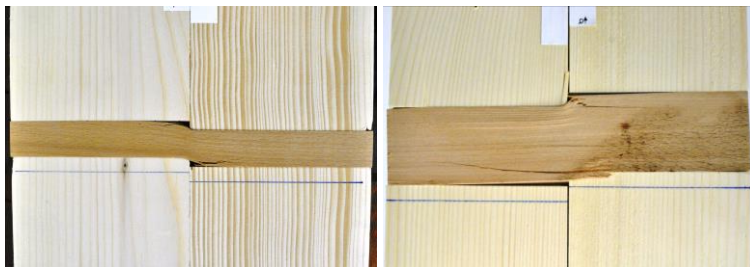
Bild 4-11 Biegezugrisse und Druckfalten im Prüfkörper für Reihe 4-1 (links) und Reihe 4-2 (rechts) und Schiefstellung der Leiste (rechts)
