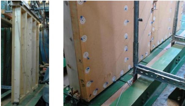
Bild 2-4 Wandtafel mit Holzfaserdämmplatte als Beplankung; Quelle: Gebhardt (2012)
