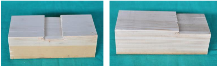
Bild 6-18 Prüfkörper nach Versuchsdurchführung
