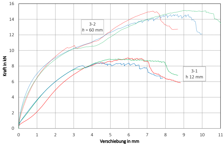
Bild 4-21 Vergleich der Dübeldurchmesser (Biegedübel) für NKL 1
