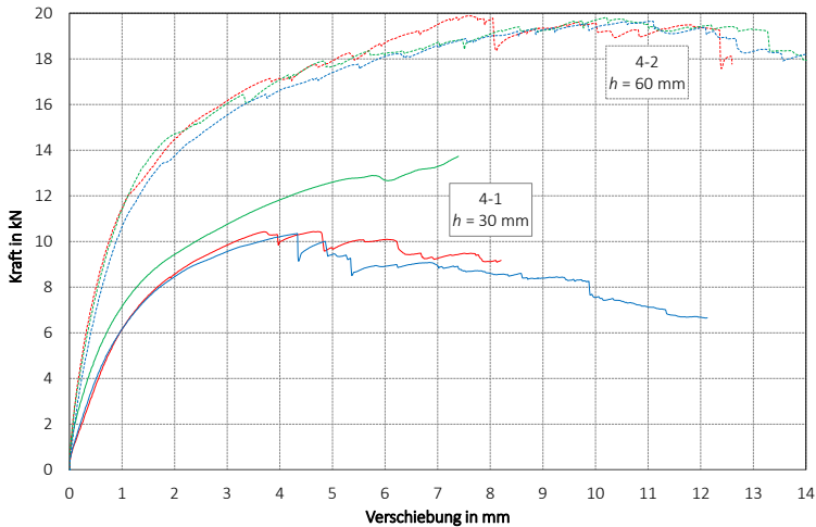
Bild 4-22 Vergleich der Bucheleistenhöhe für NKL 1
