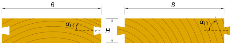
Bild 3-1 Brettquerschnitte mit dem definierten Winkel der Jahringe \alpha_{JR}
