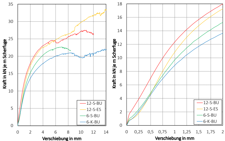
Bild 5-15 Last-Verformungskurven der Reihen mit Leistenverbindungen für gesamten Lastbereich (links) und für Anfangslastbereich (rechts)
