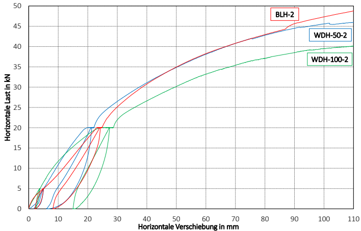
Bild 7-13 Vergleich Wandtafeln mit Bucheleistenverbindungen und Buchedübel-/Wellennagelverbindungen
