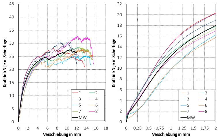
Bild A-20 Last-Verformungsdiagramme Reihe12-S-BU
