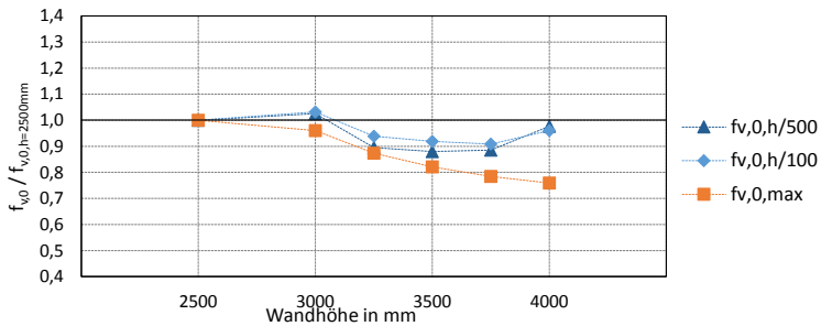
Bild 8-41 Schubflüsse der Modelle DZ in Abhängigkeit der Wandhöhe
