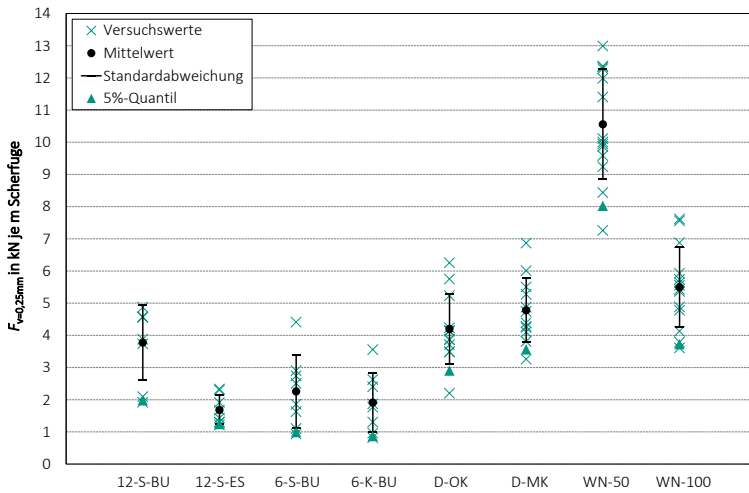
Bild 5-14 Versuchswerte und statistische Kennwerte der Last F_{v=0,25mm}
