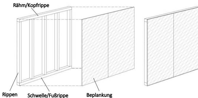
Bild 1-2 Prinzipische Skizze eines möglichen Plattenaufbaus
