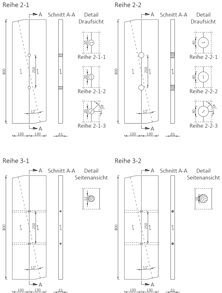
Bild 4-5 Prüfkörpergeometrie und Details für die Reihen 2 und 3
