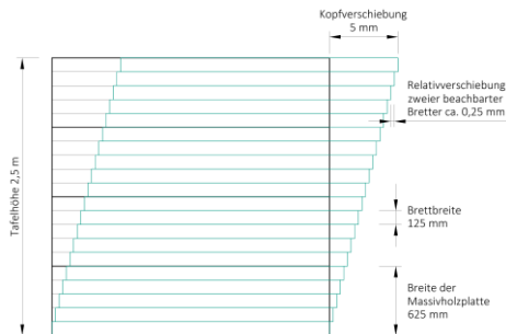
Bild 5-10 Prinzipskizze zur Definition des Ergebniswerts F_{V=0,25\text{mm}}
