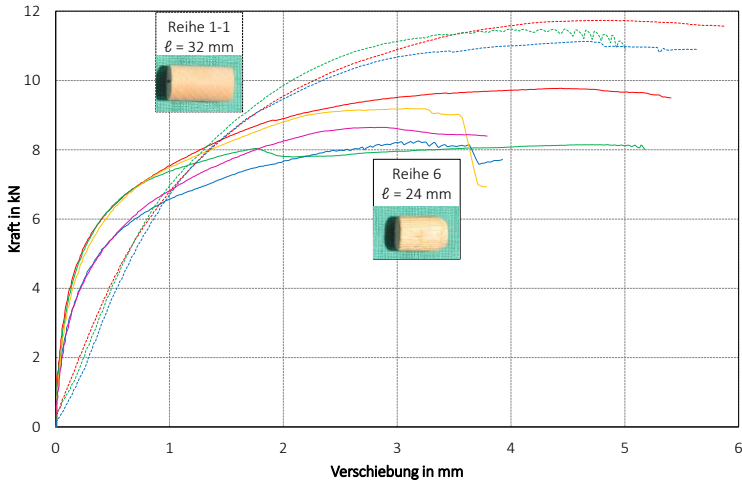
Bild 4-20 Vergleich der Einbindtiefe (Scherdübel) für NKL 1
