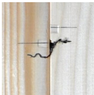
Bild 5-9 Herausgezogener Wellennagel mit Lochleibungsverformung im rechten Holz
