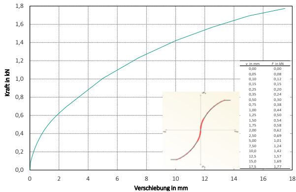
Bild 8-11 Last-Verschiebungskurve für einen Rillennagel mit einer Bezugsrohddichte von 420 \text{ kg/m}^3 und Arbeitsdiagramm für positive und negative Belastung
