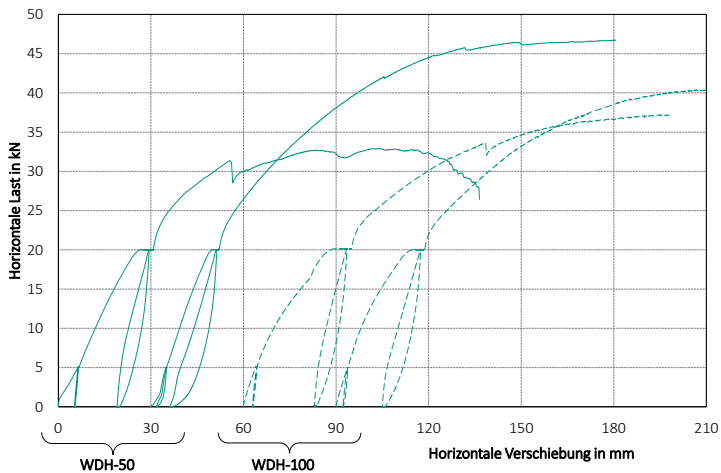
Bild A-43 Last-Verformungsdiagramme Reihe WDH
