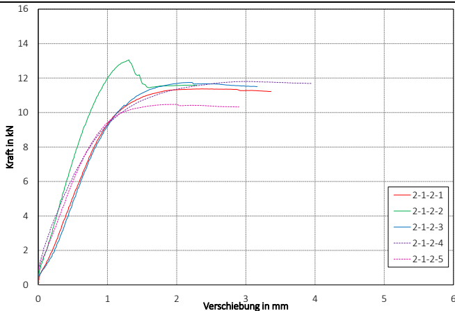
Bild A-7 Last-Verformungsdiagramm Reihe 2-1-2
