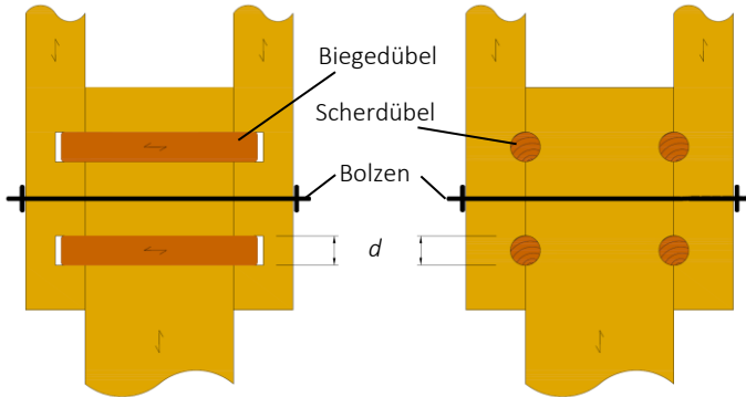
Bild 4-1 Holzverbindungen nach der CABRÖL-Bauweise mit Biegedübeln und Scherdübeln
