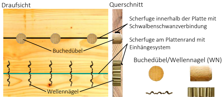
Bild 5-2 Schematische Darstellung eines Ausschnitts der Beplankung mit Buchedübel- und Wellennagelverbindungen und Detail Buchedübel und Wellennägel
