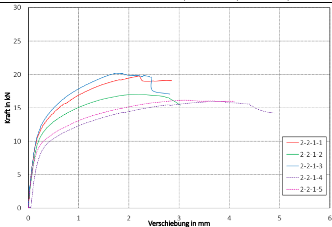
Bild A-9 Last-Verformungsdiagramm Reihe 2-2-1
