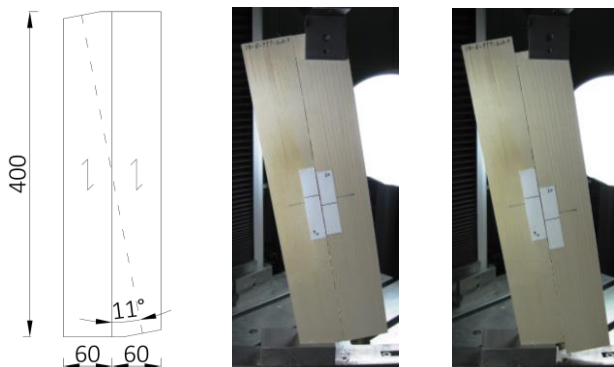
Bild 3-4 Geometrie und Versuchsaufbau vor und nach Versuchsdurchführung; Maße in mm
