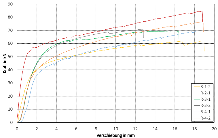
Bild A-41 Last-Verformungsdiagramme Reihe R
