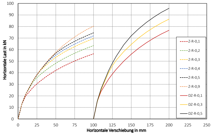
Bild 8-24 Last-Verformungsdiagramme bei Variation des Reibungskoeffizienten ( R )
