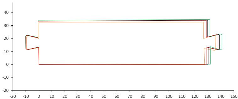
Bild 3-2 Brettquerschnitt PFT-1 bei unterschiedlichen Klimabedingungen (20°C-65 % schwarz; 20°C-85 % grün; 20°C-25 % rot; darrocken orange); Maße in mm
