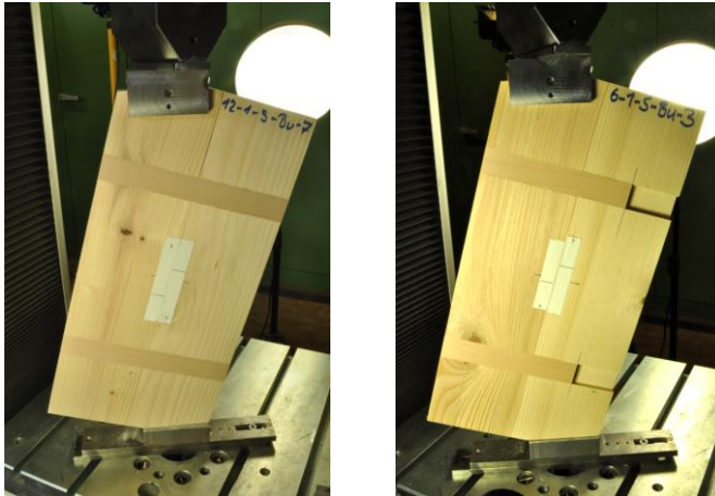
Bild 5-5 Prüfstand für Leistenverbindungen mit 120 mm Einbindetiefe (links) und 60 mm Einbindetiefe (rechts)
