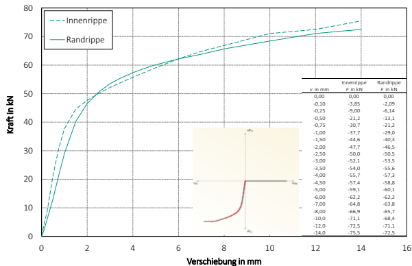
Bild 8-13 Last-Verschiebungskurven bei Belastung auf Querdruck mit einer Bezugsrohddichte von 420 kg/m 3 und Arbeitsdiagramm für positive und negative Belastung
