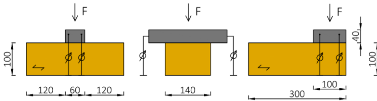
Bild 6-16 Prüfkörpergeometrie für Konfiguration der Innenrippen (links), Hirnholzansicht (Mitte) und für Konfiguration der Randrippen (rechts); Maße in mm
