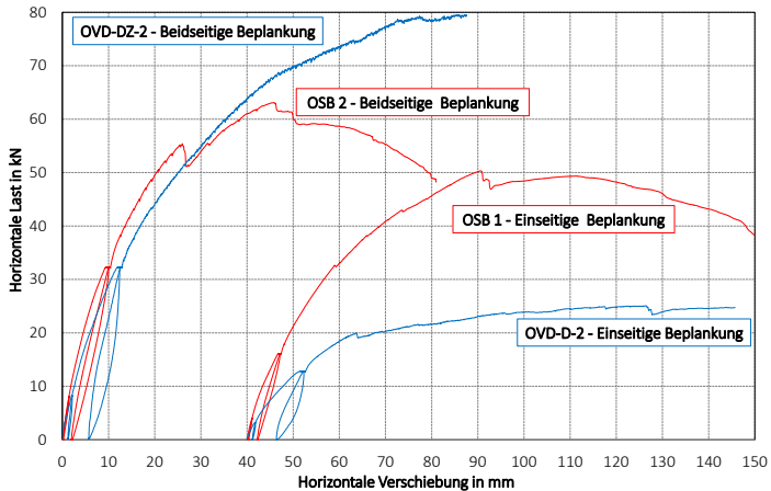
Bild 7-15 Vergleich Wandtafeln mit diagonal verlegeten Massivholzplatten und OSB-Beplankung
