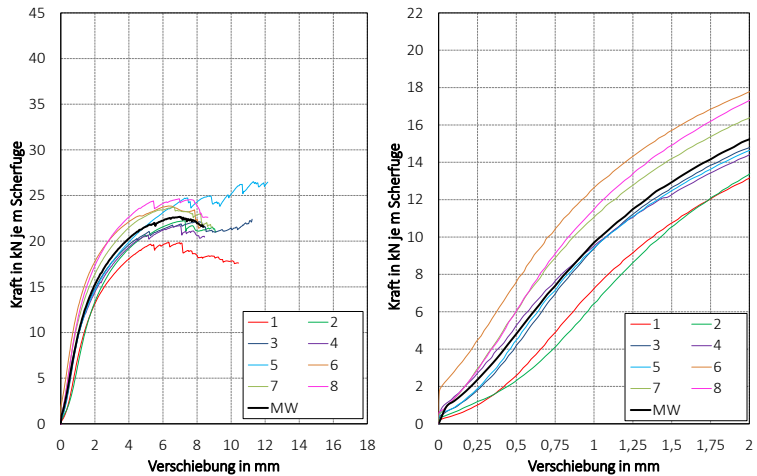
Bild A-22 Last-Verformungsdiagramme Reihe6-S-BU
