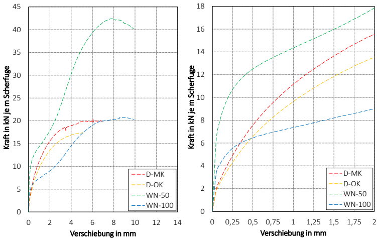
Bild 5-16 Last-Verformungskurven der Reihen mit Dübel- und Wellennagelverbindungen für gesamten Lastbereich (links) und für Anfangslastbereich (rechts)
