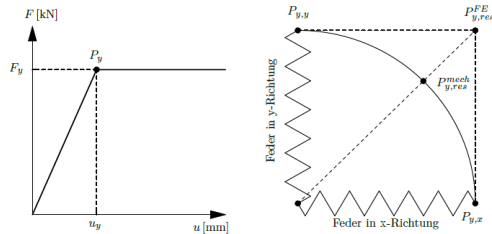
Bild 8-3 Bilineares Materialgesetz (links) und resultierende Beanspruchung (rechts) bei global ausgerichteten karthesischen Federpaaren; Quelle: Vogt (2015)
