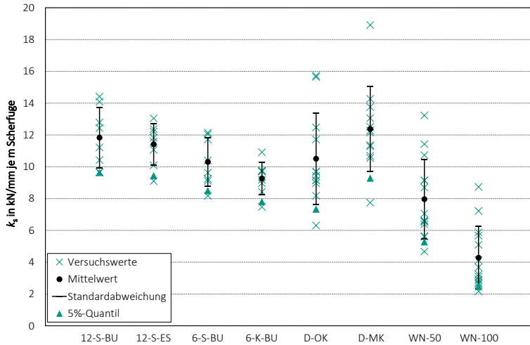
Bild 5-12 Versuchswerte und statistische Kennwerte des Verschiebungsmoduls k_s
