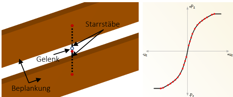
Bild 8-7 Modellierung der Verbindungen (links) und nichtlineares Federgesetz (rechts) am Beispiel einer Verbindung von zwei Brettern der Beplankung
