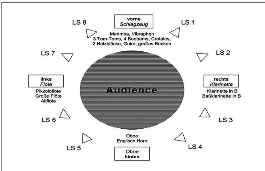
TopoSonic Lines n'Rooms with Instruments , 2002: Für ihre Klanginstallationen visualisierte das Künstlerpaar <Sabine Schäfer // Joachim Krebs> als Vorbereitung schematisch das Verhältnis von Raum und Zuhörschaft. Zu sehen ist hier eine Skizze für den Aufbau des 12-gliedrigen konzertanten RaumKlangKörpers für das ›museum mobile‹ des AUDI-Forums in Ingolstadt.
