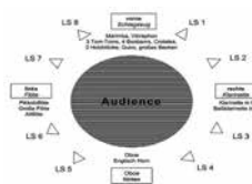
S. 168 TopoSonic Lines n' Rooms with Instruments , 2002: Für ihre Klanginstallationen visualisierte das Künstlerpaar <Sabine Schäfer // Joachim Krebs> als Vorbereitung schematisch das Verhältnis von Raum und Zuhörerschaft. Zu sehen ist hier eine Skizze für den Aufbau des 12-gliedrigen konzertanten RaumKlangKörpers für das ›museum mobile‹ des AUDI-Forums in Ingolstadt. Quelle: Problemkreise(S) 11 (2005).
