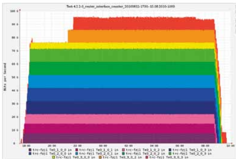
Abbildung 2: TCP-Durchsatz FZJ -> KIT, 11 TCP-Datenströme.
