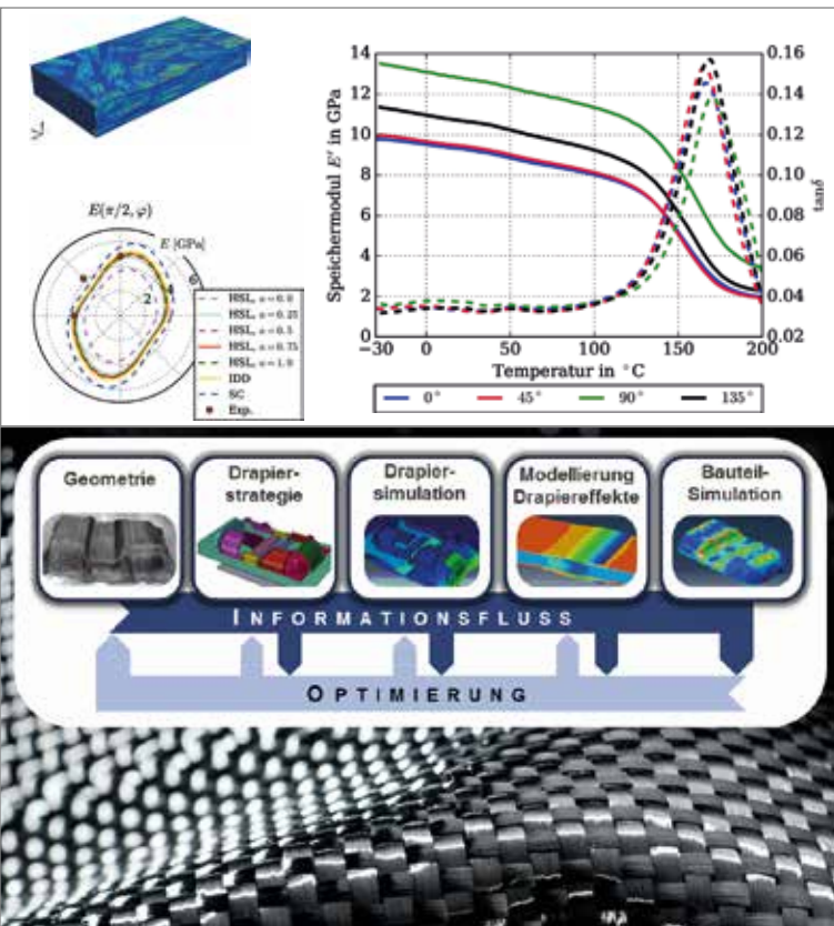
Abb.: Vorgehensweise bei der simulationsbasierten Optimierung von Fertigungsprozess und Bauteiltragfähigkeit
