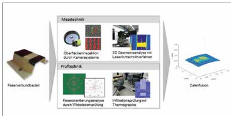
Abb.: Einbindung von in-line Mess- und Prüftechniken für Faserverbundbauteile am Institut für Produktionstechnik (wbk)
