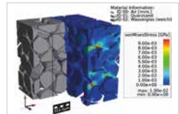
Abb.: Mikrostruktur und zugehörige Spannungsverteilung eines Sandkerns, bestehend aus Quarzsandkörnern und anorganischem Binder
