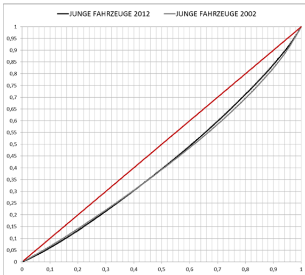
Abbildung 27: Lorenzkurven des Flottenverbrauchs 2012 und 2002 für Neuwagen bis 3 Jahre.
