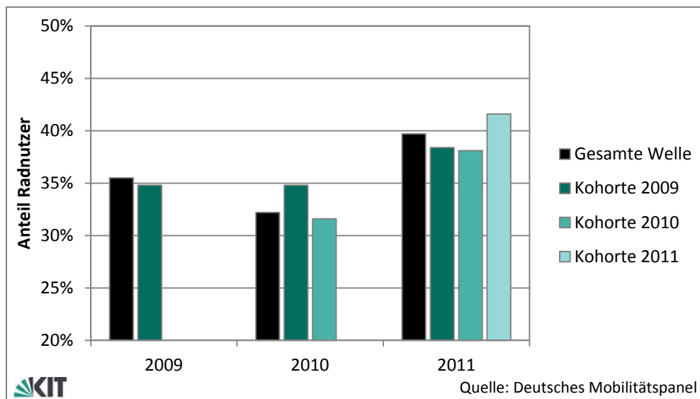
Abbildung 14: Anteil an Radnutzern in den Kohorten 2009, 2010 und 2011 der Jahre 2009 bis 2011.
