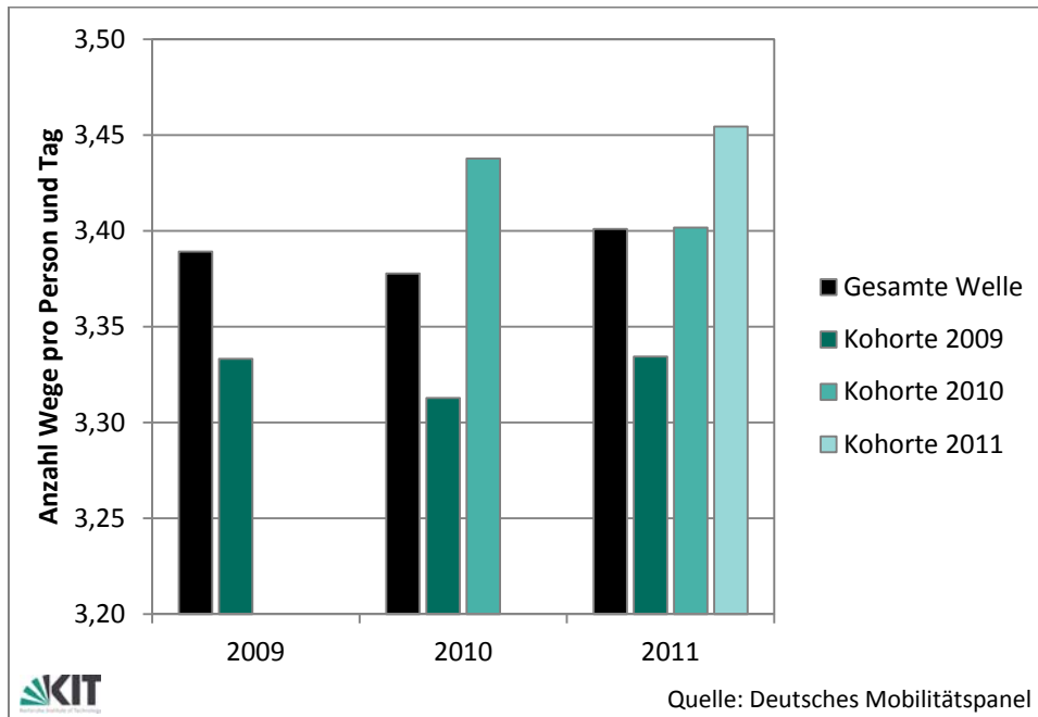
Abbildung 10: Verkehrsaufkommen der Kohorten 2009, 2010 und 2011 in den Jahren 2009 bis 2011.
