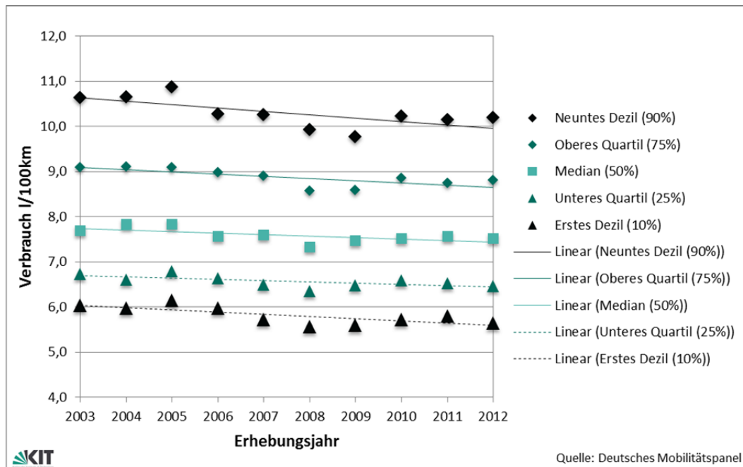
Abbildung 22: Zeitreihe ausgewählter Lagemaße des Flottenverbrauchs (2003-2012).
