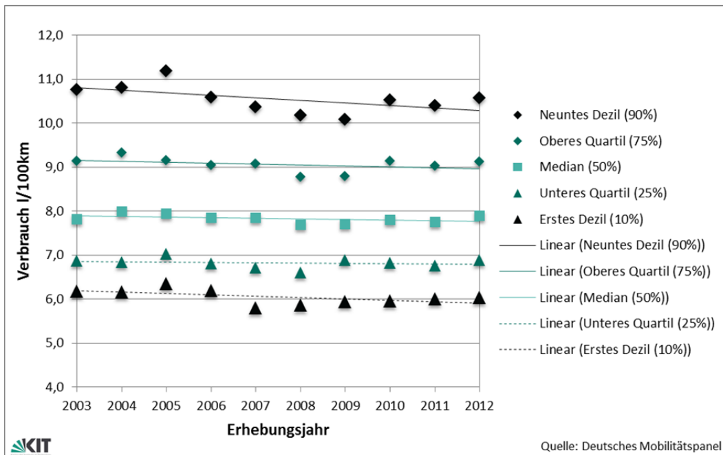
Abbildung 23: Zeitreihe ausgewählter Lagemaße des Flottenverbrauchs von Benzinfahrzeugen (2003-2012).
