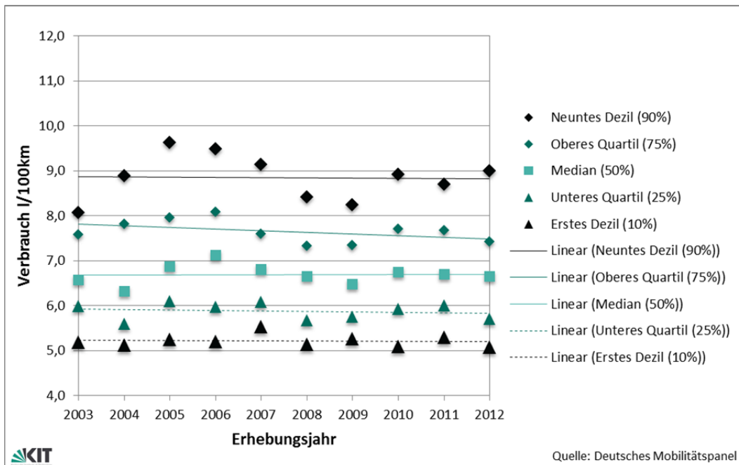
Abbildung 24: Zeitreihe ausgewählter Lagemaße des Flottenverbrauchs von Dieselfahrzeugen (2003-2012).
