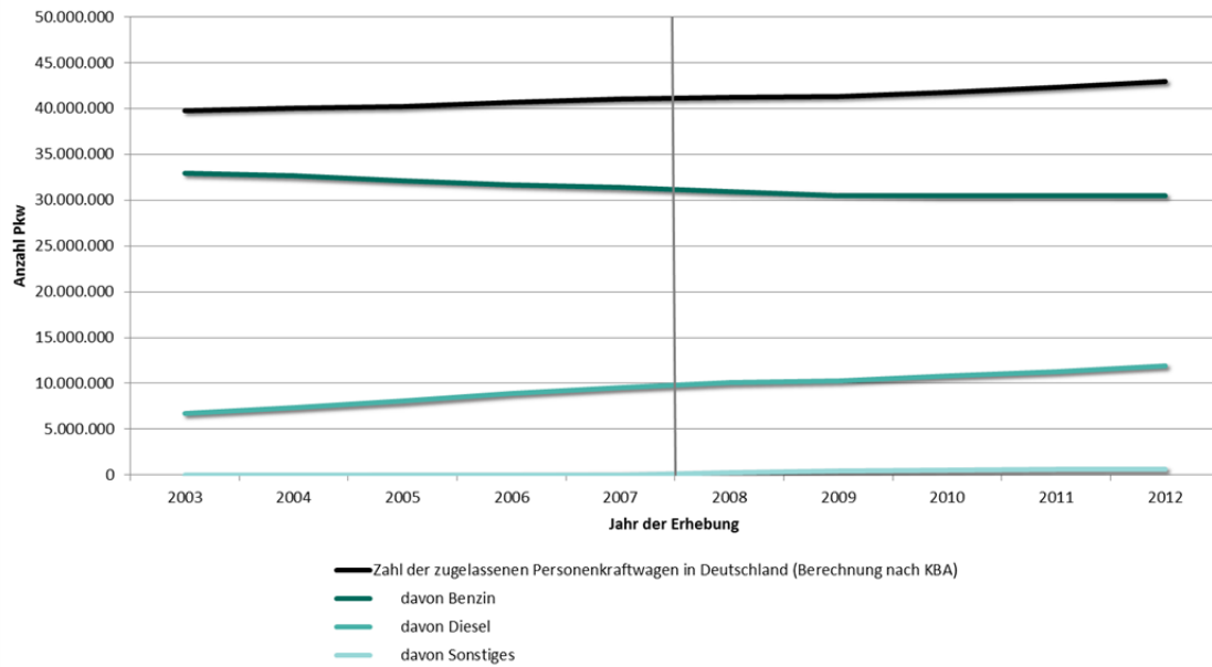
Pkw-Bestand in Deutschland seit dem Jahr 2003 nach Kraftstoffart
