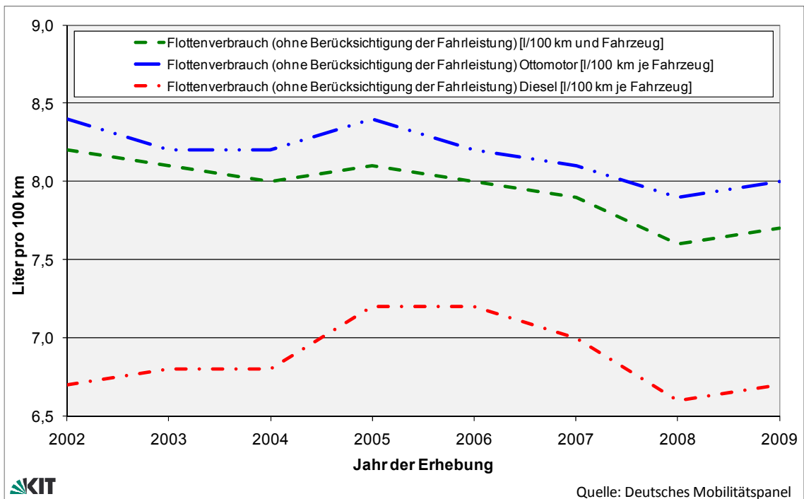
Abbildung 9: Flottenverbrauch seit 2002
