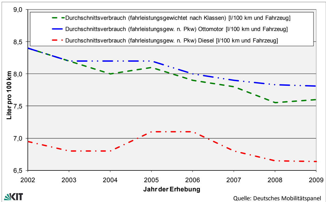
Abbildung 8: Durchschnittsverbrauch seit 2002
