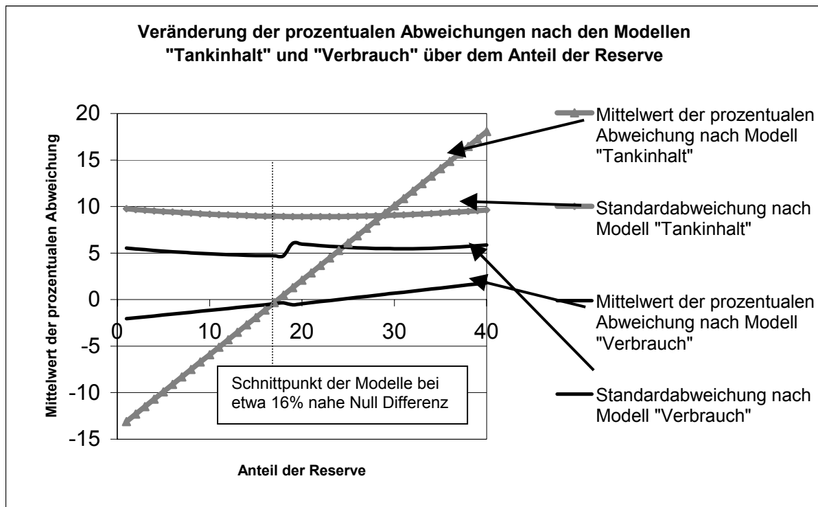
Abbildung 9: Vergleich unterschiedlicher Berechnungsmethoden zur Bestimmung des Reserveanteils am Gesamttankinhalt
