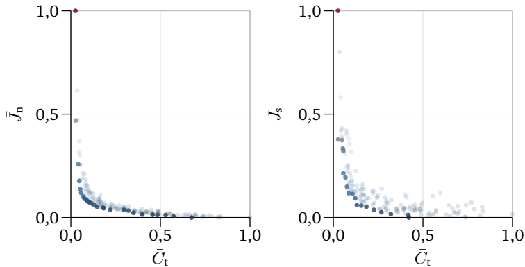
Abbildung 6.14: Vergleich der von verschiedenen Konfigurationen erreichten Planungs- \bar{J}_n und Regelgüte J_s und dem normierten notwendigen Rechenaufwand \bar{C}_t . Pareto-optimale Konfigurationen sind jeweils hervorgehoben.
