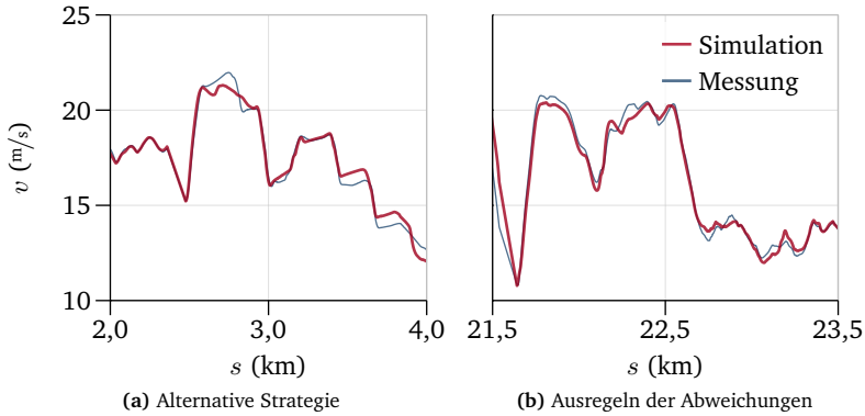
Abbildung 6.5: Unterschiedliche Systemreaktionen auf Abweichungen zwischen Simulation und Messfahrt
