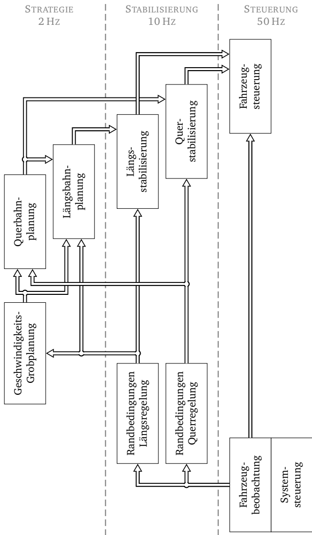
Abbildung 5.3: Softwarearchitektur der vorausschauenden Fahrregelung
