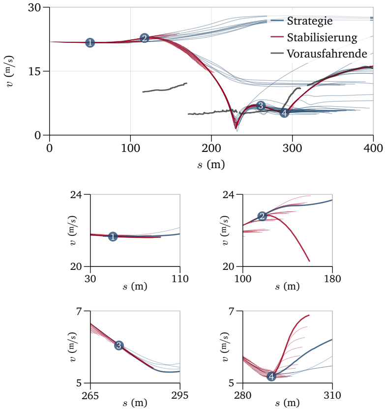
Abbildung 6.23: Strategie- und Stabilisierungsplanung der Längsregelung während einer Überholsituation. In ① und ③ verfolgt die Stabilisierung die Strategie. Unerwartete Änderungen erfordern in ② und ④ ein kurzzeitiges Abweichen der Stabilisierung von der strategischen Vorgabe.
