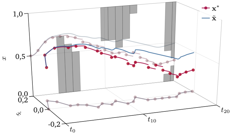
Abbildung 3.6: Vergleich zwischen interpolierter Zustandstrajektorie \mathbf{x}^* und tatsächlichem Zustandsverlauf \tilde{\mathbf{x}} . Durch systematische Rundungsfehler ergeben sich auf dem Planungshorizont erhebliche Abweichungen.
