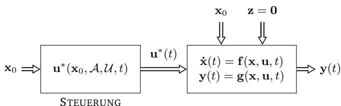
Abbildung 2.2: Optimale Steuerung eines dynamischen Systems
