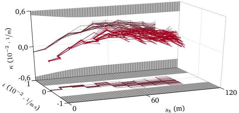
(b) Bahnkrümmung \kappa und Steuergröße \nu . Die Zustands- und Steuerbegrenzungen ergeben sich aus der Fahrzeuggeschwindigkeit v(t) .
