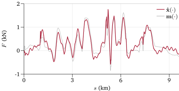
Abbildung 6.17: Vergleich der vom Simulationsmodell \dot{x}(\cdot) und vom Prädiktionsmodell m(\cdot) berechneten Fahrwiderstände F unter dem Einfluss des sinusförmigen Störungsmodells [11]
