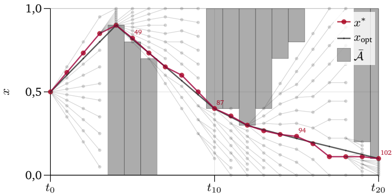
Abbildung 3.3: Umsetzung der Zustandsbeschränkungen \bar{A} durch Einschränken des Diskretisierungsraums. Die berechnete Optimalstrategie nähert sich dem Idealverlauf x_{\text{opt}} an, es werden jedoch weiterhin Zustände berechnet, die zu ungültigen Trajektorien führen.
