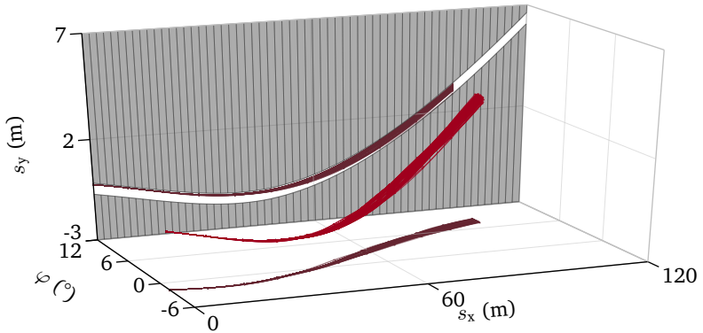
(a) Fahrzeugposition s_y und Bahnrichtung \varphi . Die Zustandsbegrenzungen für \varphi ergeben sich implizit aus dem Fahrbahnverlauf und den Steuergrenzen.
