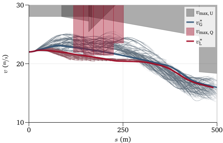
Abbildung 5.4: Ergebnistrajektorien und Suchkandidaten von Geschwindigkeitsgrobplanung ( v_G^* ) und Längsbahnplanung ( v_L^* ). Während v_G^* lediglich die Einschränkungen der Umgebung v_{\max,U} berücksichtigt, werden für v_L^* zusätzlich die der Quereinschränkung v_{\max,Q} betrachtet.
