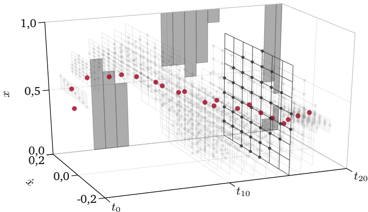
Abbildung 3.5: Dynamische Programmierung mit äquidistanter Zustandsdiskretisierung in jedem Zeitschritt. Der optimale Zustandsknoten jedes Zeitschritts ist hervorgehoben.
