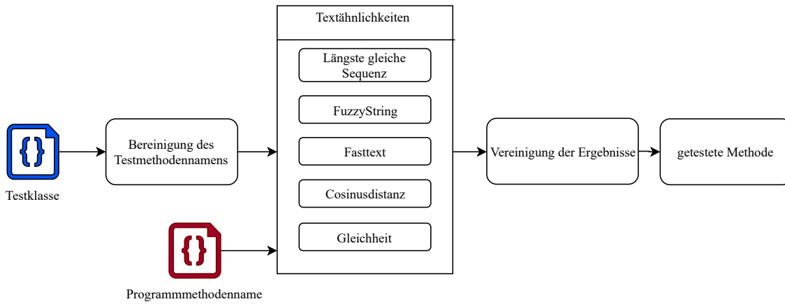
Abbildung 5.4: Verfahren zur Auswertung der Methodennamen einer Testklasse.
