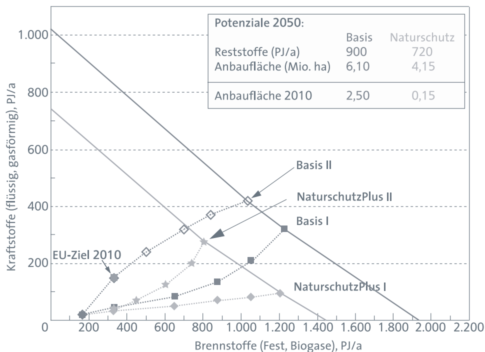
ABB. 18 DARSTELLUNG VON JE ZWEI PFADEN EINER MÖGLICHEN NUTZUNG DER ERMITTELTEN BIOMASSEPOTENZIALE FÜR DIE STATIONÄRE UND MOBILE NUTZUNG IN DEN DLR/IFEU/WI-2004-SZENARIEN BASIS UND NATURSCHUTZPLUS
