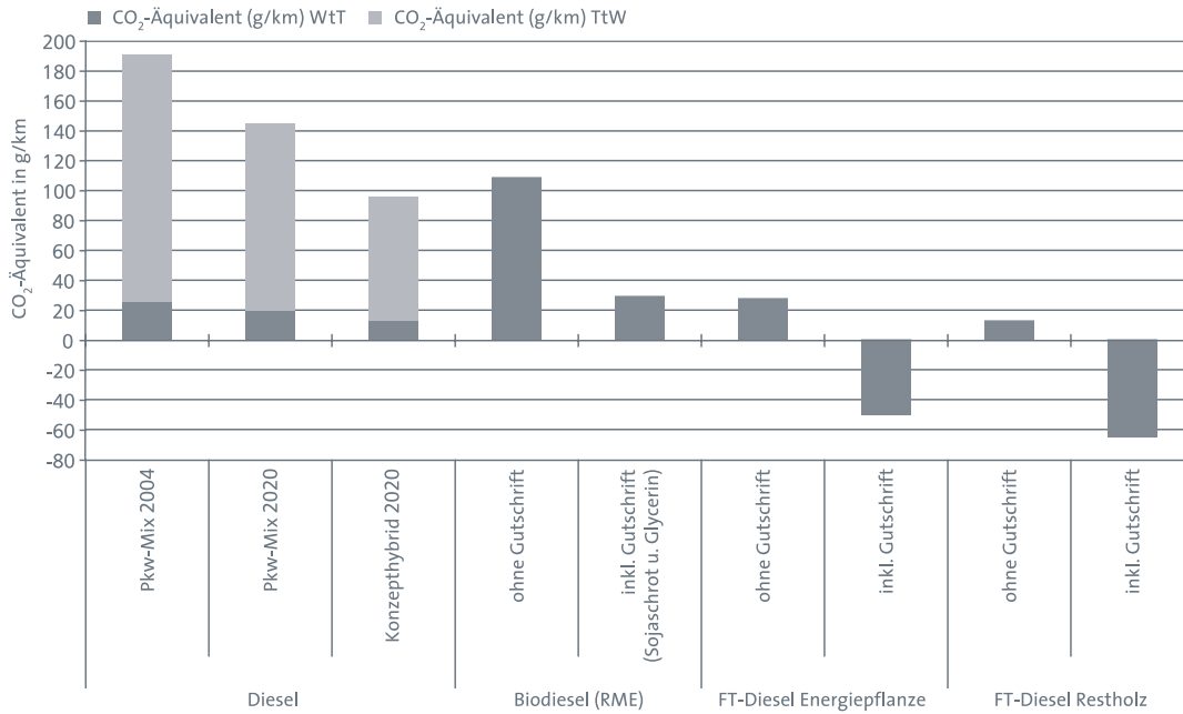
ABB. 12 WTW-DARSTELLUNG FÜR PKW MIT DIESELMOTOR 2020
