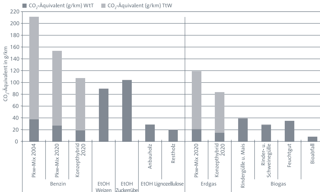
ABB. 13 WTW-DARSTELLUNG FÜR PKW MIT OTTOMOTOR 2020
