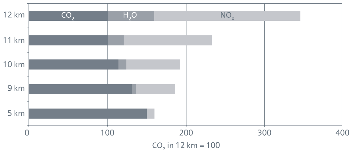
ABB. 3 RELATIVE WIRKUNG BESTIMMTER ABGASE FÜR DEN TREIBHAUSEFFECT IN ABHÄNGIGKEIT VON DER FLUGHÖHE
