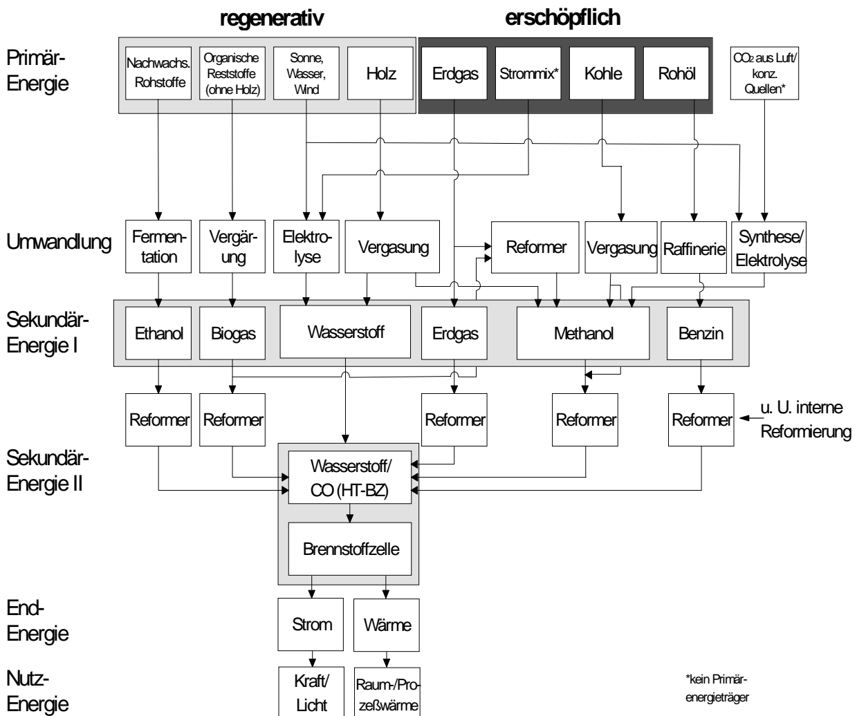
Abb. 6: Brennstoffpfade für Brennstoffzellensysteme
