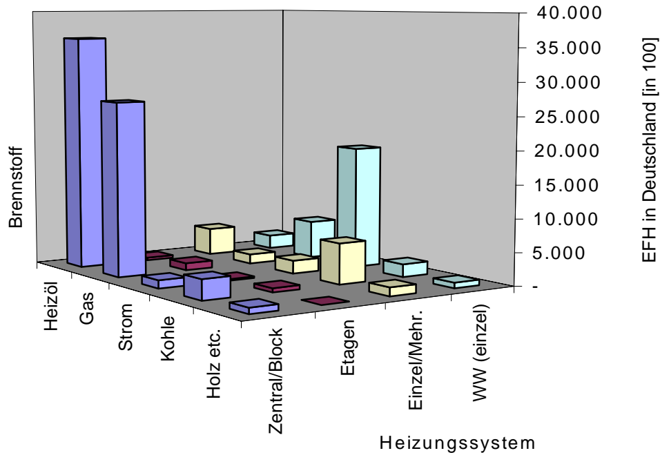
Abb. 24: Installiertes Heizungssystem und eingesetzter Brennstoff in Einfamilienhäusern in Deutschland (Baualterklasse 1991-1993)
