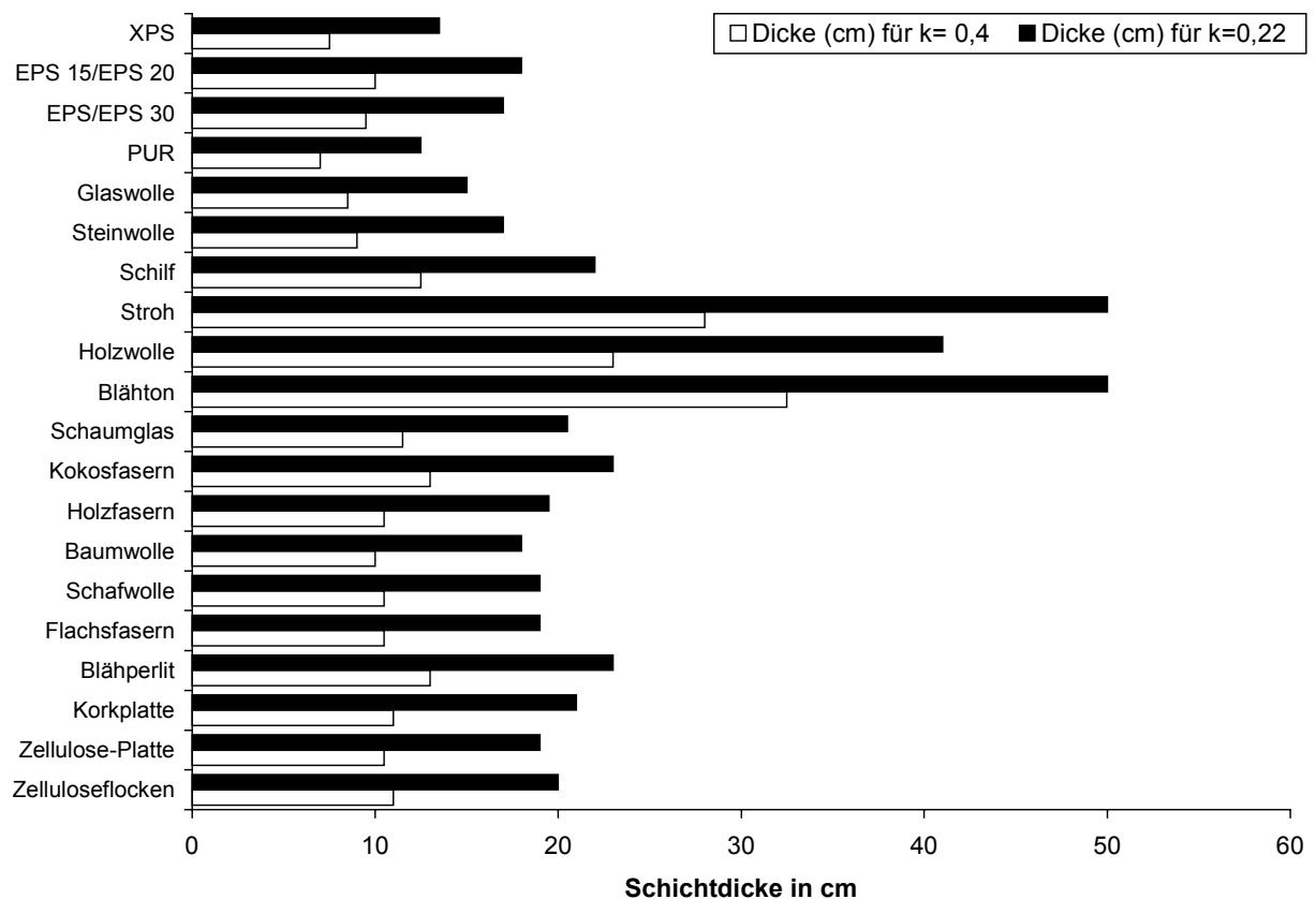
Abb. 3: Schichtdicke der Dämmung zur Erreichung eines k-Wertes von 0,4 bzw. 0,22 W/m 2 K
