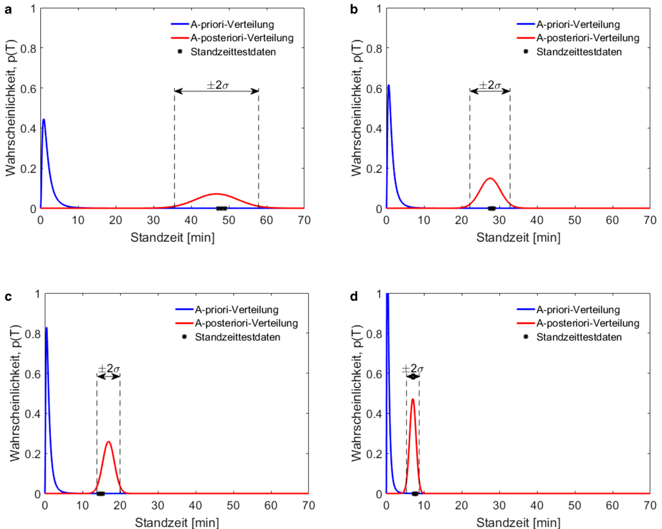
Abb. 10 A-posteriori-Funktionen mit Unsicherheitsintervallen der Standardabweichung von \pm 2\sigma unter Verwendung der Schnittgeschwindigkeiten: a 300, b 325, c 350 und d 400 m/min
