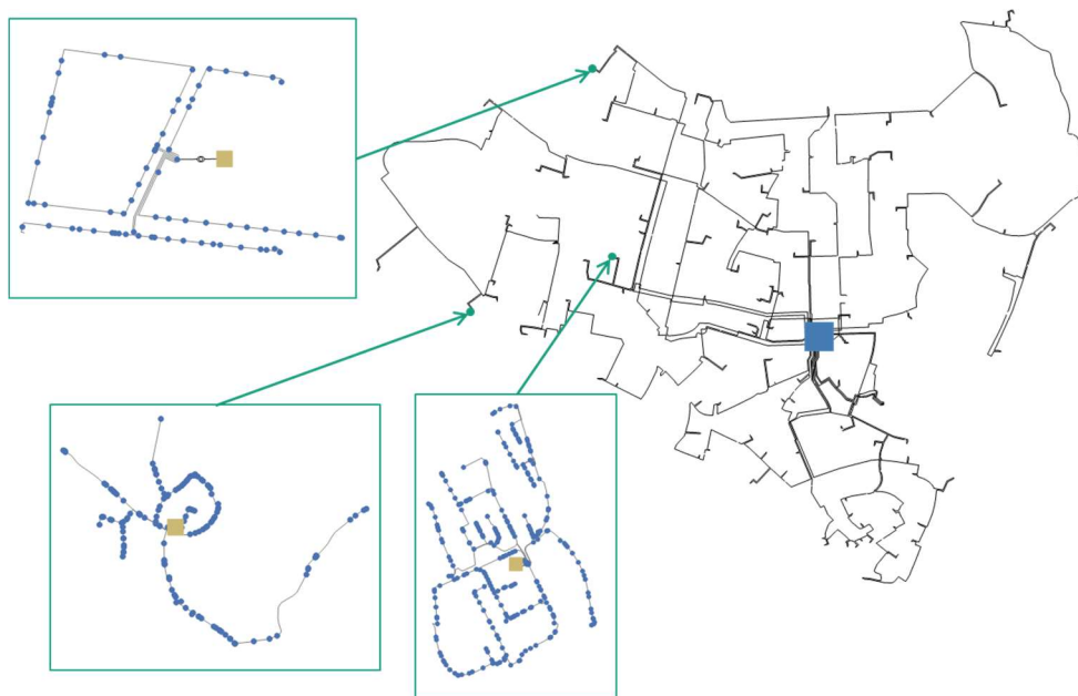
Abbildung 37: Versorgungsknoten-9-Netz mit beispielhaft zugeordneten Niederspannungsnetzen
