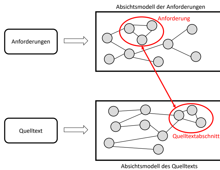
Abbildung 3.1: Veranschaulichung des Lösungsansatzes von INDIRECT
