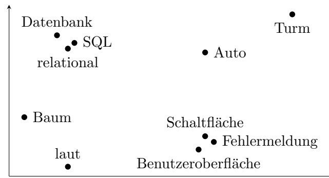
Abbildung 2.2: Schematische Darstellung von Wortembeddings im Vektorraum
