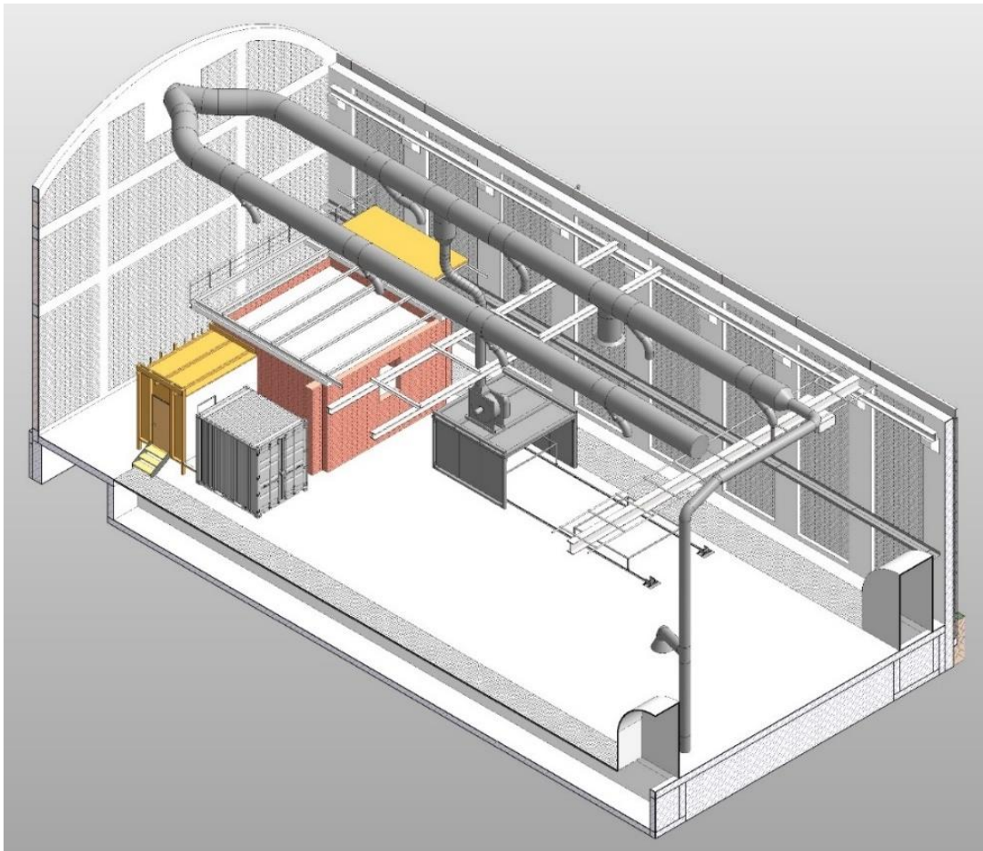
Abb. 21: „Wohnzimmer“ (rot) und Vorraum (gelb mit Treppe) in der Versuchshalle
