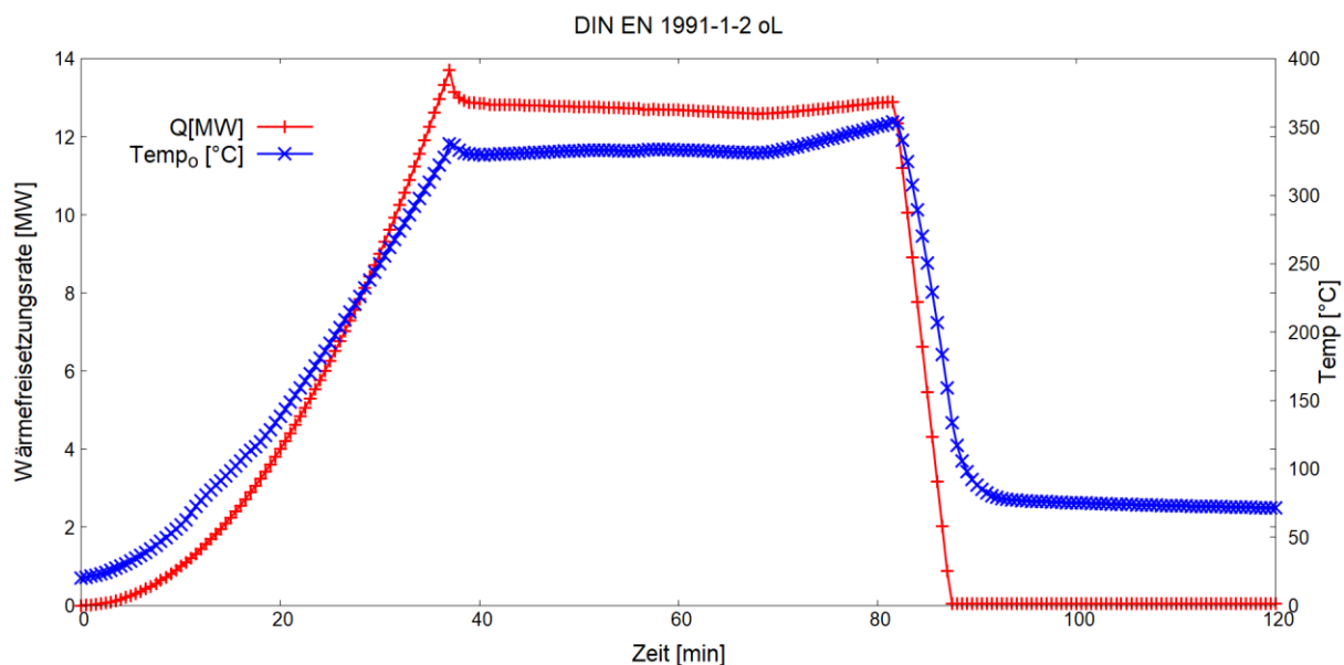
Abbildung 16 Ergebnisse-Verlauf der Wärmefreisetzungsrates und der Heißgastemperatur für das Szenario oL
