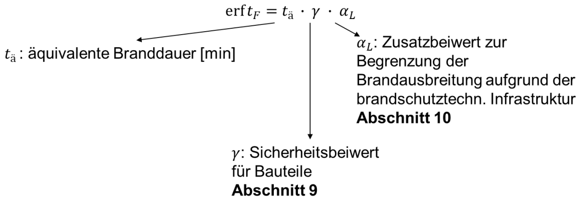
Abbildung 7 Bestimmung der erforderlichen Feuerwiderstandsdauer erft_F nach DIN 182301 und den Einflussgrößen und deren Abschnitten der DIN 18230-1 [5]
