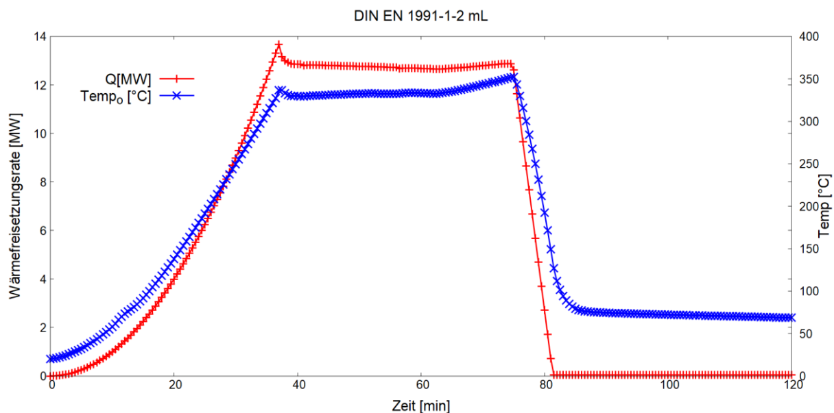
Abbildung 17 Ergebnisse-Verlauf der Wärmefreisetzungsrates und der Heißgastemperatur für das Szenario mL
