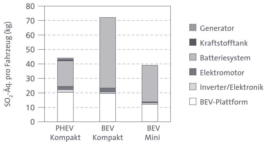
ABB. III.3 VERSAUERUNGSPOTENZIAL BEI DER FAHRZEUGHERSTELLUNG
