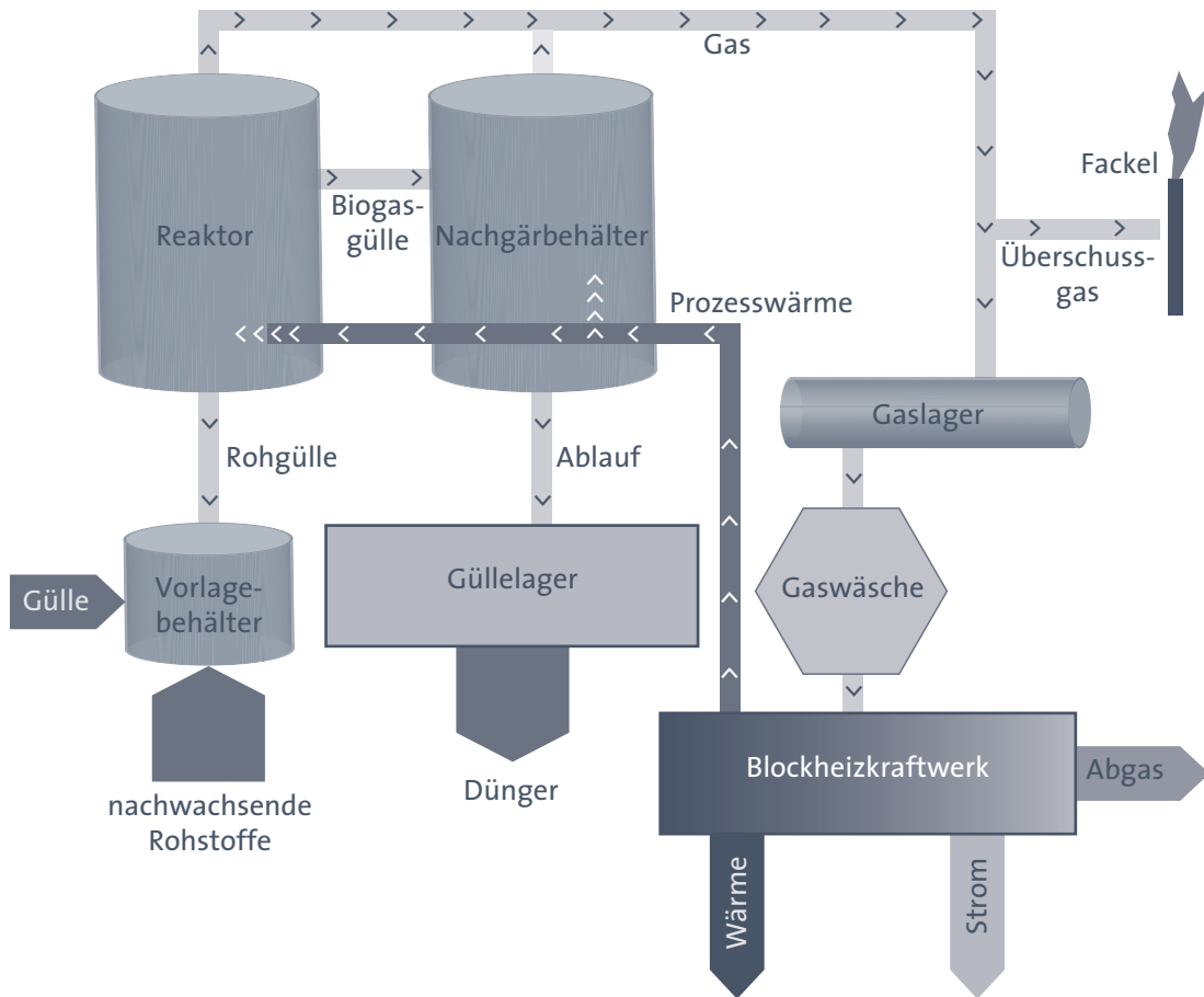
ABB. IV.8 SCHEMATISCHER AUFBAU EINES BIOGASBLOCKHEIZKRAFTWERKS
