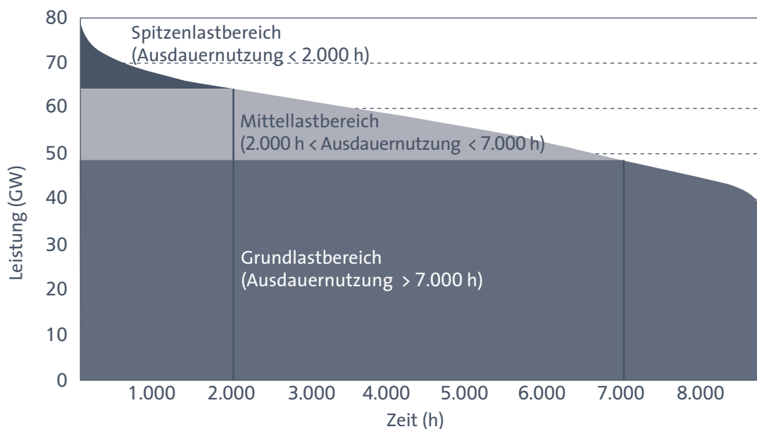
ABB. II.6 VERDEUTLICHUNG DER LASTSEGMENTE ANHAND EINER JAHRESDAUERLINIE
