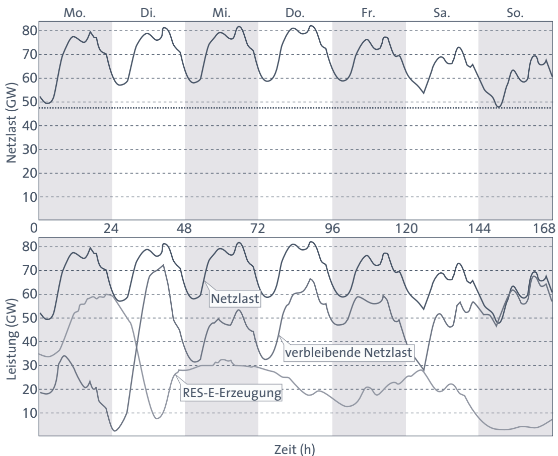
ABB. II.9 OBEN: NETZLAST IM TYPISCHEN WOCHENVERLAUF; UNTEN: RESIDUALLAST NACH ABZUG DER RES-E-ERZEUGUNG
