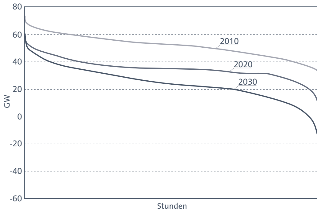
ABB. V.6 RESIDUALLAST MIT FLEXIBILISIERUNGSOPTIONEN FÜR DIE JAHRE 2010 BIS 2030
