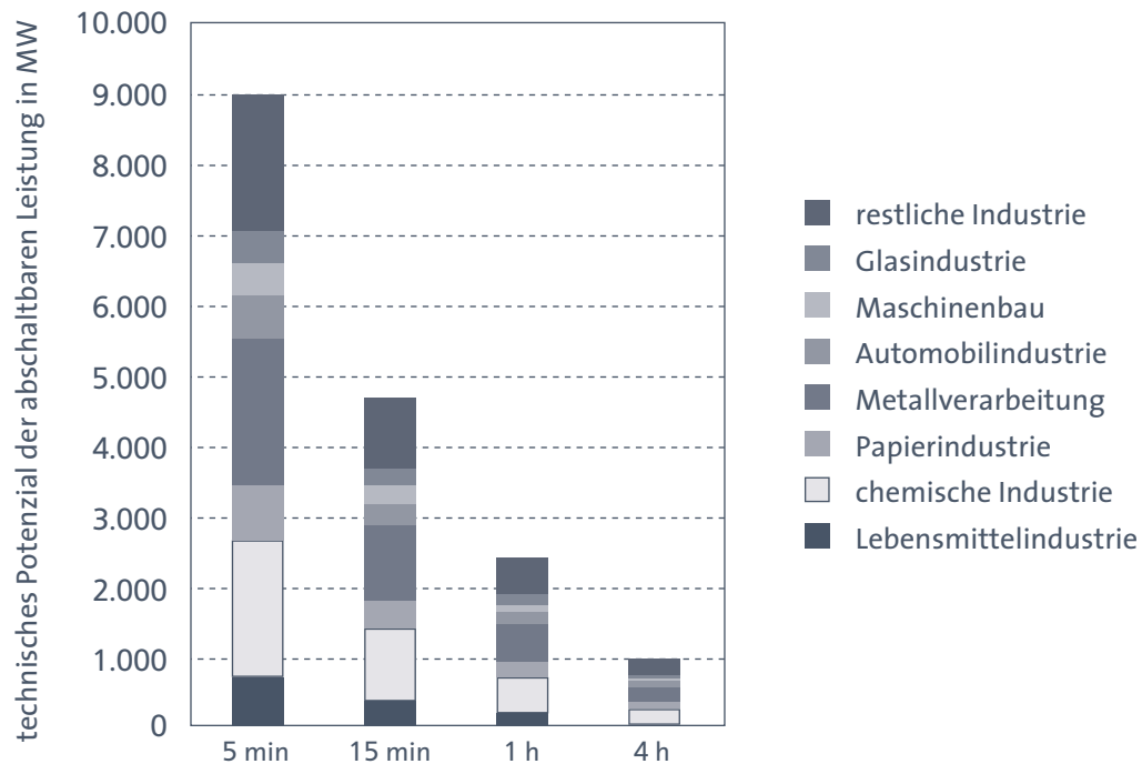
ABB. IV.12 TECHNISCHES POTENZIAL VON LASTMANAGEMENT VERSCHIEDENER BRANCHEN IN ABHÄNGIGKEIT DER ABSCHALTZEIT
