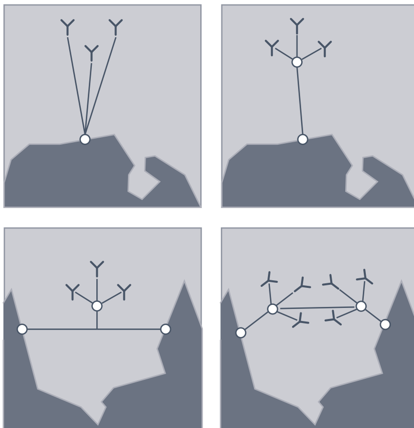
ABB. III.5 MÖGLICHKEITEN ZUR NETZANBINDUNG VON OFFSHOREWINDPARKS
