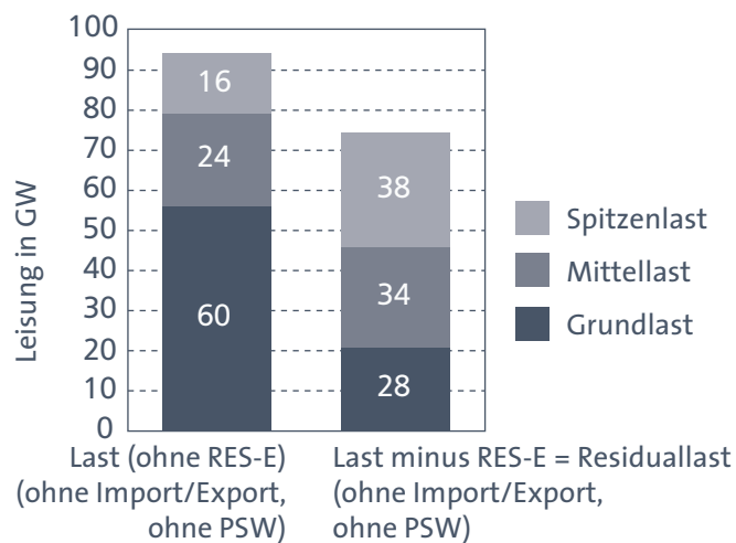
ABB. II.10 BEDARF AN GRUND-, MITTEL-, UND SPITZENLAST MIT UND OHNE RES-E-EINSPESUNG IN % (2020)
