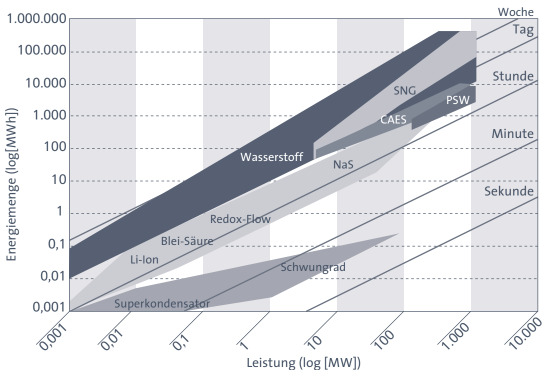
ABB. IV.1 EINSATZBEREICHE VERSCHIEDENER SPEICHERTECHNOLOGIEN
