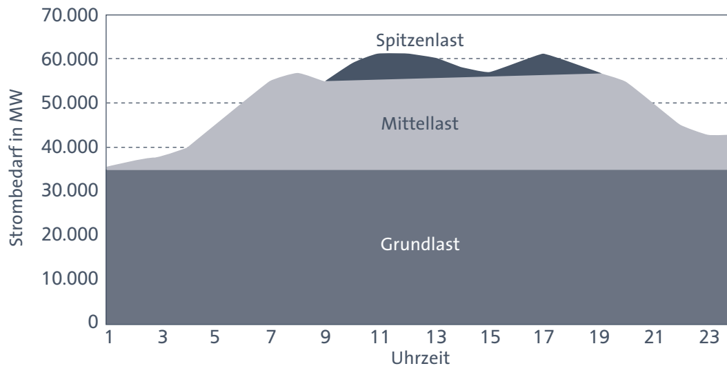
ABB. II.5 ÜBLICHE EINTEILUNG DES STROMBEDARFS IN LASTSEGMENTE
