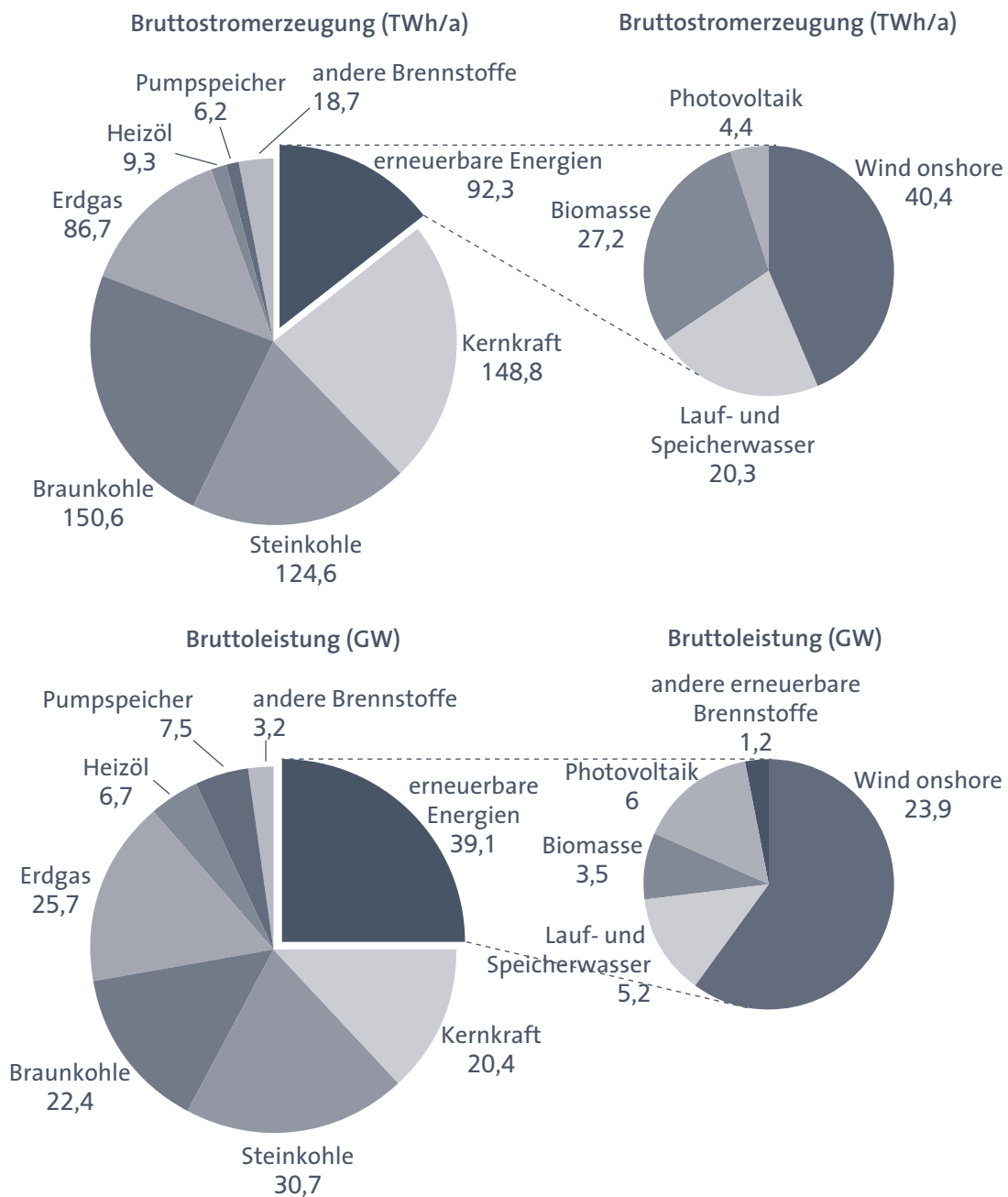
ABB. II.1 STRUKTUR DER STROMERZEUGUNG UND INSTALLIERTEN KRAFTWERKSLEISTUNG IM JAHR 2008
