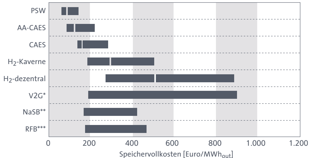
ABB. IV.5 KOSTENVERGLEICH ZWISCHEN VERSCHIEDENEN STROMSPEICHERTECHNOLOGIEN (TÄGLICHER ZYKLUS)
