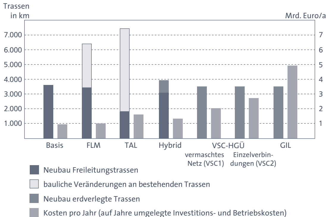
ABB. III.1 DENA-NETZSTUDIE II: NETZAUSBAUVARIANTEN UND KOSTEN
