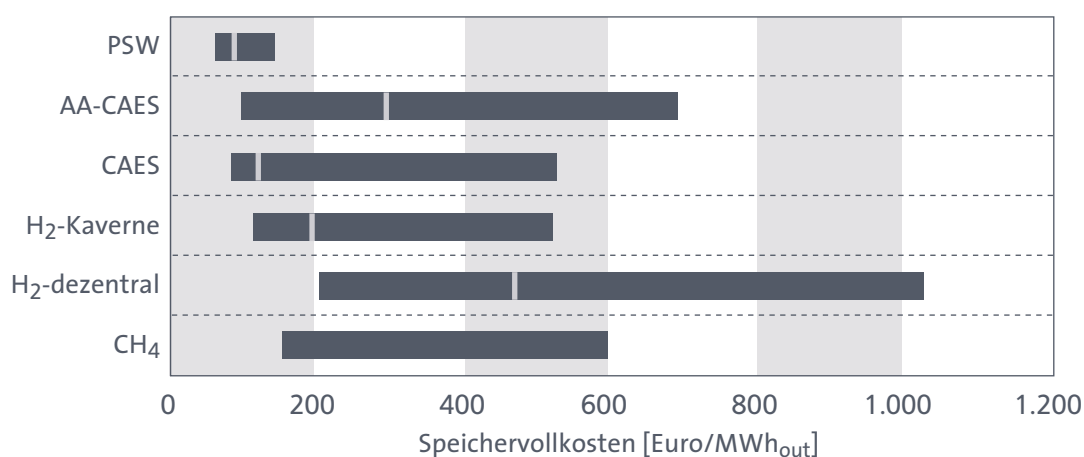
ABB. IV.4 KOSTENVERGLEICH ZWISCHEN VERSCHIEDENEN STROMSPEICHERTECHNOLOGIEN (WÖCHENTLICHER ZYKLUS)
