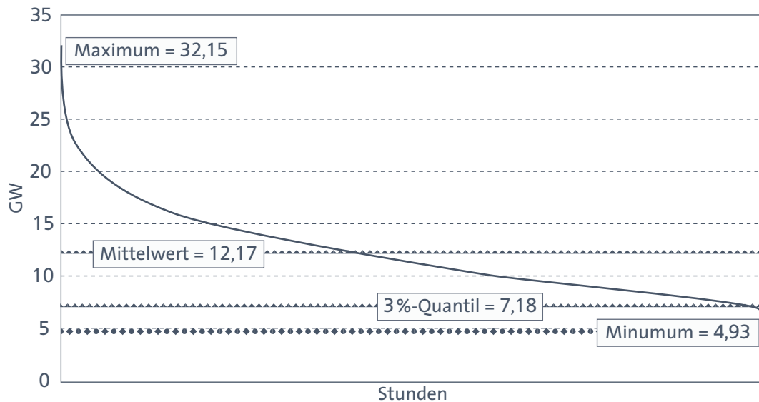
ABB. V.1 DAUERLINIE DER RES-E-EINSPEISUNG 2010
