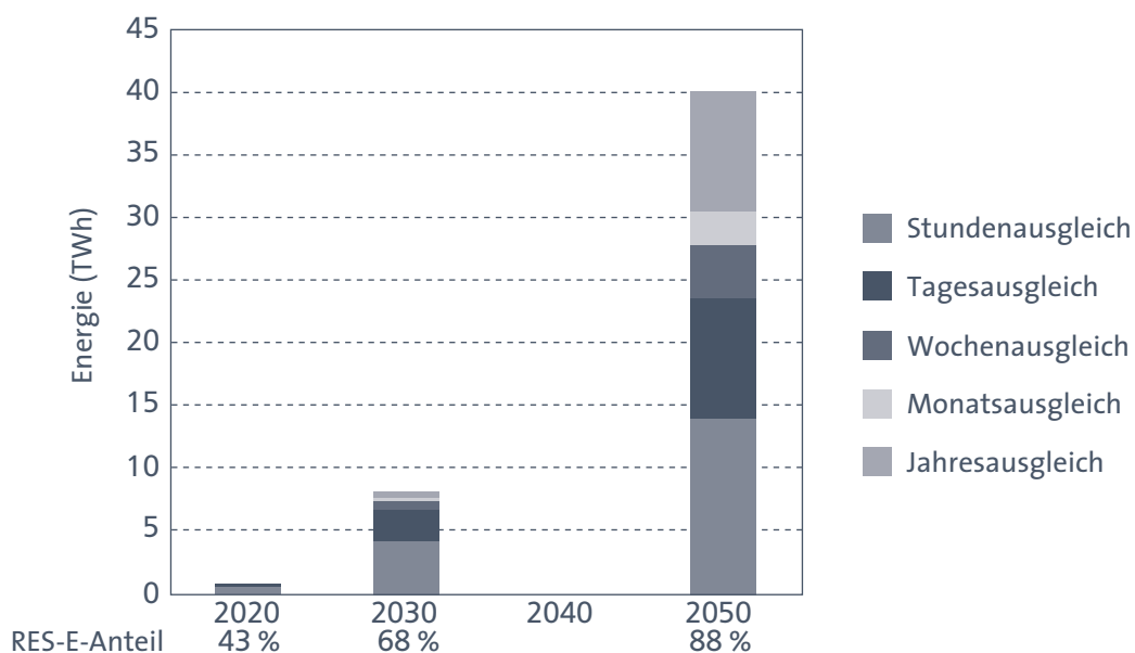
ABB. IV.2 SPEICHERBEDARF IN DEUTSCHLAND BIS 2050
