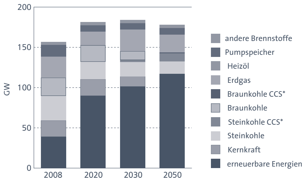
ABB. II.3 INSTALLIERTE KRAFTWERKSLEISTUNG IM PROGNOSES/EWI/GWS-SZENARIO IIA
