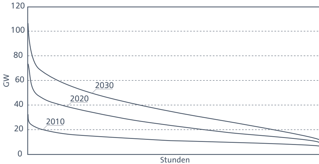
ABB. V.3 DAUERLINIE DER RES-E-EINSPEISUNG BIS 2030
