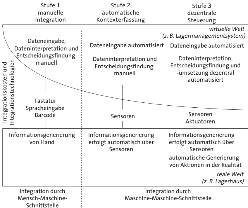
ABB. 18 INTEGRATION VON REALER UND VIRTUELLER WELT
