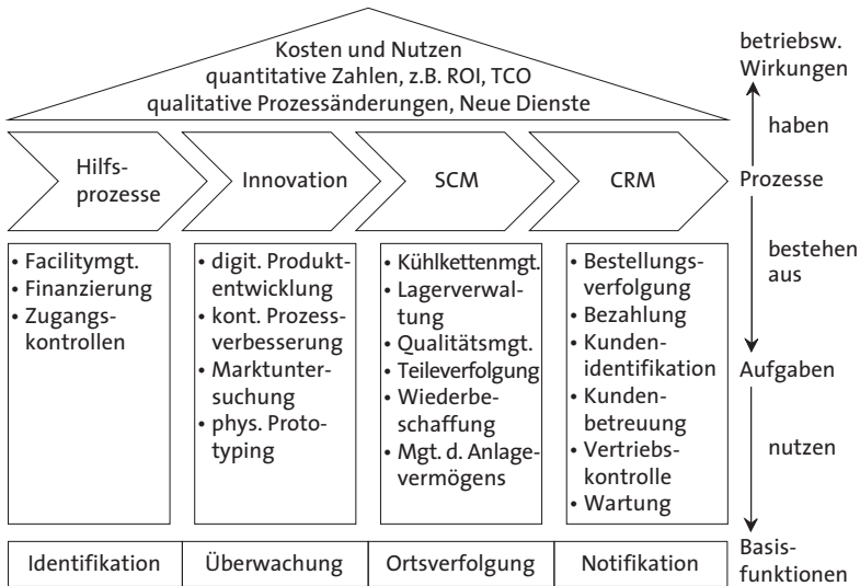
ABB. 14 MODELL ZUR PROZESSUNTERSTÜTZUNG DURCH UBIQUITÄRES COMPUTING IM UNTERNEHMEN
