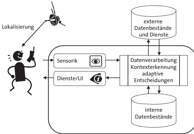
ELEMENTE EINES UBICOMP-SYSTEMS
