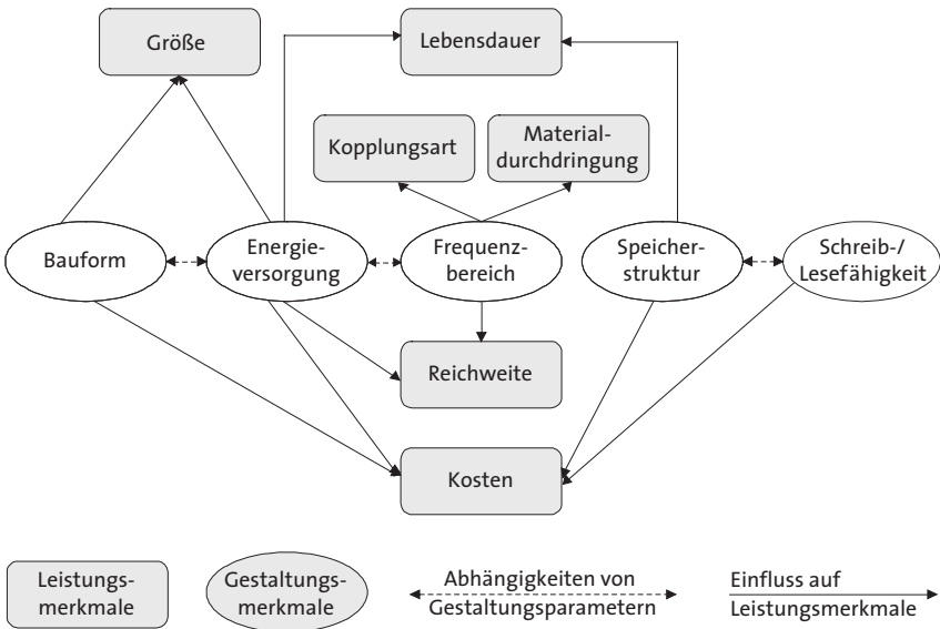
ABB. 11 GESTALTUNGS- UND LEISTUNGSMERKMALE EINES TRANSPONDERS
