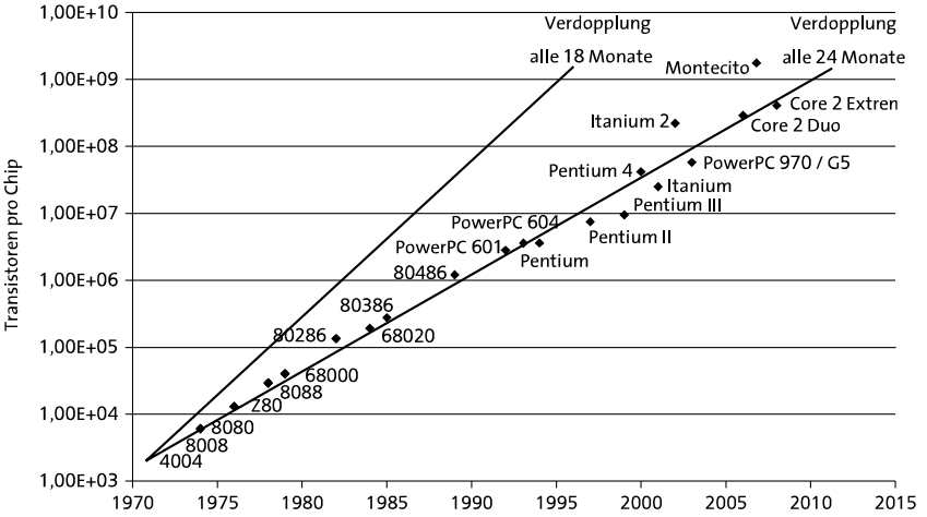
ABB. 4 MOORES GESETZ (AM BEISPIEL VON MIKROPROZESSOREN)
